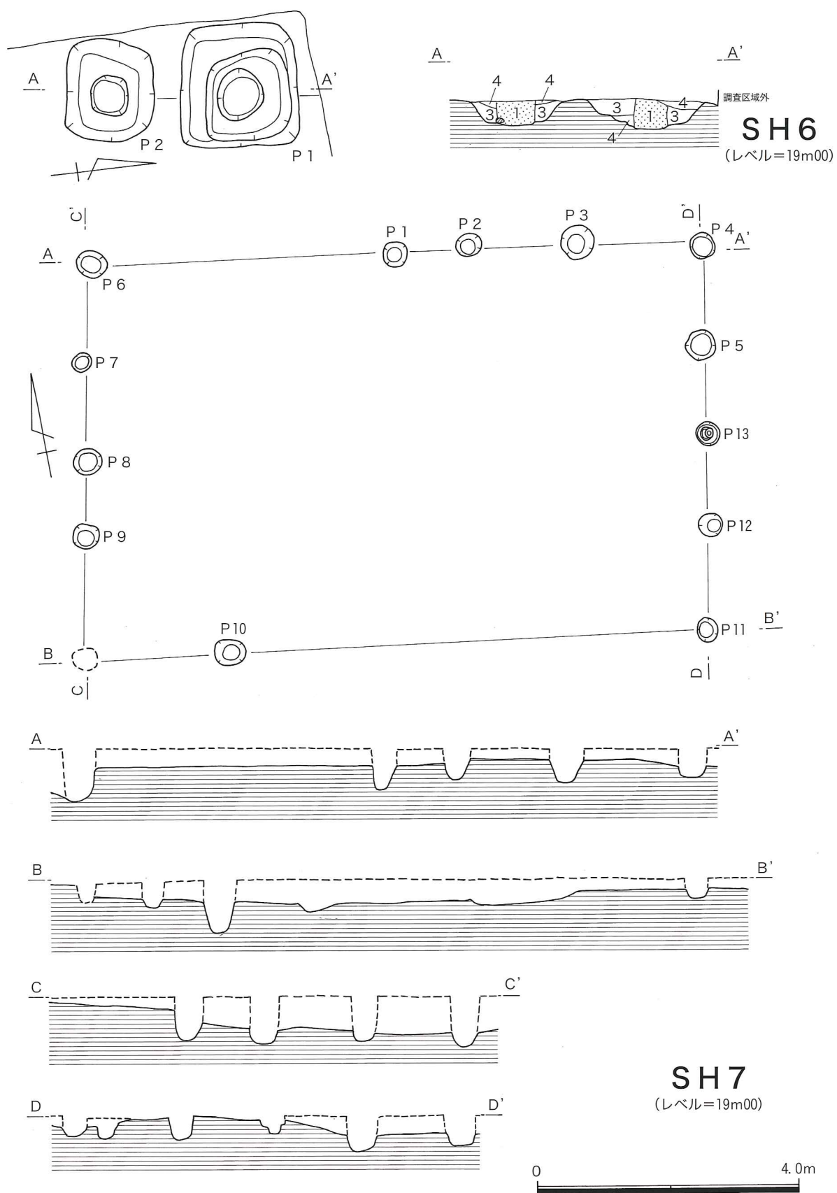
第9図 SH6・7 実測図
