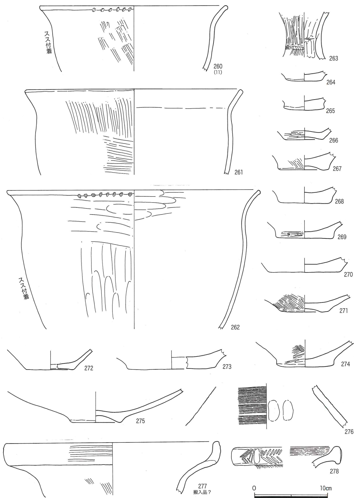
第40図 土器実測図13
