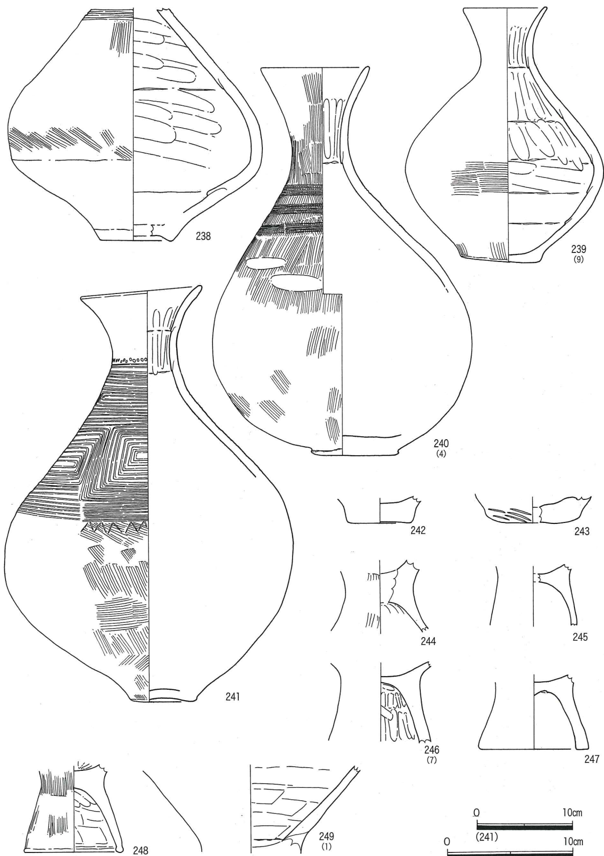
第38図 土器実測図11
