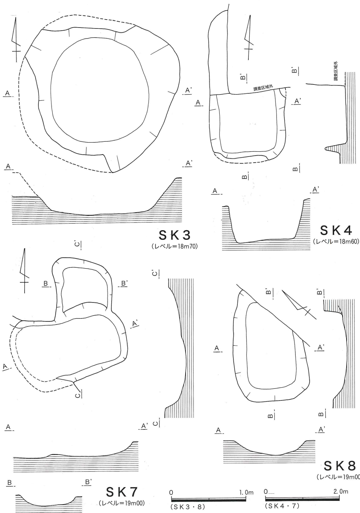
第25図 SK 3・4・7・8 実測図
