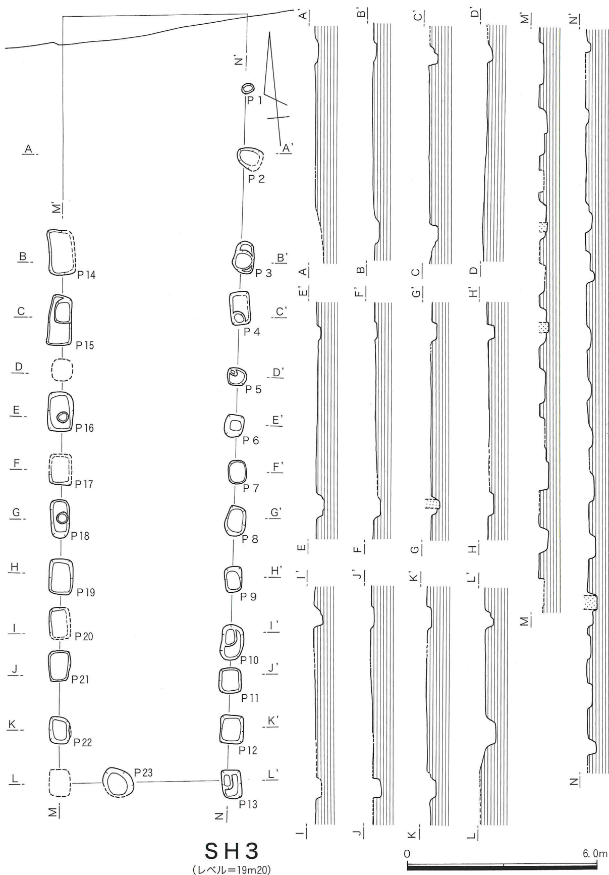
第7図 SH3 実測図
