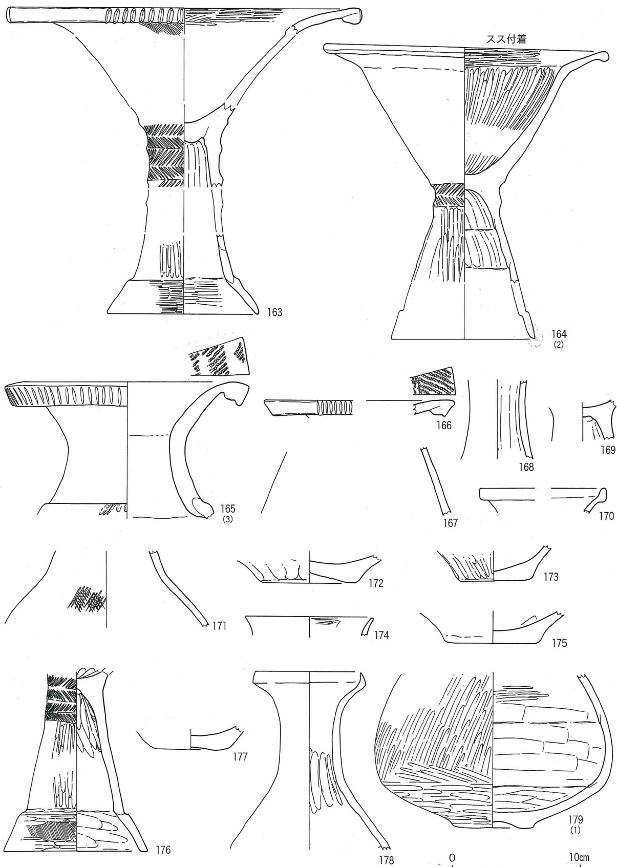
第34図 土器実測図7
