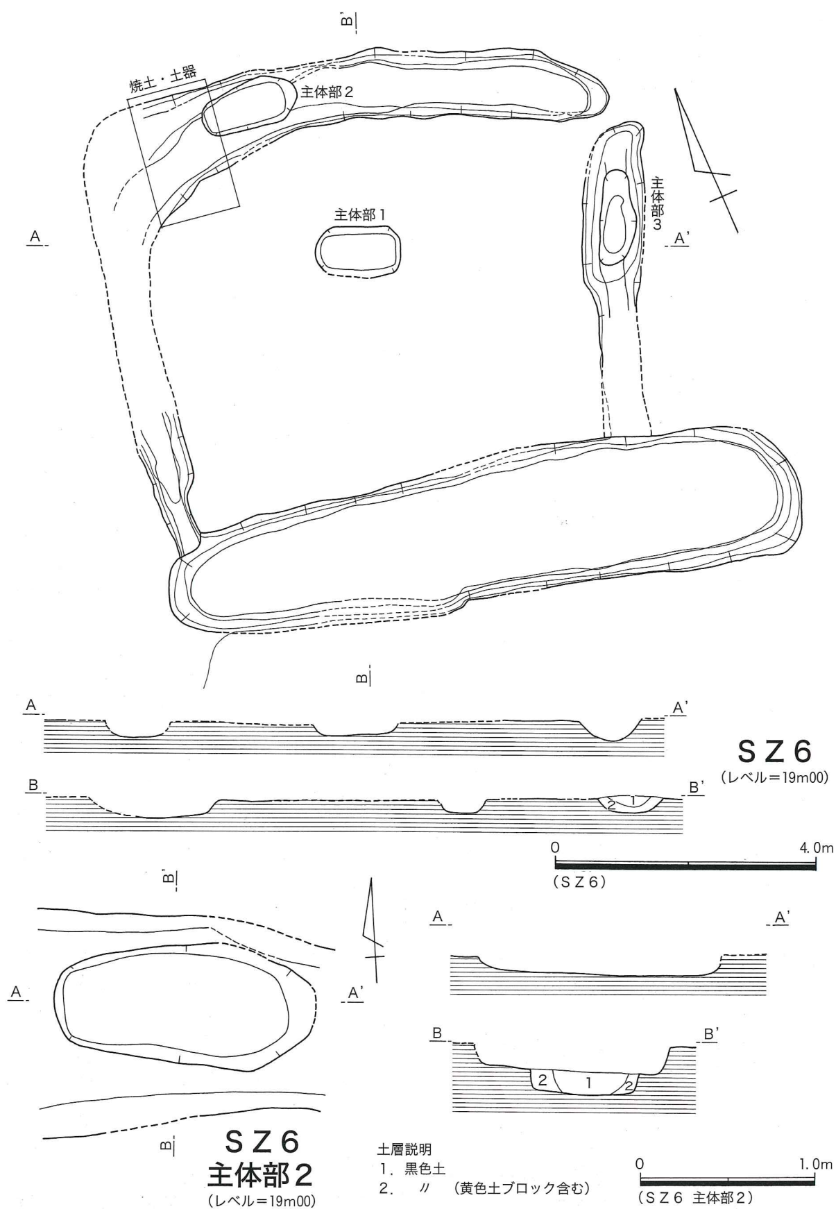
第20図 SZ 6・SZ 6主体部 2 実測図
