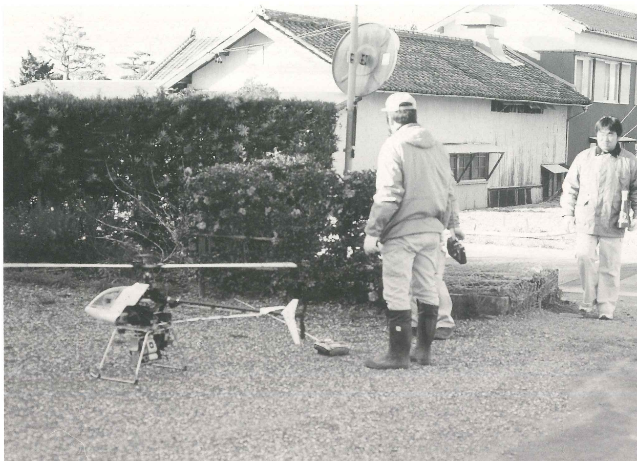
(1) 空中写真測量のためのラジコンヘリコプター
