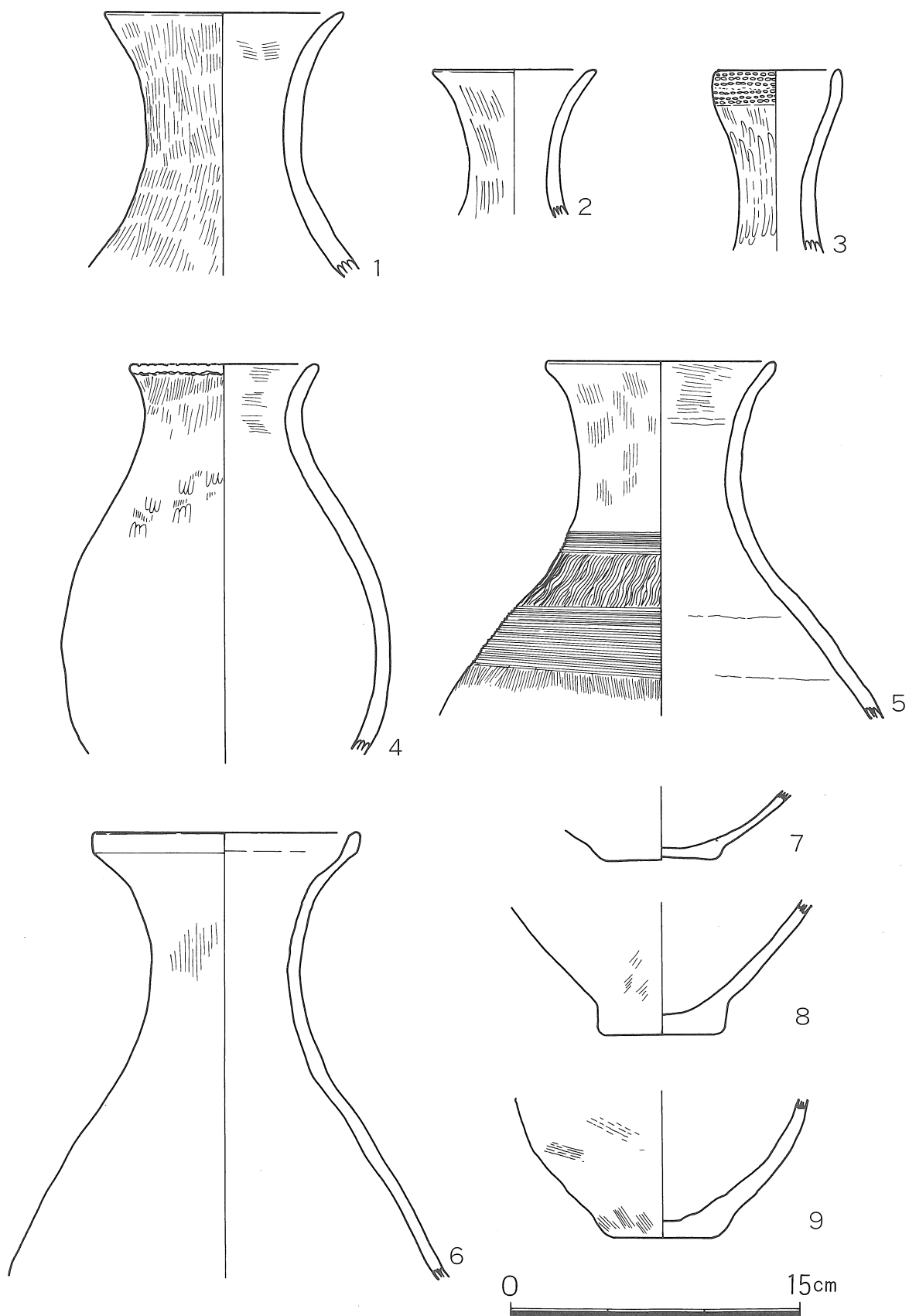
第8図 溝跡030 出土土器実測図(1)
