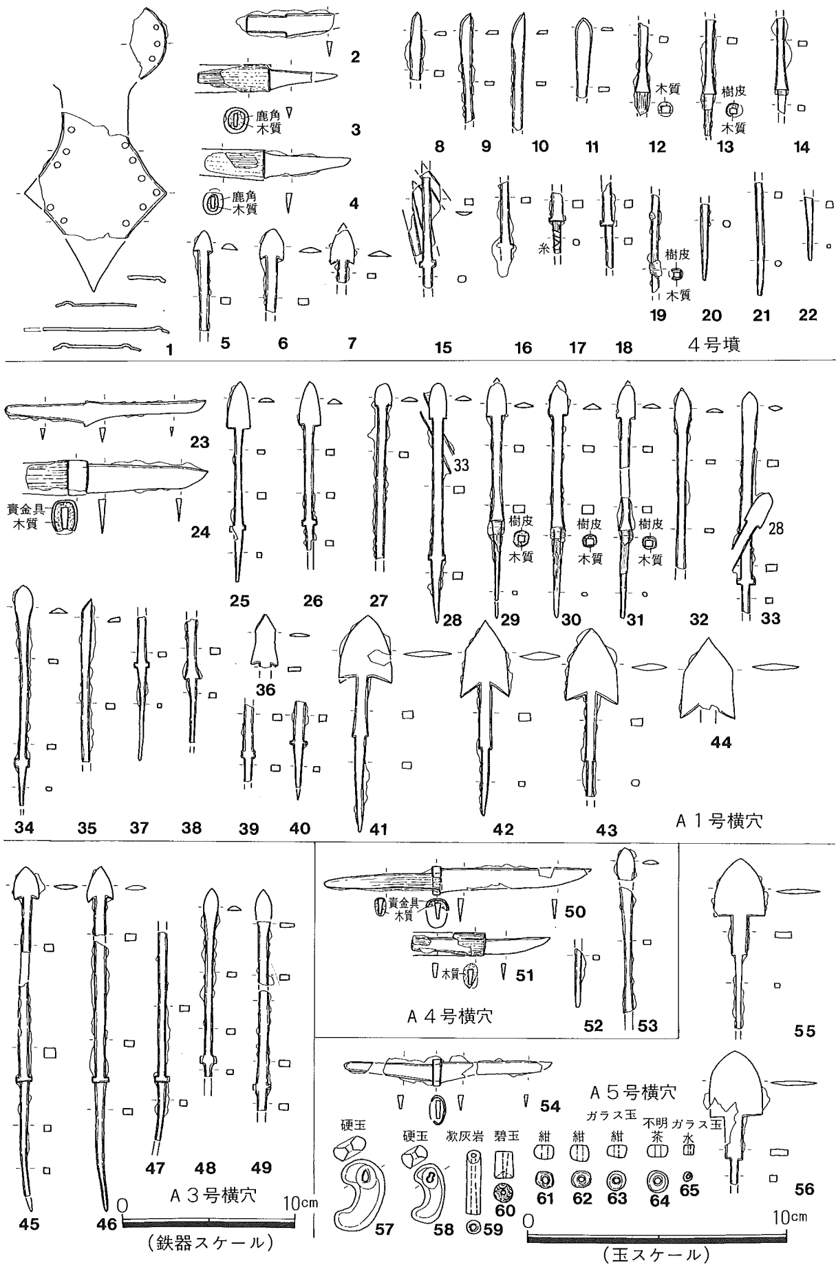
第34図 鉄製品実測図 (2)
