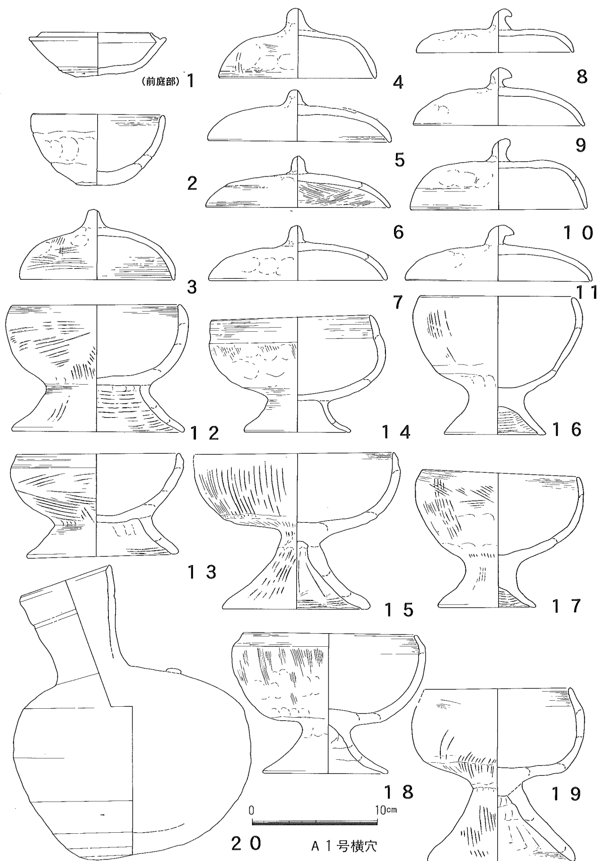
第24図 須恵器・土師器実測図 (1)
