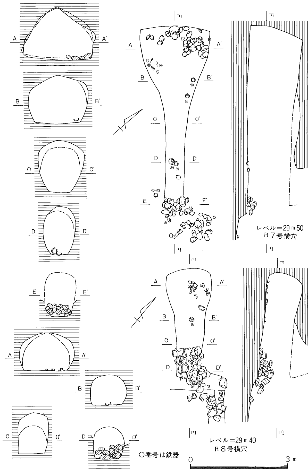
第18図 B 7号・B 8号横穴実測図
