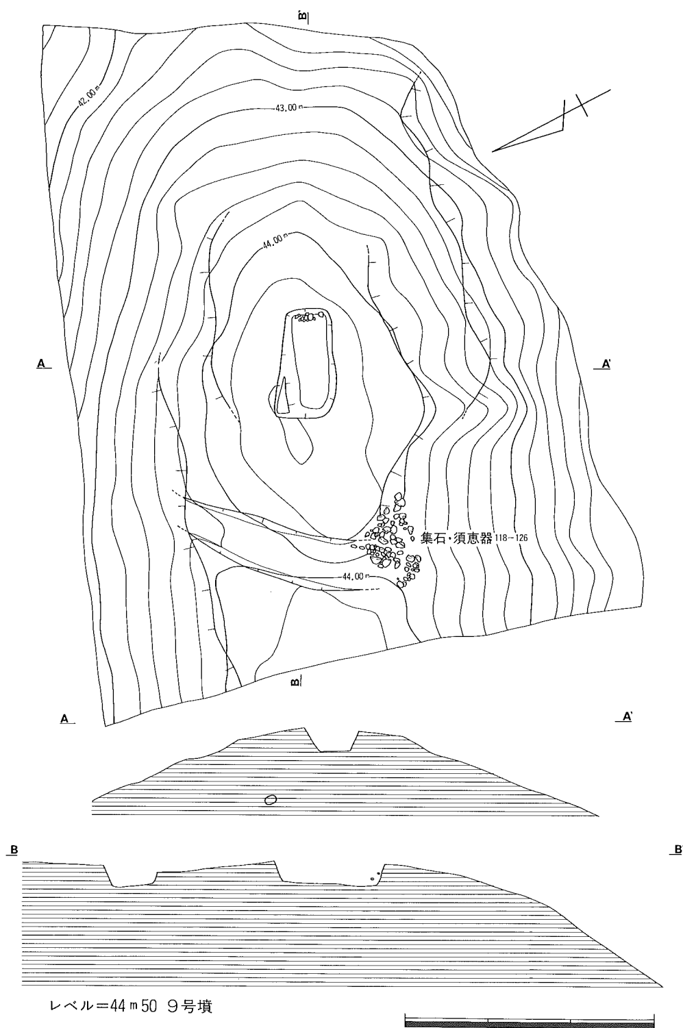
第8図 9号墳墳丘実測図
