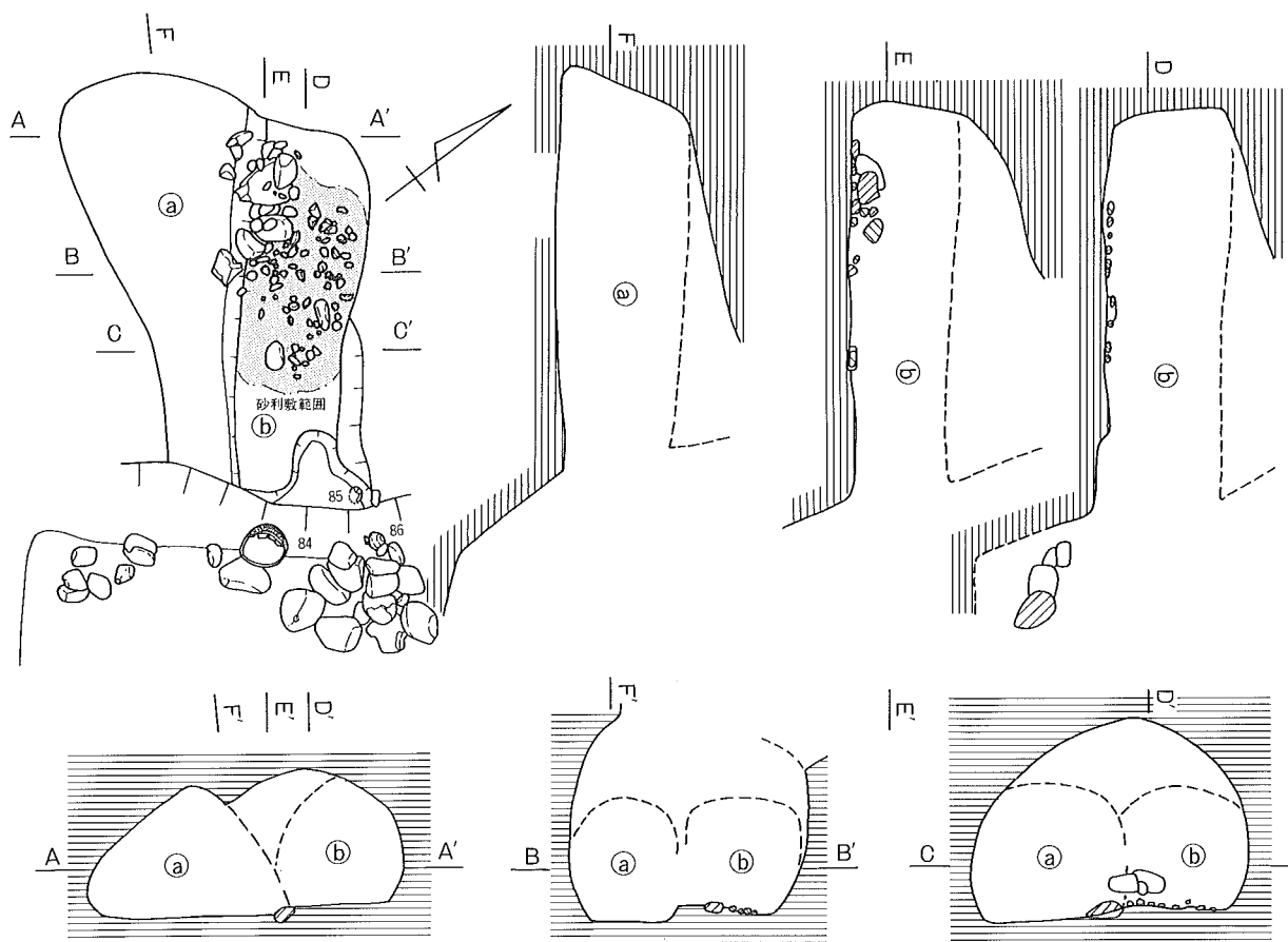
レベル=29 m 90 B 5号横穴
