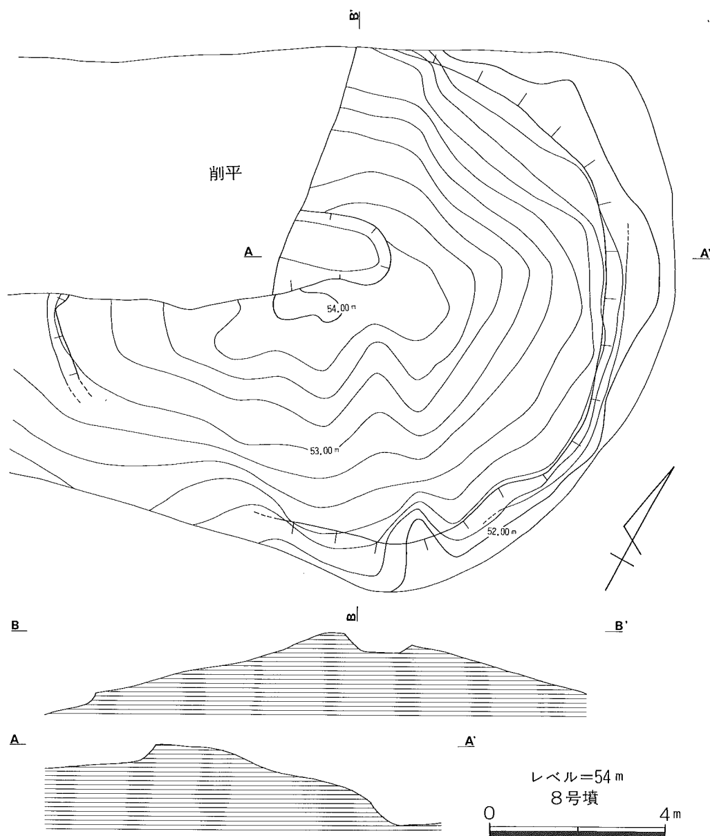
第7図 8号墳墳丘実測図
