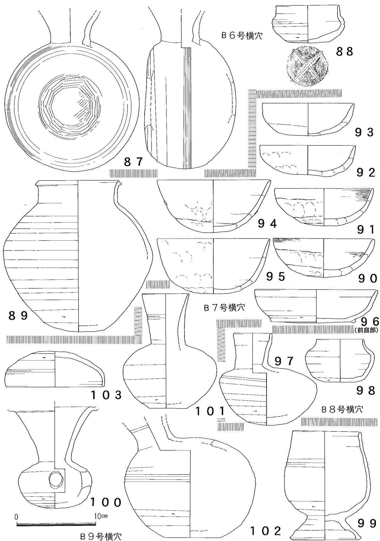
第30図 須恵器・土師器実測図 (7)
