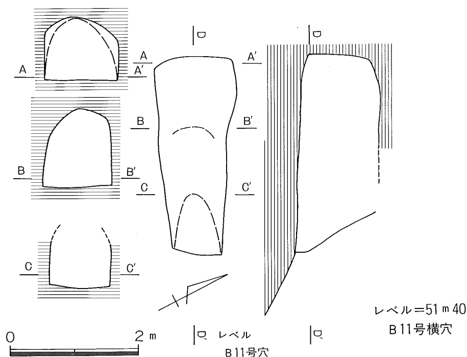
第20図 B11号横穴実測図
