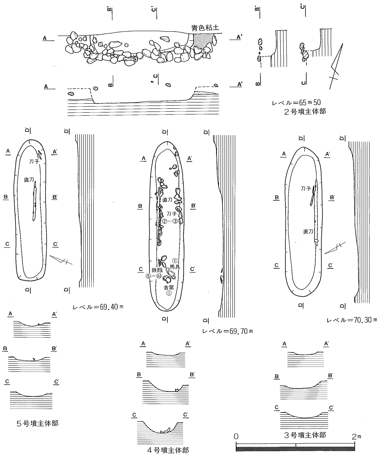
第6図 2～5号墳主体部実測図
