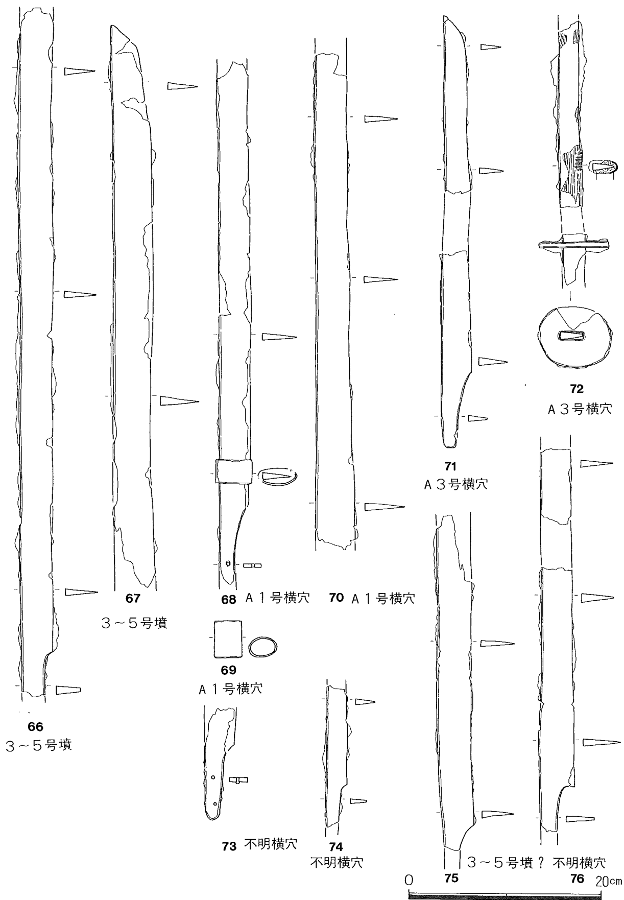
第35図 鉄製品実測図 (3)
