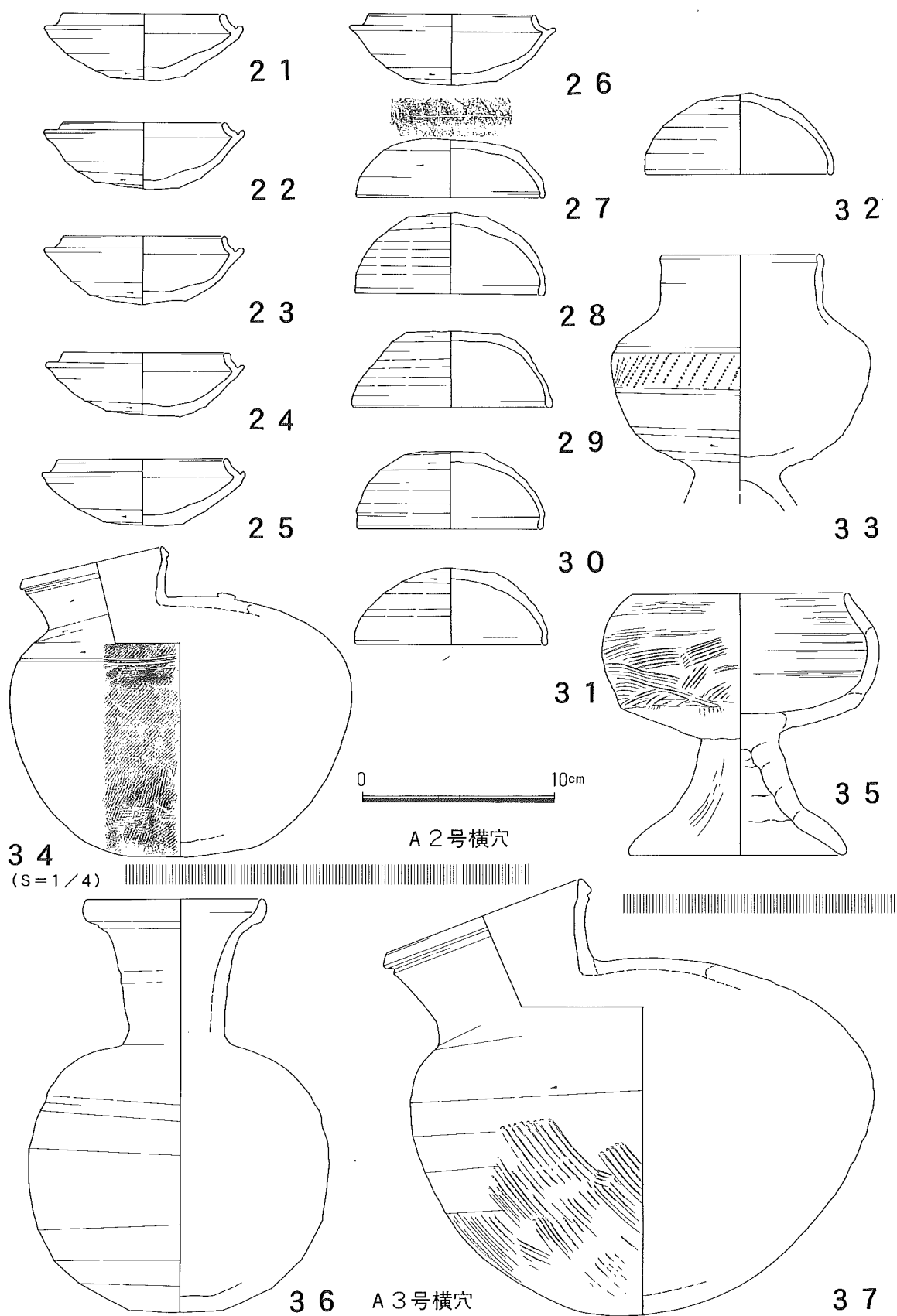
第25図 須恵器・土師器実測図 (2)
