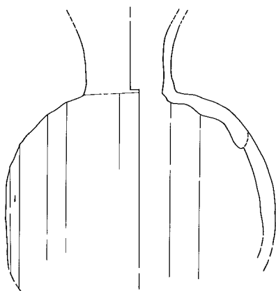
第26図 須恵器・土師器実測図 (3)
