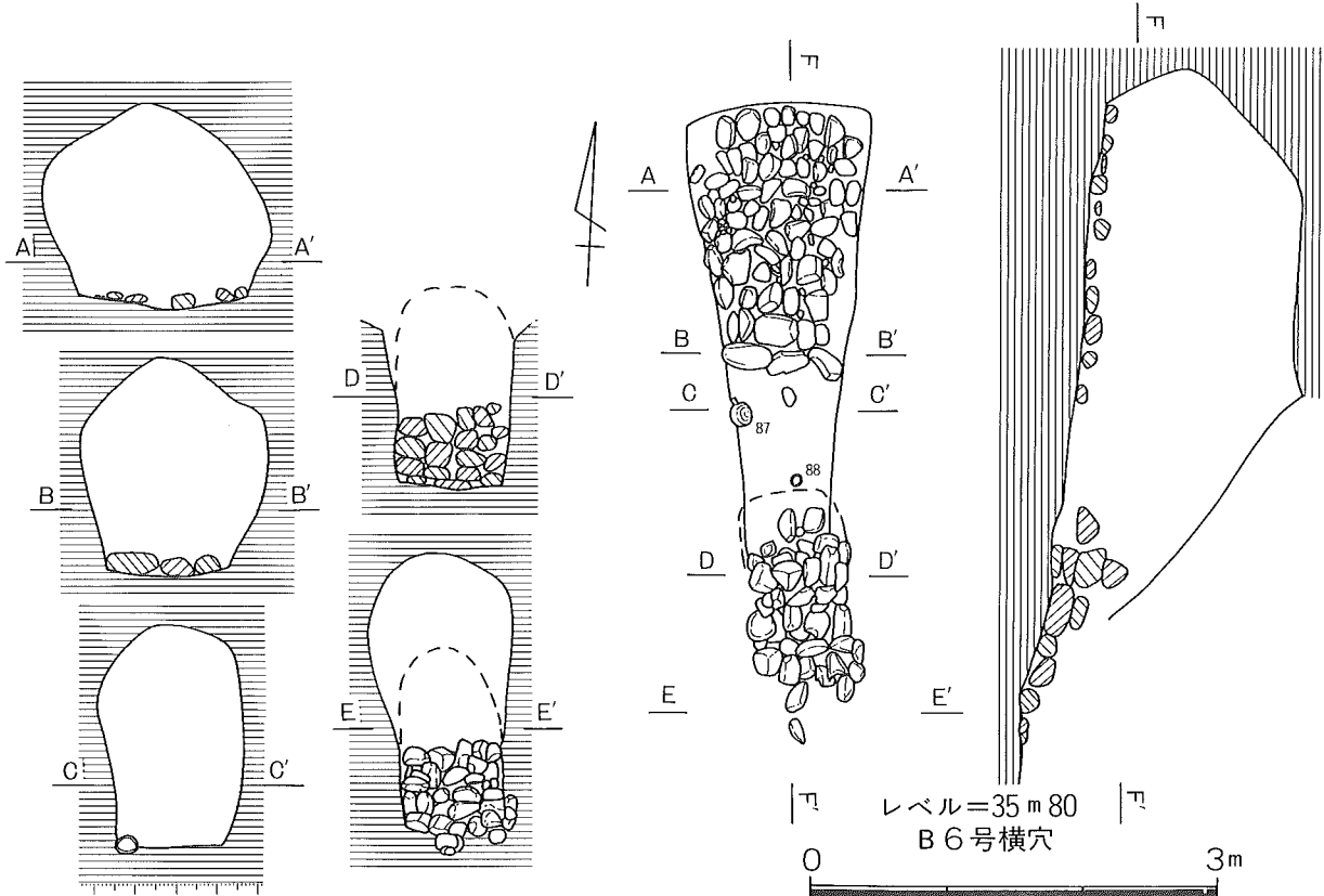
第17図 B 5号・B 6号横穴実測図
