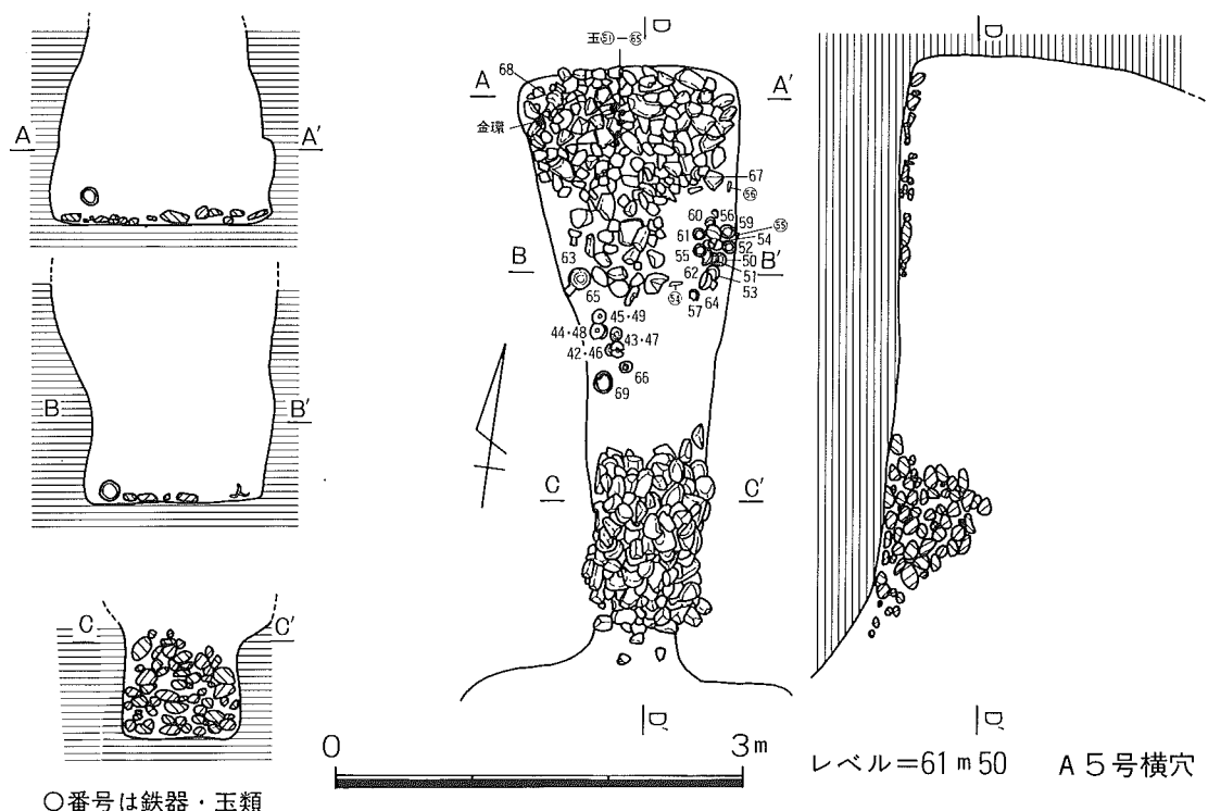
第14図 A 5号横穴実測図
