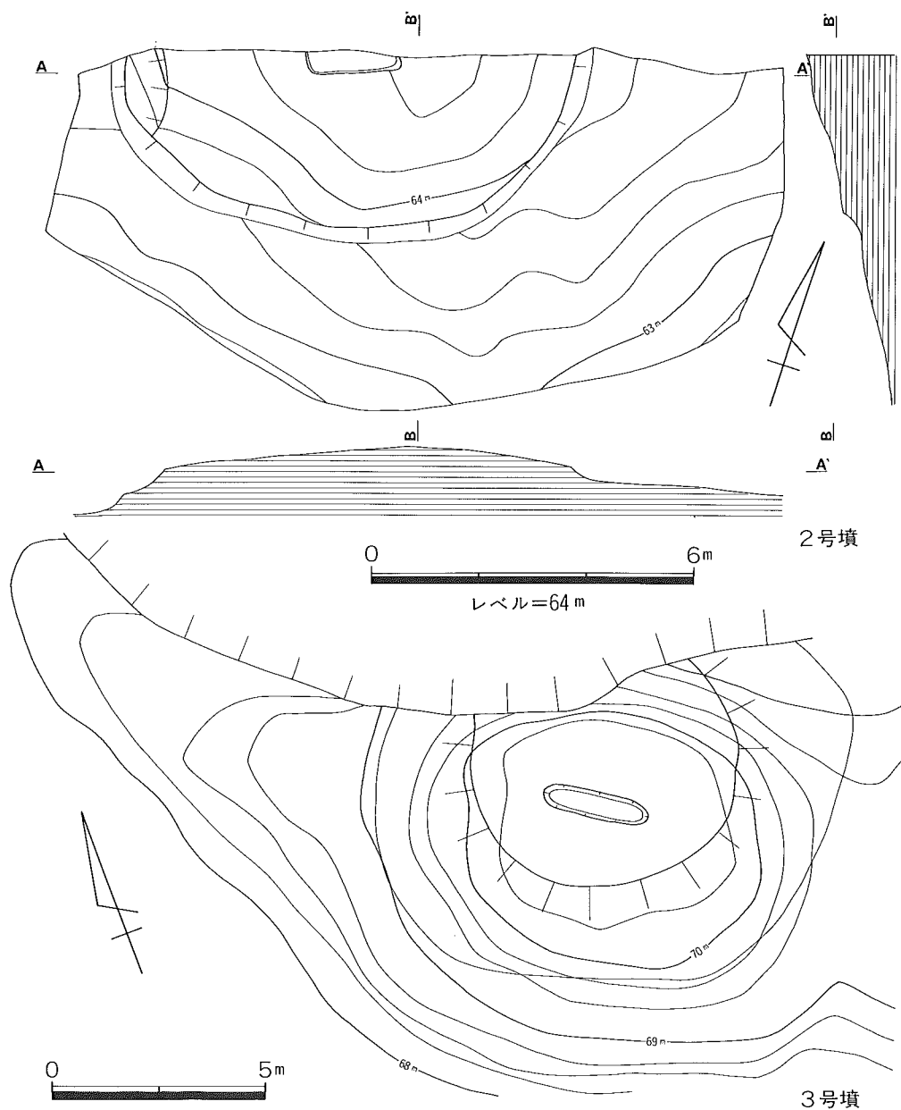
第4図 2号墳・3号墳墳丘実測図
