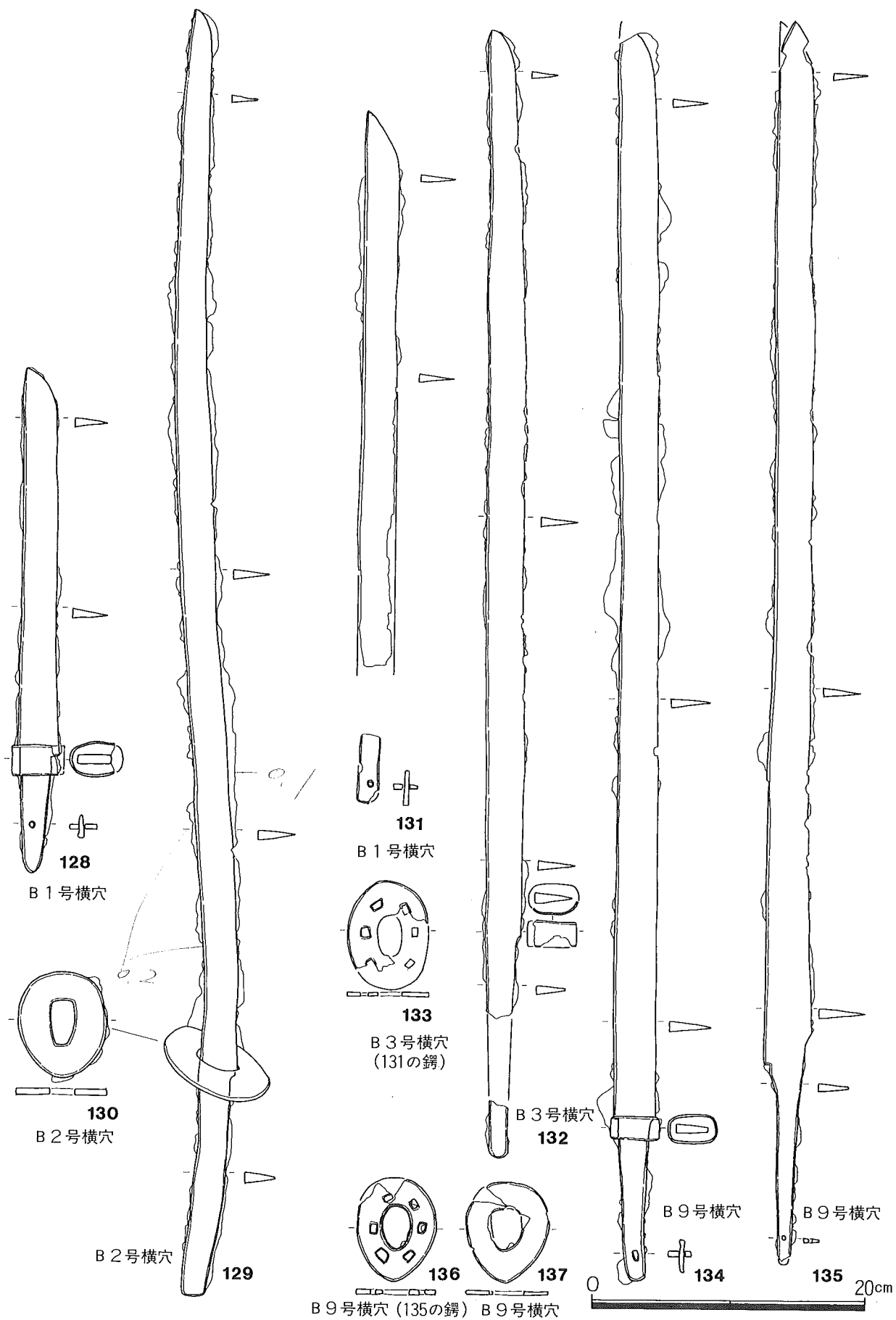
第37図 鉄製品実測図 (5)
