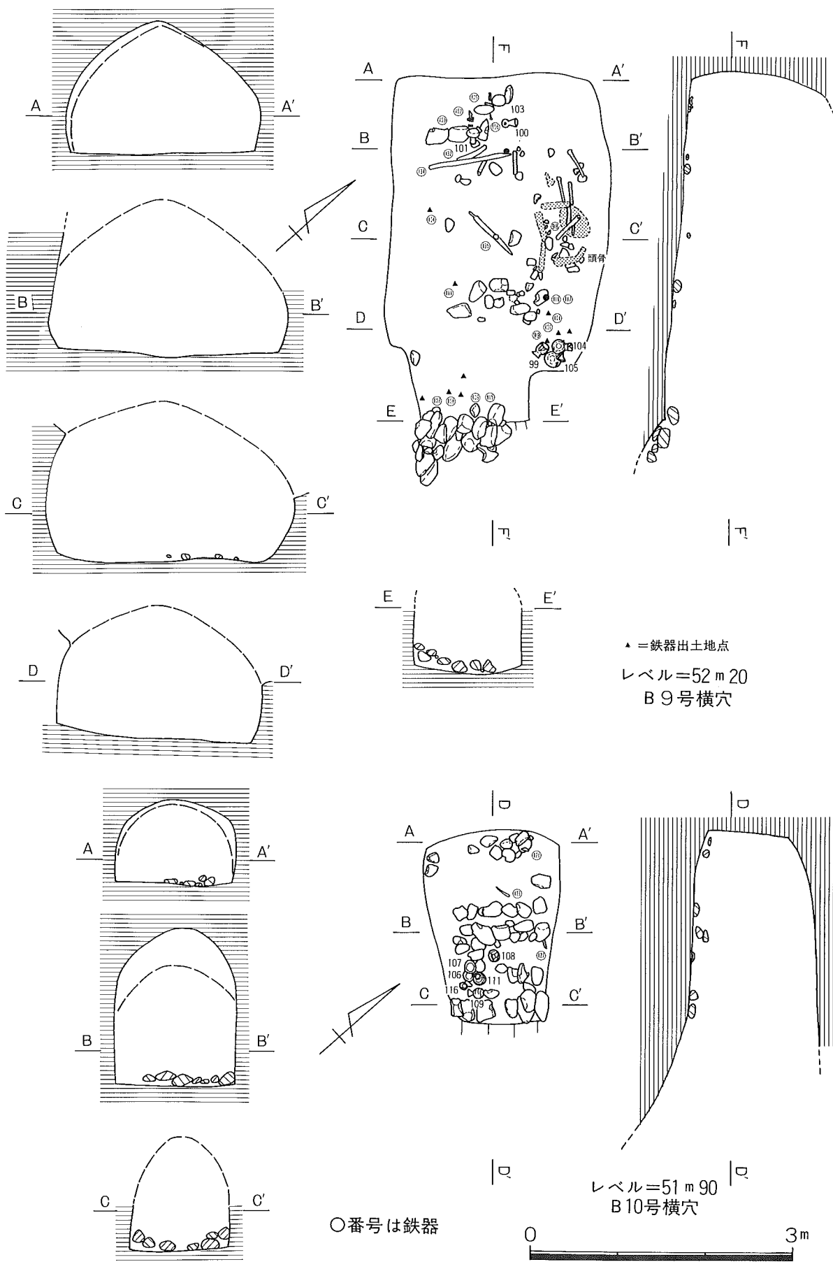
第19図 B 9号・B10号横穴実測図
