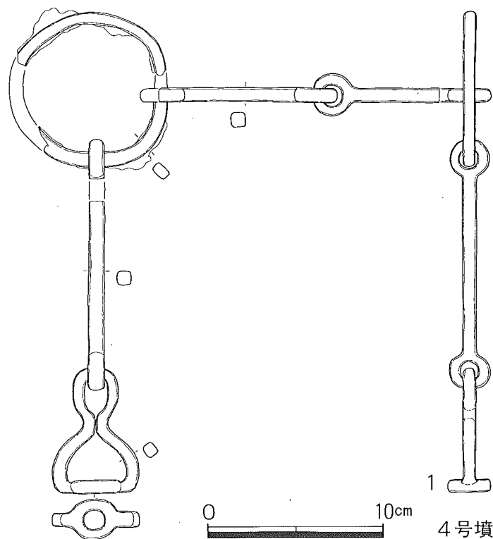
第33図 鉄製品実測図 (1)
