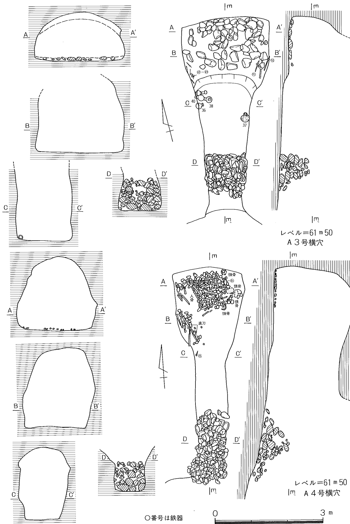
第13図 A 3号・A 4号横穴実測図
