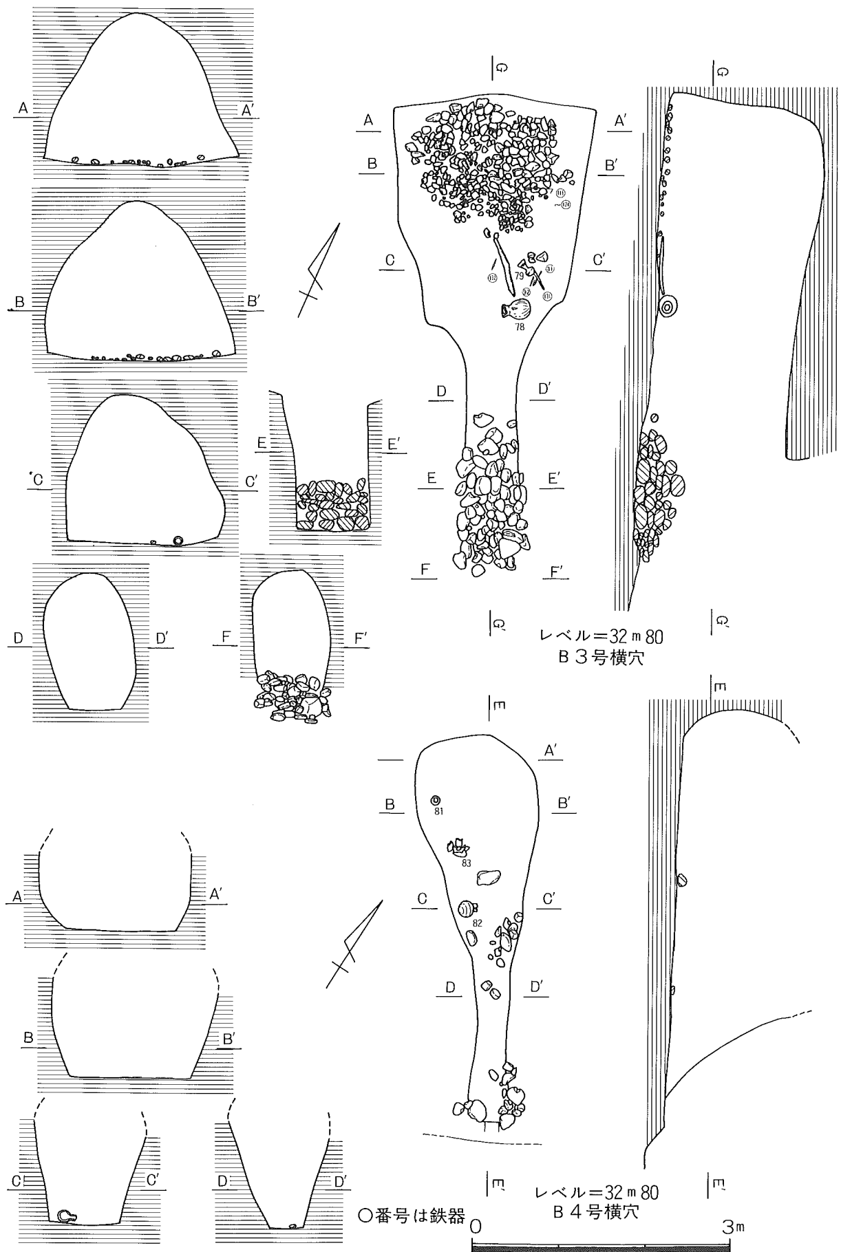
第16図 B 3号・B 4号横穴実測図
