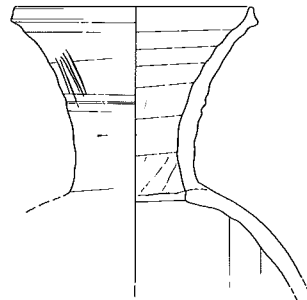
第31図 須恵器・土師器実測図 (8)
