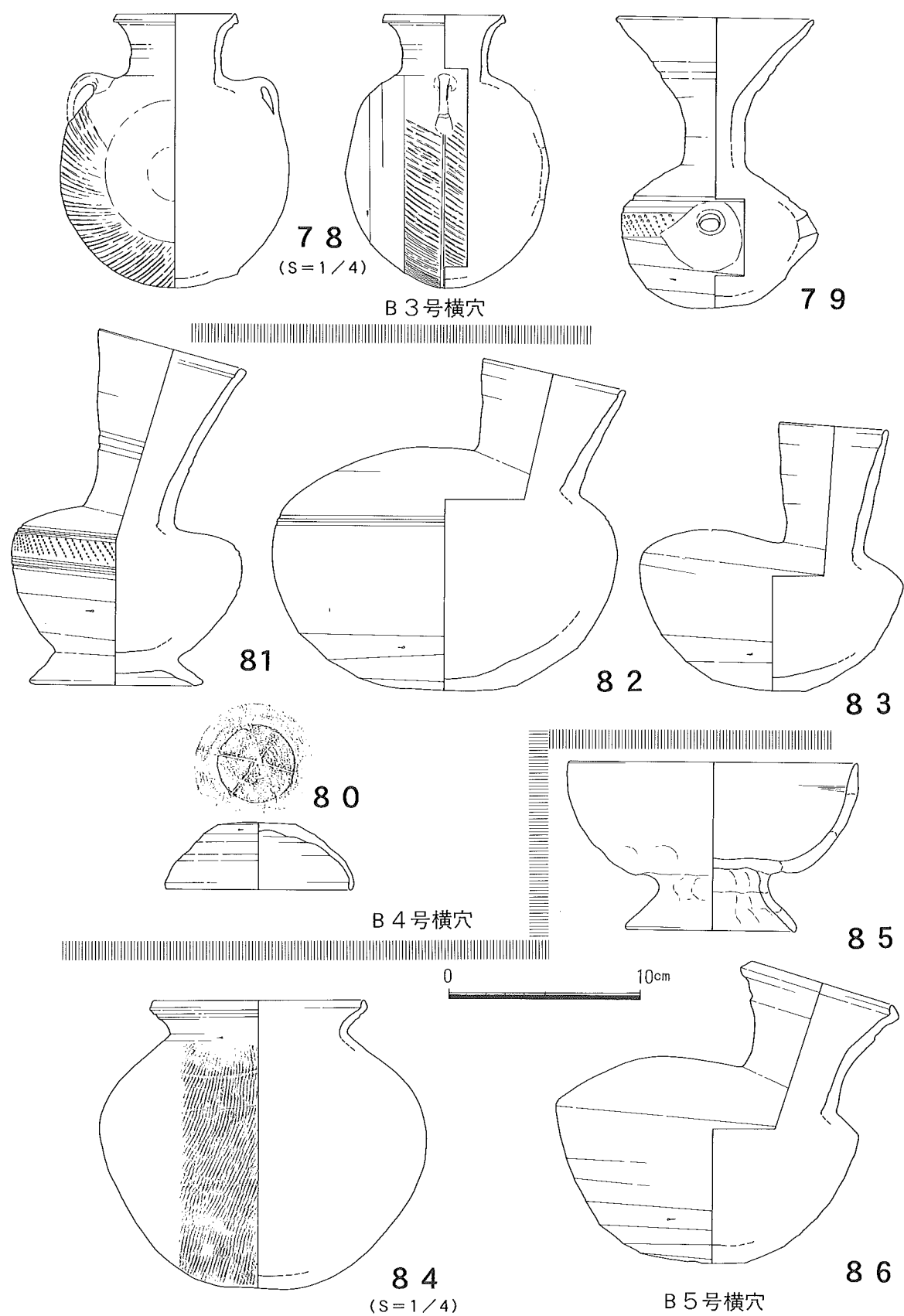
第29図 須恵器・土師器実測図 (6)
