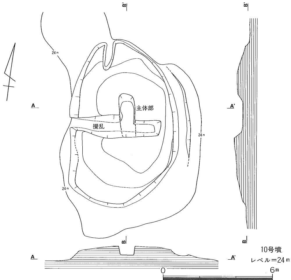
第9図 10号墳墳丘実測図
