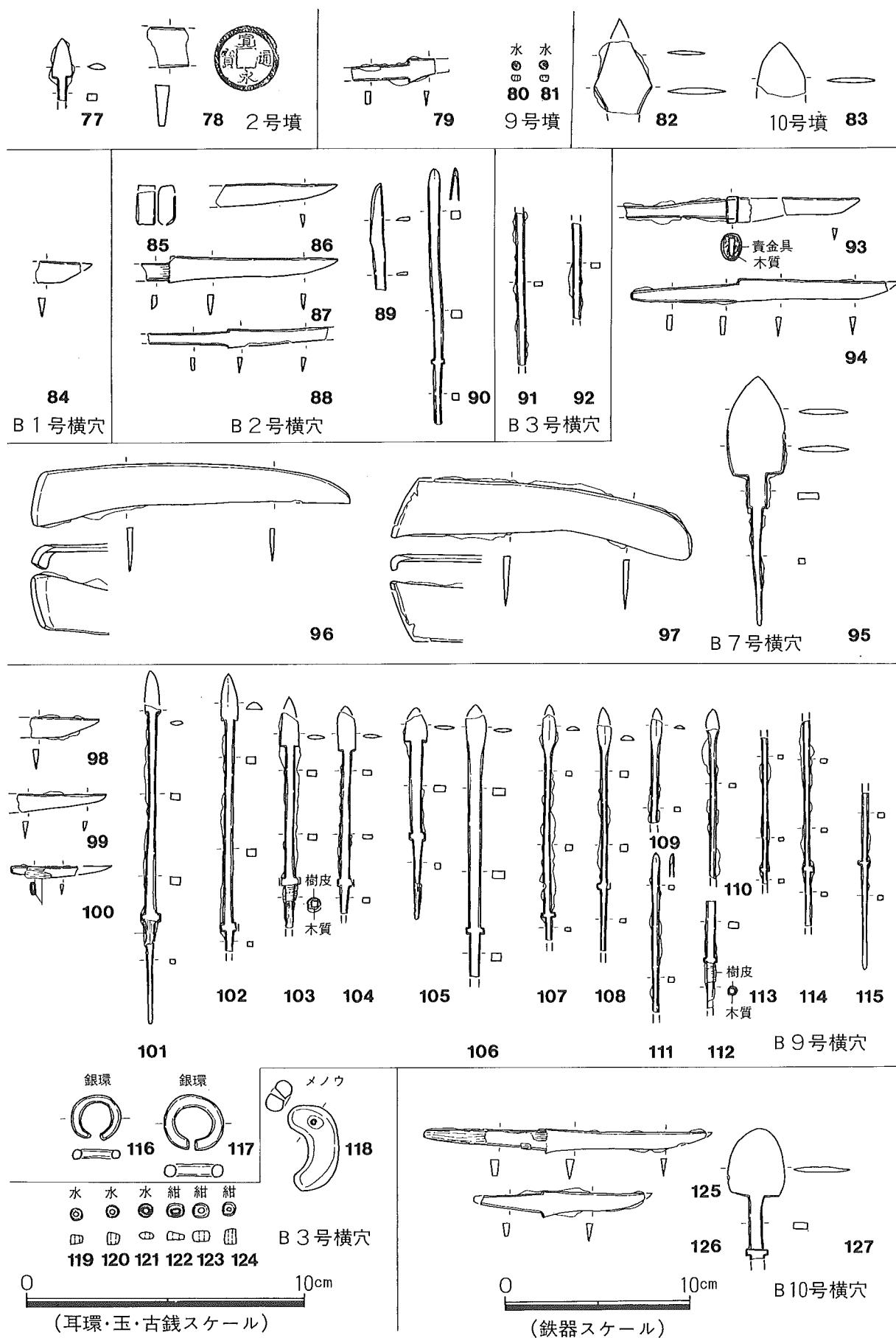
第36図 鉄製品実測図 (4)
