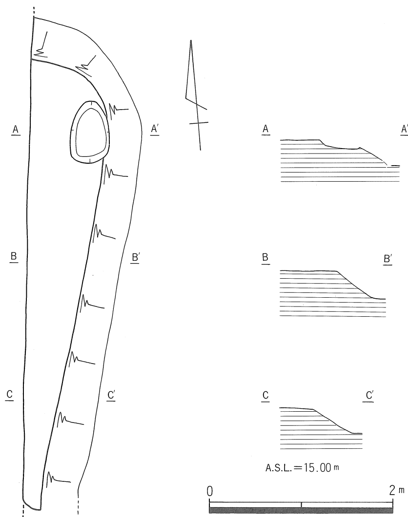
第4図 南地区実測図
