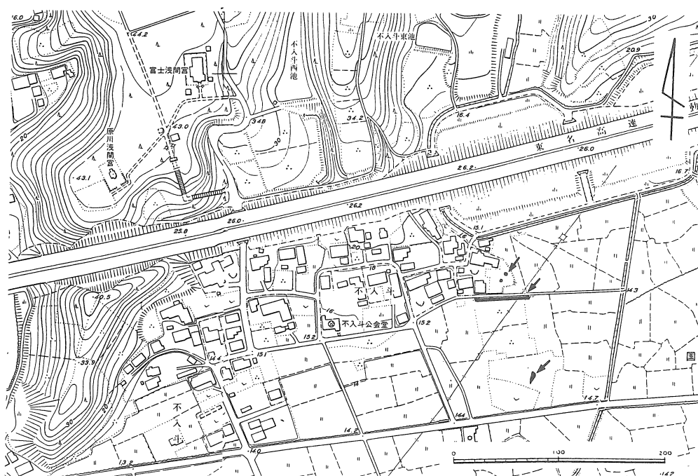
第2図 発掘調査区の位置図 (1/5,000)
