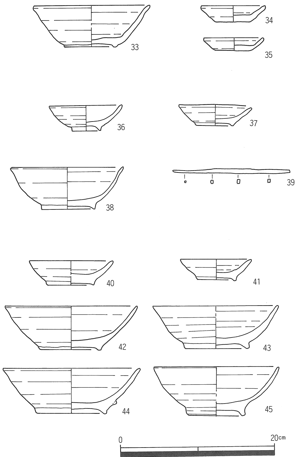
第17図 出土遺物実測図(3)
