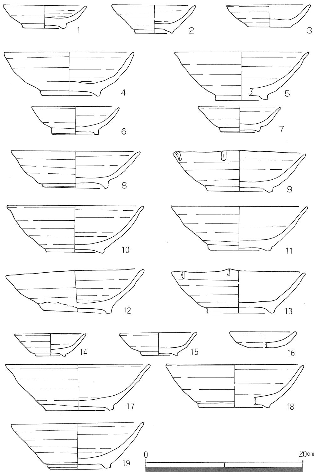
第15図 出土遺物実測図(1)
