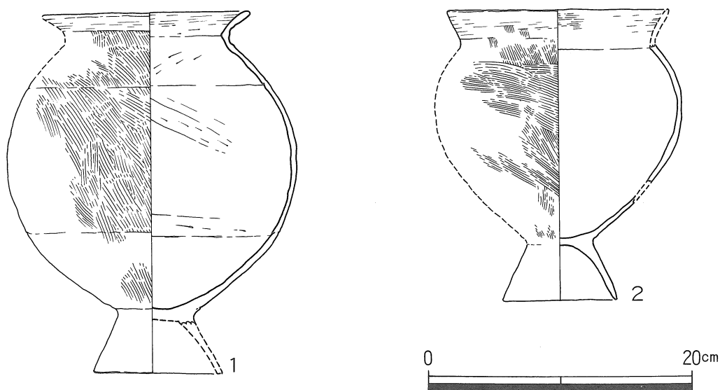
第3図 SK-17出土土器実測図
