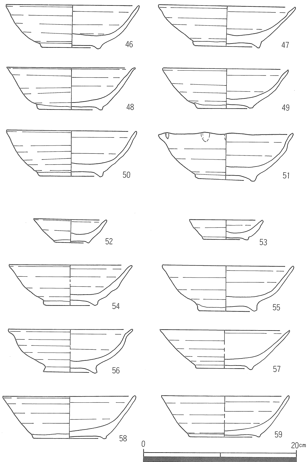
第18図 出土遺物実測図(4)
