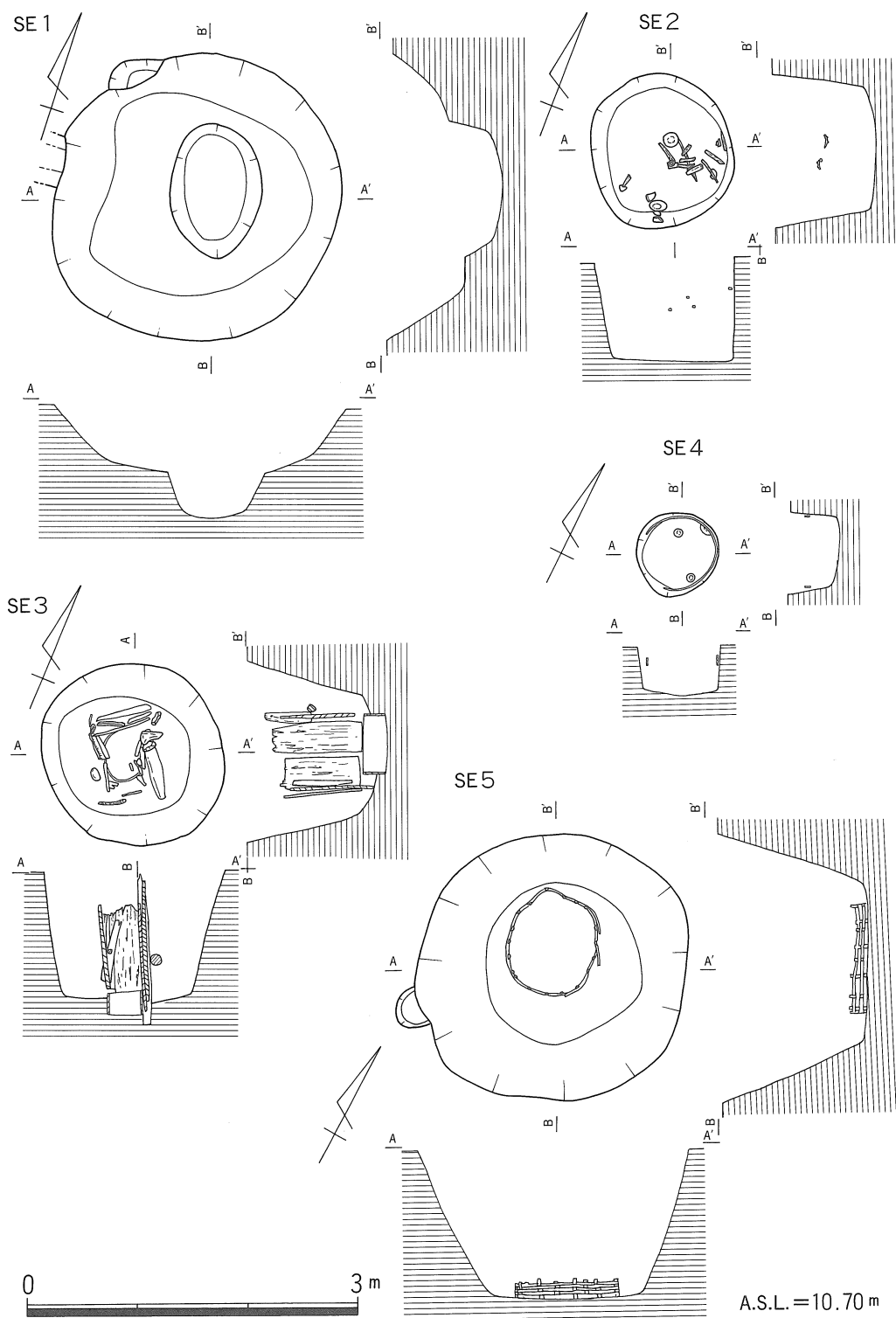
第11図 遺構実測図(8) SE 1・SE 2・SE 3・SE 4
