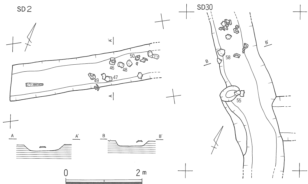
第13図 遺構実測図 SD2・SD30
