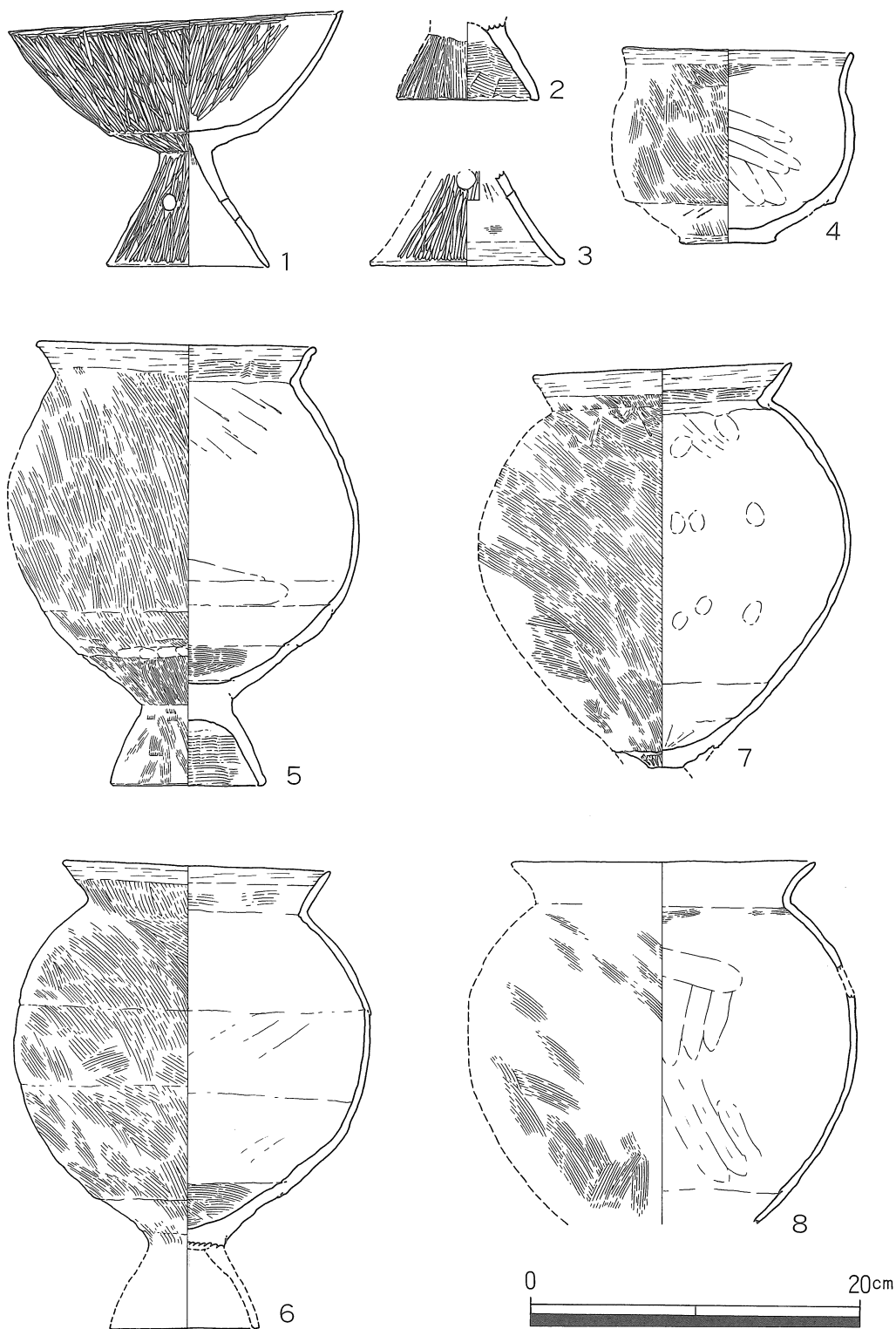
第2図 SK-17出土土器実測図
