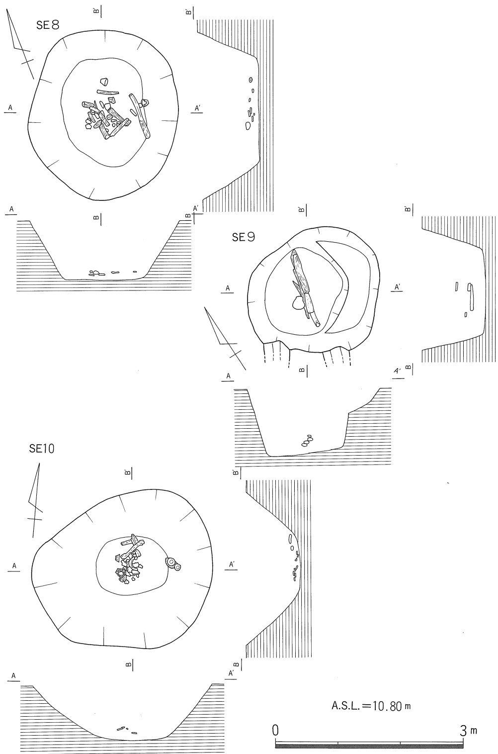
第 6 図 遺構実測図(3) SE 8・SE 9・SE 10
