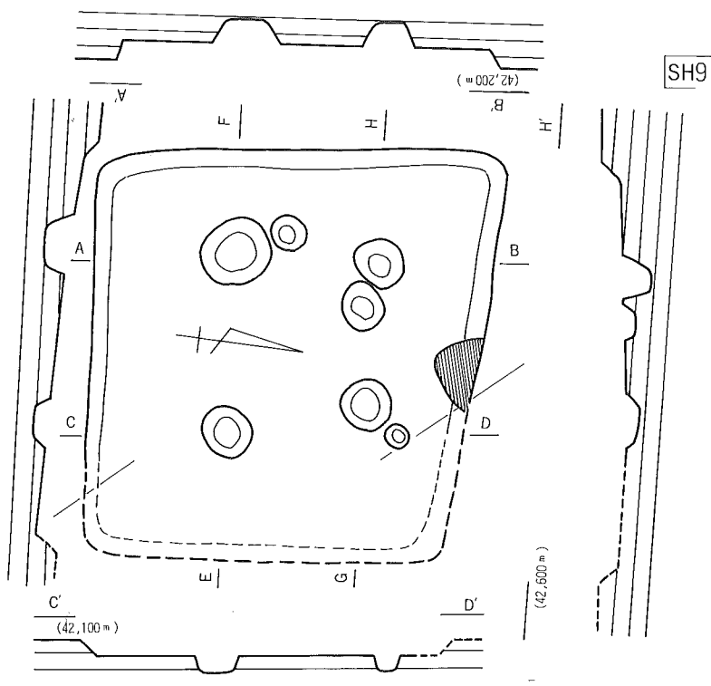
第11図 掘立柱建物跡SB1、竪穴住居跡SH9実測図
