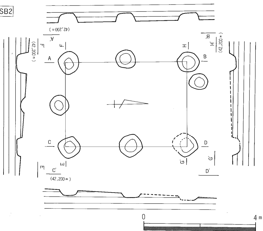
第12図 掘立柱建物跡SB3、SB2実測図
