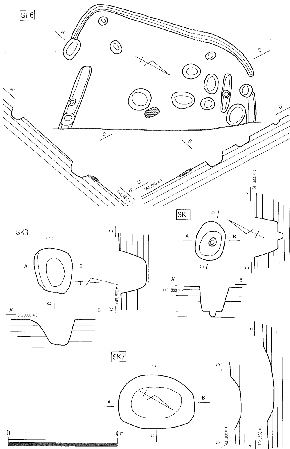
第10図 竪穴住居跡SH 6、土壇状遺構SK 1・SK 3・SK 7実測図
