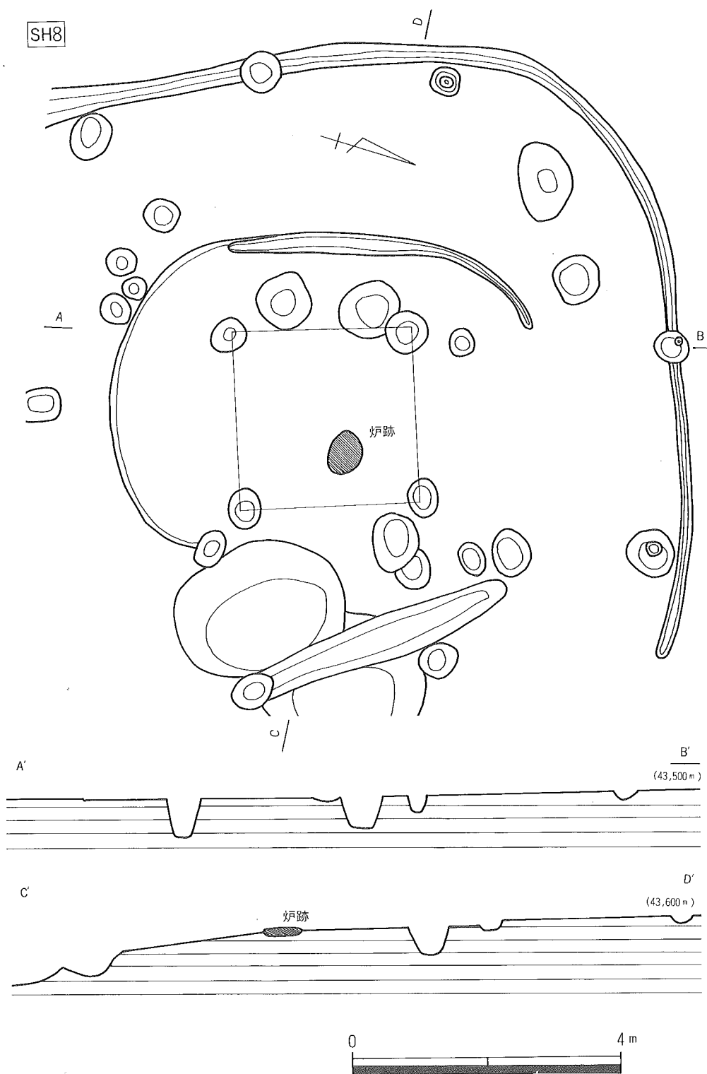
第9図 竖穴住居跡SH8実測図
