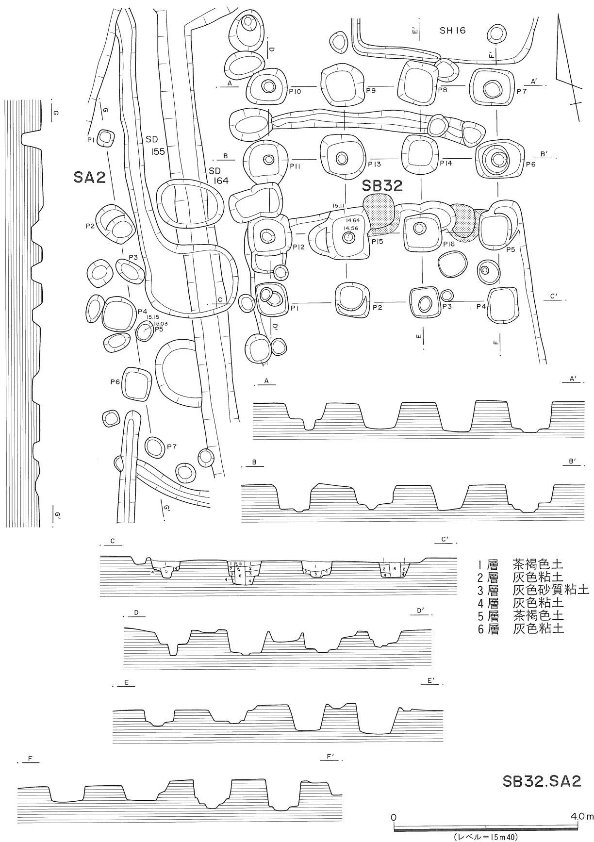
第17図 SB32・SA2 実測図
