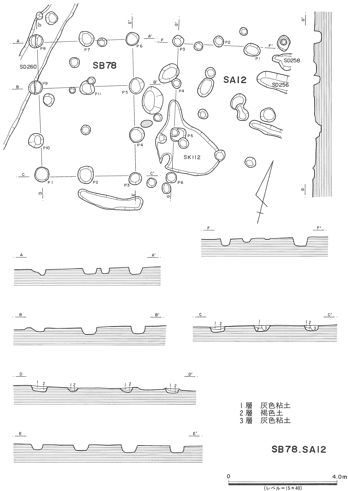
第42図 SB78・SA12実測図
