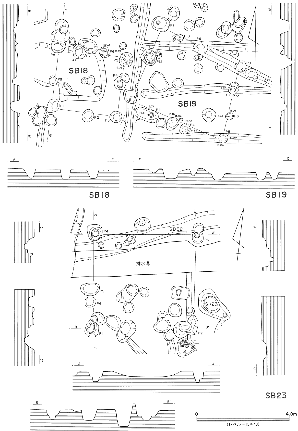
第12図 SB18・SB19・SB23実測図
