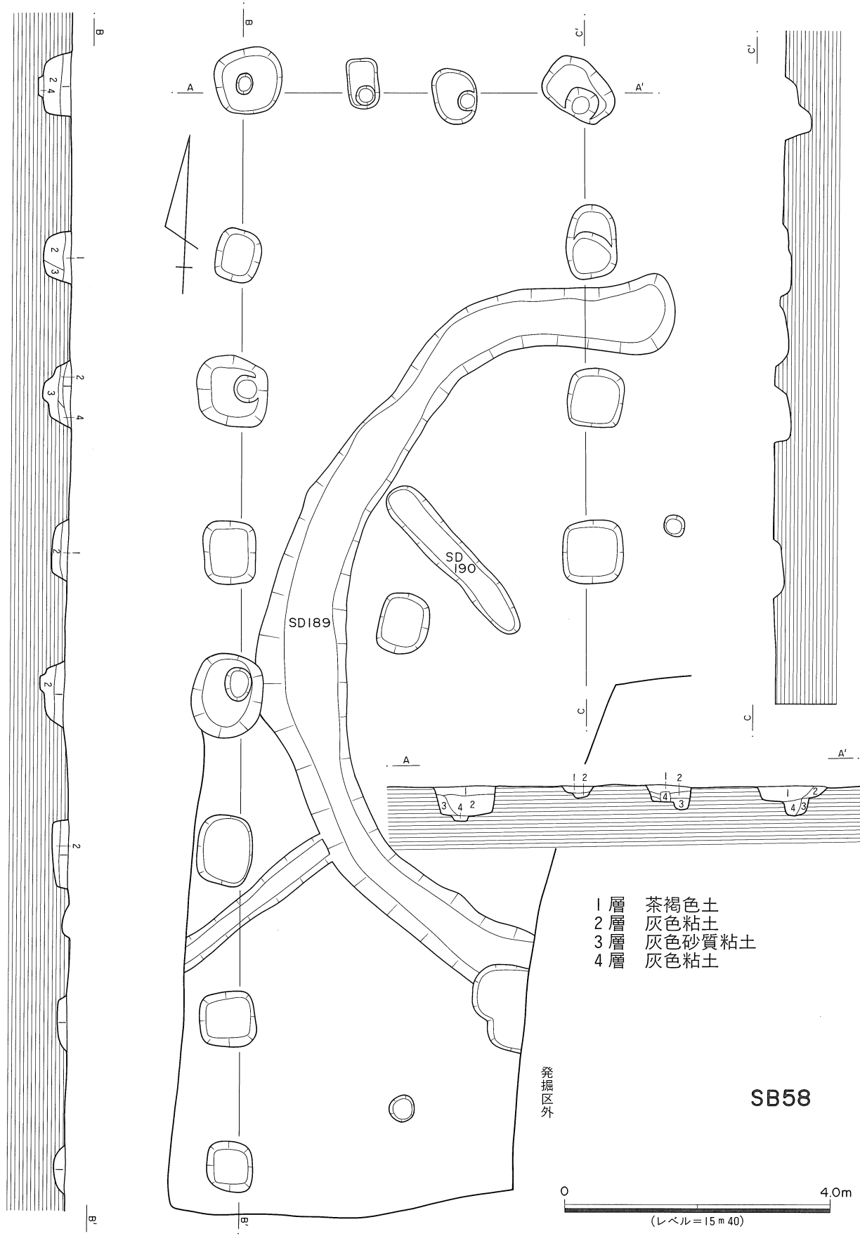
第29図 SB58実測図
