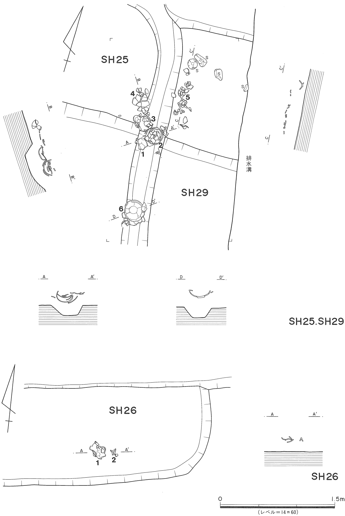
第90図 SH25・SH26・SH29実測図
