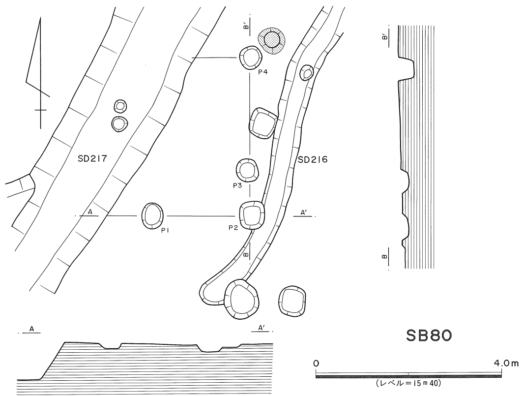
第43図 SB79・SB80実測図
