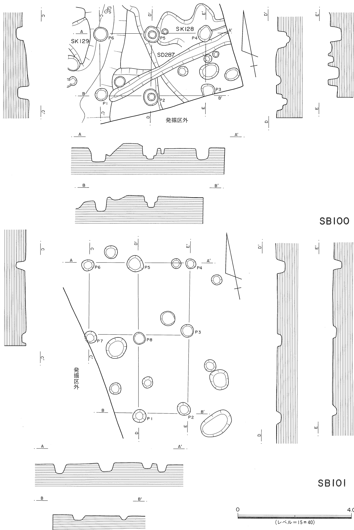
第54図 SB100・SB101実測図
