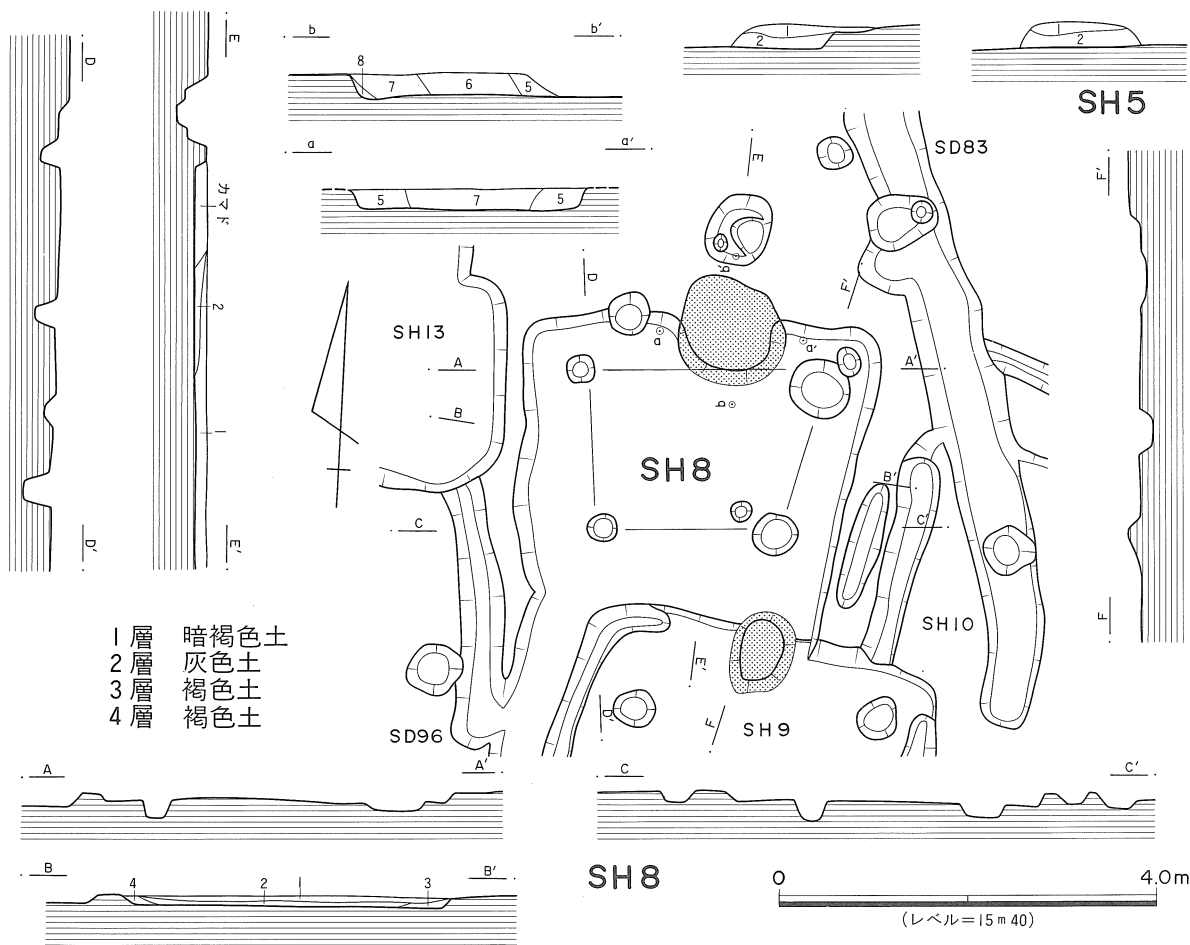
第76図 SH5・SH8実測図
