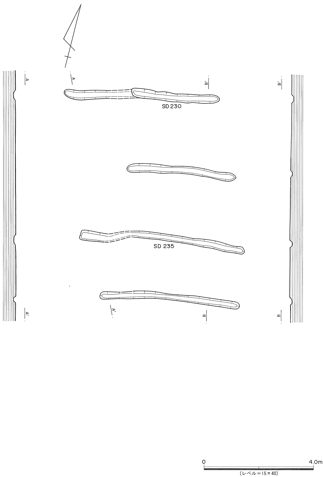
第155図 畝2実測図
