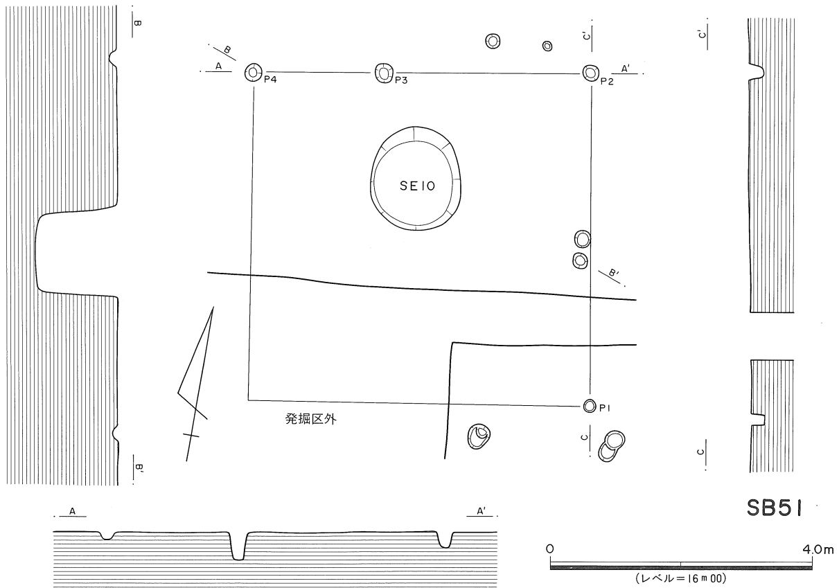
第26図 SB50・SB51実測図
