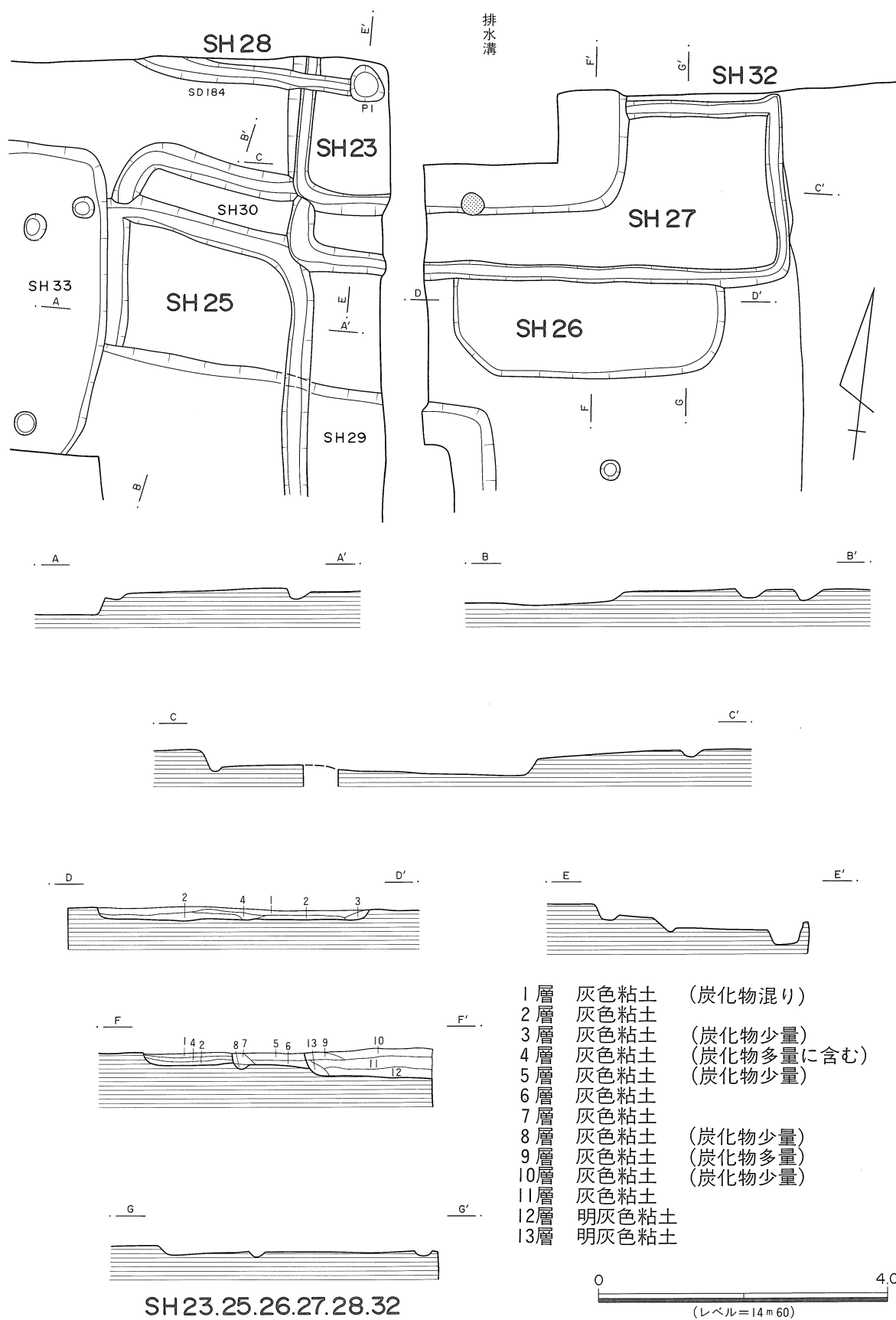
第87図 SH23・25・26・27・28・32実測図
