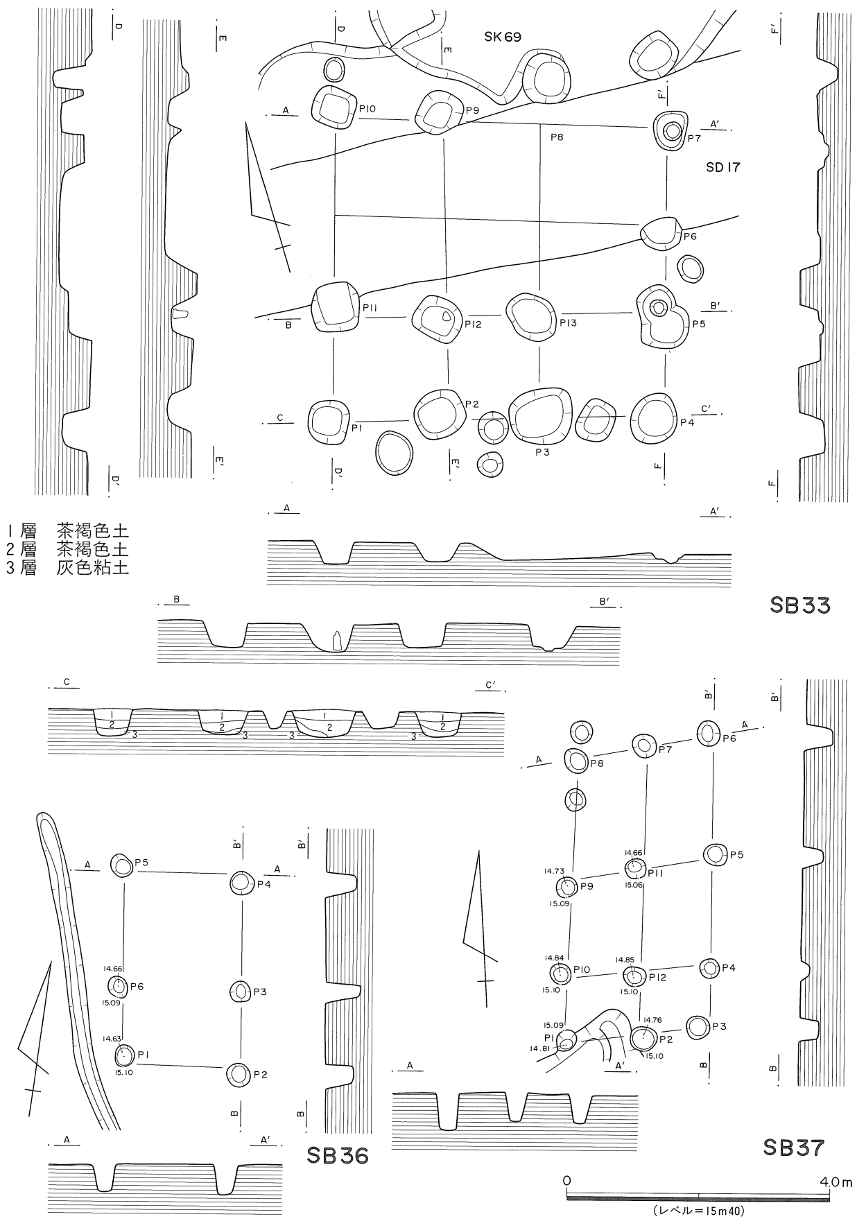
第18図 SB33・SB36・SB37実測図
