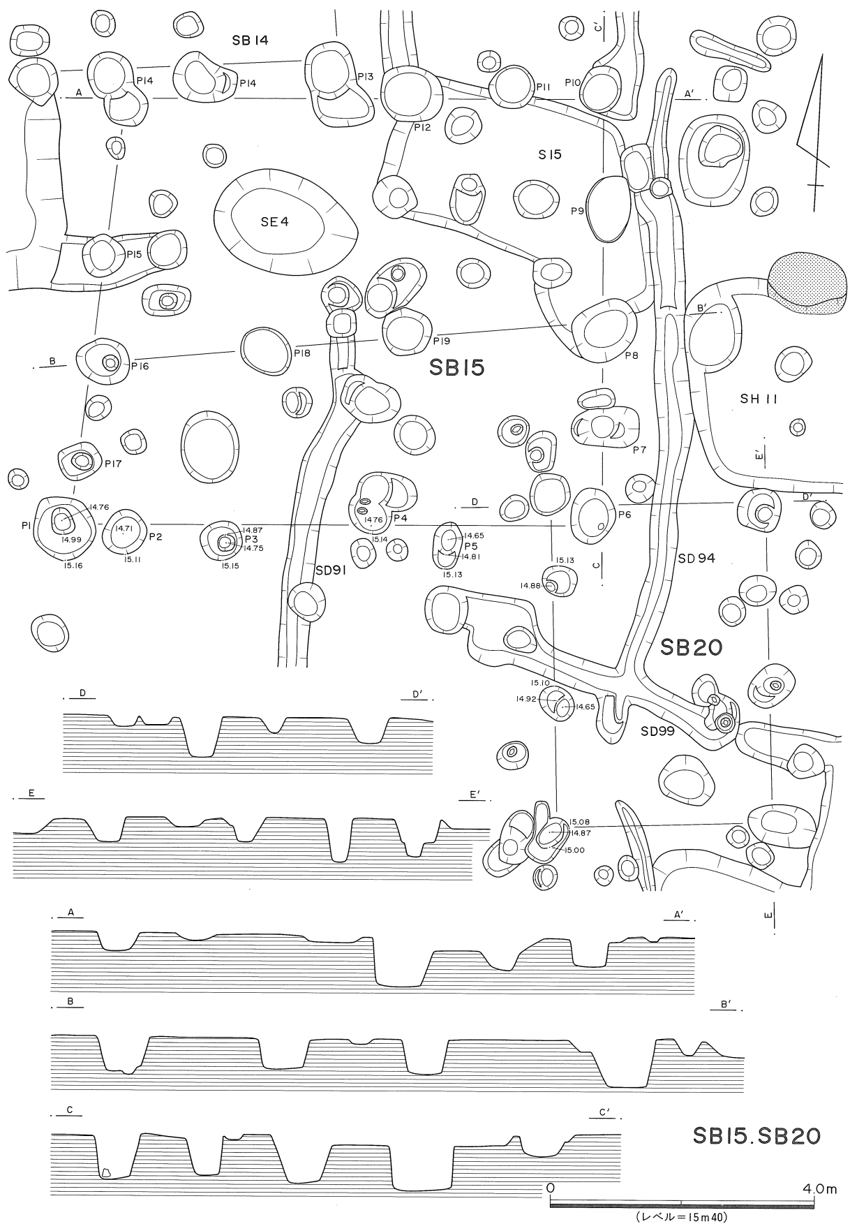
第10図 SB15・SB20実測図
