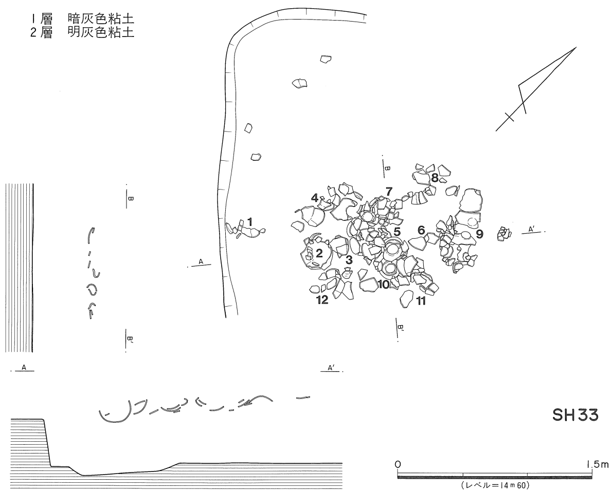
第91図 SH33実測図
