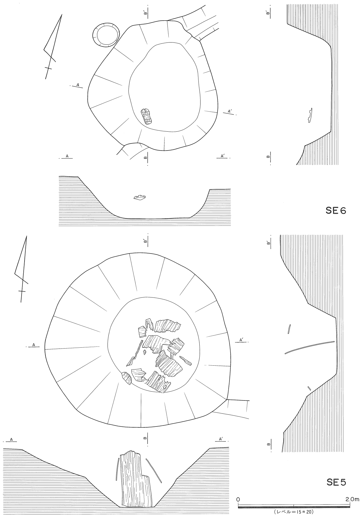
第63図 SE5・SE6 実測図
