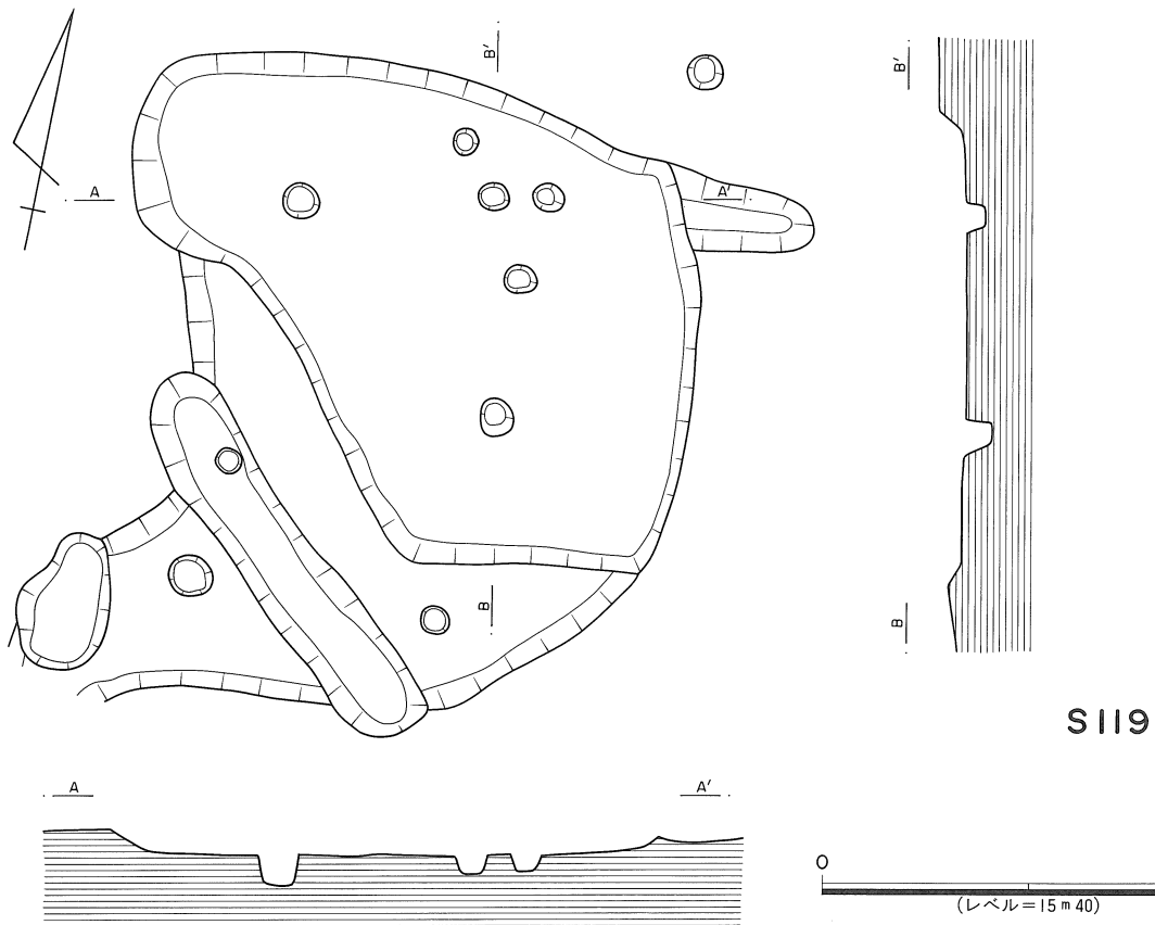
第114図 SI16・SI18・SI19実測図
