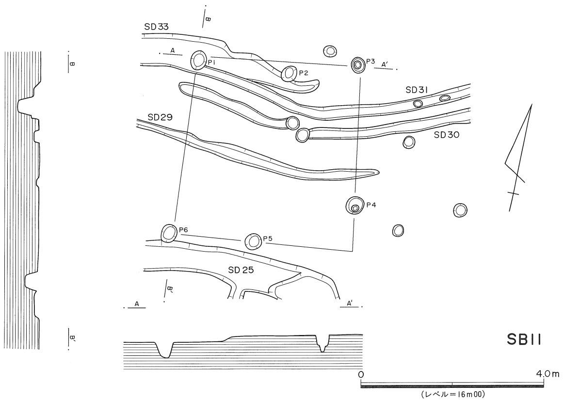
第5図 SB7・SB11実測図
