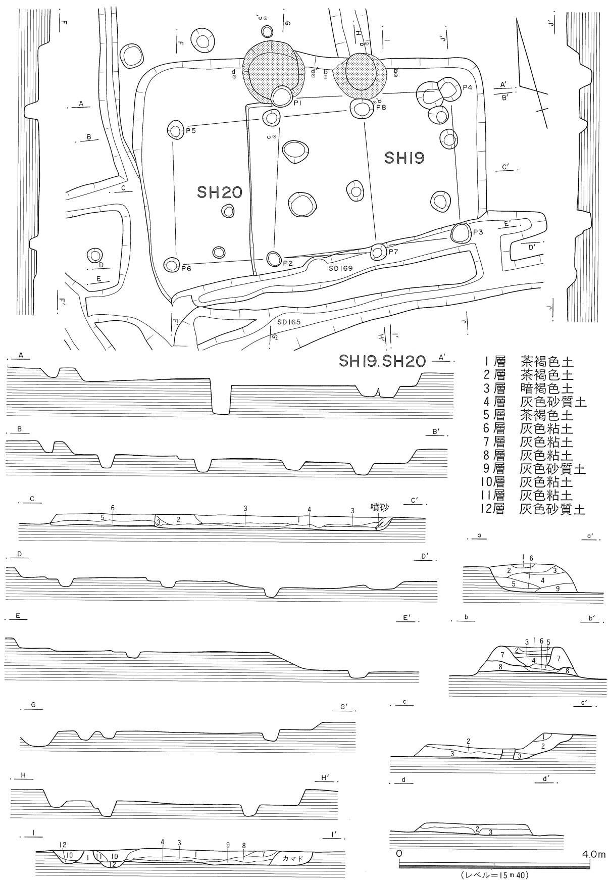
第85図 SH19・SH20実測図
