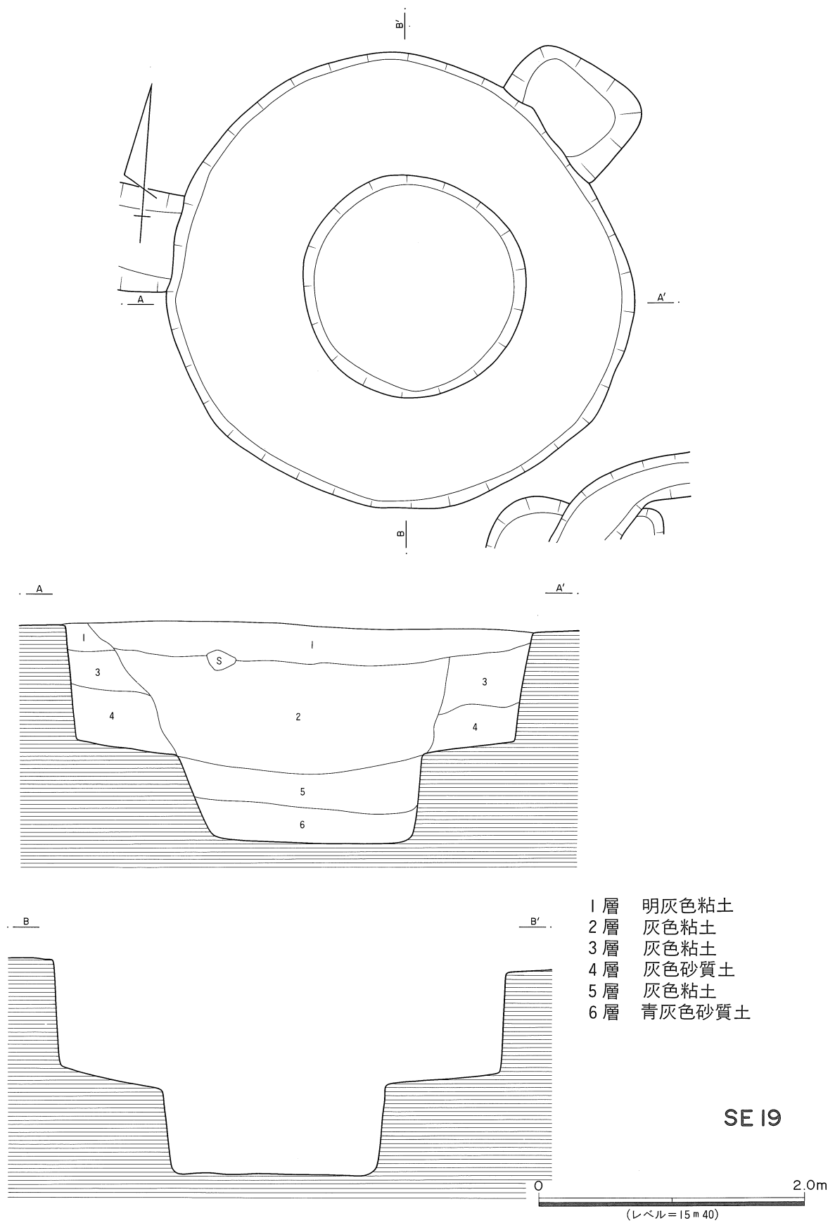
第70図 SE19実測図
