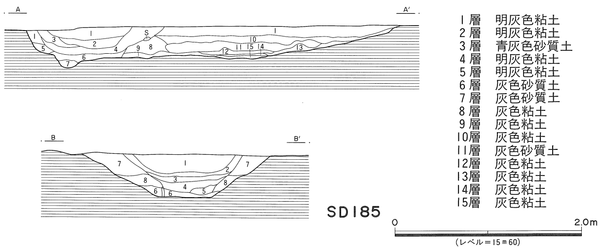
第146図 SD16・SD17・SD185実測図
