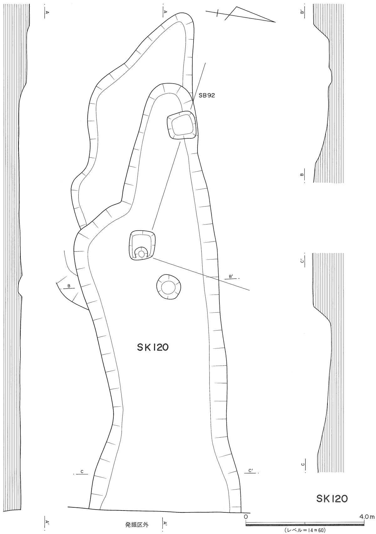
第134図 SK120実測図
