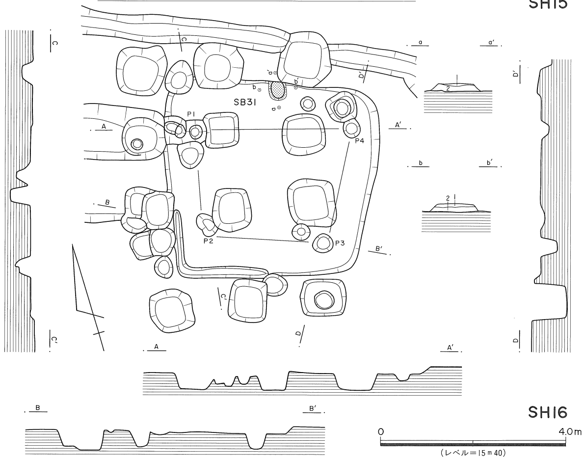
第82図 SH15・SH16実測図
