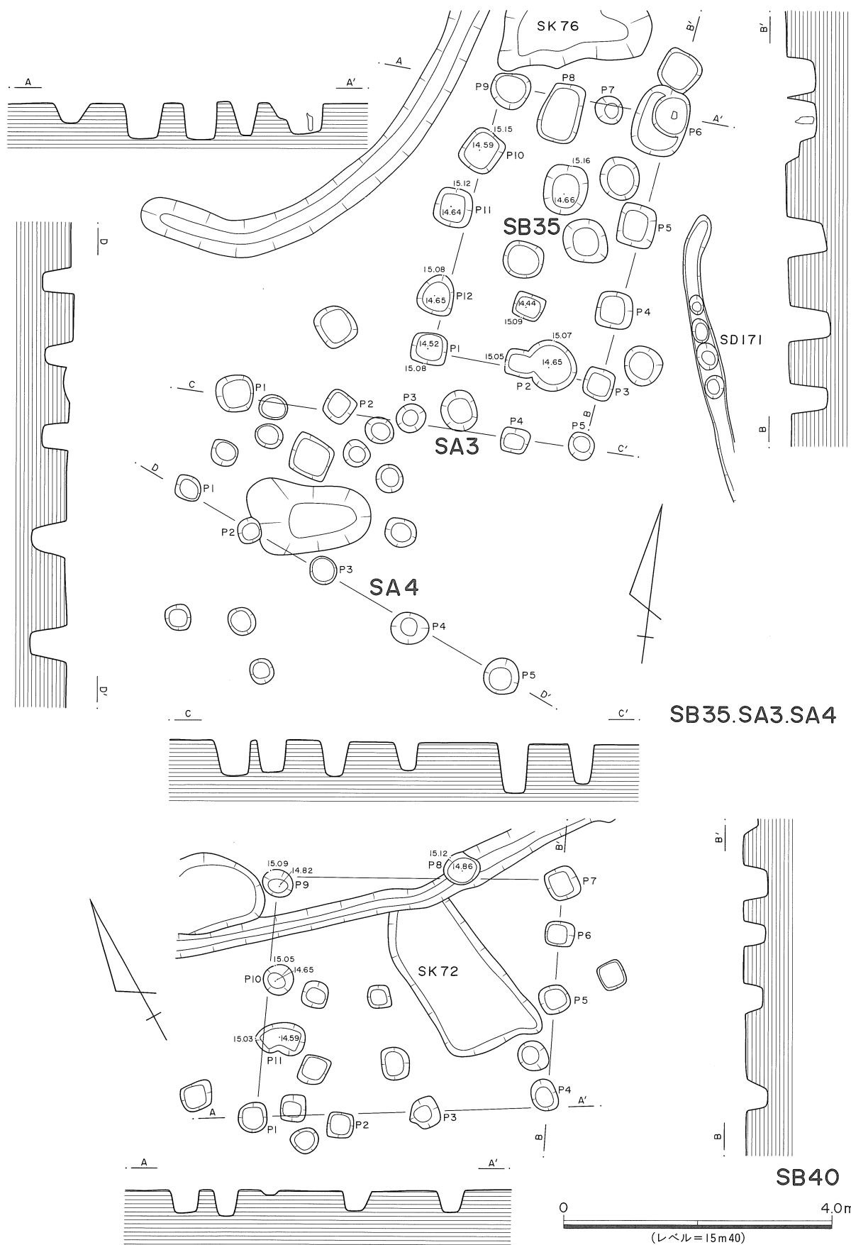
第19図 SB35・SA3・SA4・SB40実測図
