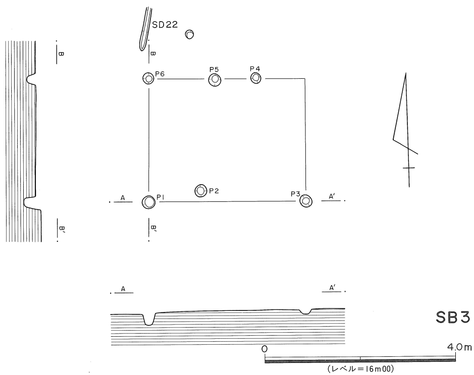
第1図 SB1・SB3実測図
