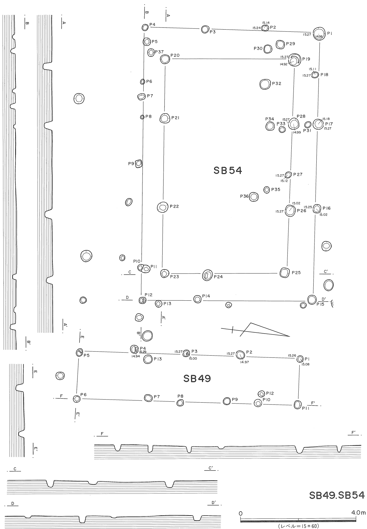
第25図 SB49・SB54実測図
