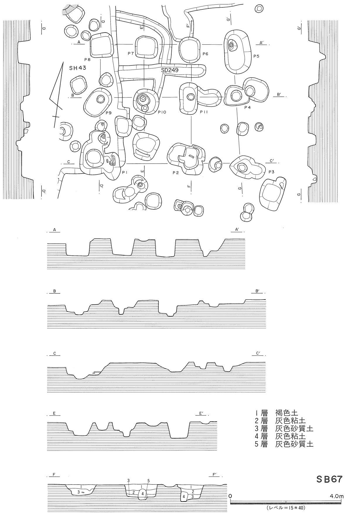
第34図 SB67実測図
