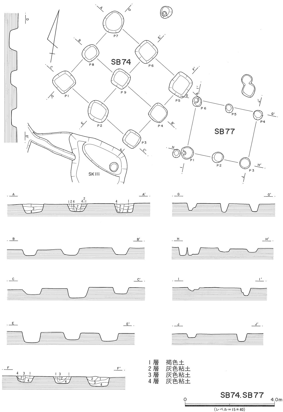
第40図 SB74・SB77実測図
