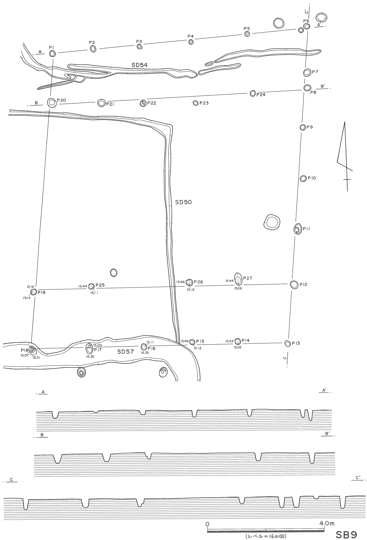
第7図 SB9 実測図
