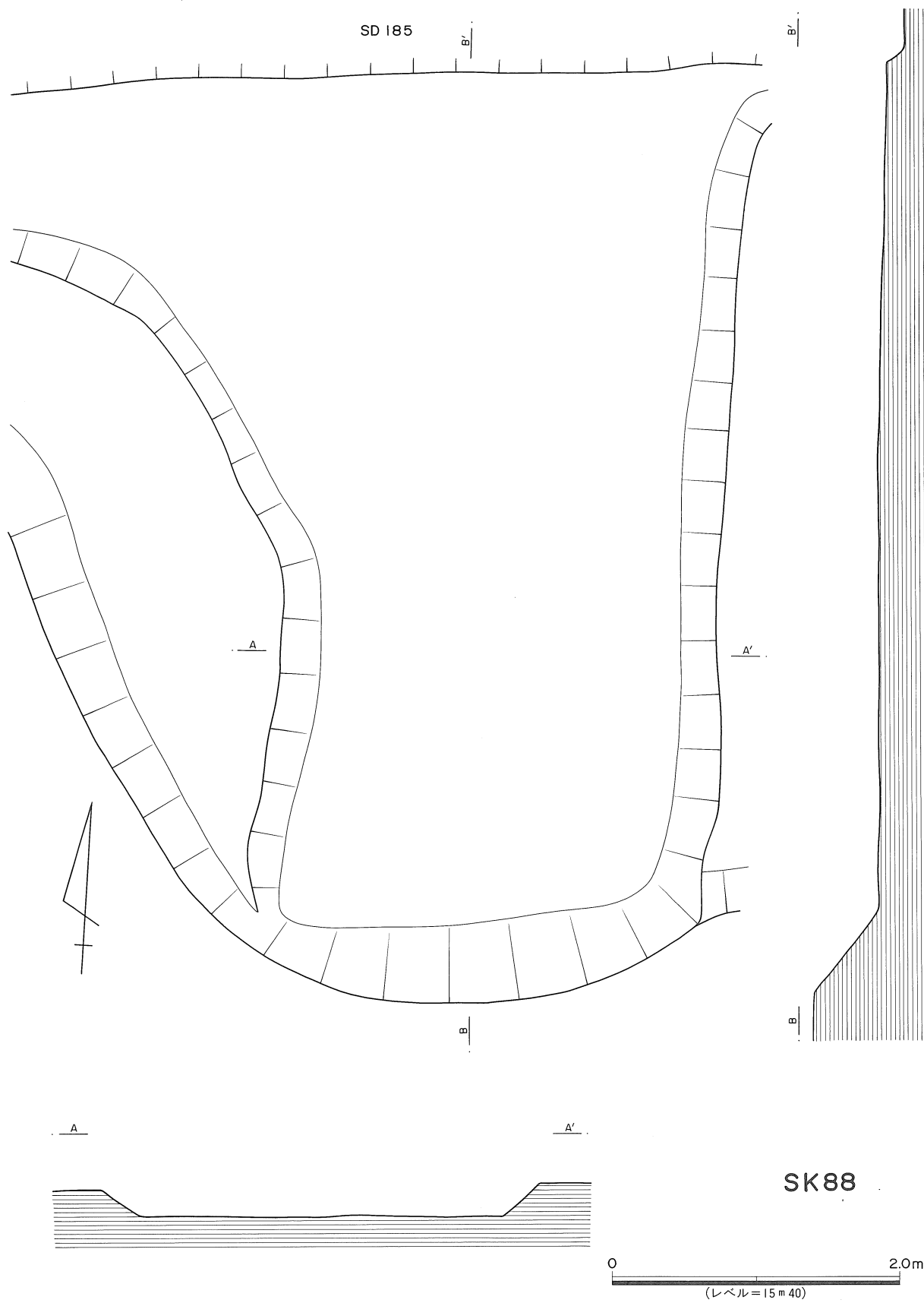
第126図 SK88実測図
