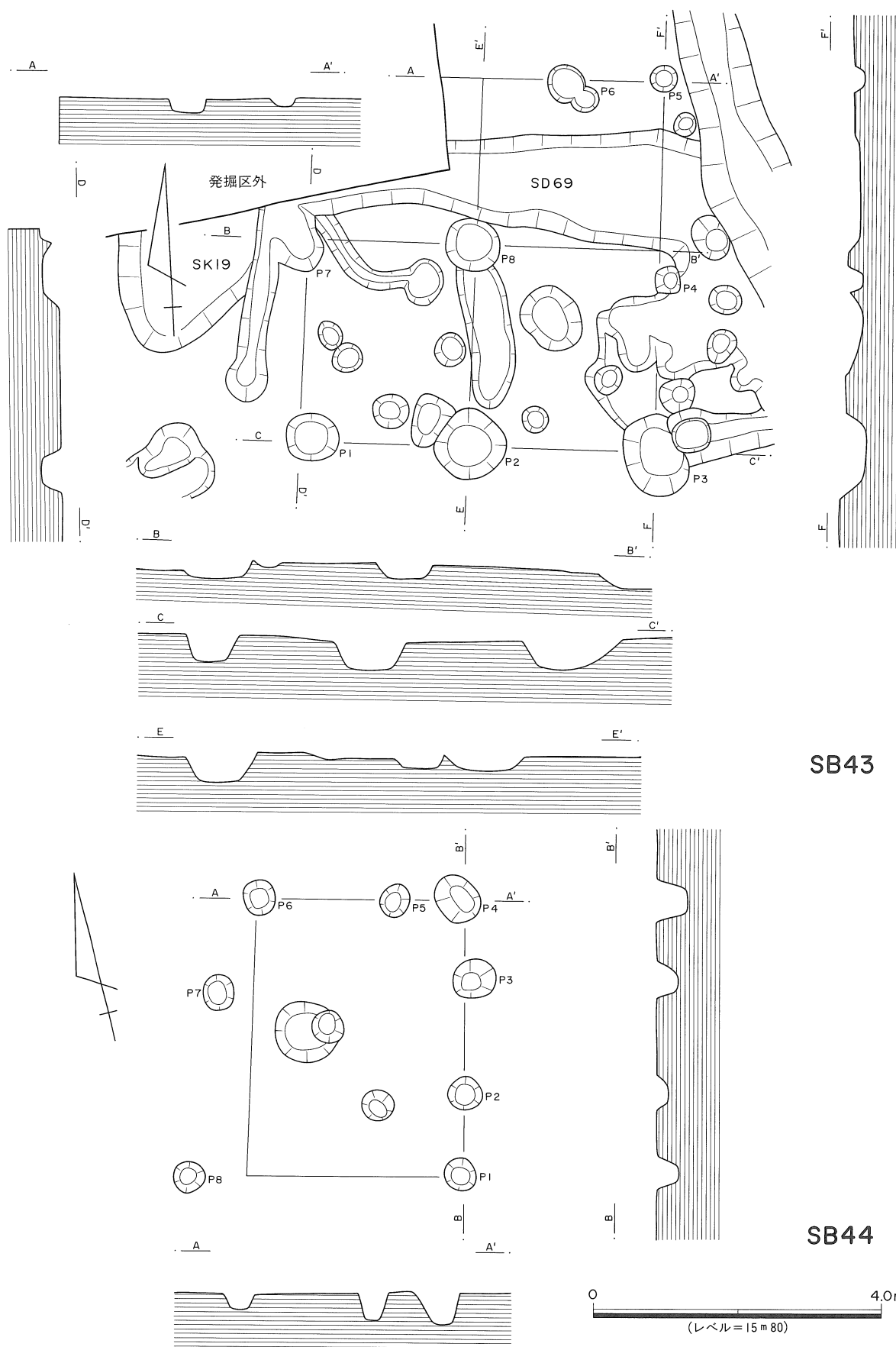
第21図 SB43・SB44実測図
