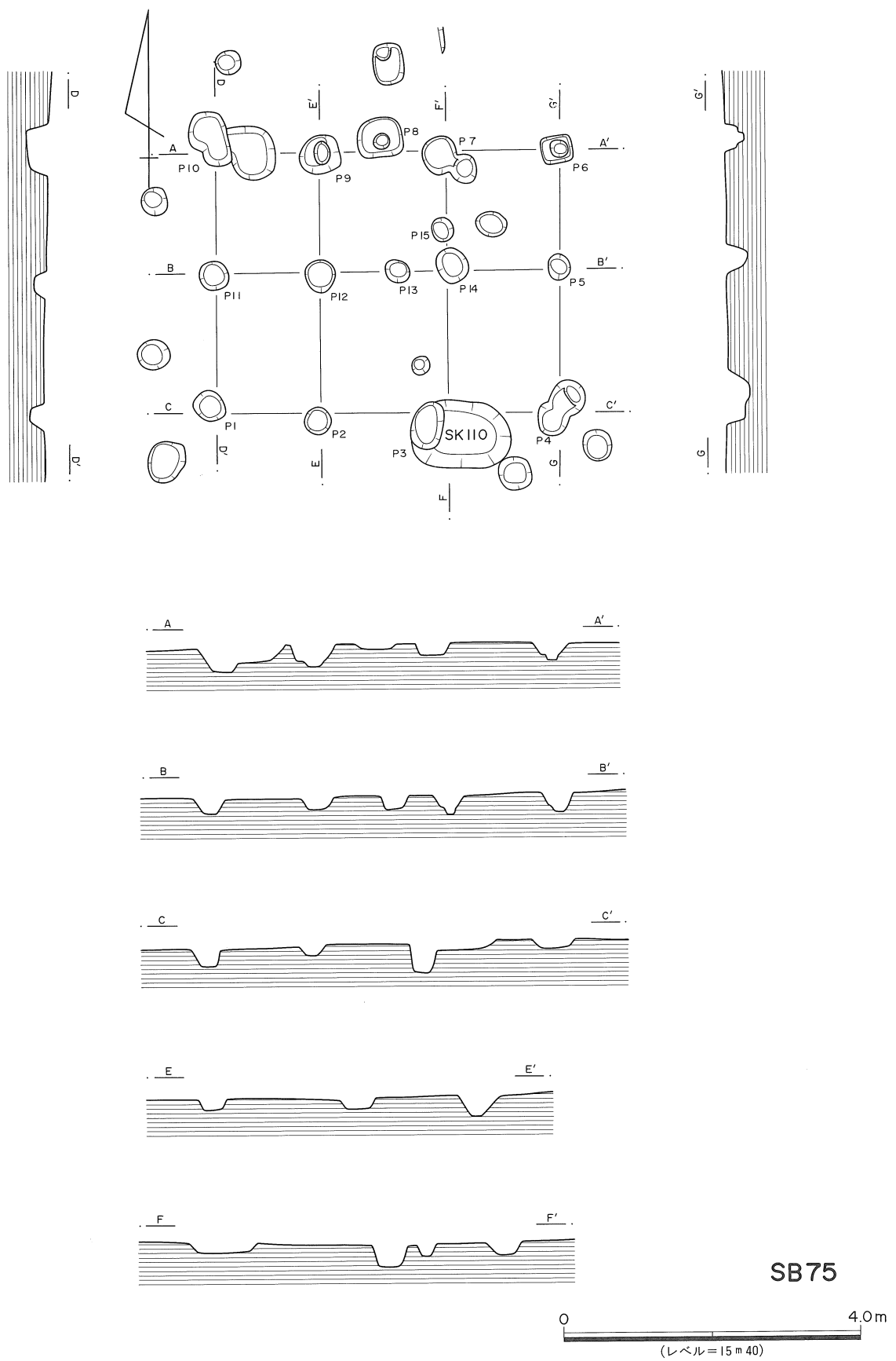
第41図 SB75実測図
