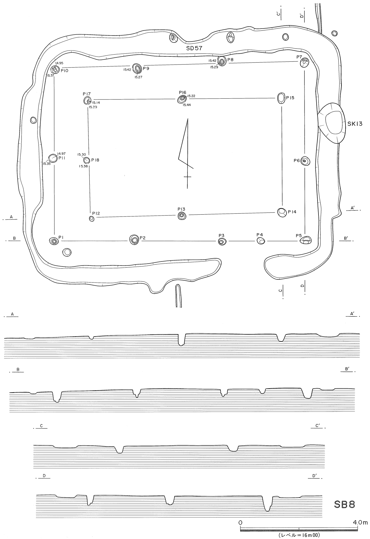
第6図 SB8 実測図
