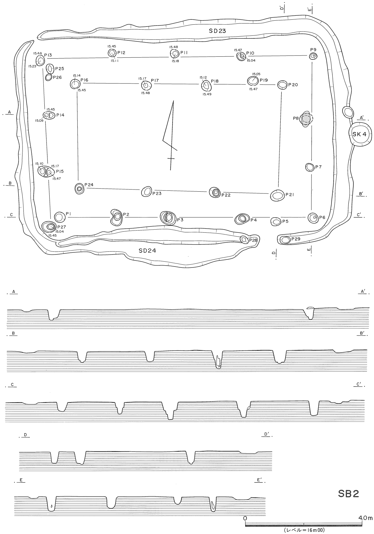
第2図 SB2 実測図
