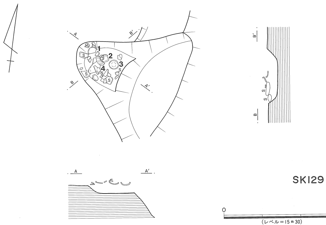
第137図 SD123・SK129実測図
