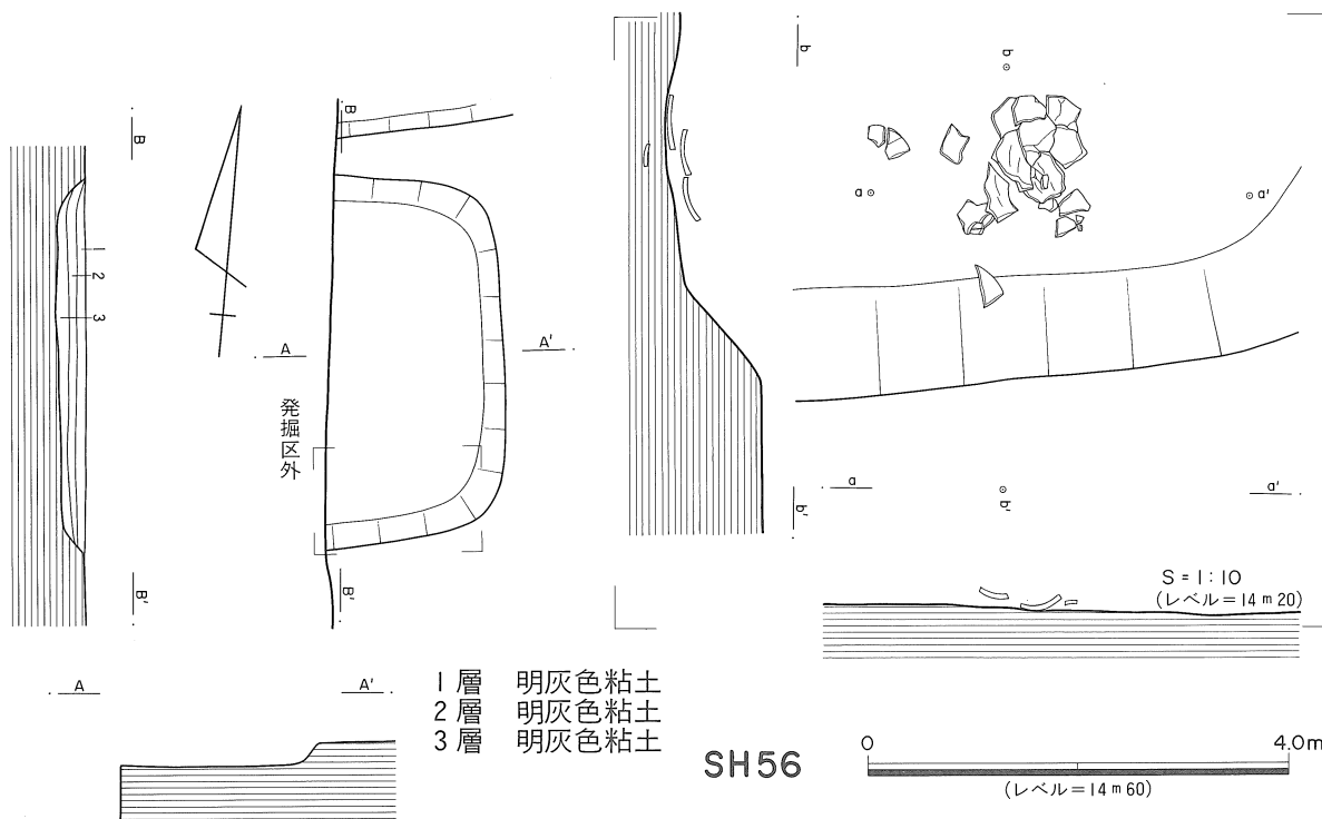
第108図 SH52・SH56実測図
