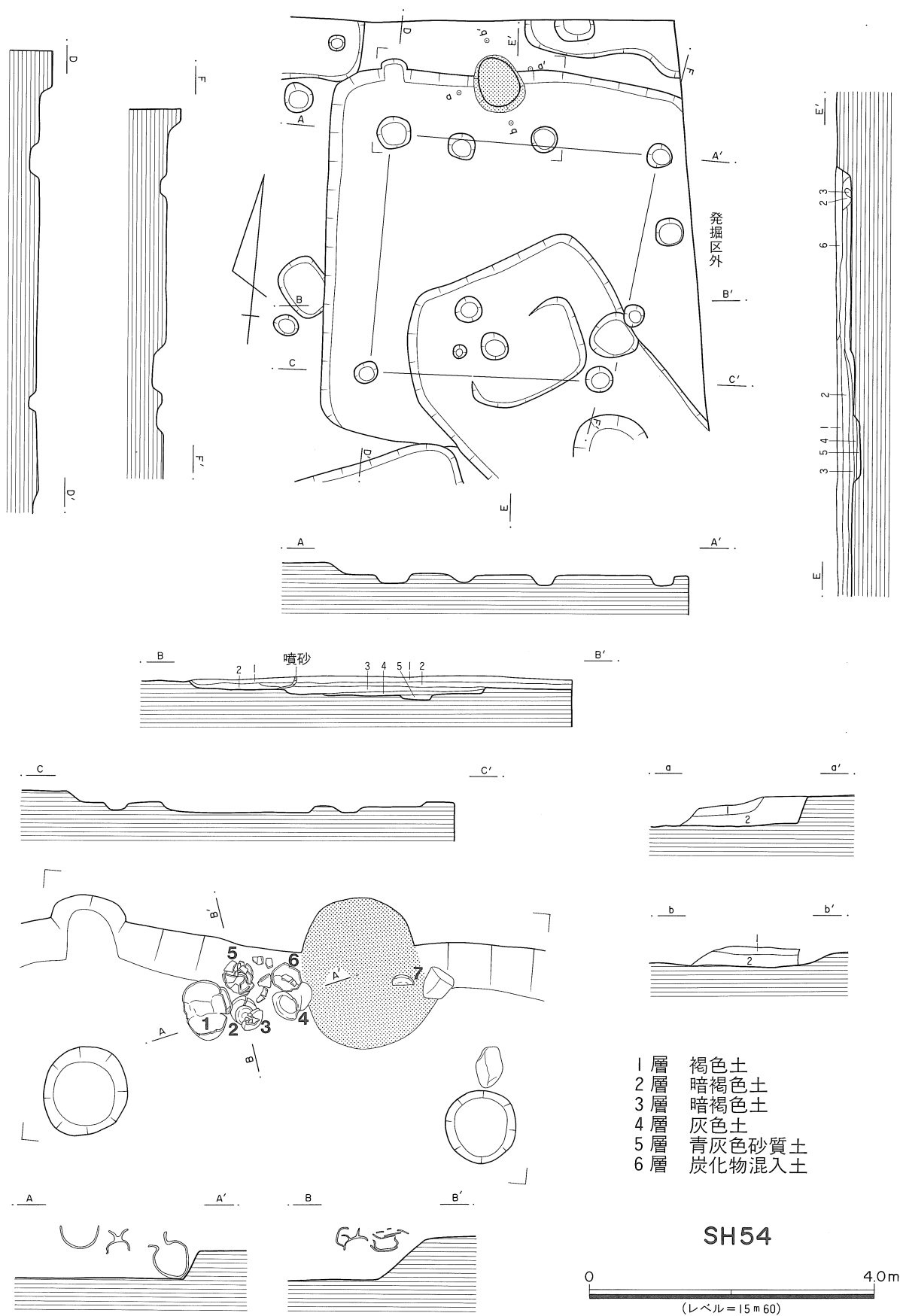
第109図 SH54実測図
