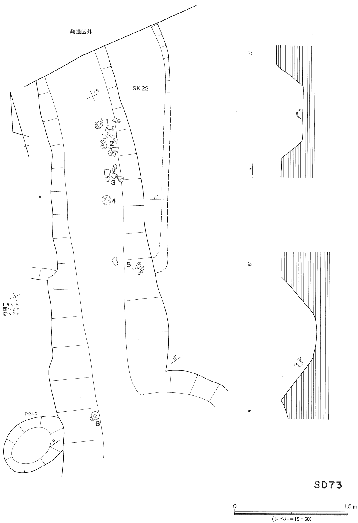
第141図 SD73実測図
