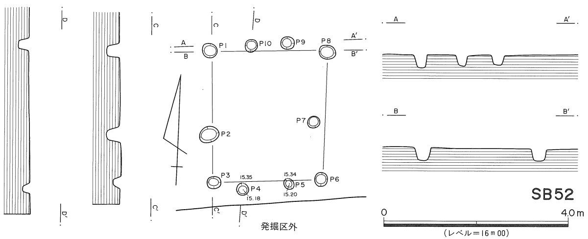
第24図 SB48・SB52実測図
