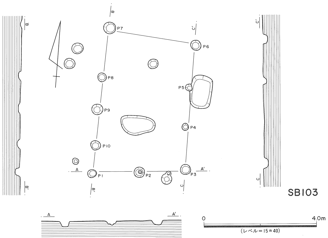
第55図 SB102・SB103実測図
