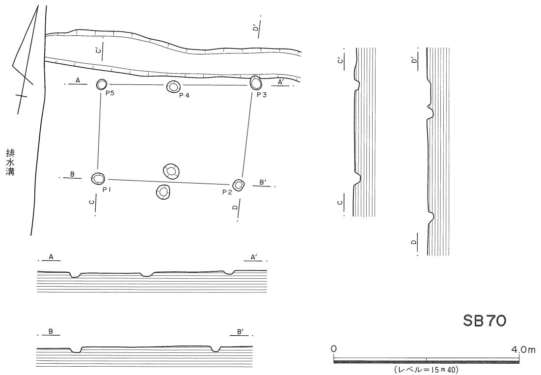
第36図 SB69・SB70実測図
