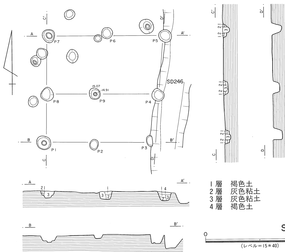
第31図 SB63・SB65実測図
