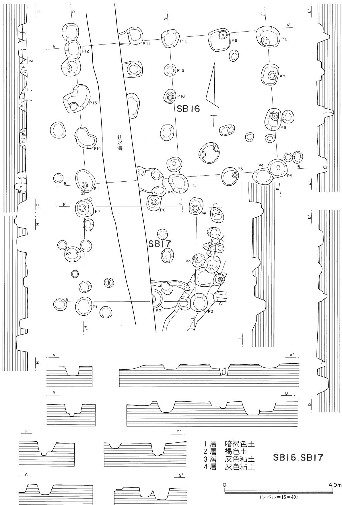
第11図 SB16・SB17実測図
