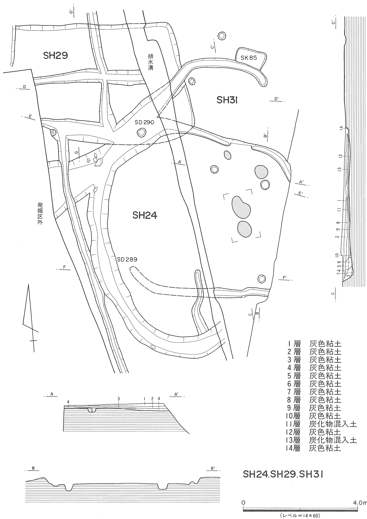
第88図 SH24・SH29・SH31実測図
