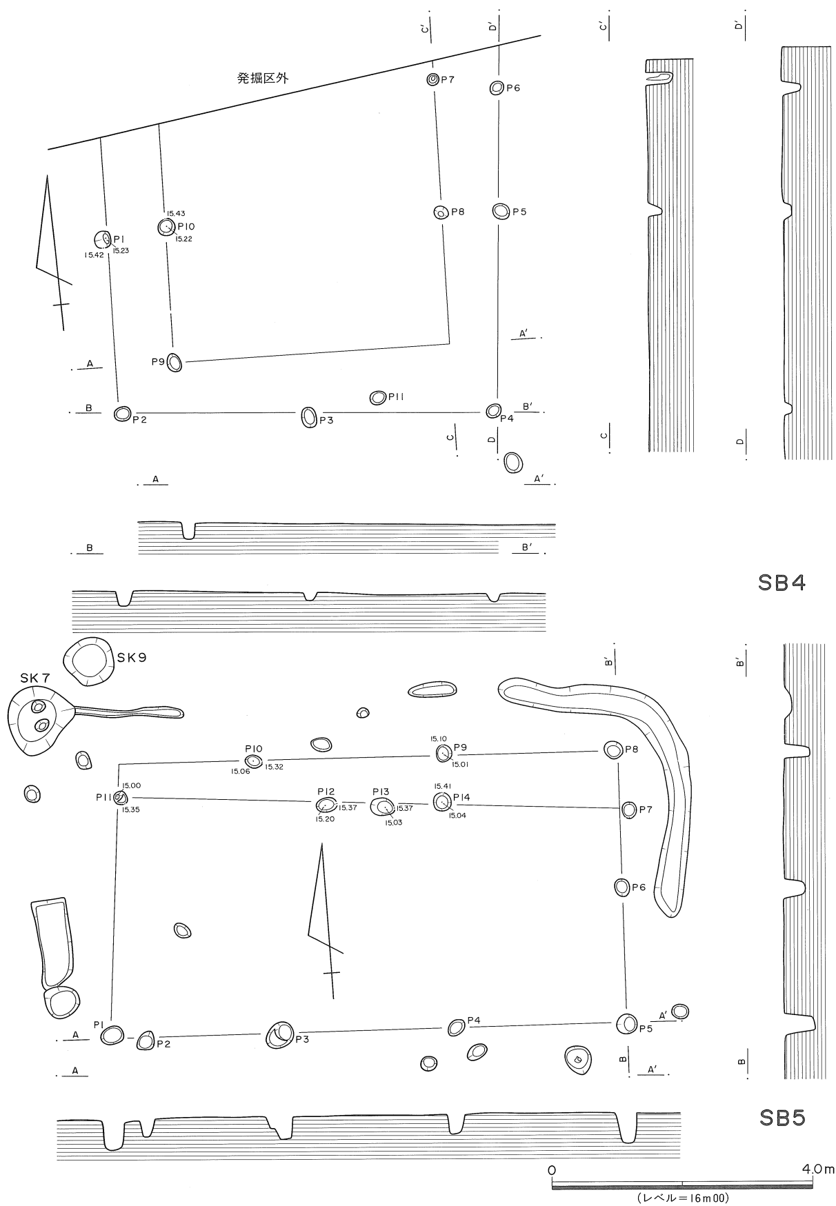
第3図 SB4・SB5実測図
