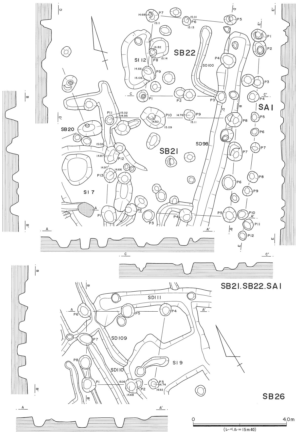
第13図 SB21・SB22・SA1・SB26実測図
