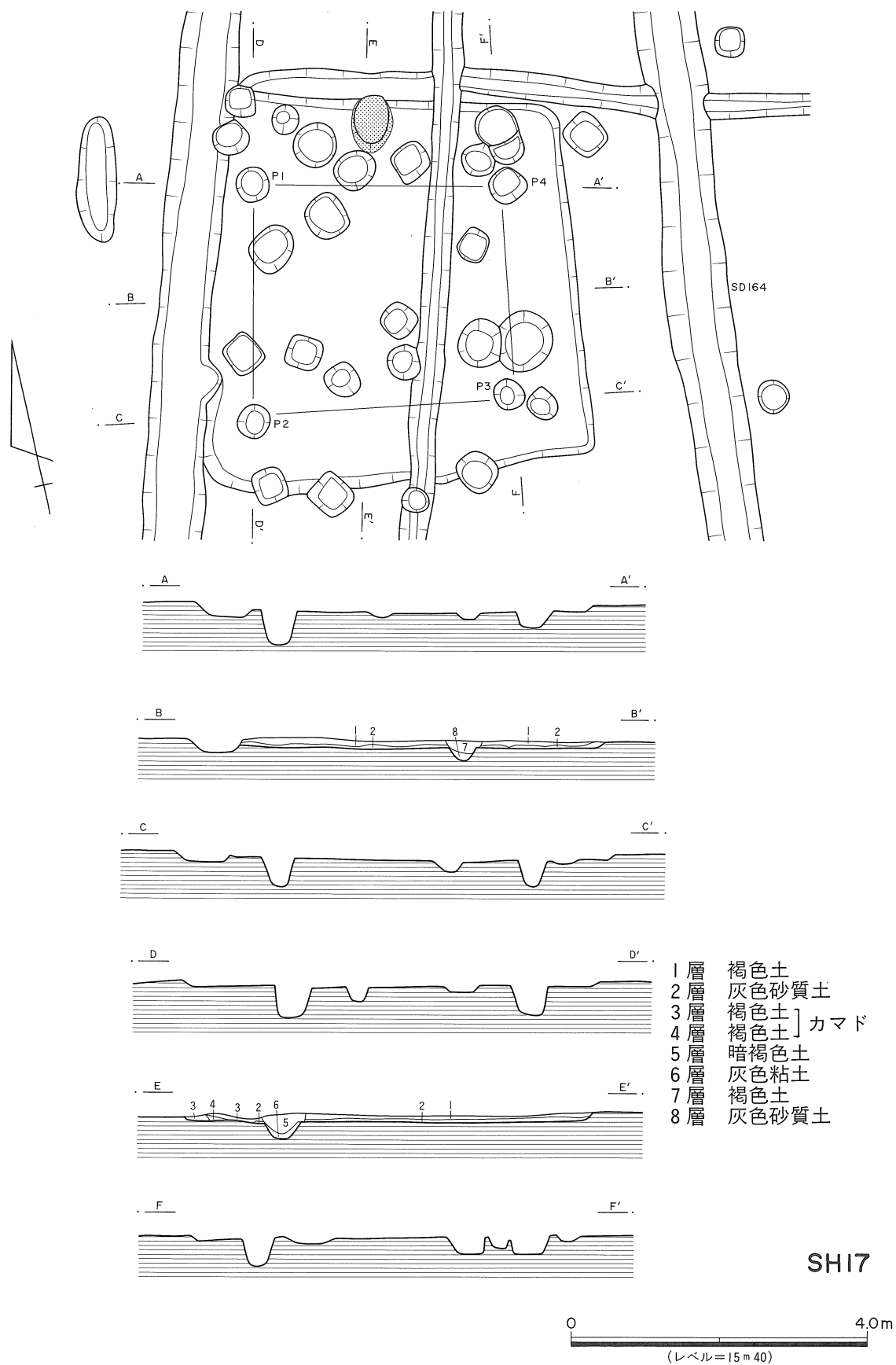
第83図 SH17実測図
