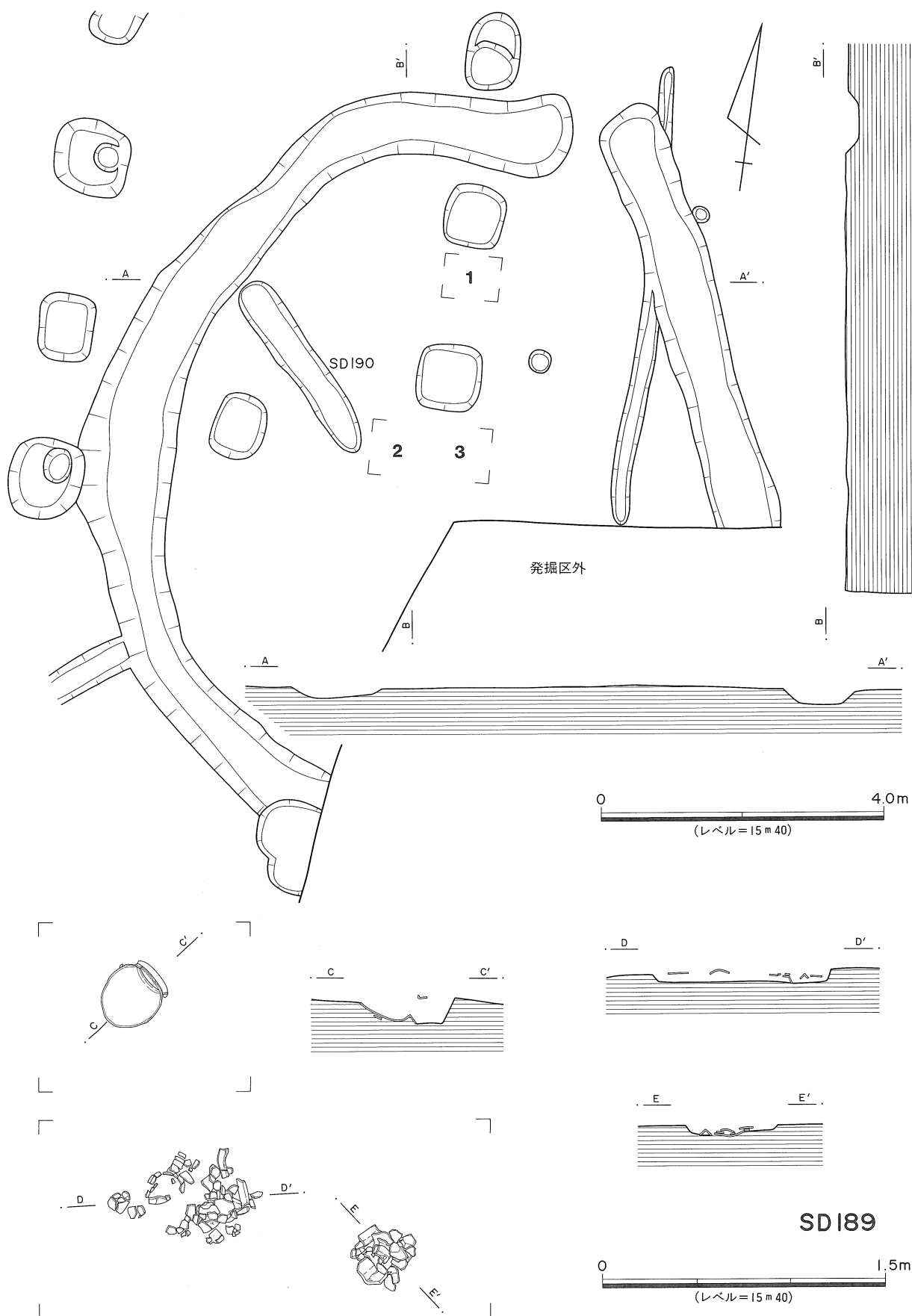
第143図 SD189実測図
