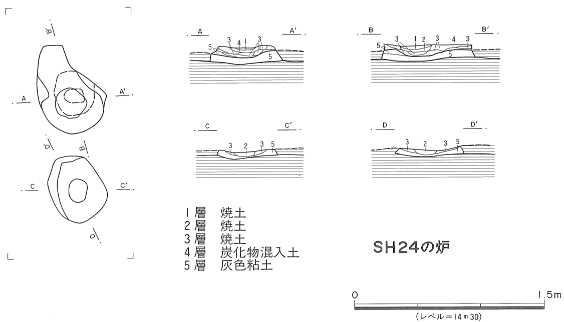
第89図 SH24・SH29・SH31実測図
