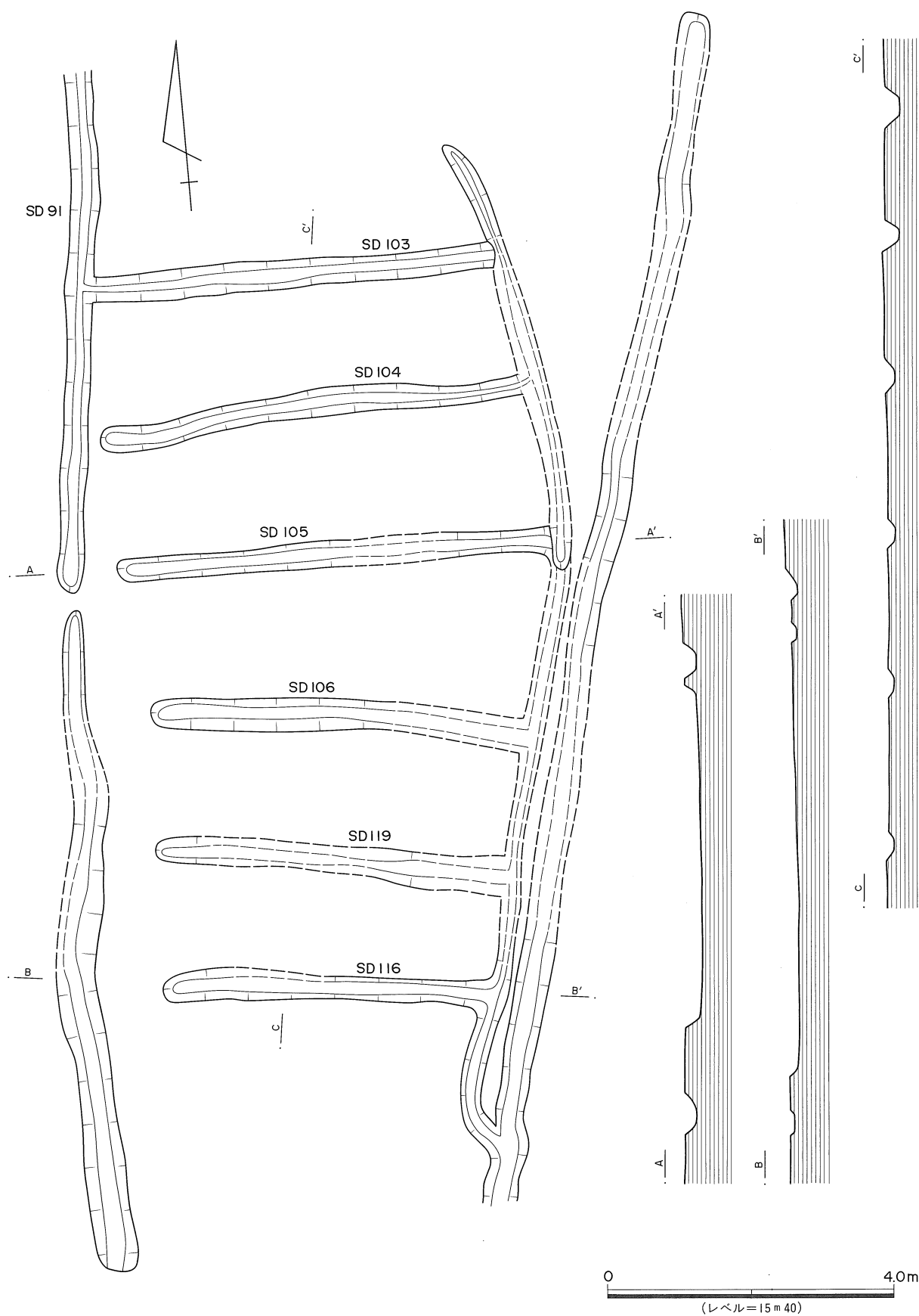
第154図 畝 1 実測図
