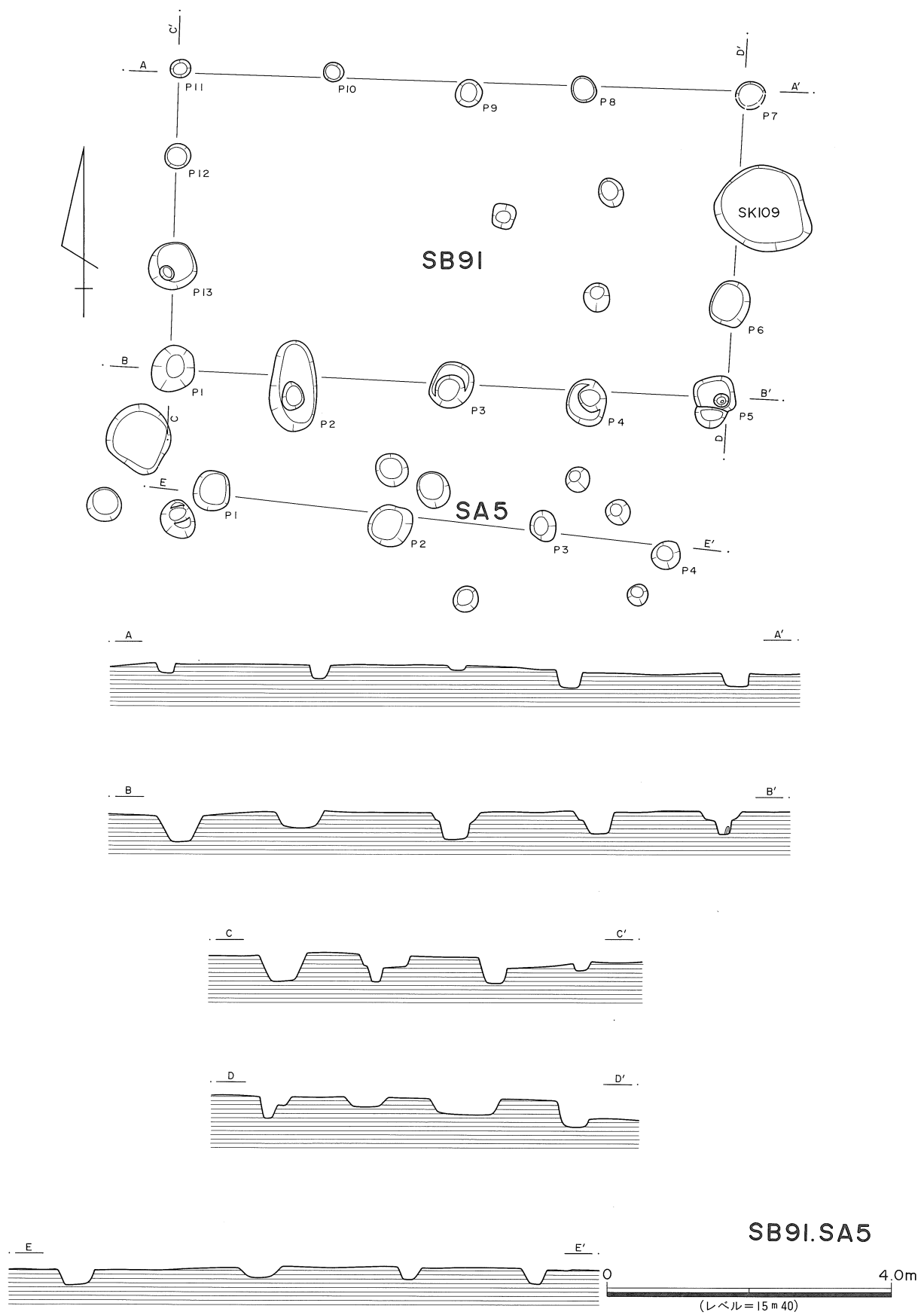
第50図 SB91・SA5 実測図
