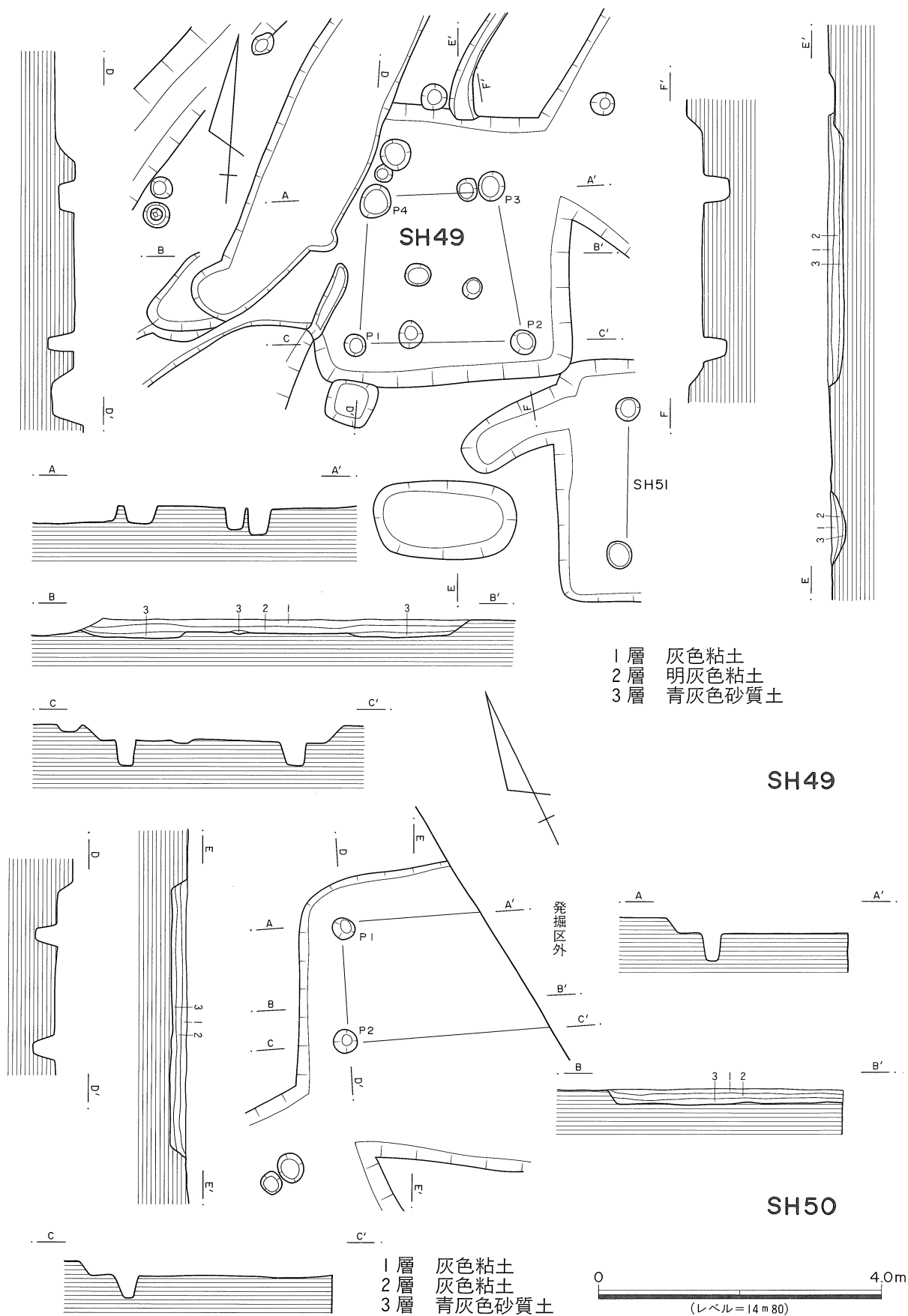
第106図 SH49・SH50実測図
