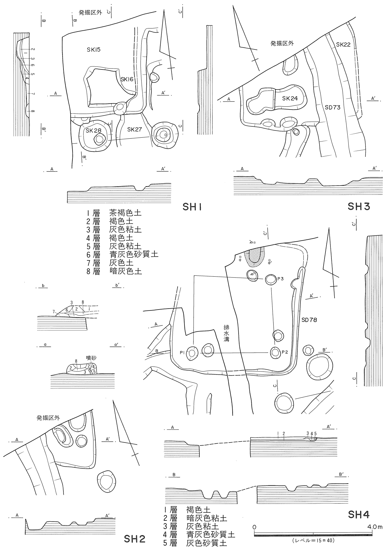
第75図 SH1・SH2・SH3・SH4実測図
