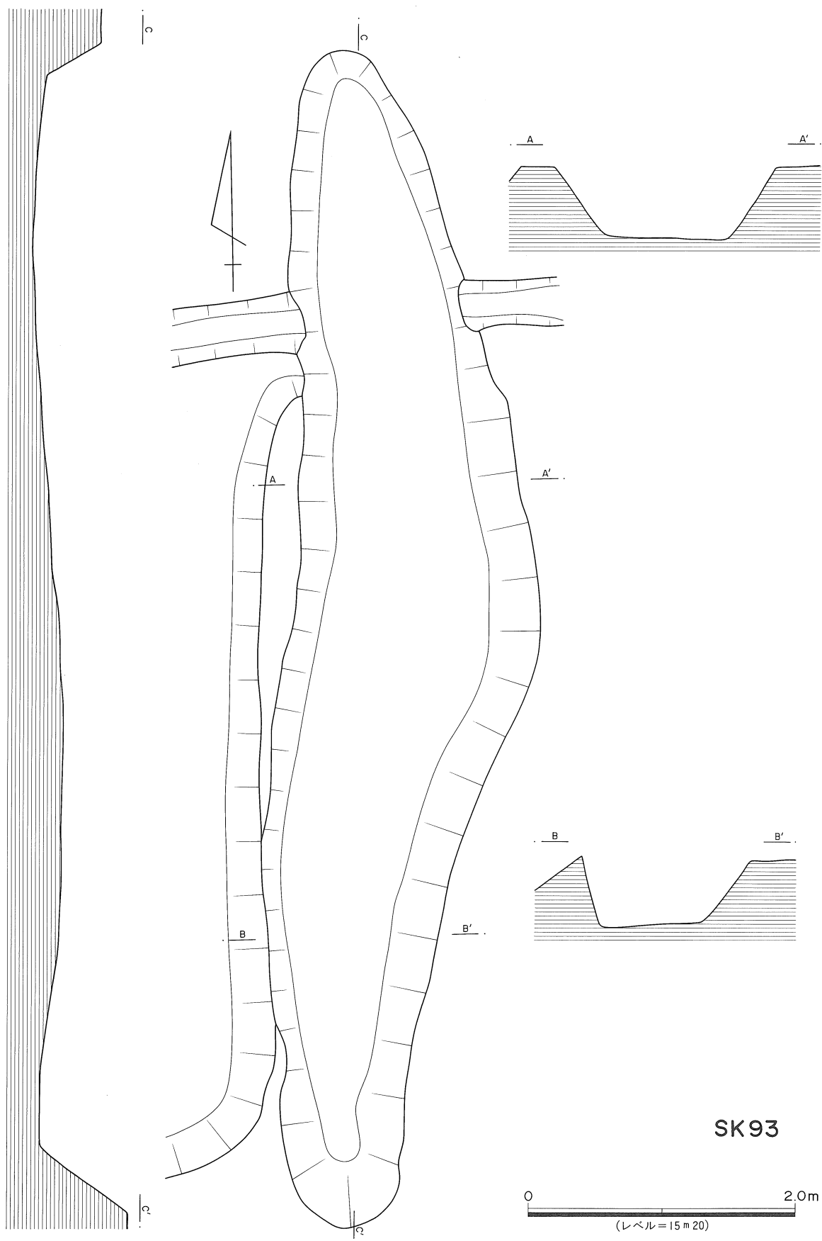
第128図 SK93実測図
