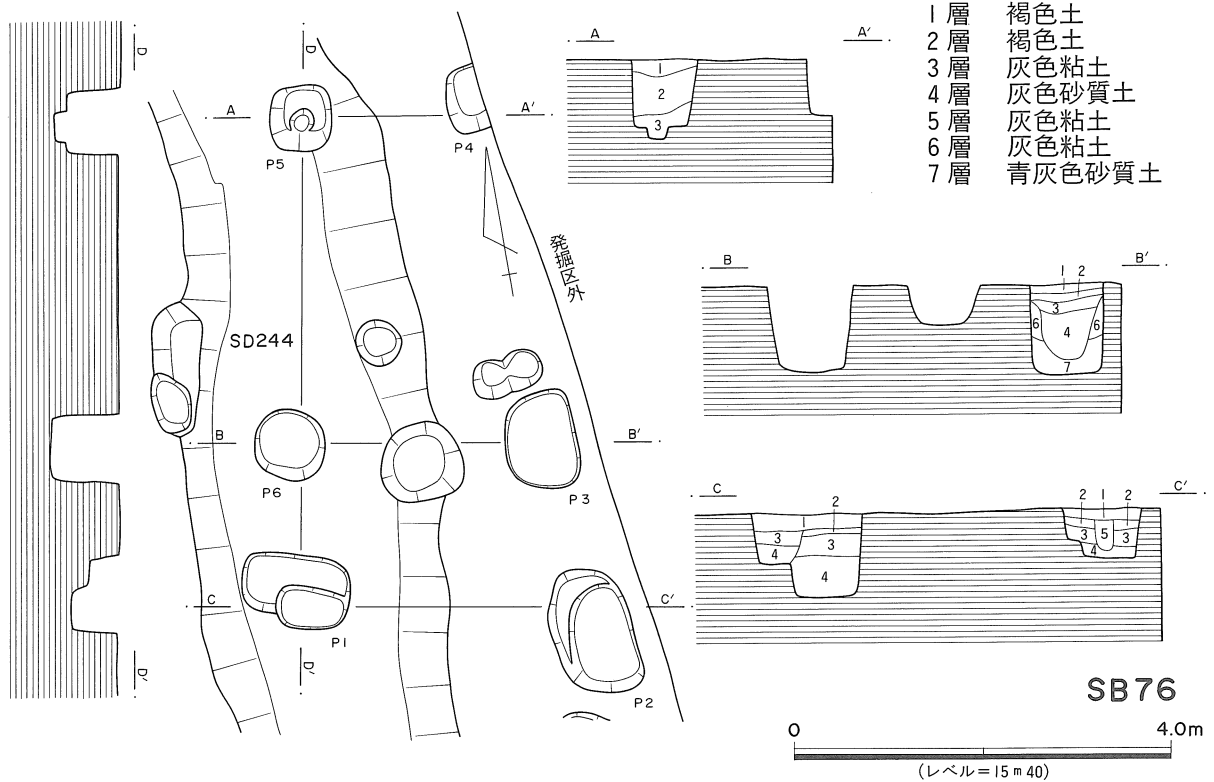
第38図 SB72・SB76実測図
