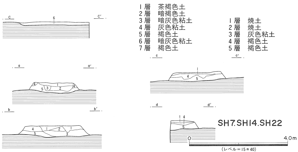
第77図 SH 7・SH14・SH22実測図
