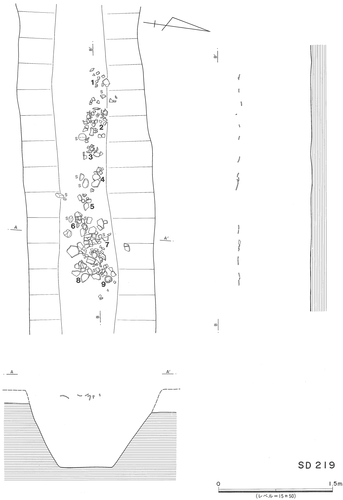
第145図 SD219実測図
