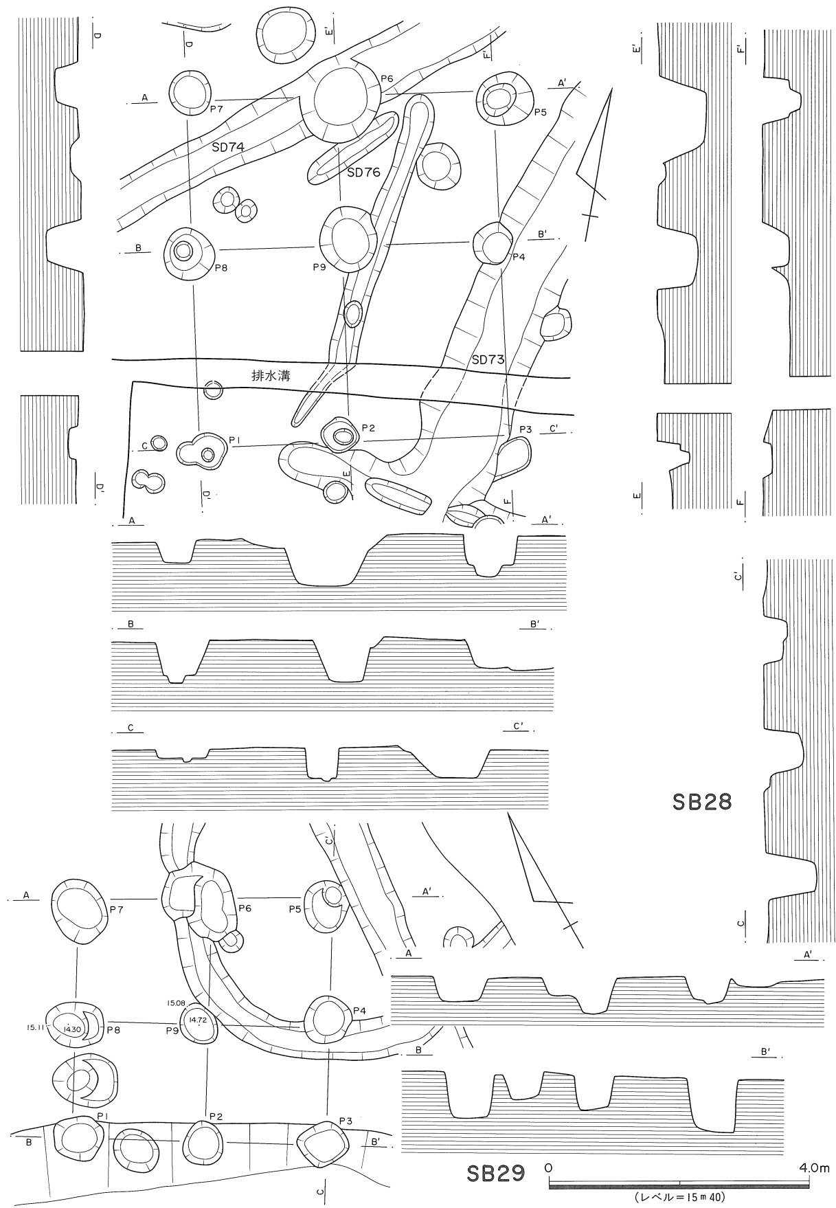
第15図 SB28・SB29実測図
