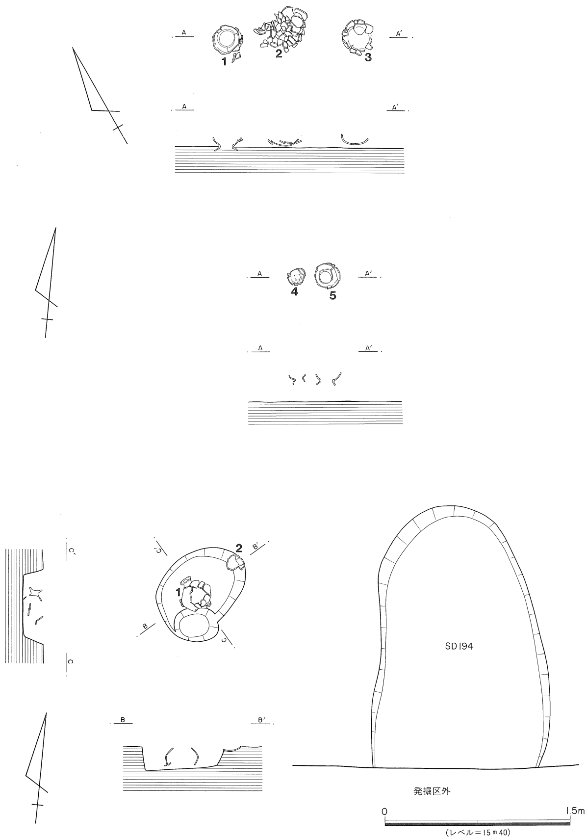
第144図 SD189・SD194実測図
