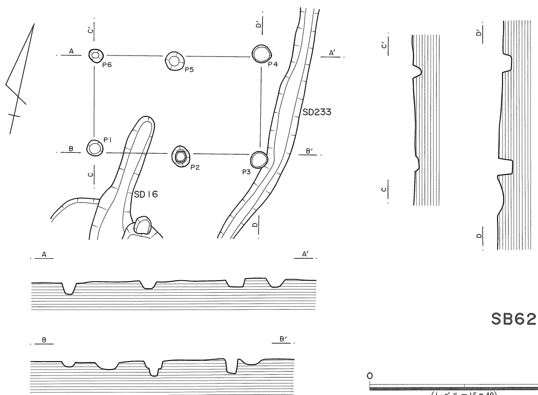
第30図 SB61・SB62実測図
