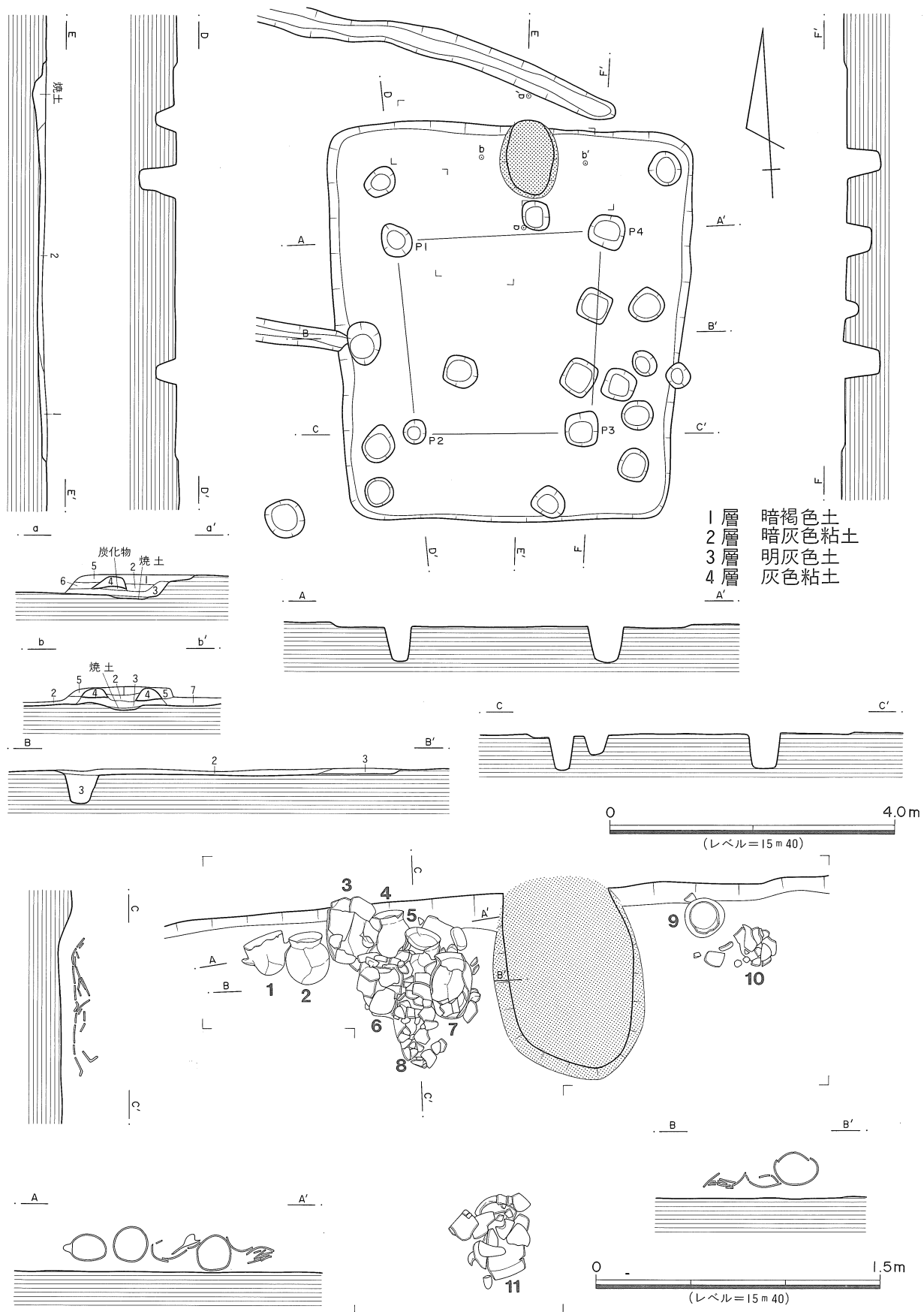
第84図 SH18実測図
