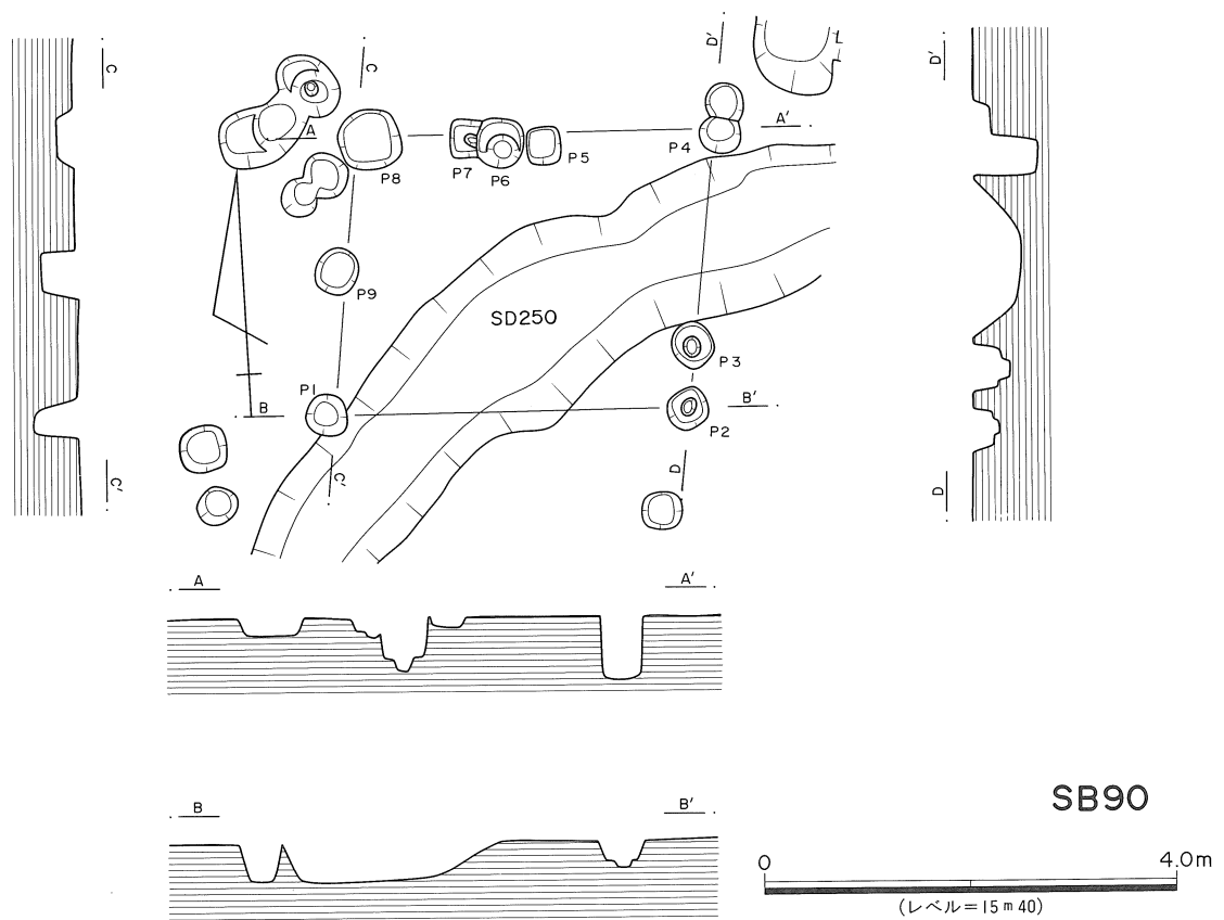
第49図 SB89・SB90実測図
