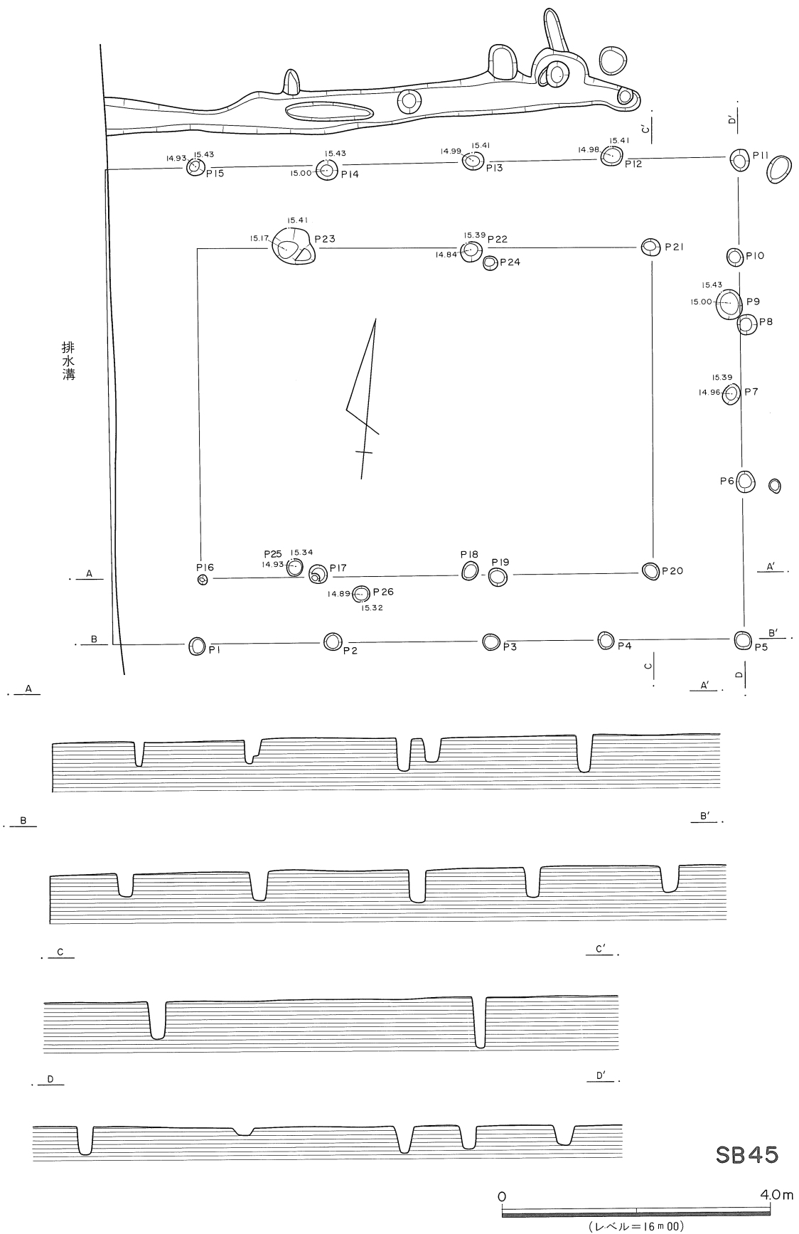
第22図 SB45実測図
