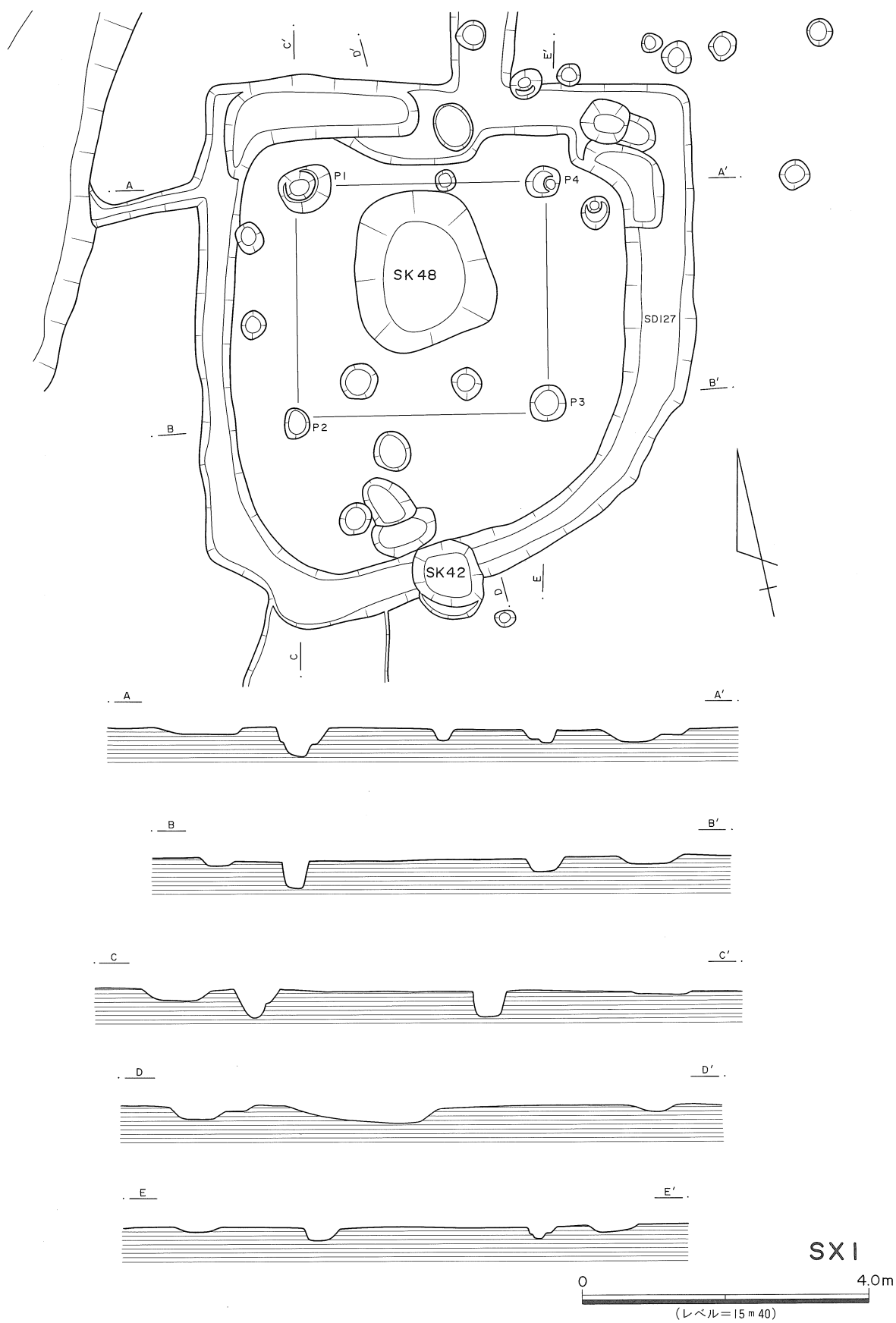
第73図 SX1 実測図
