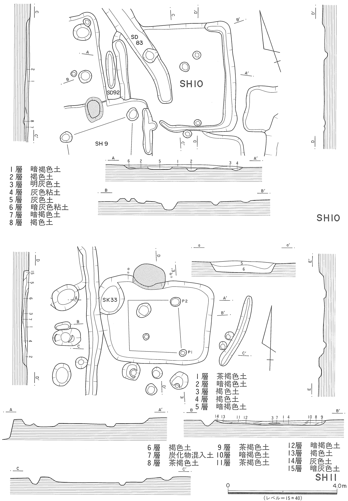
第80図 SH10・SH11実測図
