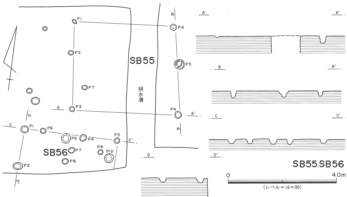
第27図 SB53・SB55・SB56実測図
