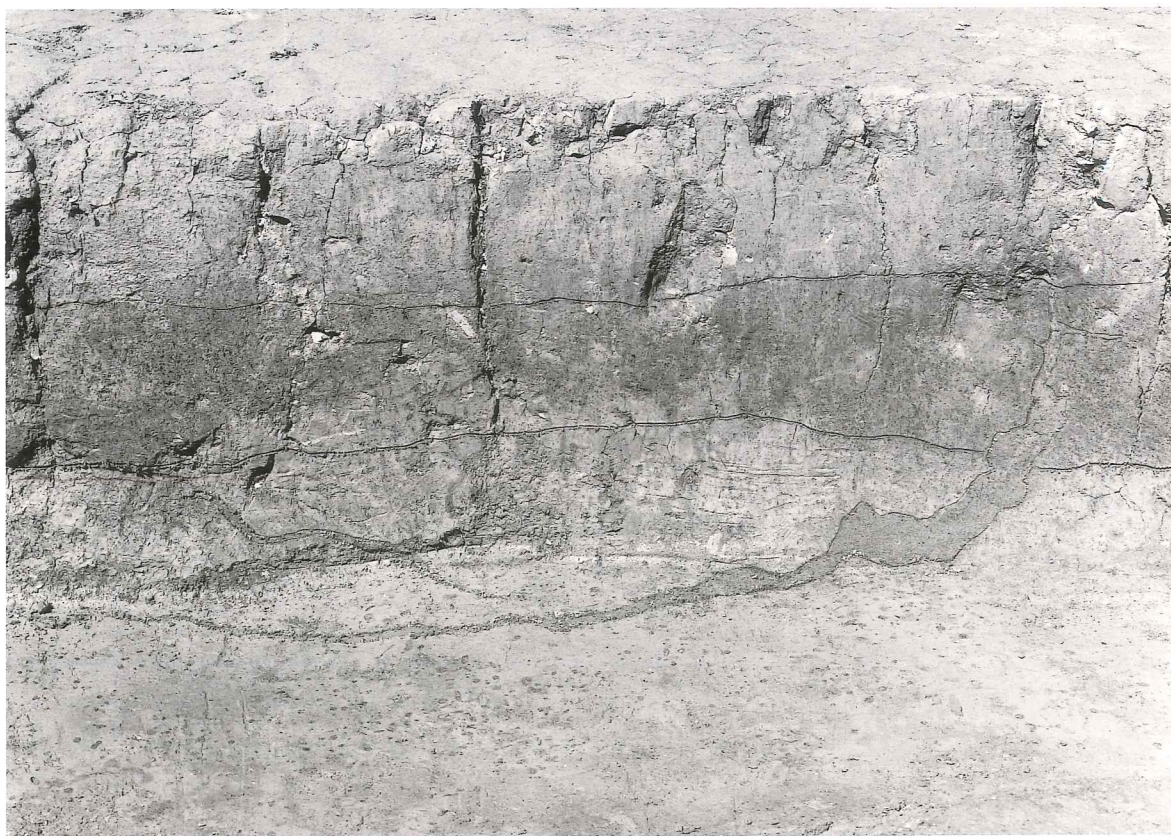
噴砂検出状況
