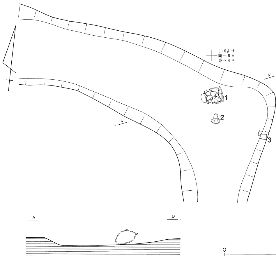
第142図 SD82・SD150実測図
