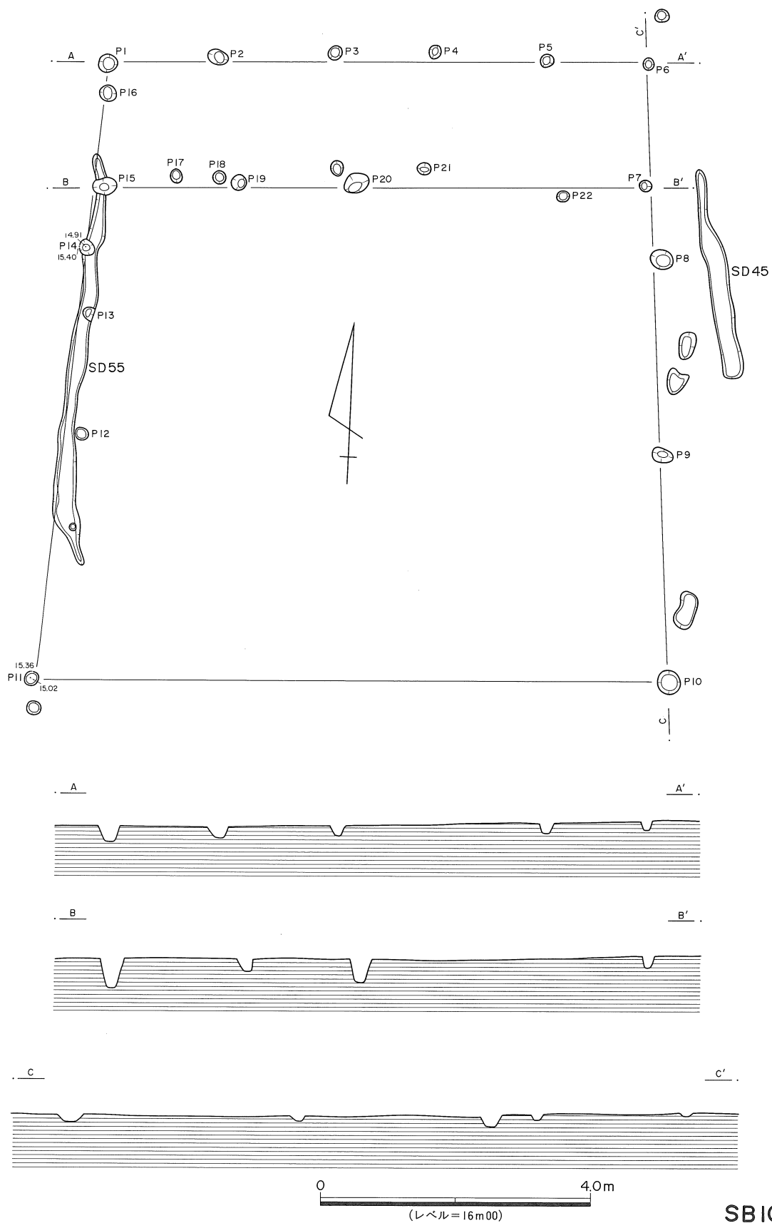
第8図 SB10実測図
