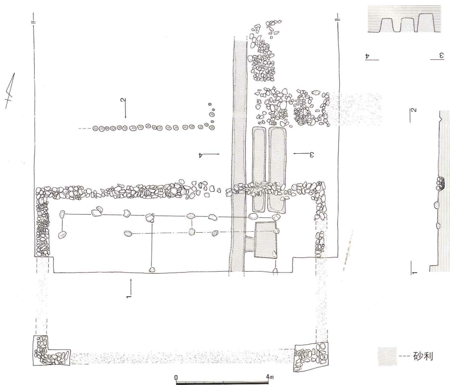
第4図 平成4年度調査区平面図
