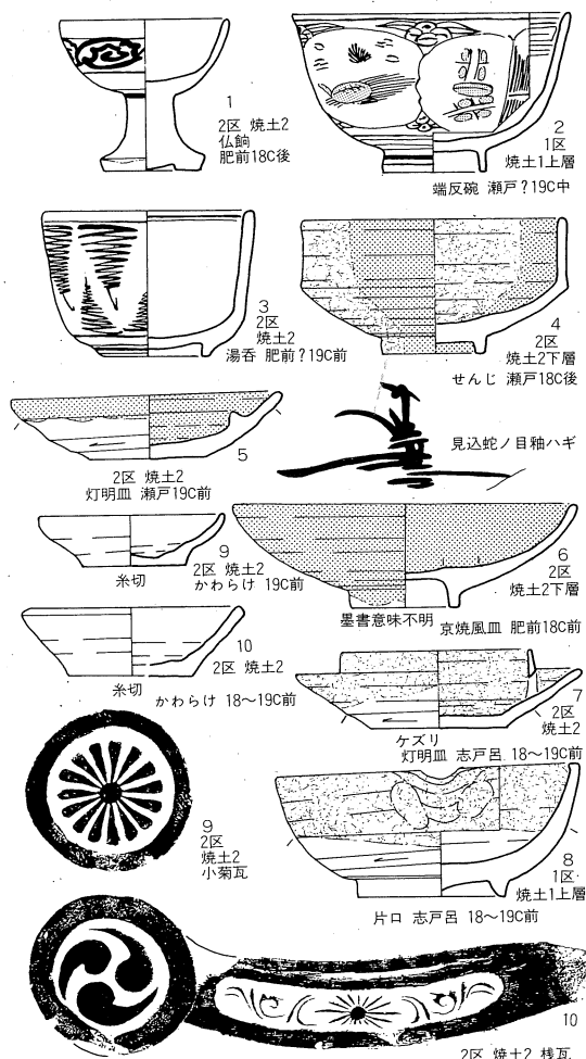
第6図 代表的な出土品実測図（陶磁器縮尺=1/3 瓦縮尺=1/4） 【松井一明】
