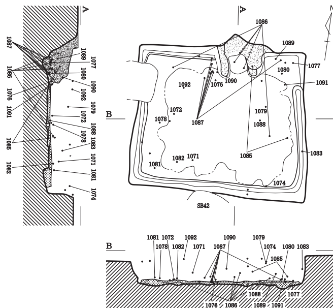
1. N51-S I 307実測図 (1/80)
