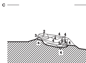
2. N51-S I 306竈実測図 (1/40)
