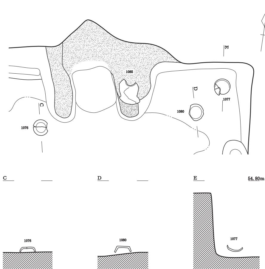
2. N51-S I 307遺物出土状況図 (1/20)
