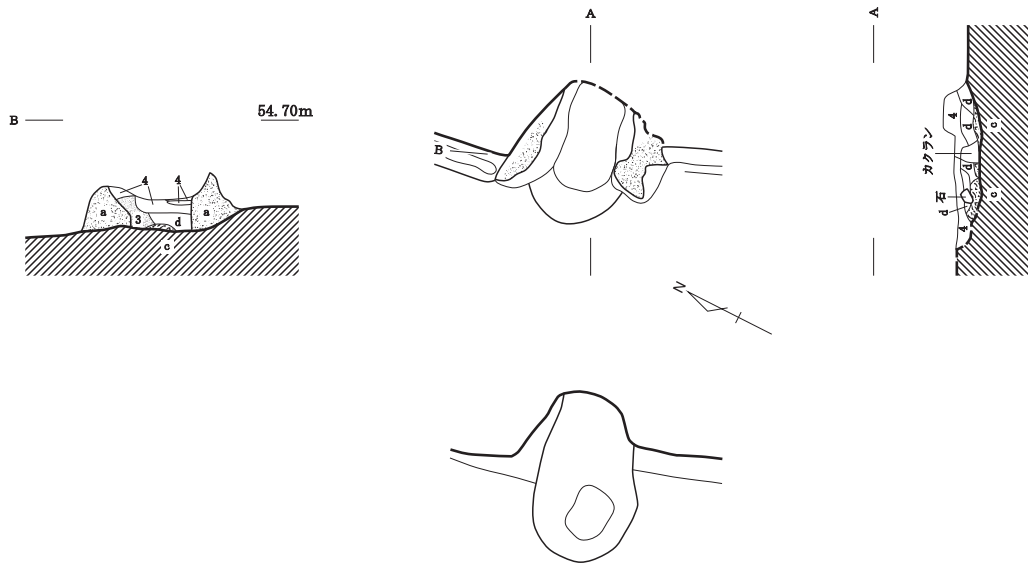
1. N51-S I 301竈実測図 (1/40)
