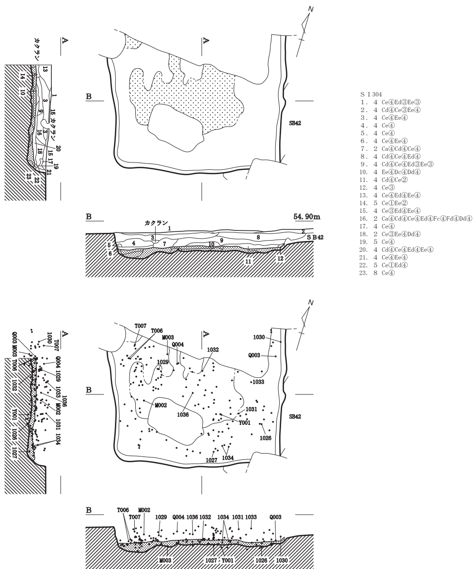
1. N51-S I 304実測図 (1/80)
