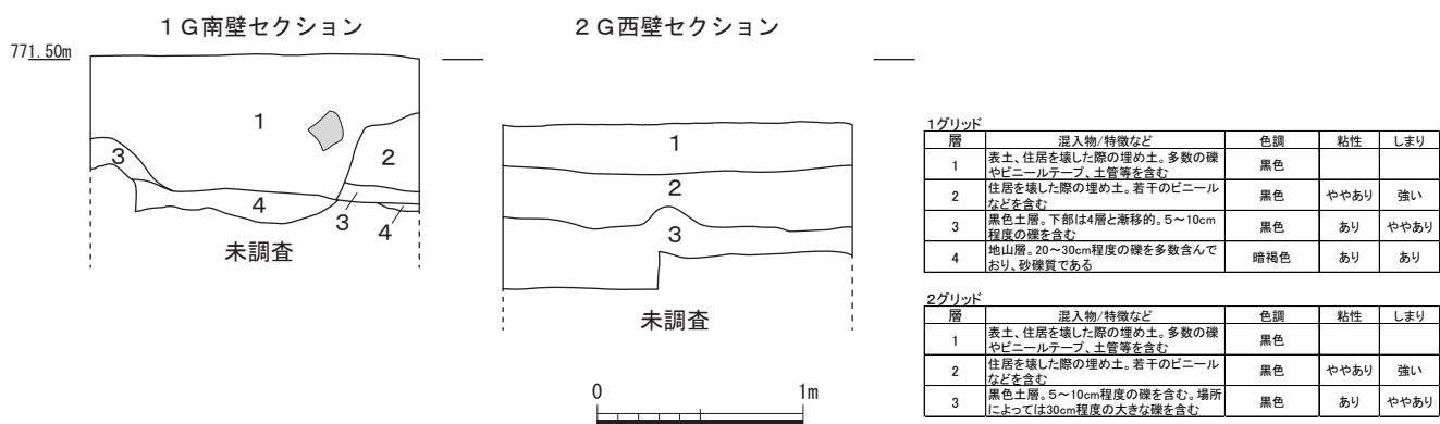
第 15 図 土層断面図 (S=1/40)
