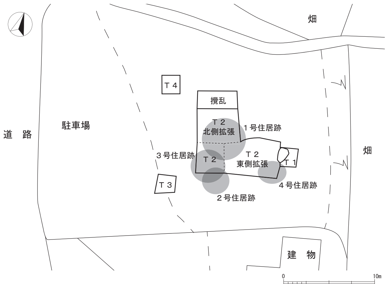
第10図 調査区設定図 (S=1/250)
