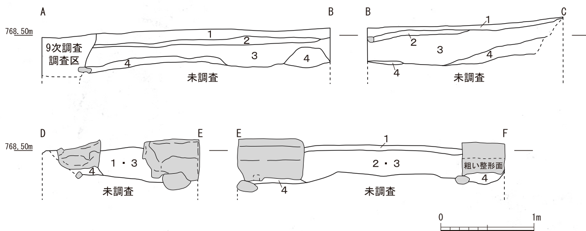
第7図 土層断面図 (S=1/40)
