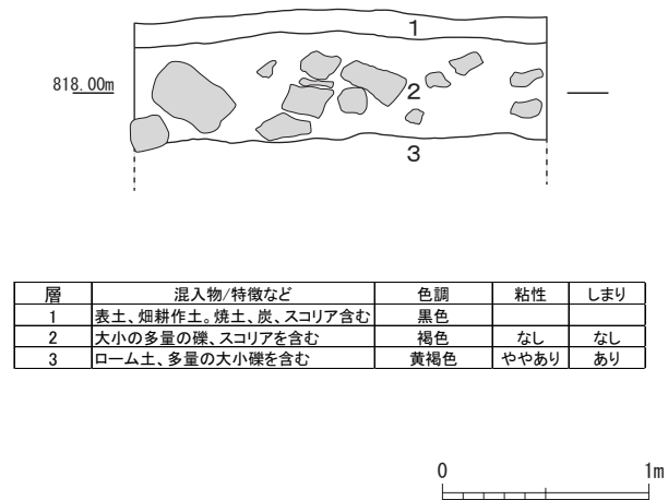
第4図 土層断面図 (S=1/40)
