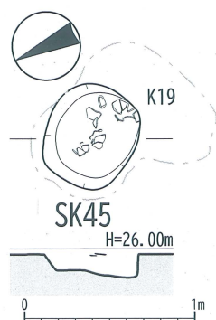
第43図 茶ノ木ノ本遺跡 45号土坑【SK45】〔1/40〕
