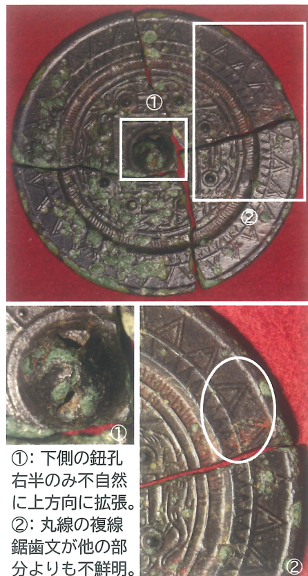
図5 鑄造欠陥
