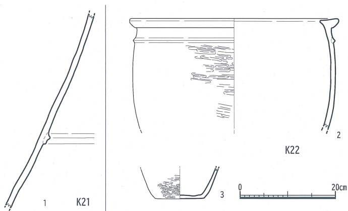
第89図 茶ノ木ノ本遺跡出土遺物 21号、22号甕棺墓【K21, 22】 〔1/8〕
