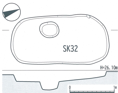
第32図 茶ノ木ノ本遺跡 32号土坑【SK32】 〔1/40〕
