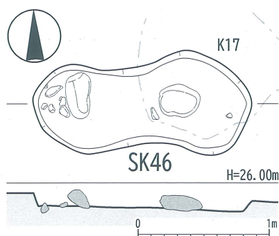
第44図 茶ノ木ノ本遺跡 46号土坑【SK46】 〔1/40〕
