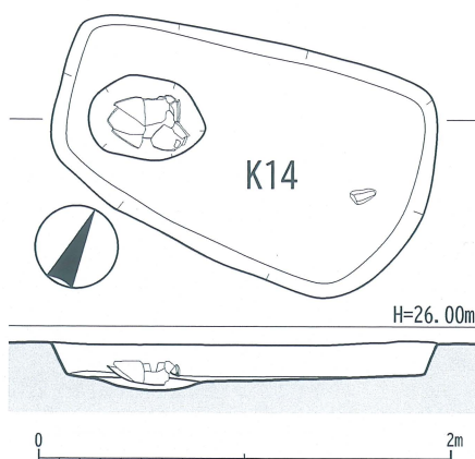
第70図 茶ノ木ノ本遺跡 14号甕棺墓 【K14】〔1/40〕
