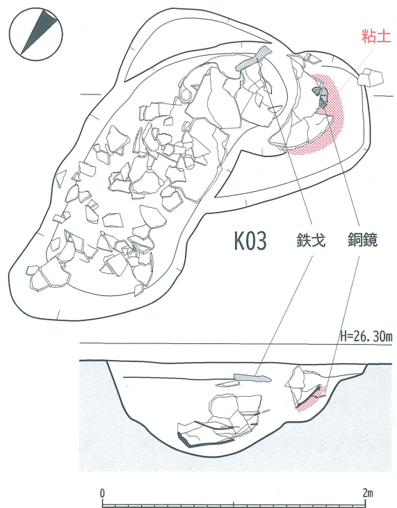
第59図 茶ノ木ノ本遺跡 3号甕棺墓【K03】〔1/40〕
