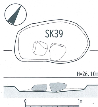
第38図 茶ノ木ノ本遺跡 39号土坑【SK39】〔1/40〕
