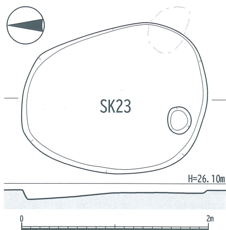
第25図 茶ノ木ノ本遺跡 23号土坑【SK23】 〔1/40〕
