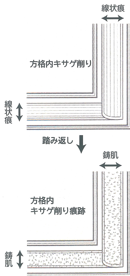
図3 キサゲ削り痕跡の発生過程
