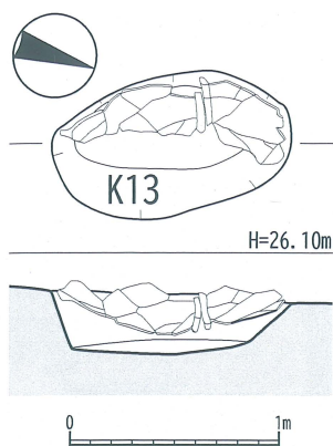
第69図 茶ノ木ノ本遺跡 13号甕棺墓【K13】 〔1/40〕
