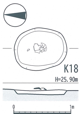
第74図 茶ノ木ノ本遺跡 18号甕棺墓 【K18(SK38)】〔1/40〕
