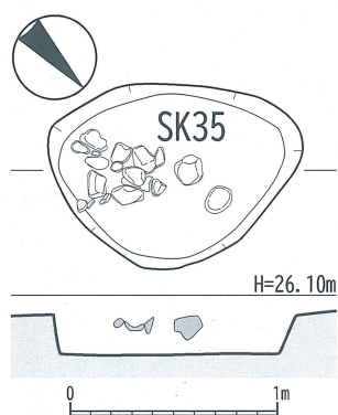
第35図 茶ノ木ノ本遺跡 35号土坑【SK35】〔1/40〕
