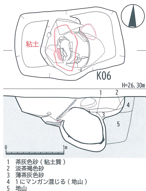
第62図 茶ノ木ノ本遺跡 6号甕棺墓【K06】 〔1/40〕
