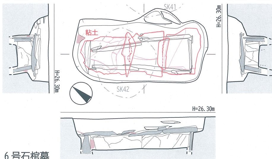
第55図 茶ノ木ノ本遺跡 6号石棺墓【ST06】〔1/40〕
