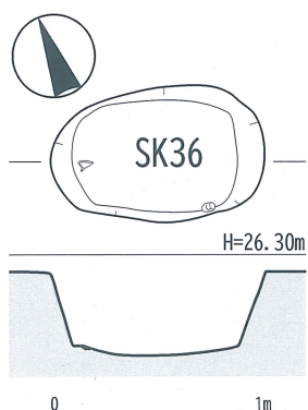
第36図 茶ノ木ノ本遺跡 36号土坑【SK36】〔1/40〕
