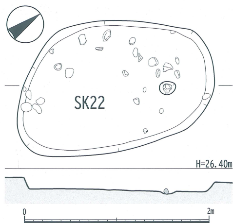
第24図 茶ノ木ノ本遺跡 22号土坑【SK22】 〔1/40〕
