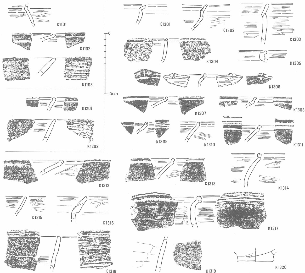
Fig.27 土壌出土土器実測図3 <SK11~13> (1/3)
