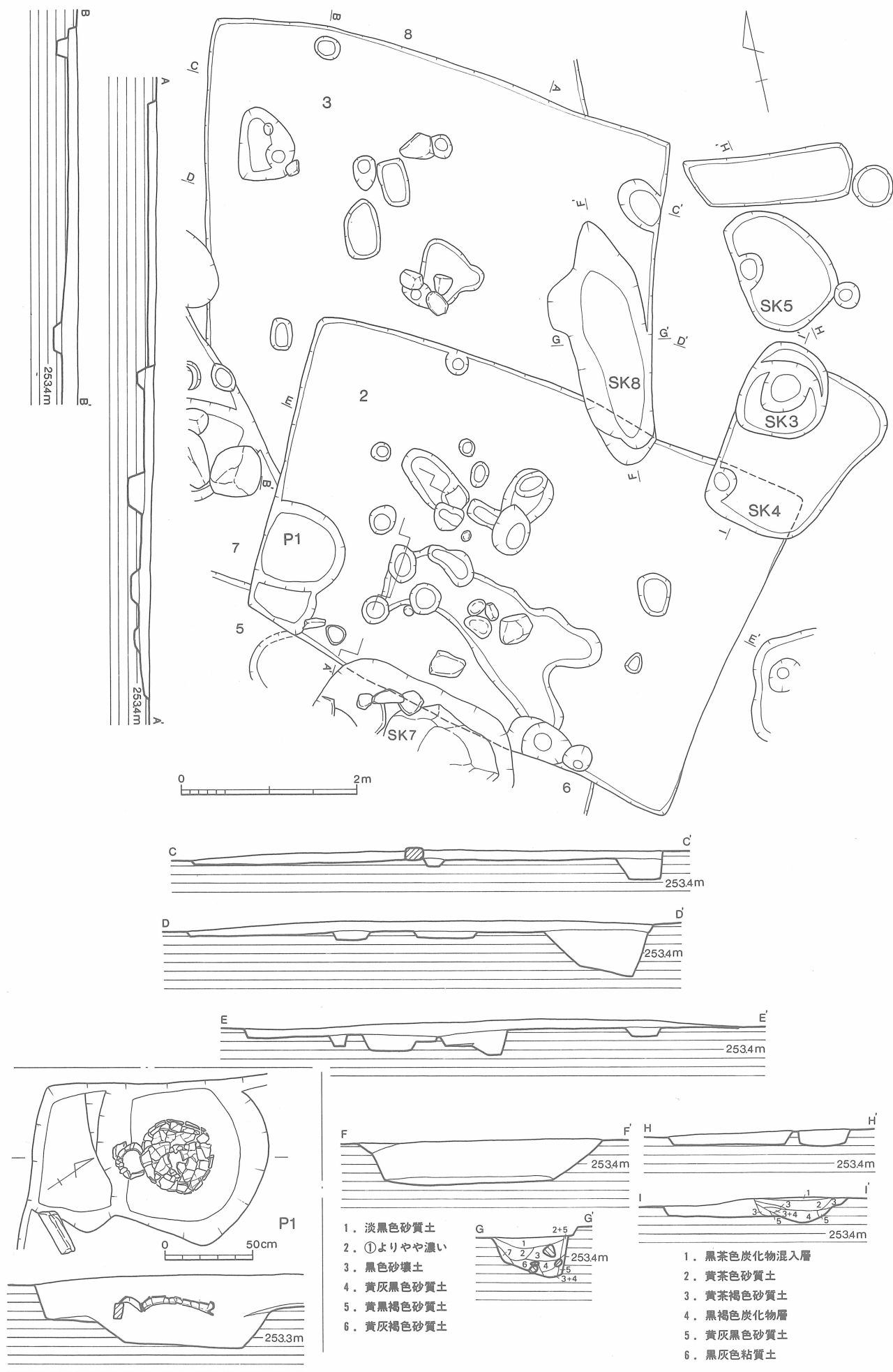
Fig. 7 2・3号住居跡、SK3～5・8、2号住居跡P1土器出土状態実測図 (1/60・1/30)
