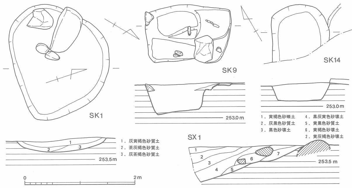
Fig.12 SK1・9・14、SX1土層実測図 (1/40)
