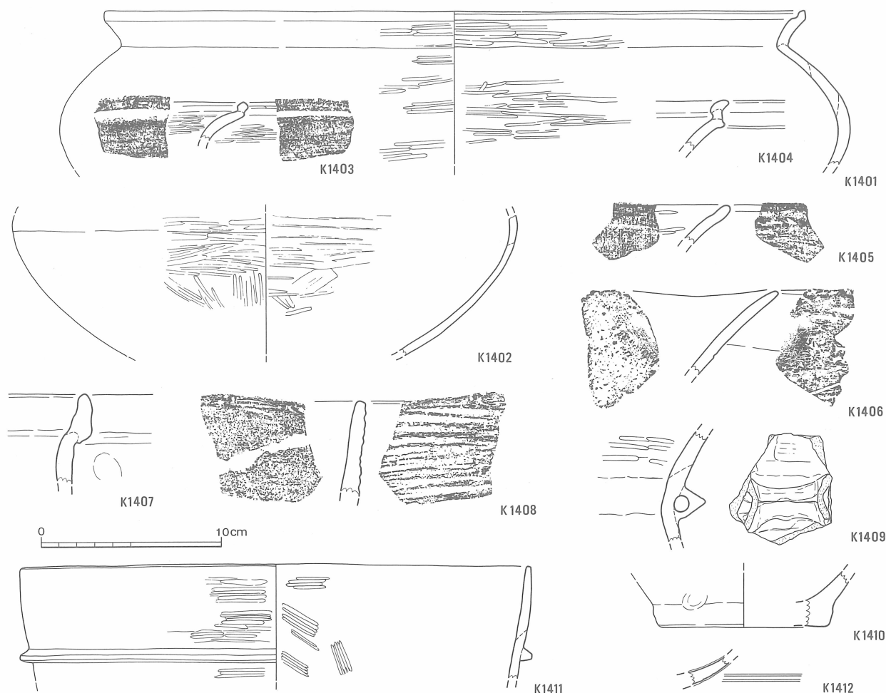
Fig.28 土壇出土土器実測図4 <SK14> (1/3)
