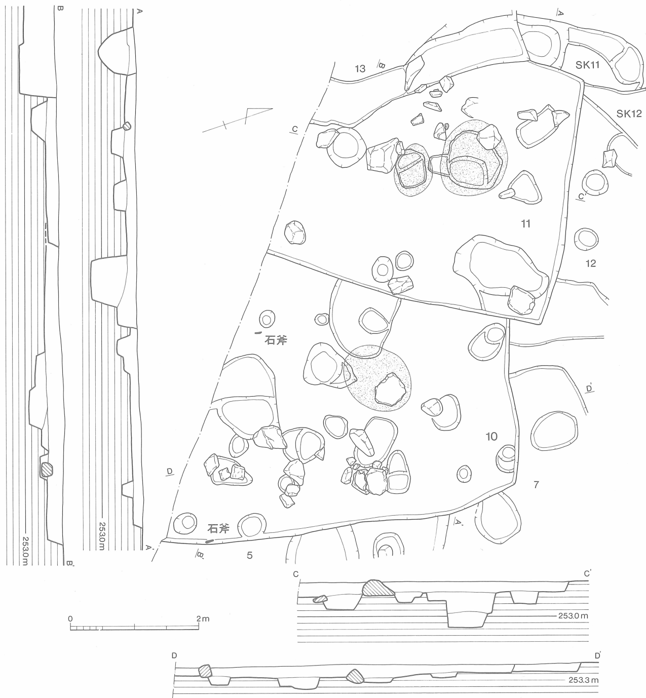
Fig.10 10・11号住居跡実測図 (1/60)
