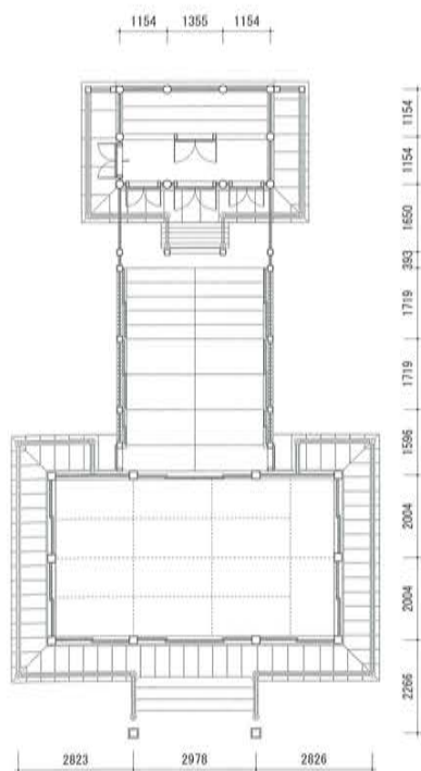
↑ 素盞鳴神社拝殿及び神殿現状平面図
