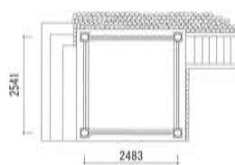
↑覺法寺鐘樓現狀平面図
