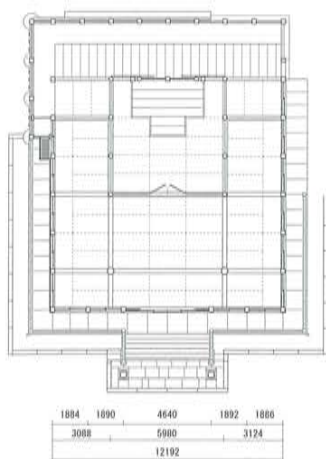
←宗真寺本堂現狀平面図
