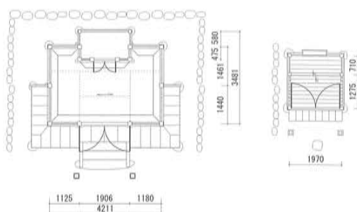
↑ 下町観音堂及び弘法堂現状平面図
