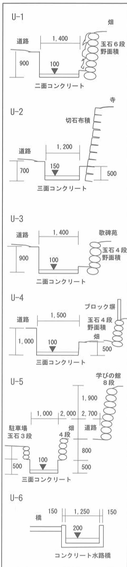
図3-8 水路断面図 (単位: mm)
