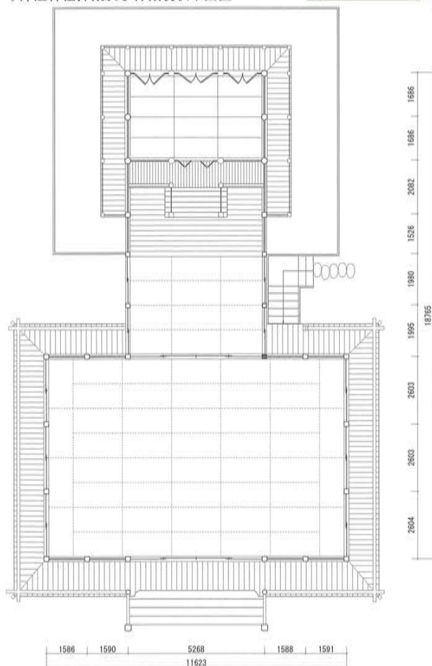
↓ 津江神社拝殿及び神殿現状平面図
