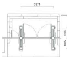
↑覺法寺山門現狀平面図
