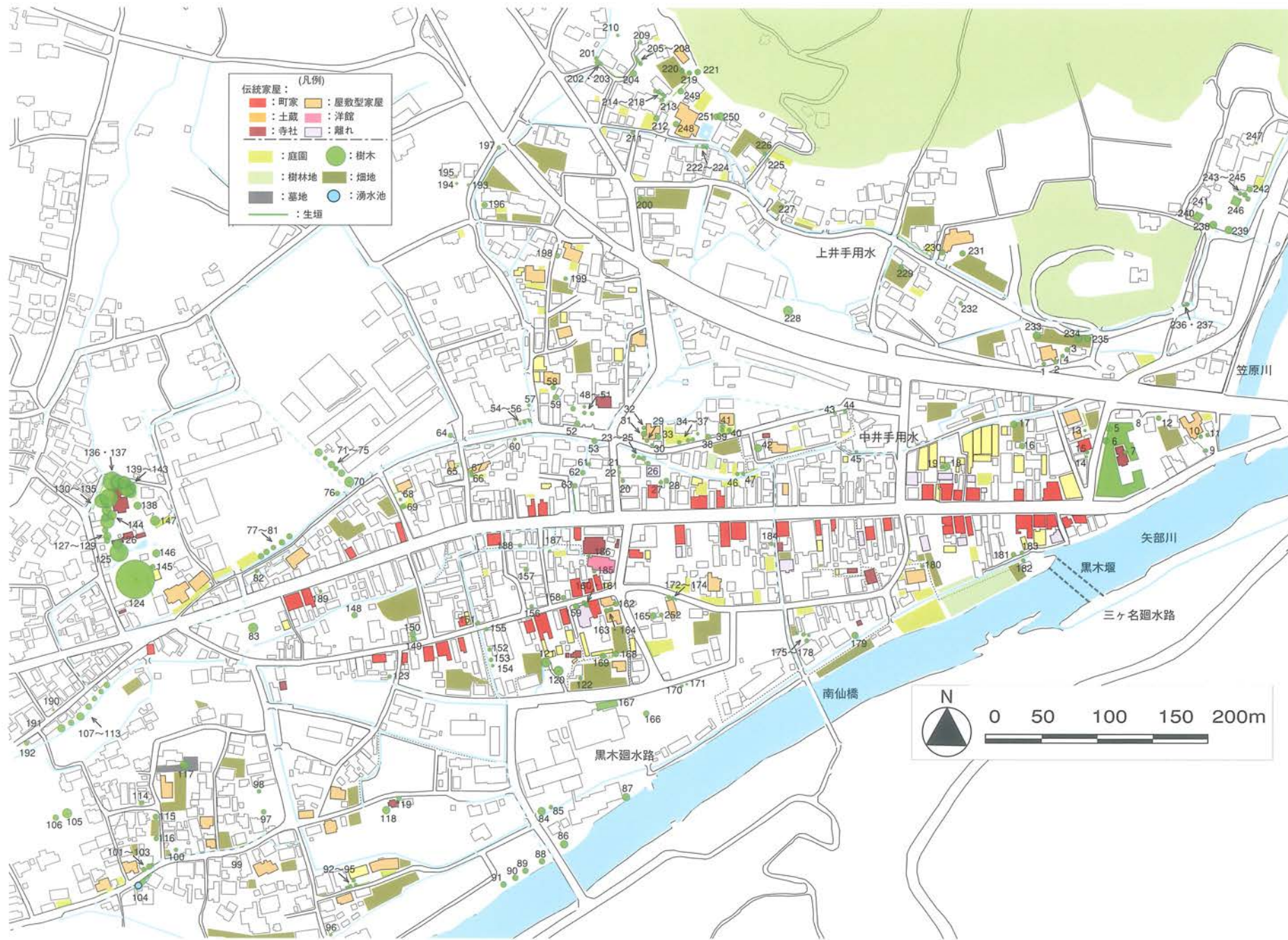
↑ 樹木分布図
