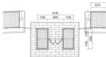
↑ 津江神社楼門現状平面図
