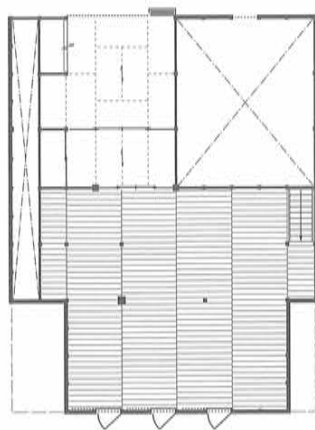
↑ 明治 13 年大火後の町家復原二階平面図
