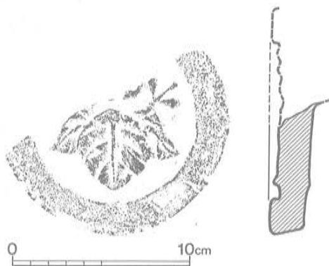
第26図 Ⅱ区異櫓址出土瓦実測図(1/3)
