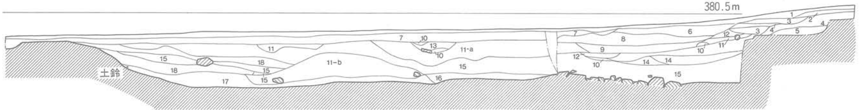
第4図 I区第1トレンチ(上)、Ⅲ区南北トレンチ(下)土層図 (1/60)
