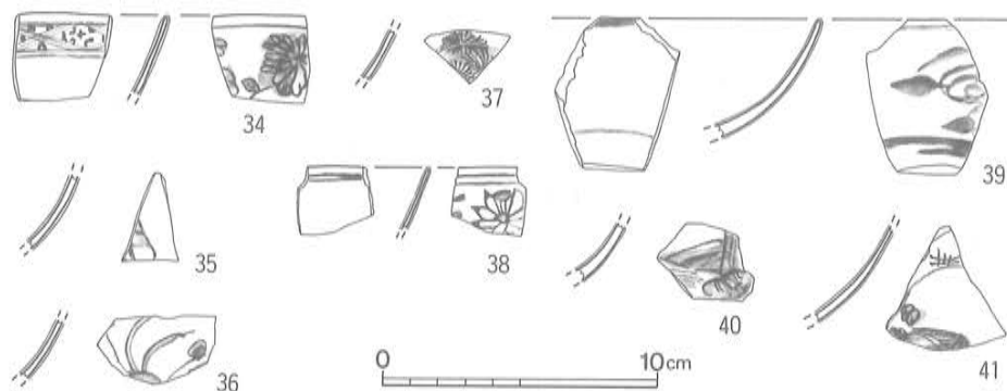
第28図 III区南北トレンチ出土土器実測図その2 (1/3)
