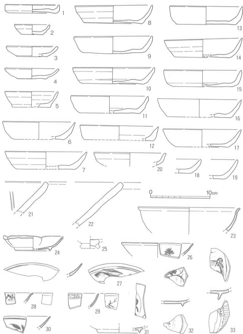
第27図 III区南北トレンチ出土土器実測図その1 (1/3)
