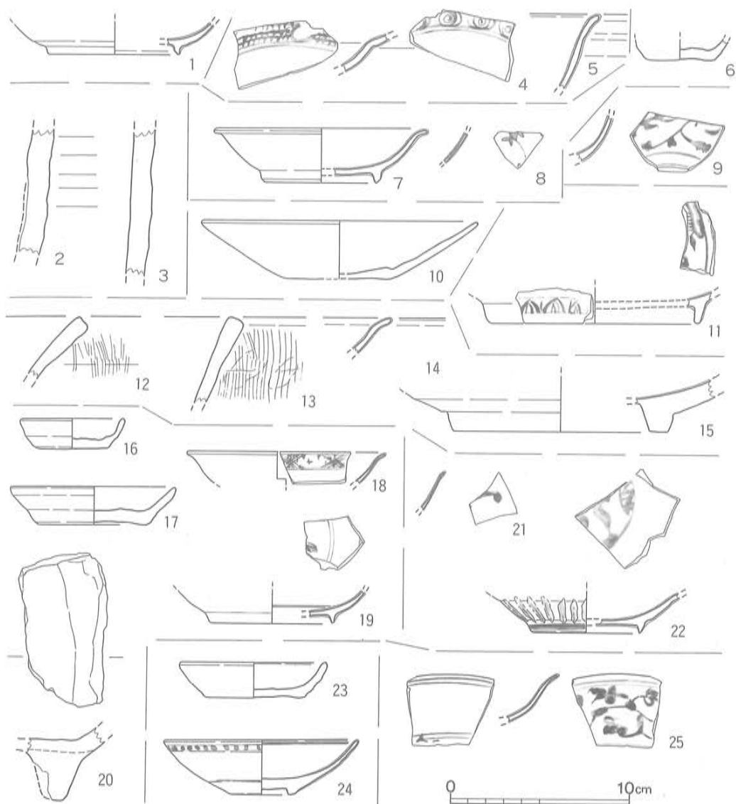
第30図 各トレンチ出土土器実測図 (1/3)
