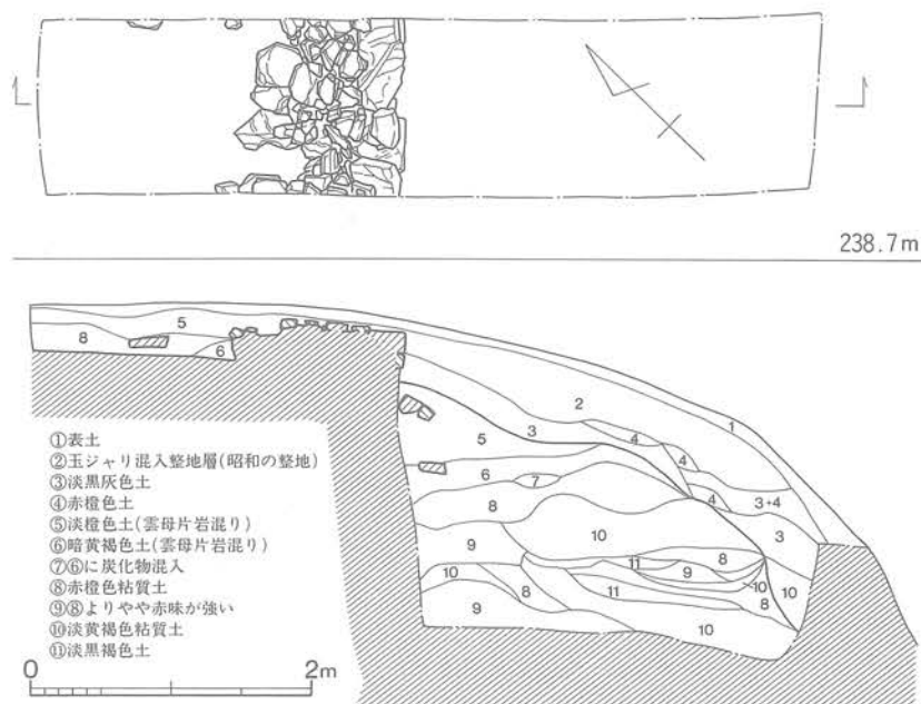
第19図 第15トレンチ遺構実測図 (1/60)
