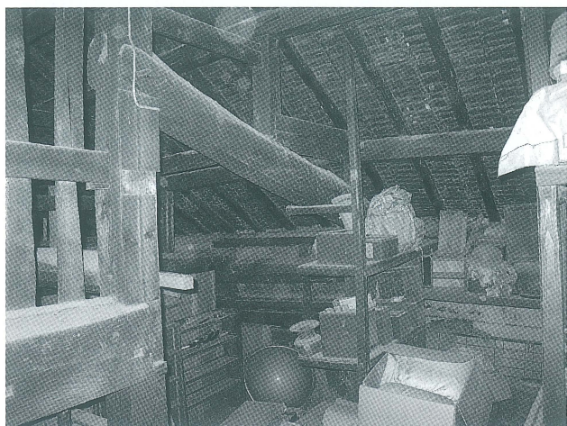
写真 15 架け替えられたと考えられる十通りの登り梁
