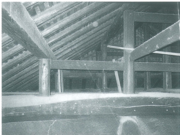
写真 13 十四通り小屋組
