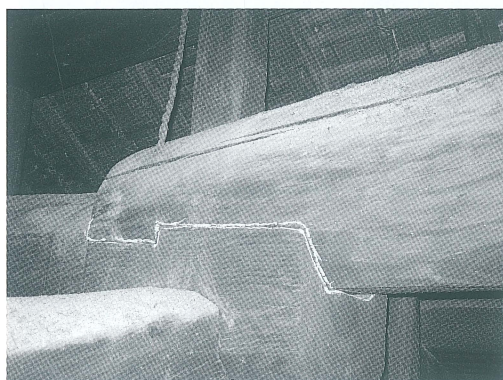
写真 19 地棟の継手
