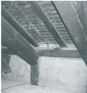
写真 20 登り梁と2階桁
