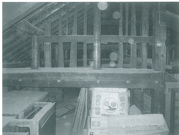
写真 14 十通り中柱より東の小屋組
