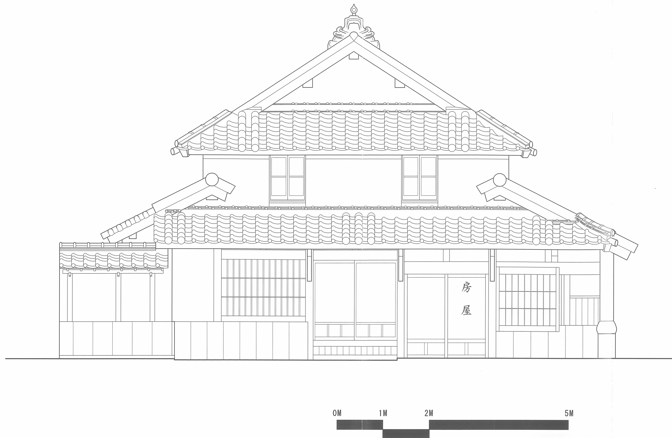
图面4 現況南側立面图 1/50
