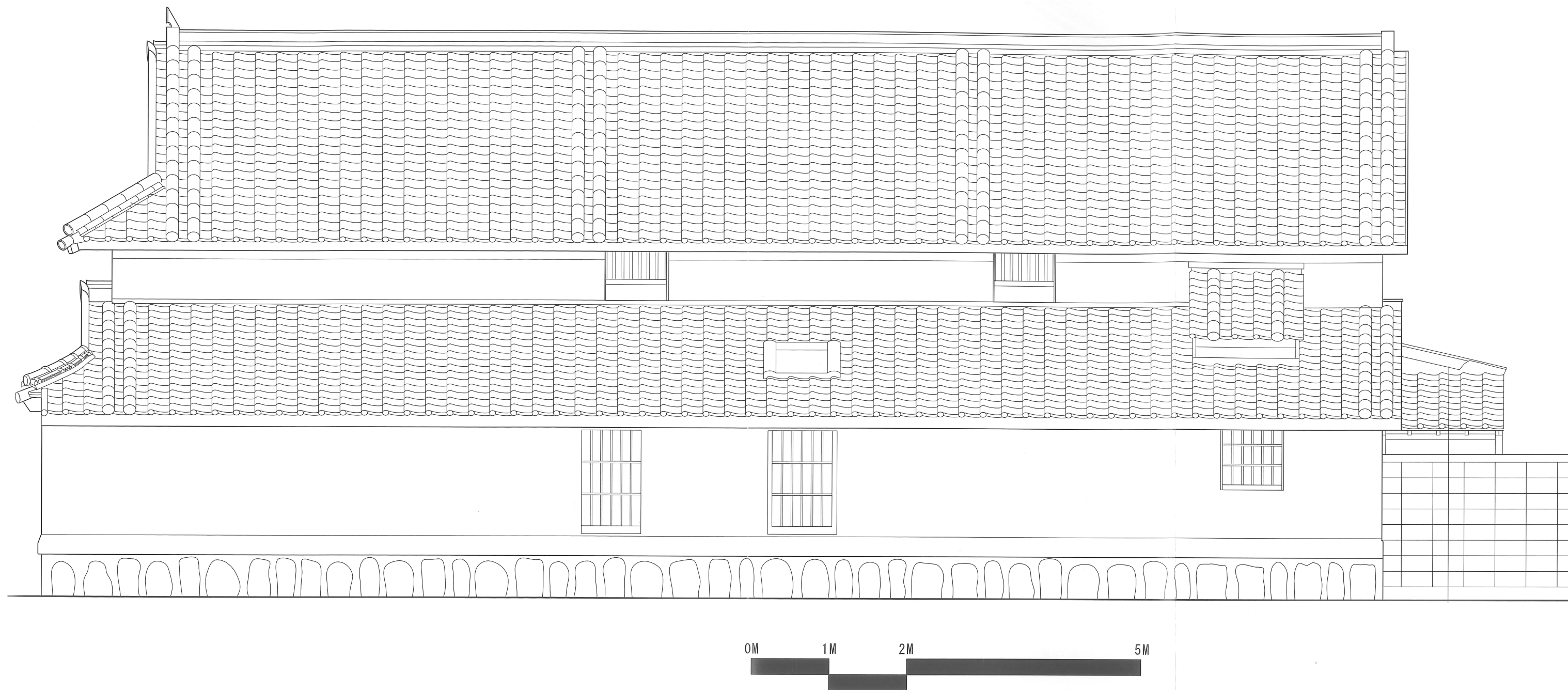
図面5 現況東側立面図 1/50
