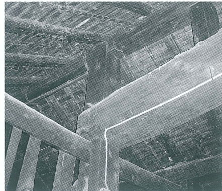
写真 21 直接棟木を載せている通し柱
