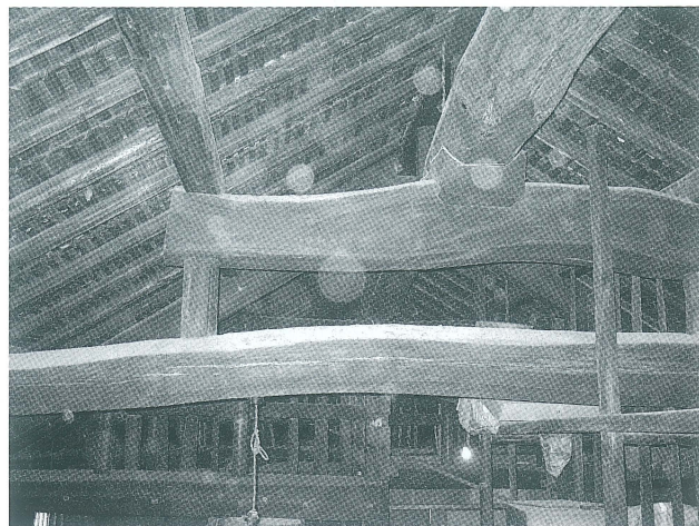
写真 16 七通り小屋組
