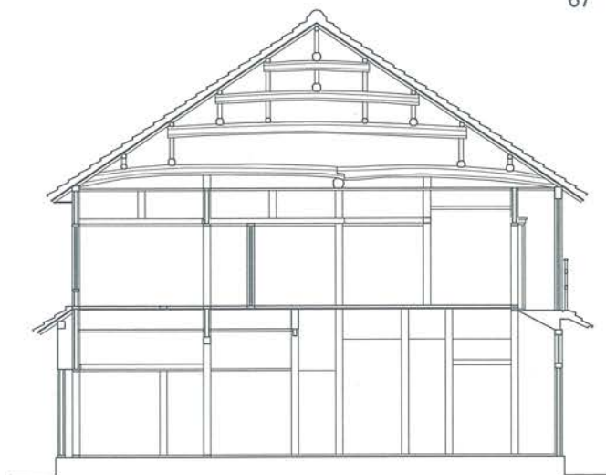
↑宮崎勝家断面図 小島妙子家復原平面図 ↓二階 ↓一階
