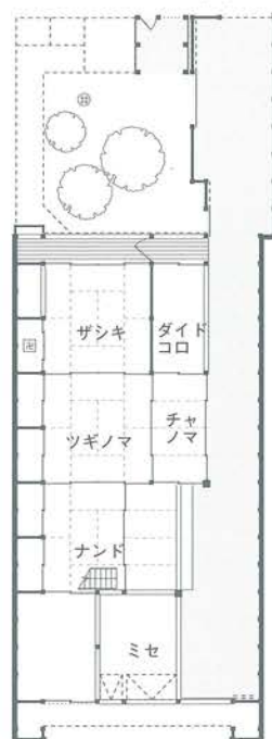
↓ 諸富弘家 復原平面図(3)
