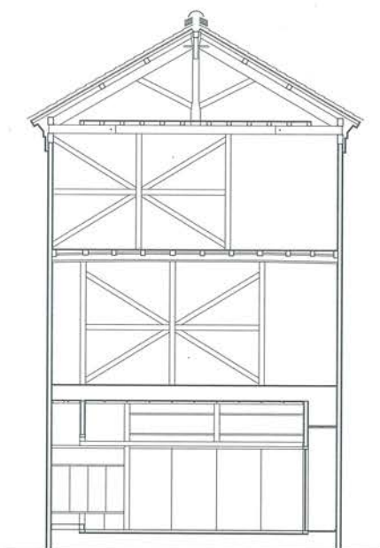
↑ 田中茂行家断面図
