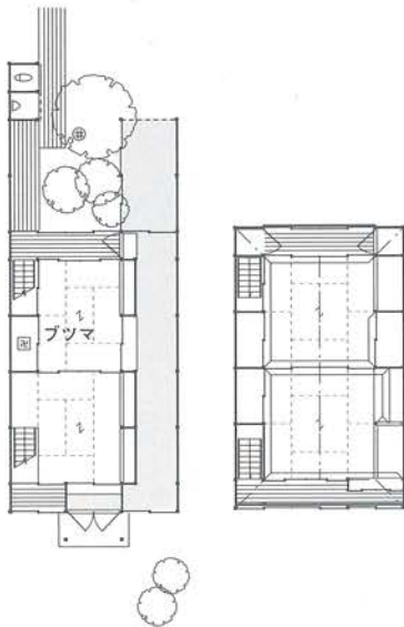
古池哲夫家復原平面図 ↑一階 ↑二階
