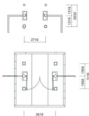
↑ 正福寺山門平面図
