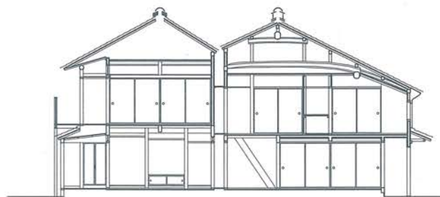
↑平井博家断面図
