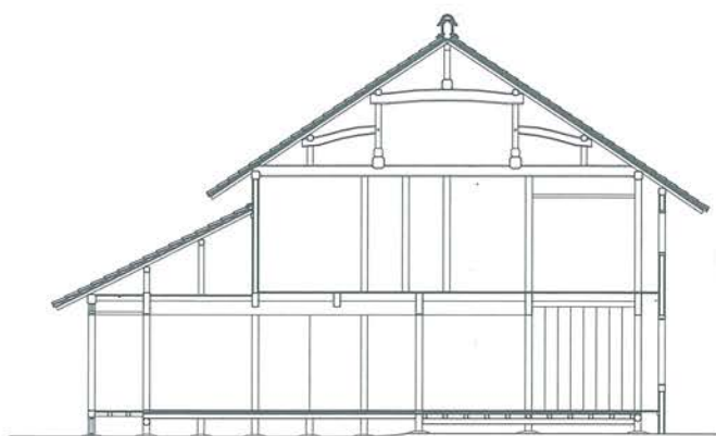
↑木下喜八郎家南棟断面図
