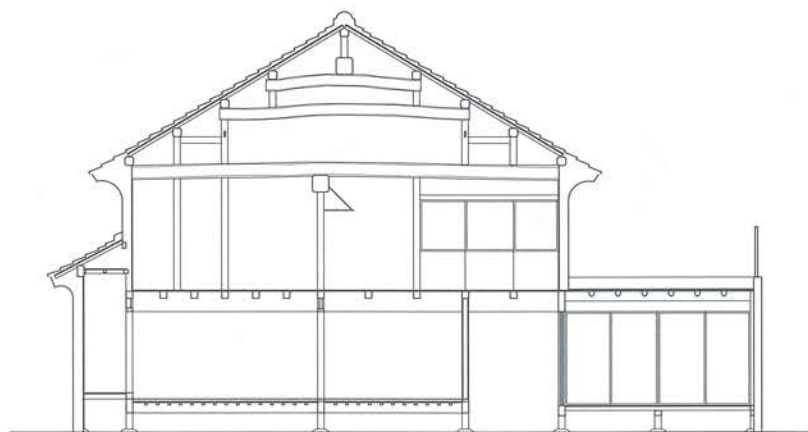
↑高橋博之家断面図
