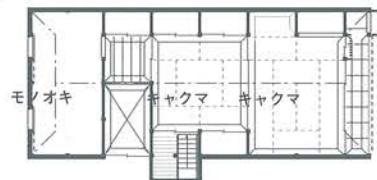
高橋貞記家復原平面図 ↑二階 ↓一階
