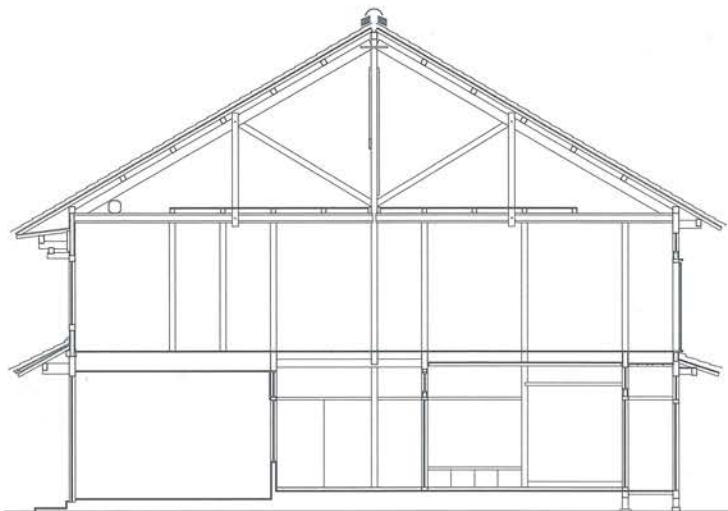
↑ 丸林恭一・志郎家断面図 丸林恭一・志郎家復原平面図 ↓二階 ↓一階
