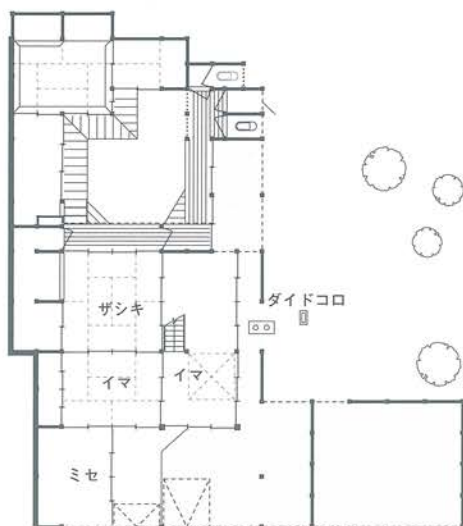
渡辺正博家復原平面図 ↑ 一階
