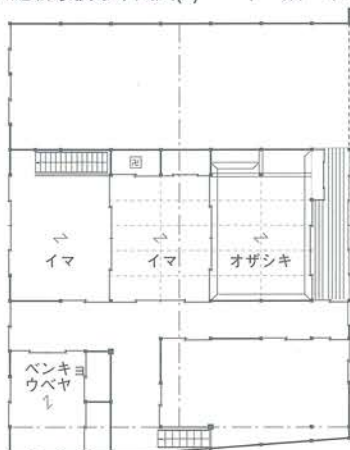
松延新家復原平面図(3) ↑一階 ↓二階
