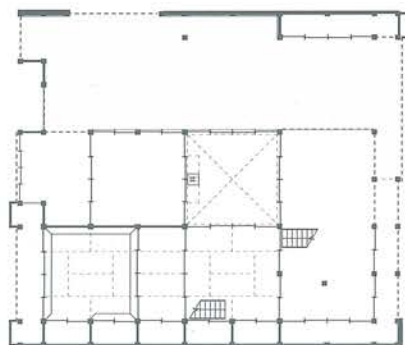
木下茂家復原平面図 ↑二階 ↓一階
