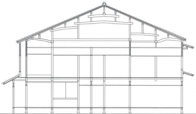
↑ 酒井広悦家断面図
