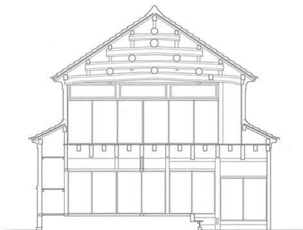
↑ 諸富弘家 断面図 ↓ 田中義博家断面図
