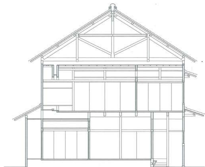
↑ 鶴篤介家断面図
