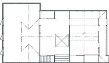
川山ハル子家復原平面図(3) ↑一階 ↓二階
