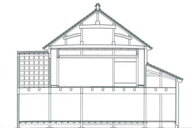
↑木下喜八郎家北棟断面図
