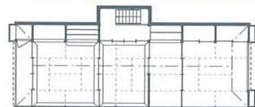
朝山邦彦家復原平面図 ↑二階 ↓一階 由留部進家復原平面図 ↑二階 ↓一階
