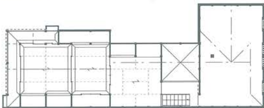
若菜静子家復原平面図 ↑一階 ↓二階
