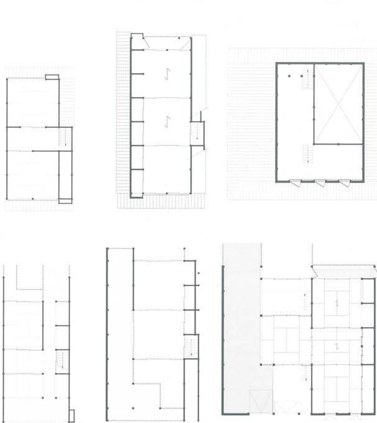
↓間口3間の真壁造町家 ↓間口3間の土蔵造町家 ↓間口6間の土蔵造町家
