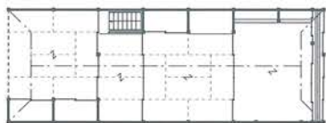
清田久恵家復原平面図(3) ↑一階 ↓二階
