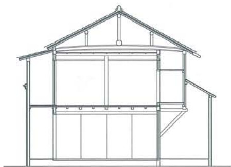
↑ 宗勝紀家断面図
