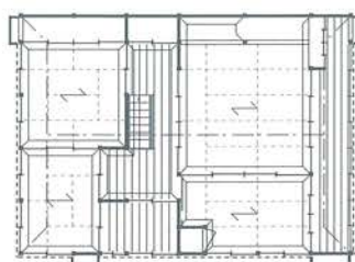
鶴篤介家復原平面図 ↑二階 ↓一階
