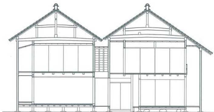
↑ 高橋練蔵家断面図
