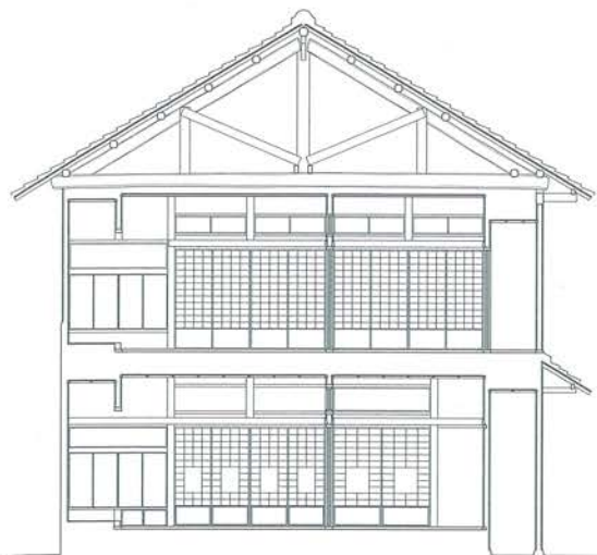
↑ 角和憲家断面図
