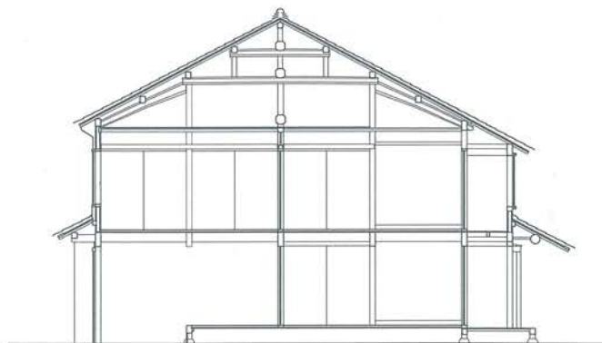
↑ 高橋正二家断面図
