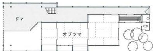
清田久恵家復原平面図(3) ↑一階 ↓二階
