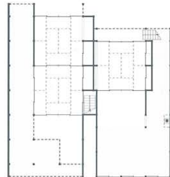
藤井孝雄家復原平面図 ↑二階 ↓一階
