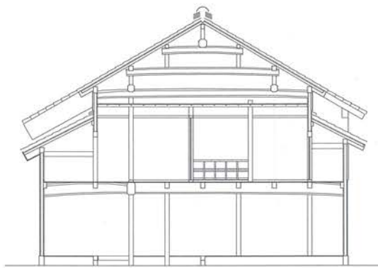
↑平井朋吉家断面図 ↓坂口哲治家断面図
