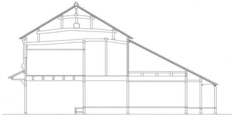
↑ 原田春恵家断面図
