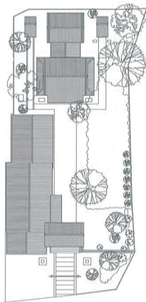
秋葉社 ↑配置図(5) ↓神殿・拝殿平面図(3)
