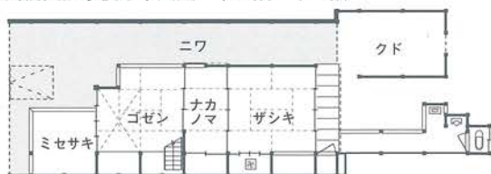
高橋貞記家復原平面図 ↑二階 ↓一階
