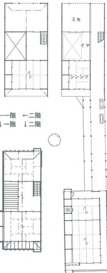
井上良雄家復原平面図 馬場英子家復原平面図
