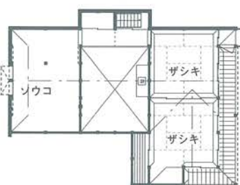
高橋久雄家復原平面図 ↑二階 ↓一階
