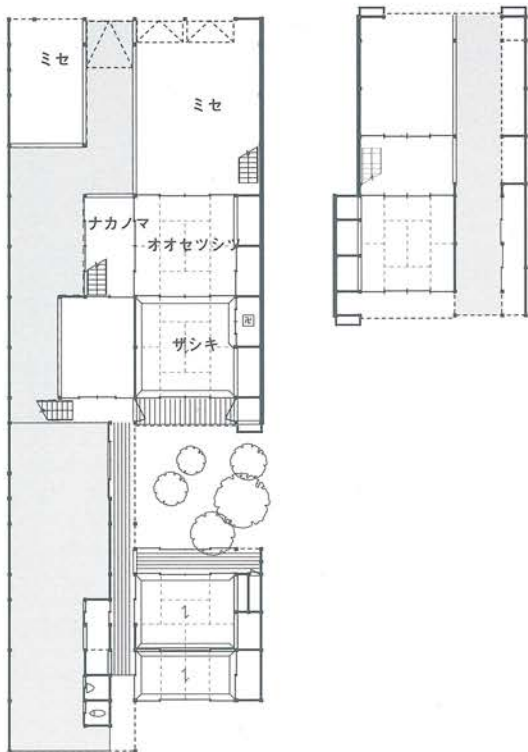
平井儀助家・平井博家復原平面図 ↑一階 ↓二階
