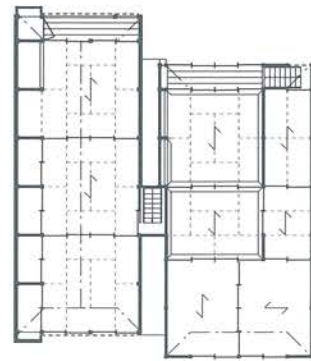
藤井孝雄家復原平面図 ↑二階 ↓一階
