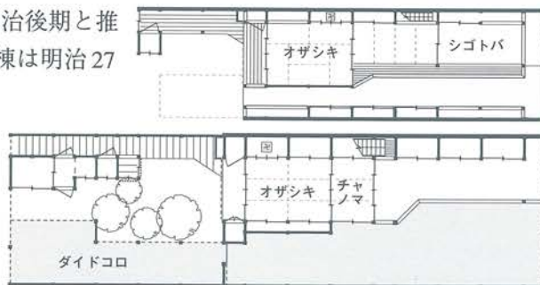
朝山邦彦家復原平面図 ↑二階 ↓一階 由留部進家復原平面図 ↑二階 ↓一階
