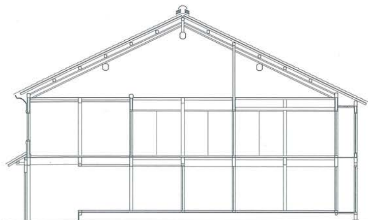
↑ 丸林周司家中棟断面図
