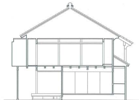
↑ 丸林周司家北棟断面図
