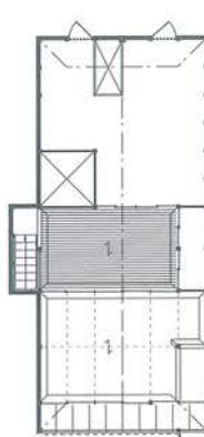
↑宮崎勝家断面図 小島妙子家復原平面図 ↓二階 ↓一階
