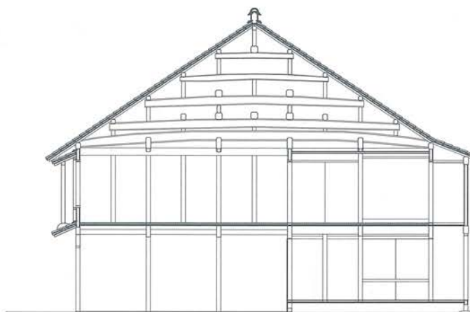
↑ 高橋靖雄・今里勲家断面図
