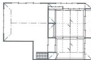
高木益一家復原平面図 ↑二階 ↓一階
