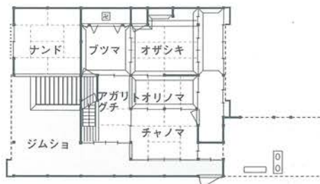
鶴篤介家復原平面図 ↑二階 ↓一階
