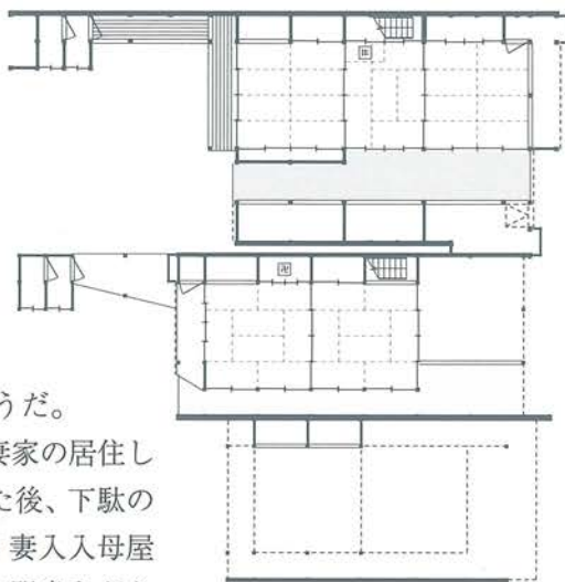
丸林周司家復原平面図 ↓一階 ↓二階
