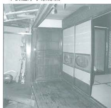
↑伊藤文二家小屋組 ↓安達厚子家縁側
