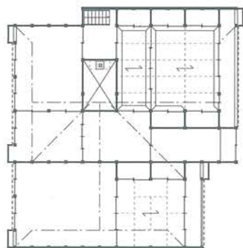
高橋靖雄・今里勲家復原平面図 ↑二階 ↓一階
