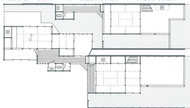
高橋章家 ↑ 茶室 ↑ 二階復原平面図 ↓ 一階復原平面図
