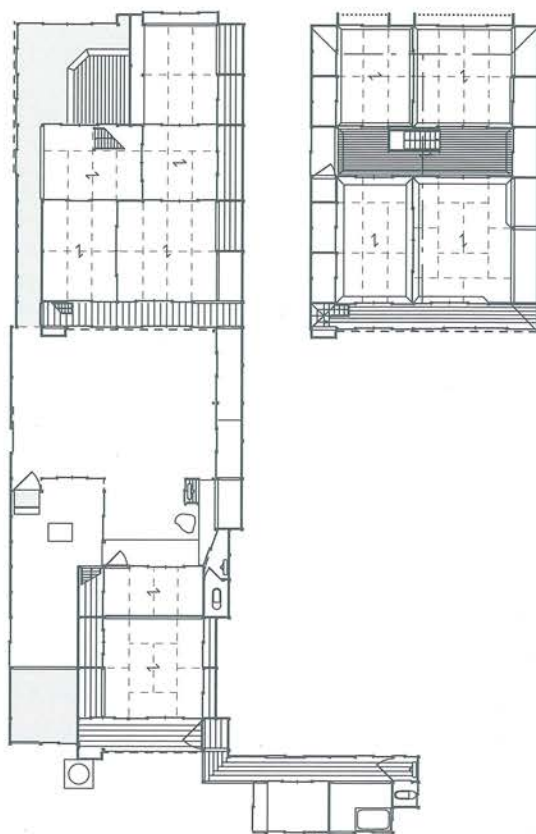
角和憲家復原平面図 ↑一階 ↑二階
