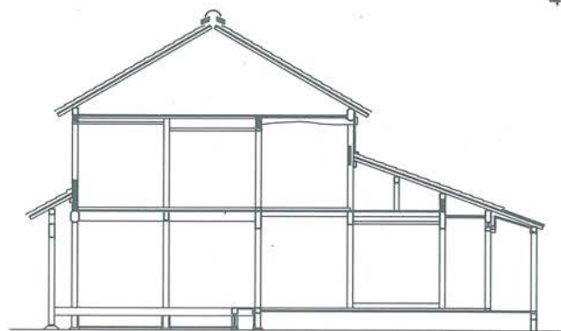
↑ 江崎忠助家断面図
