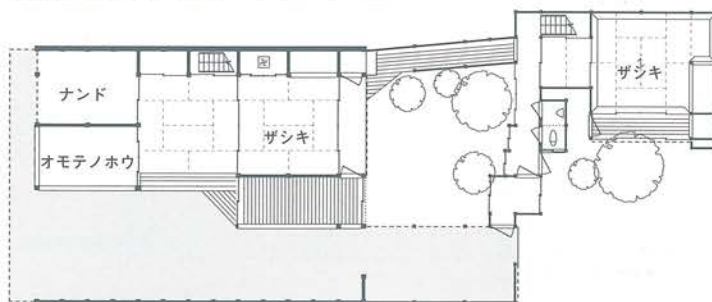
高橋久雄家復原平面図 ↑二階 ↓一階
