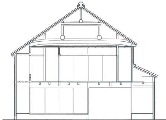
↑馬場強家断面図
