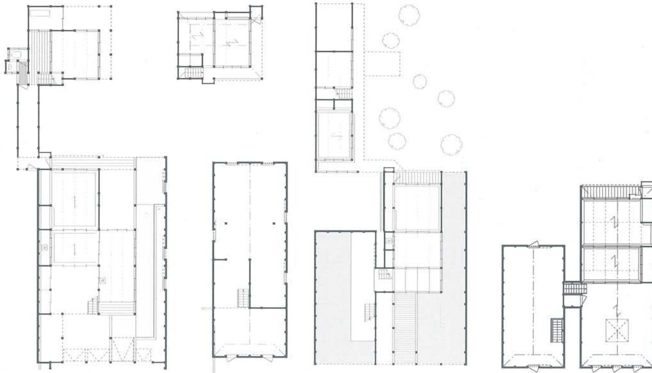
今里亨家復原平面図 ↑一階 ↑二階
