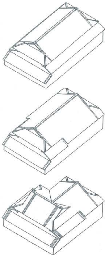
↓両袖下屋形式の3類型
