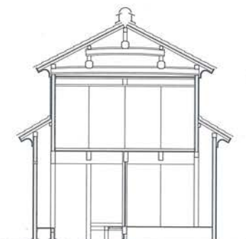
↑ 朝山邦彦家断面図
