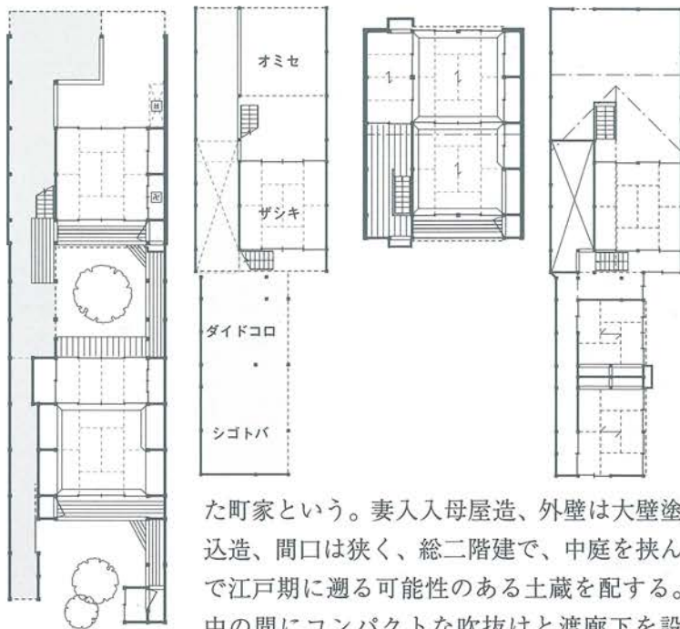
高橋正二家・宗勝紀家復元平面図 ↓一階 ↓二階
