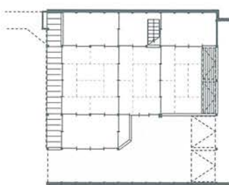
木下喜八郎家北棟復原平面図 木下喜八郎家南棟復原平面図
