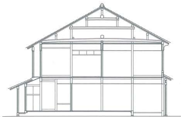
↑坂口逸次家断面図
