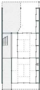
大石喜八郎家復原平面図 ↓一階 ↓二階
