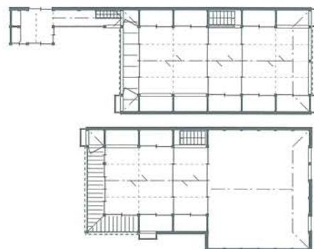
高橋章家 ↑ 茶室 ↑ 二階復原平面図 ↓ 一階復原平面図
