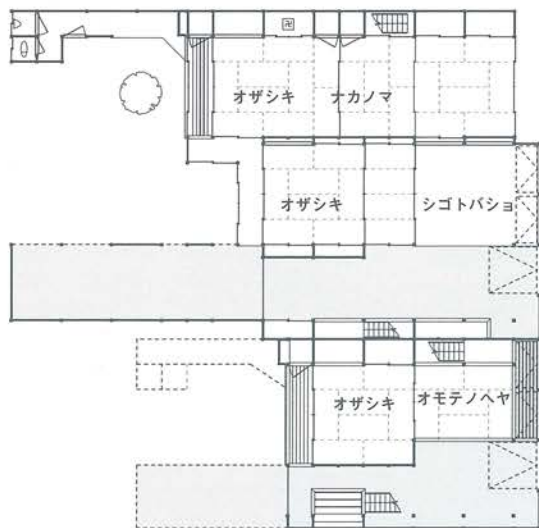
酒井広悦家・古賀繁樹家復原平面図 ↑一階
