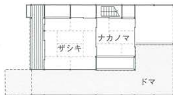
松延カツエ家復原平面図(3) ↑一階 ↓二階
