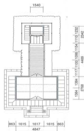
秋葉社 ↑配置図(5) ↓神殿・拝殿平面図(3)
