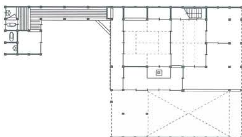
木下喜八郎家北棟復原平面図 木下喜八郎家南棟復原平面図
