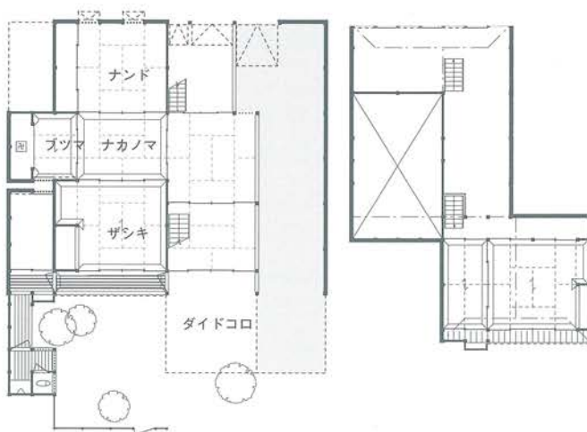
田中義博家復原平面図 ↑一階 ↑二階
