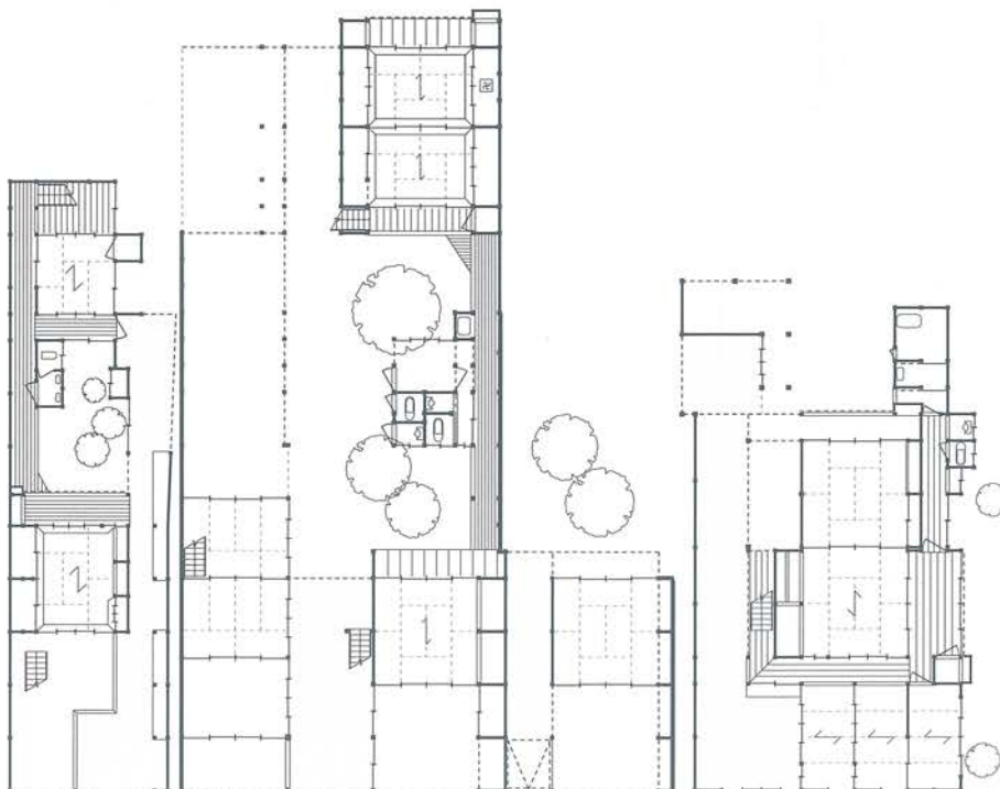
一階復原平面図 ↓村上康代家
