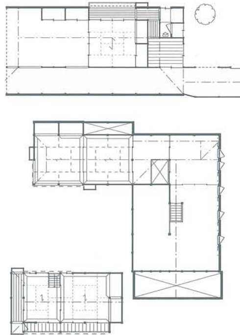
↓ 井上長蔵家倉庫復原平面図
