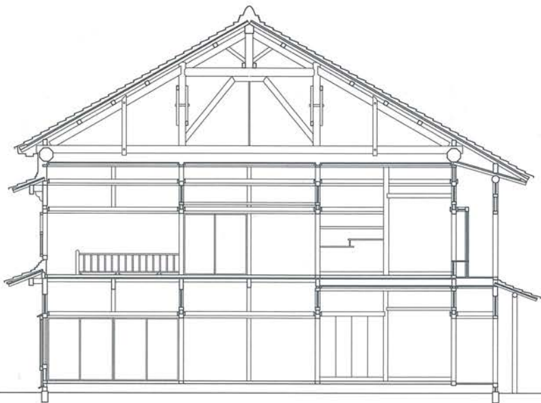
↑松延新家断面図(1.5)
