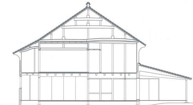
↑ 角和憲家東棟断面図
