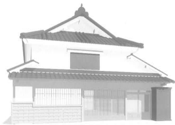
腰壁 格子付き腰高窓 掃出し ガラス戸 戸袋
