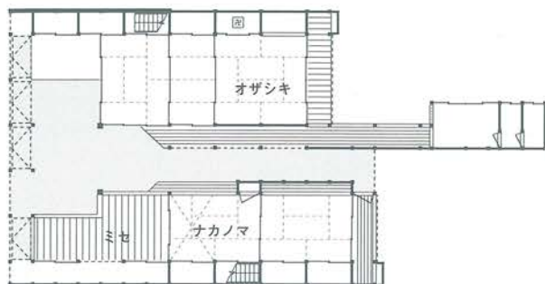
高橋練蔵家復原平面図 ↑二階 ↓一階
