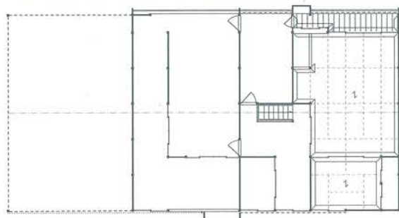
宮崎勝家復原平面図 ↑二階 ↓一階
