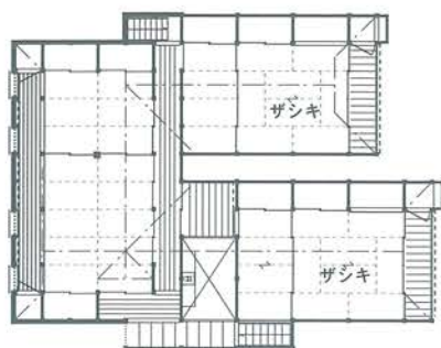
高橋練蔵家復原平面図 ↑二階 ↓一階
