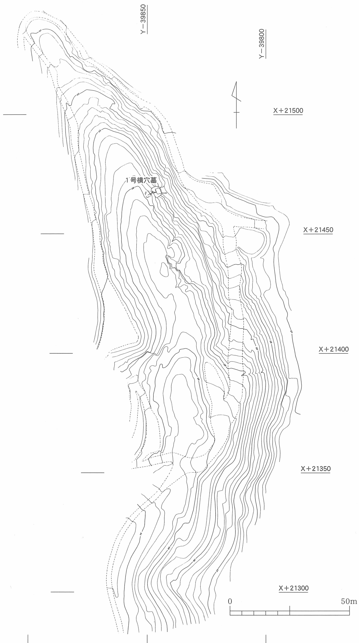
第3図 野広尾横穴墓群調査区地形測量図 (1/1,000)
