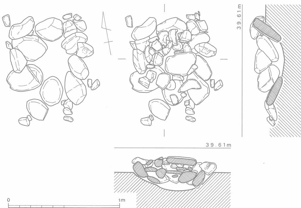
Fig. 5 石組炉実測図 (1/20)
