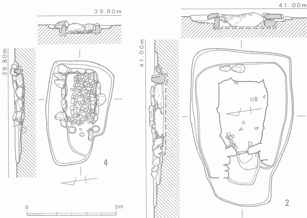
Fig. 8 2・4号墳石室実測図 (1/60)
