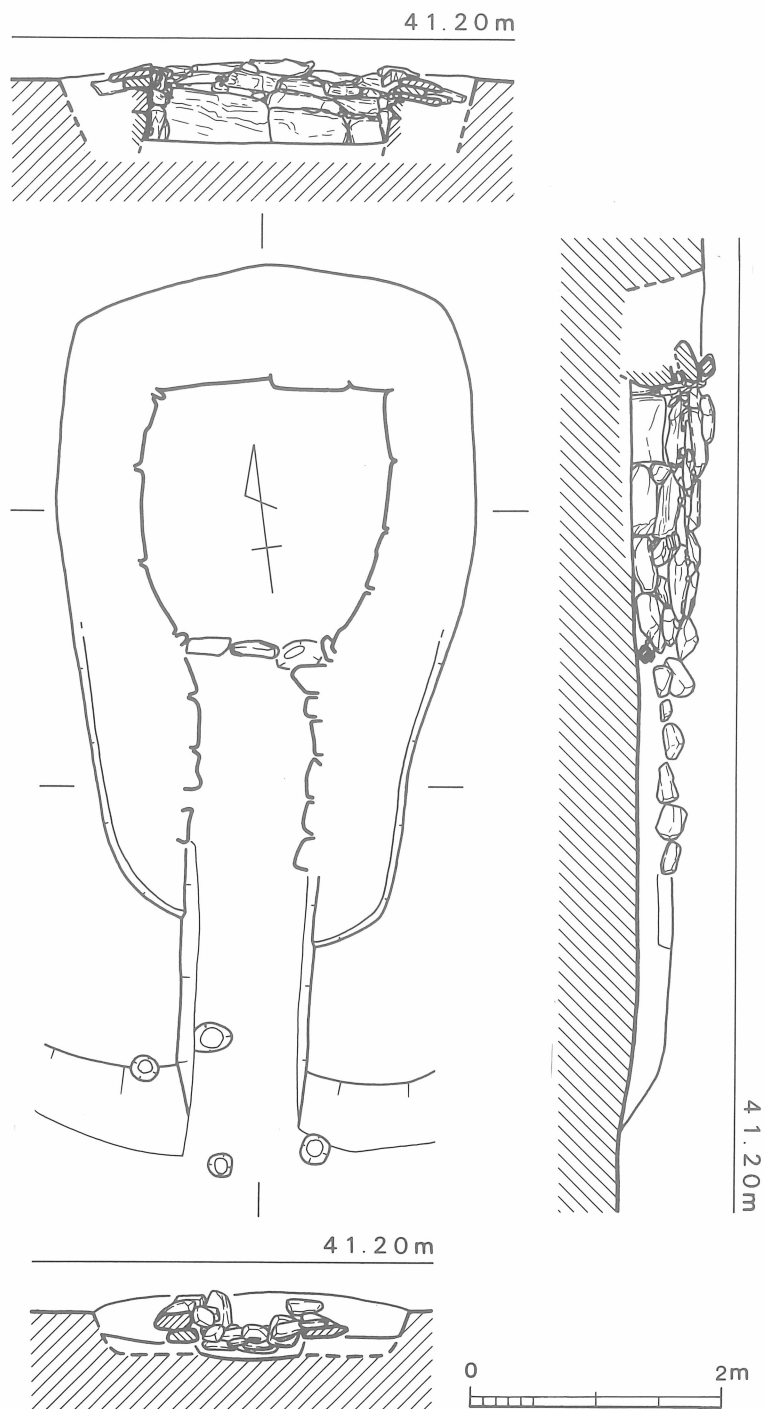
Fig. 9 1号墳石室実測図 (1/60)
