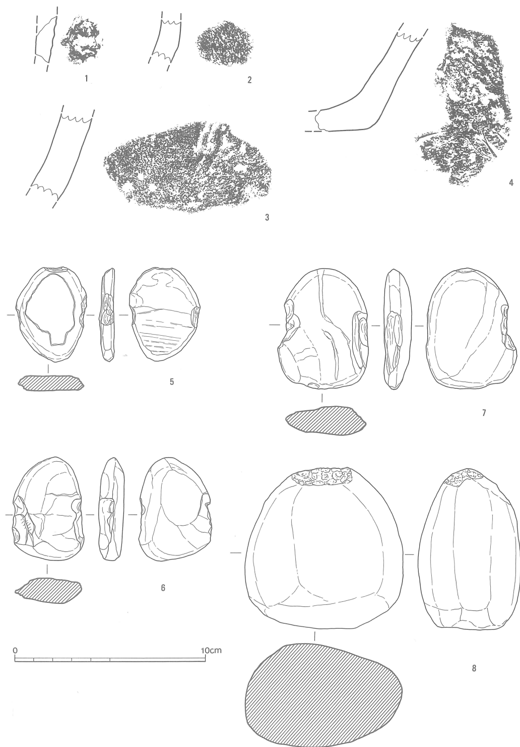
Fig.11 北山小学校遺跡出土遺物実測図1 (1/2)
