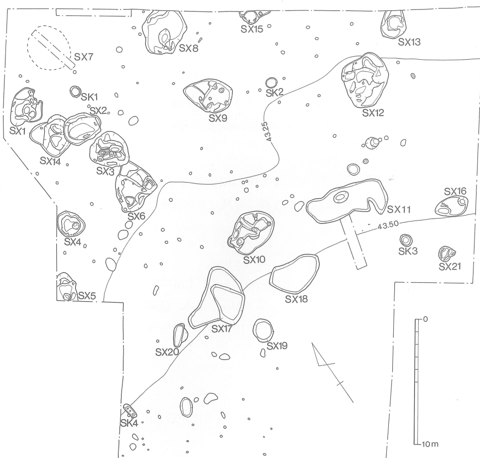
Fig. 5 北山小学校遺跡遺構配置図 (1/300)
