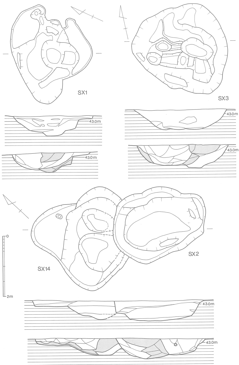
Fig. 7 SX 1 ~ 3 · 14実測図 (1/60)
