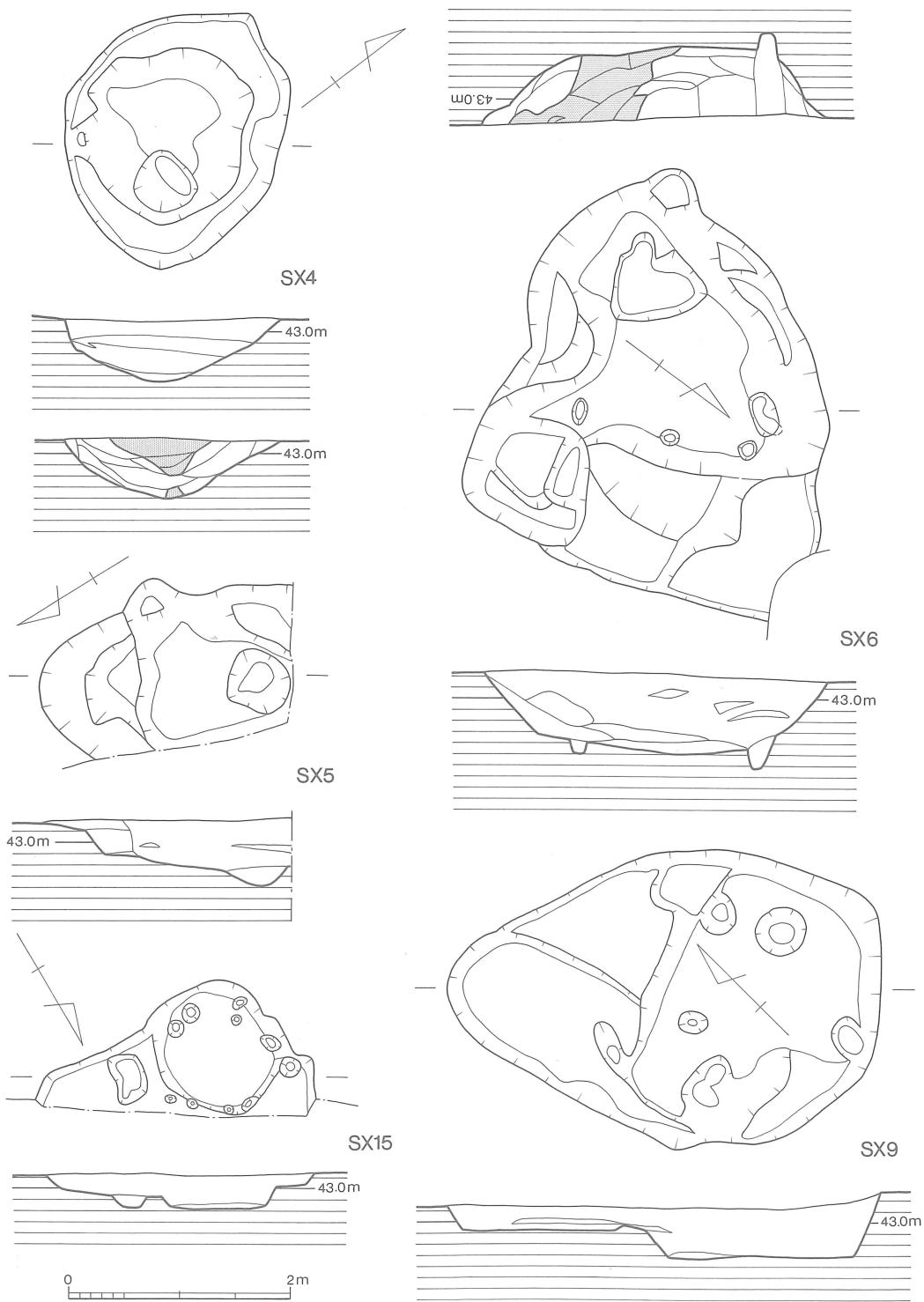
Fig. 8 SX 4 ~ 6 · 9 · 15実測図 (1/60)
