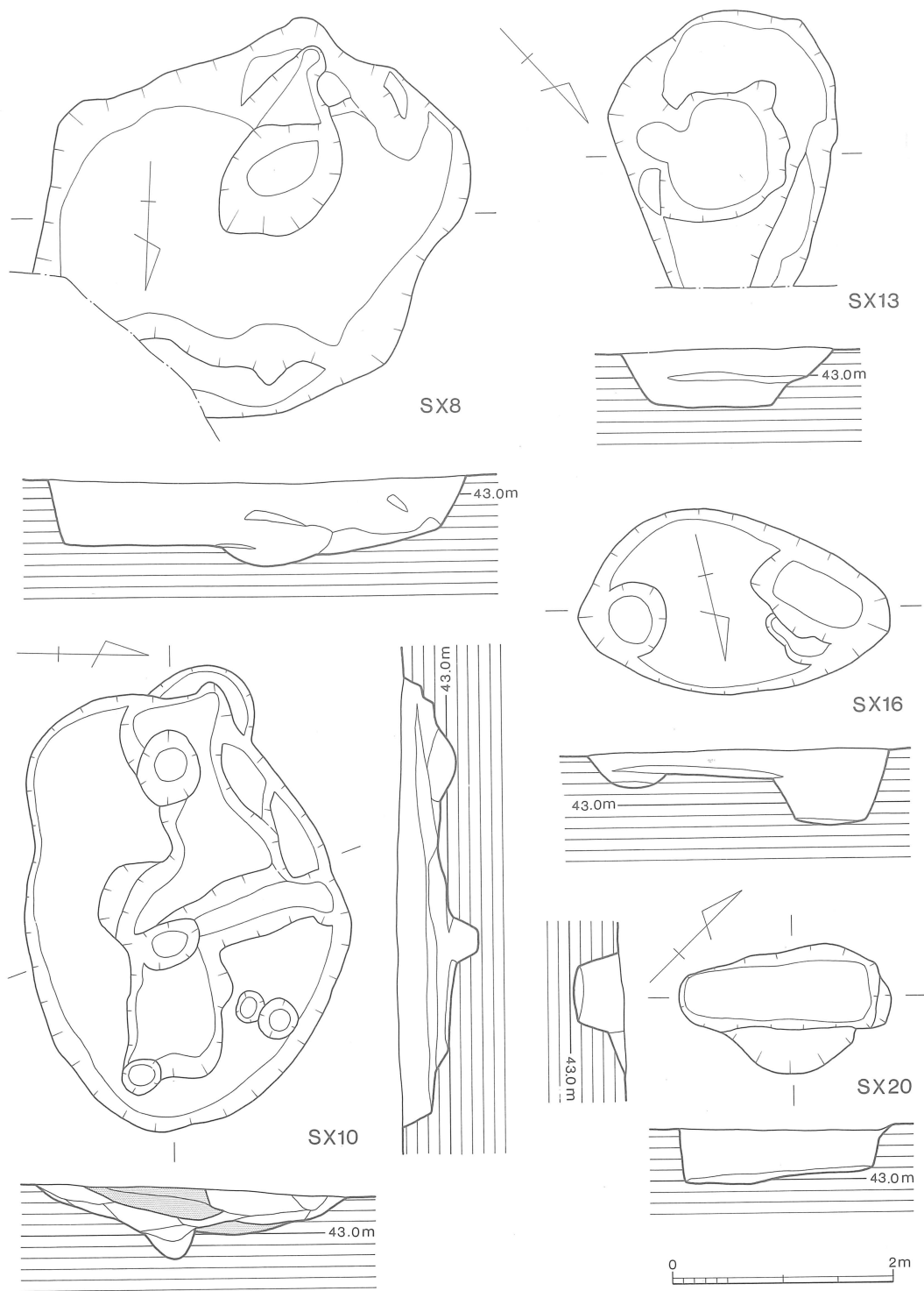
Fig. 9 SX 8・10・13・16・20実測図 (1/60)
