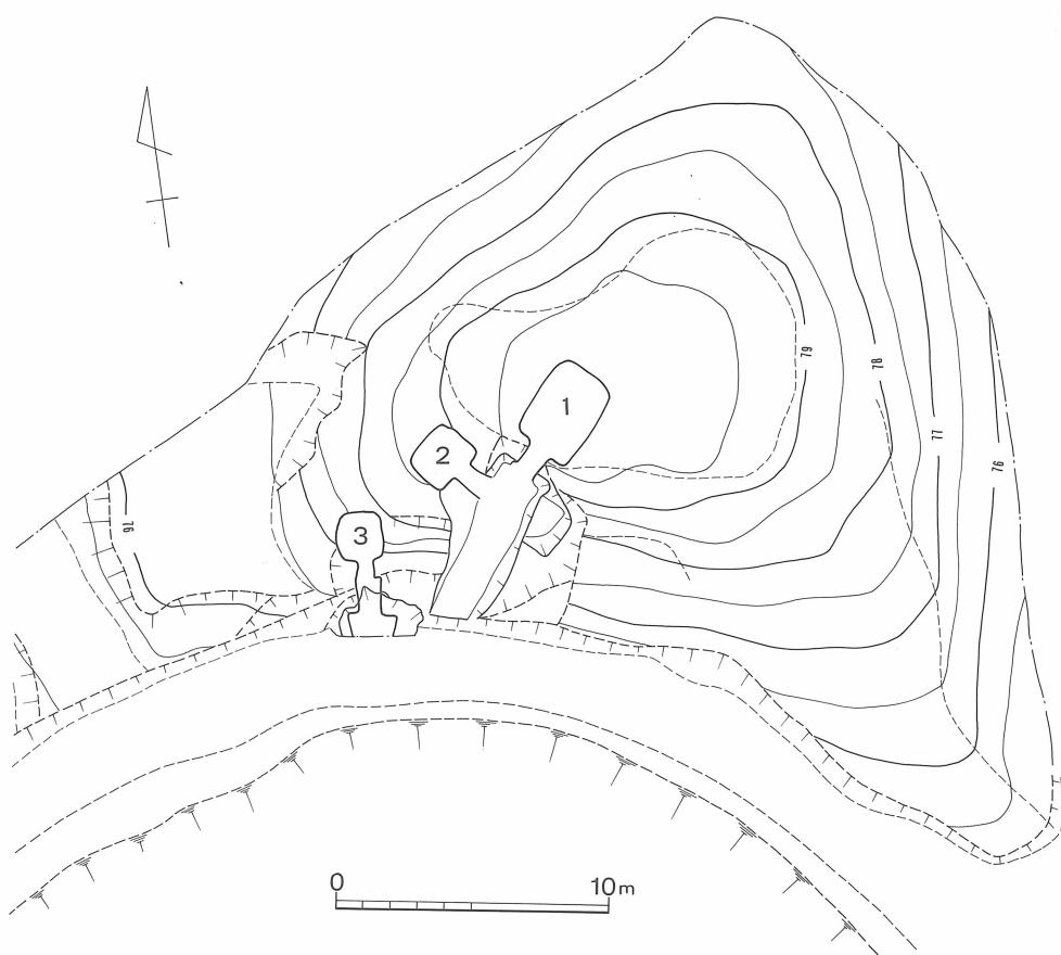
第3図 小倉谷横穴群 配置図（第4次調査、1/300）
