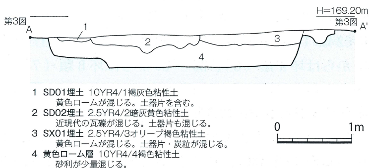
第13図 上小野遺跡SD01・SD02・SX01 土層図(S=1/50)
