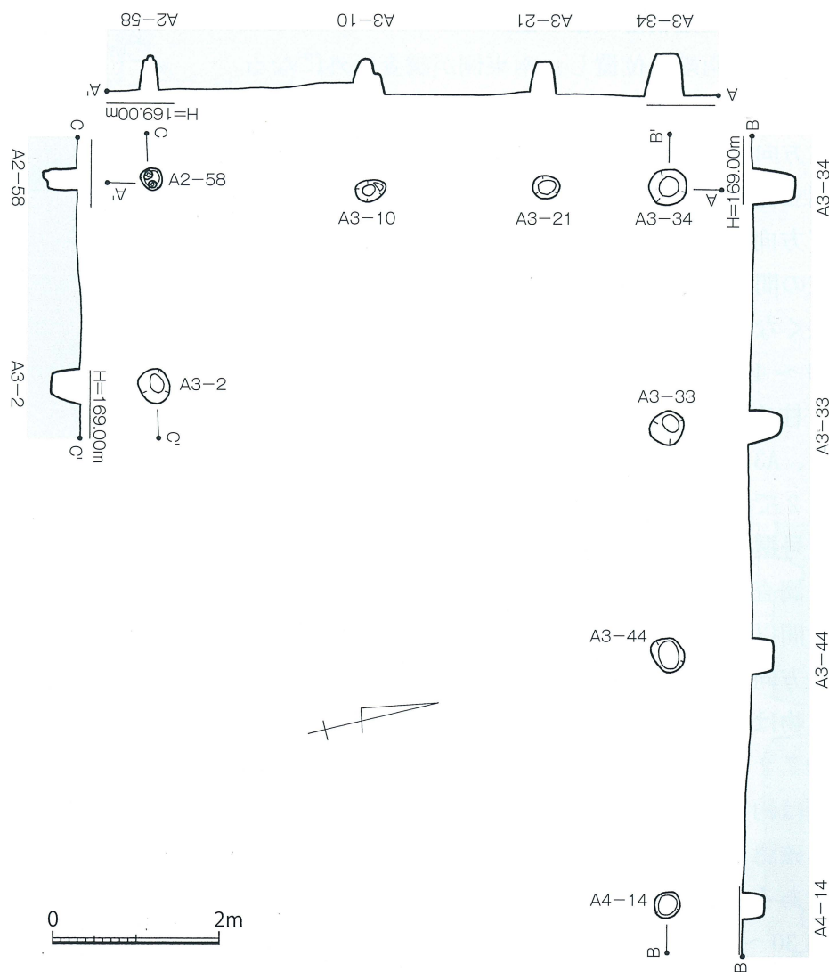
第5図 上小野遺跡1号掘立柱建物跡実測図 (S=1/80)
