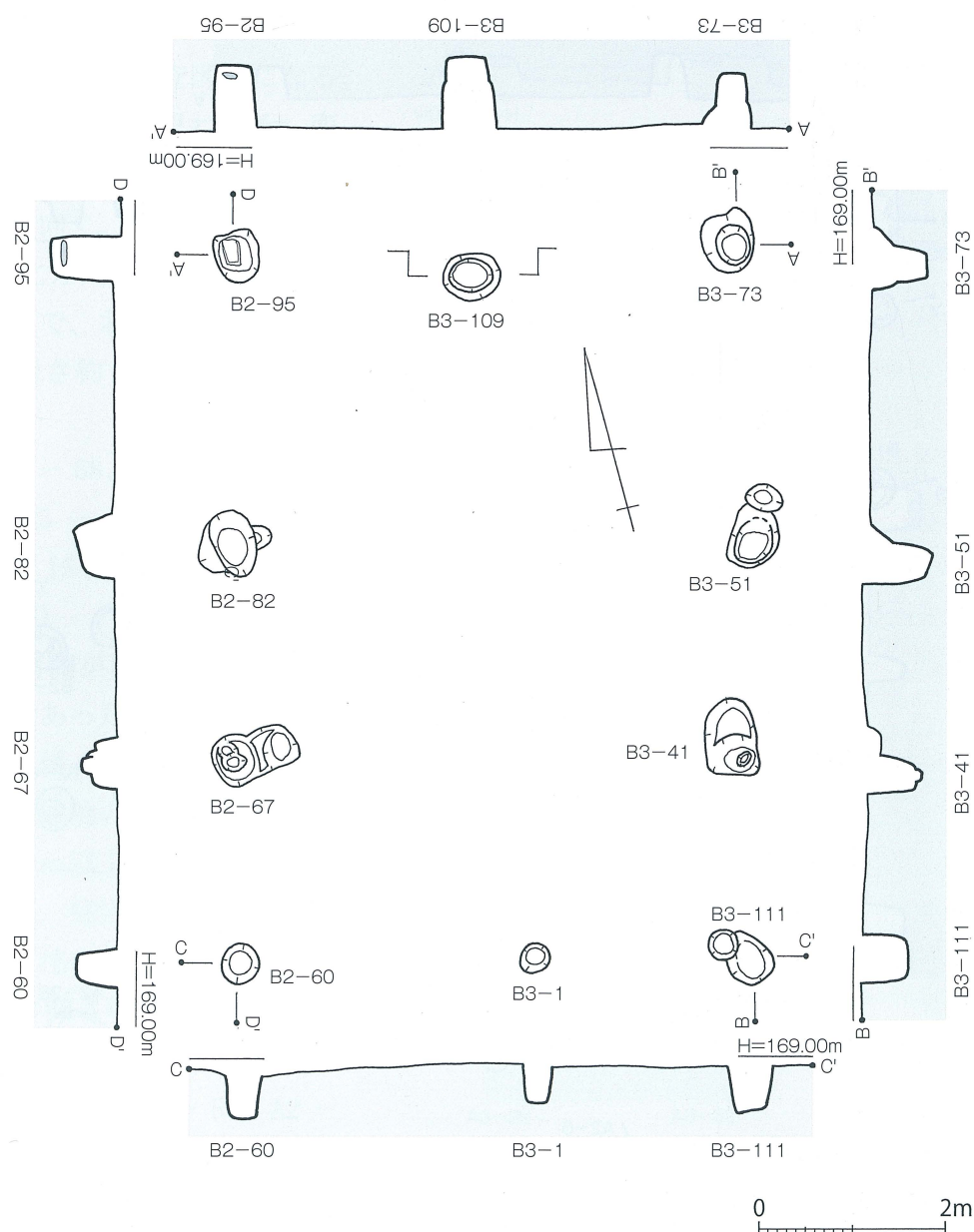
第 8 図 上小野遺跡 4 号掘立柱建物跡実測図 (S=1/80)
