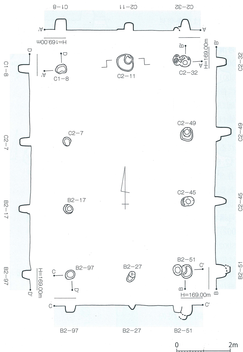
第10図 上小野遺跡6号掘立柱建物跡実測図（S=1/80）
