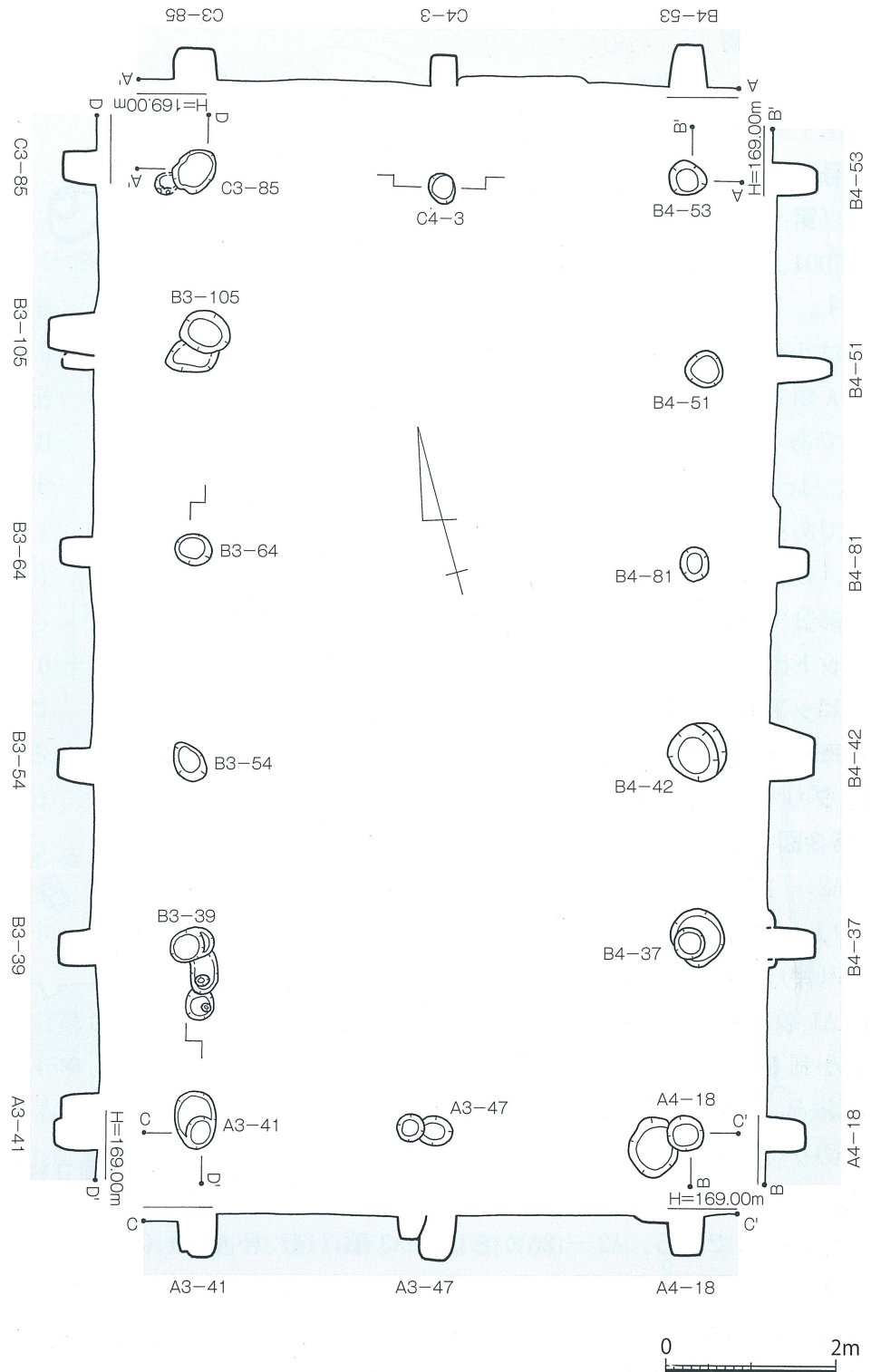
第9図 上小野遺跡5号掘立柱建物跡実測図 (S=1/80)
