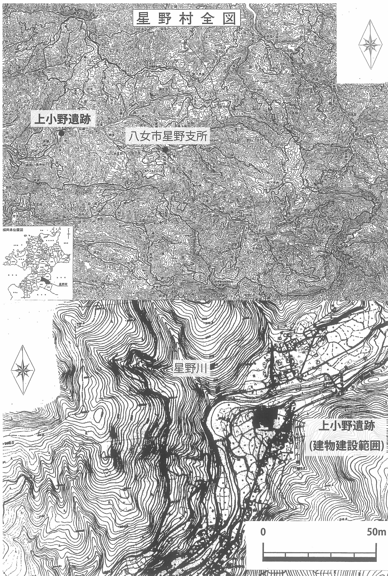
第2図 上小野遺跡周辺図 (S=1/25,000、S=1/1,000)
