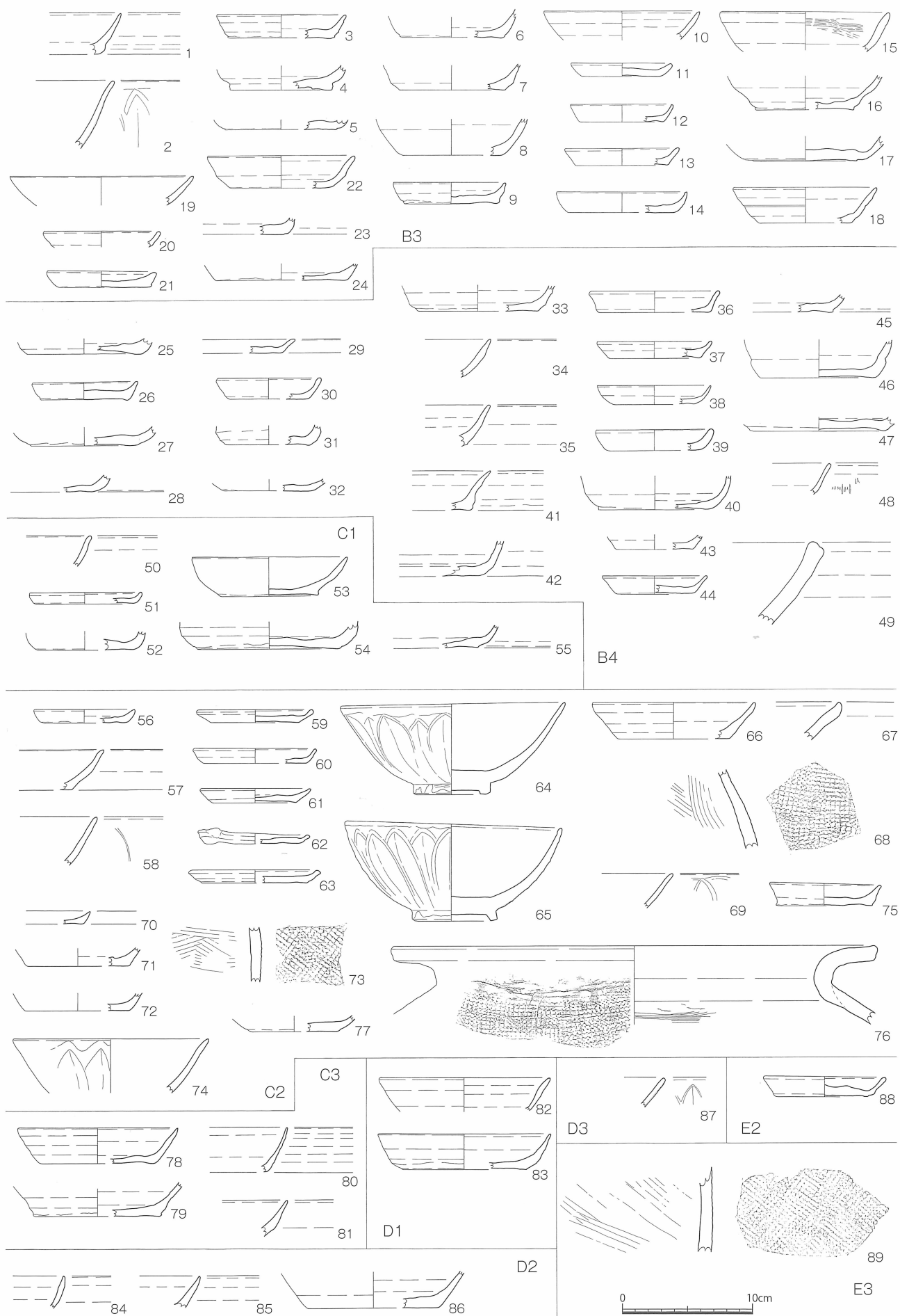
第 16 図 上小野遺跡出土遺物実測図② (S=1/4)
