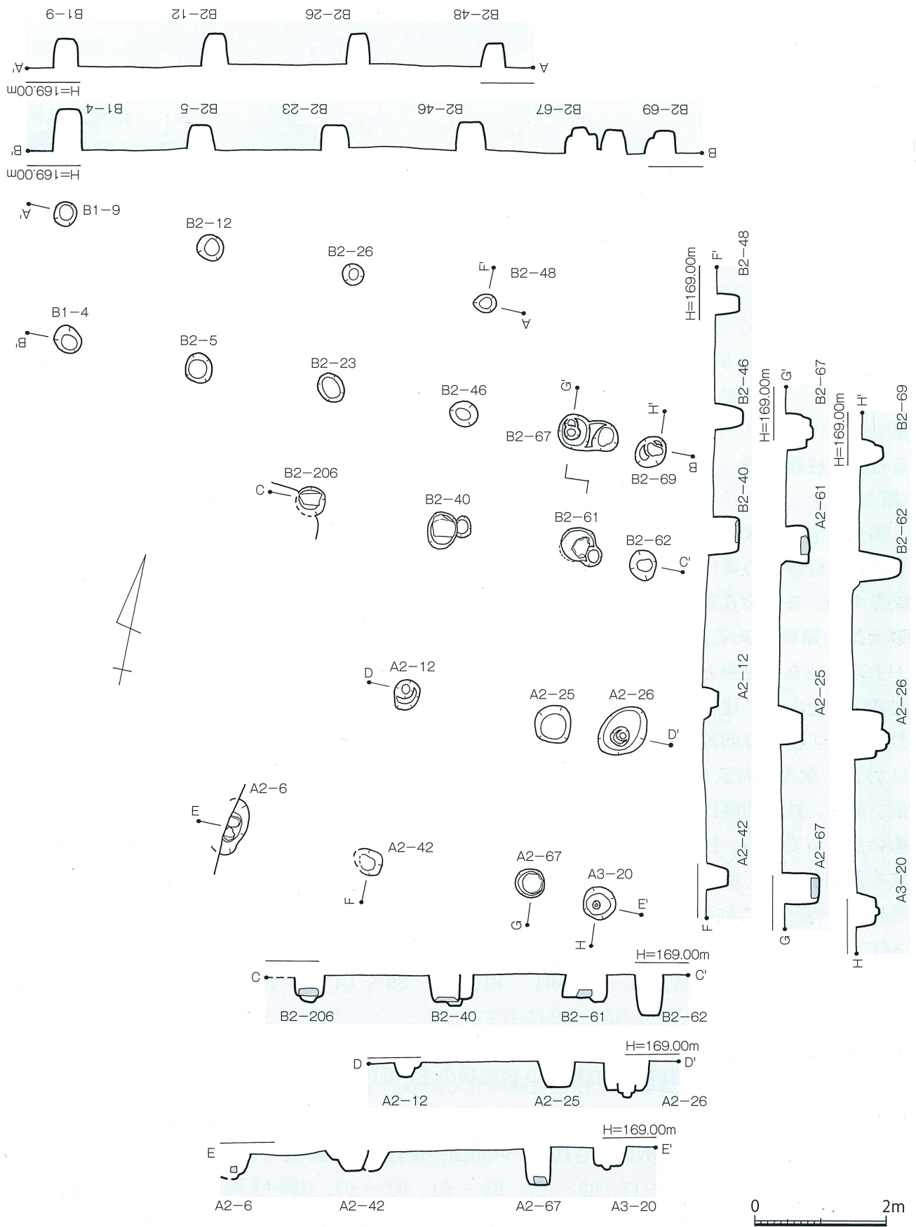
第7図 上小野遺跡3号掘立柱建物跡実測図 (S=1/80)
