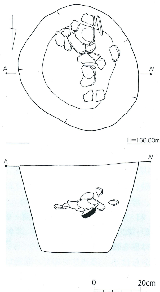
第11図 上小野遺跡C 2-9 実測図 (S=1/10)
