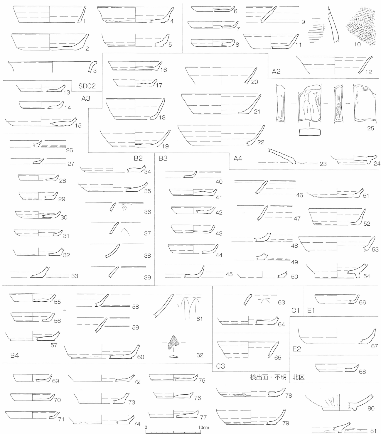
第17図 上小野遺跡出土遺物実測図③ (S=1/4)
