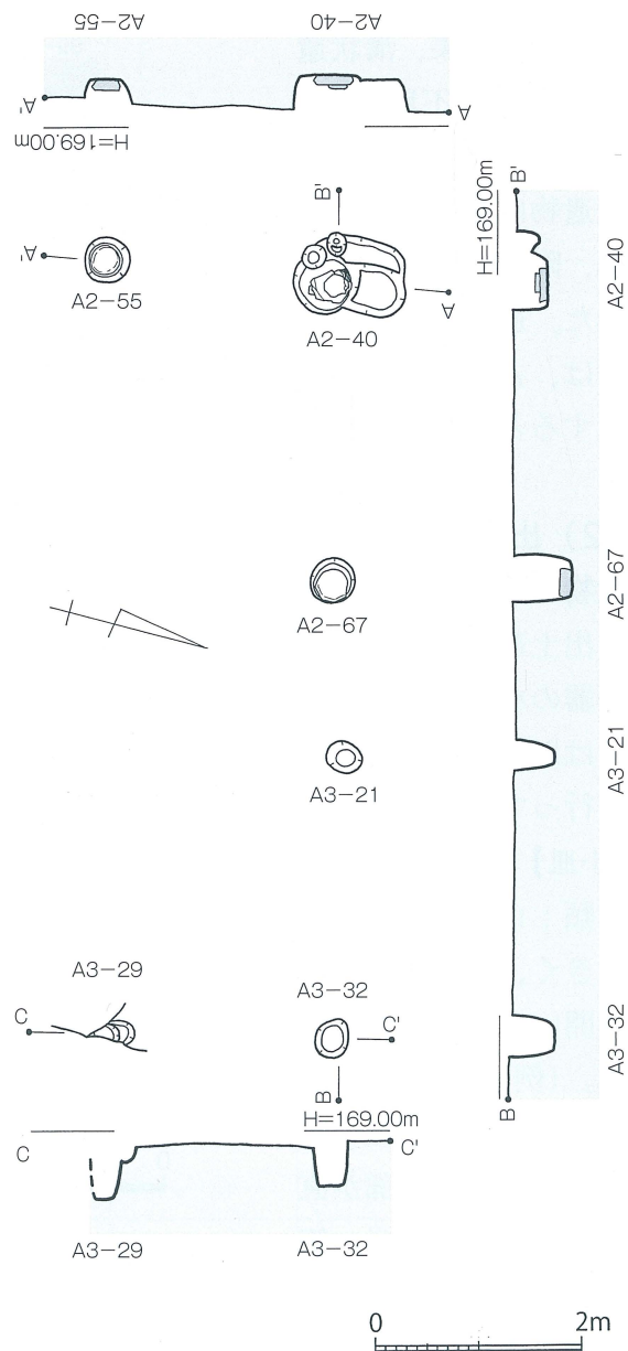
第6図 上小野遺跡2号掘立柱建物跡実測図 (S=1/80)
