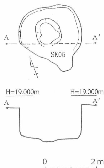
第 15 図 弥五郎遺跡 2 次 1 区 SK05 実測図 (S=1/80)
