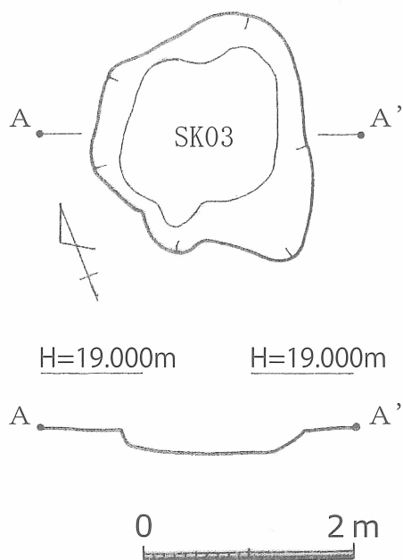
第 24 図 弥五郎遺跡 2 次 2 区 SK03 (S=1/80)
