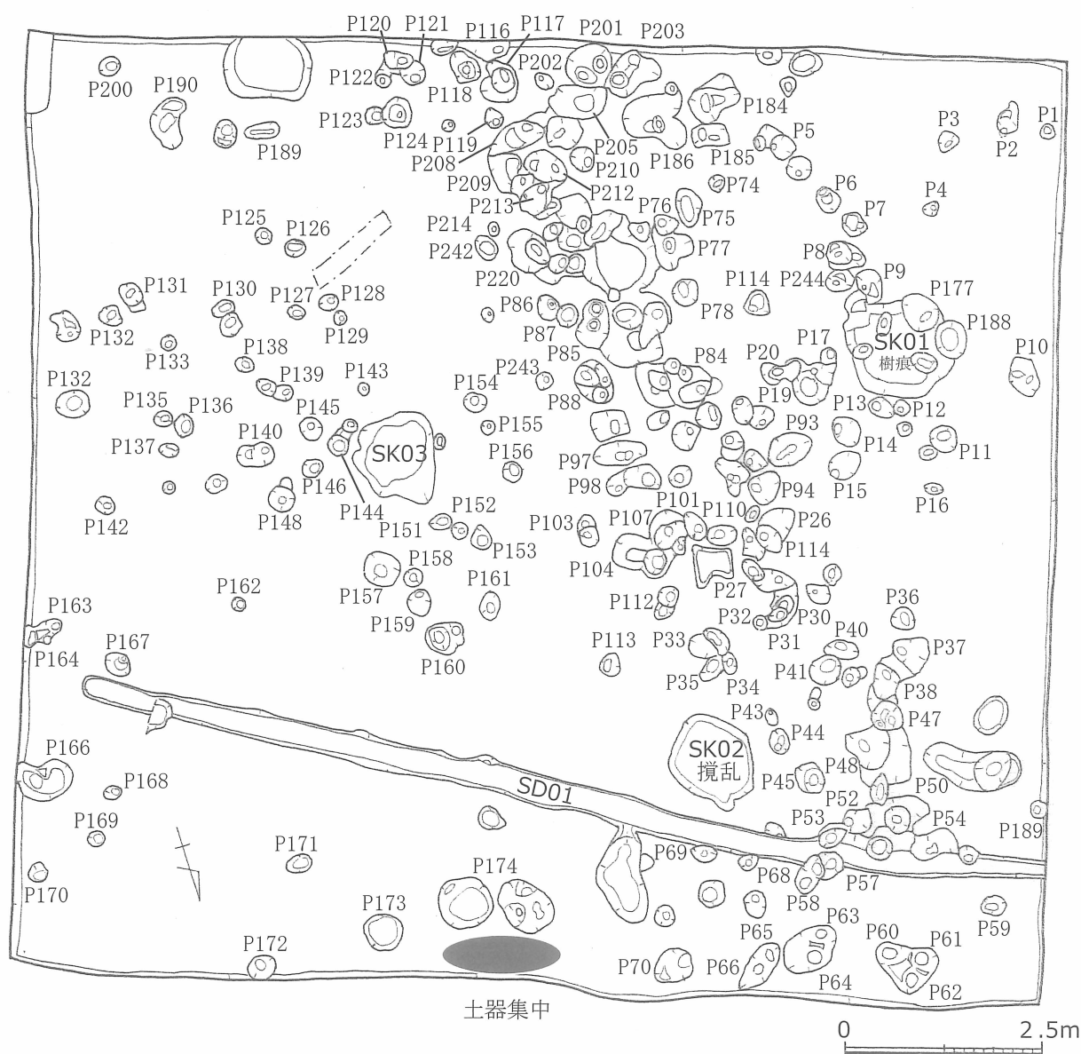
第22図 弥五郎遺跡2次2区調査区全体図 (S=1/200)
