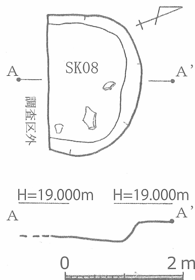
第 16 図 弥五郎遺跡 2 次 1 区 SK08 実測図 (S=1/80)
