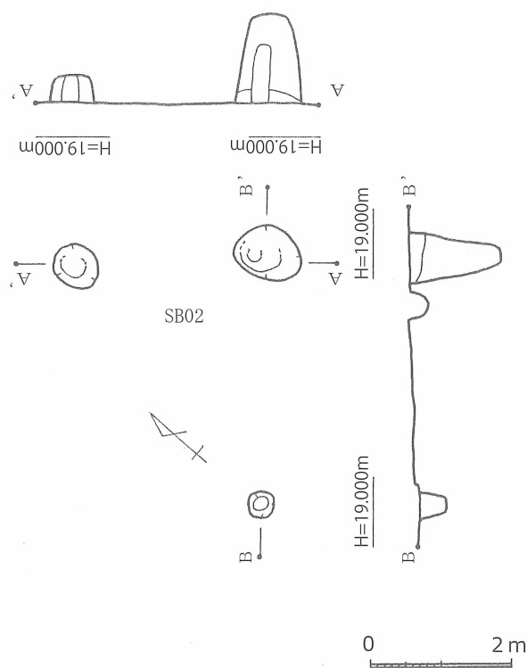
第6図 弥五郎遺跡2次1区SB02実測図 (S=1/80)
