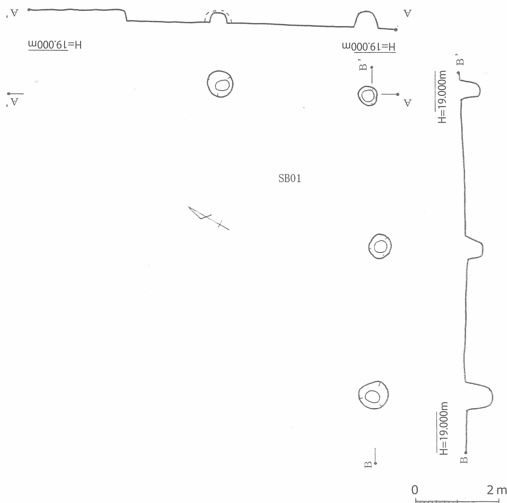
第5図 弥五郎遺跡2次1区SB01実測図（S=1/80）
