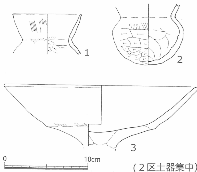
第26図 弥五郎遺跡2次2区土器集中部出土遺物 (S=1/4)
