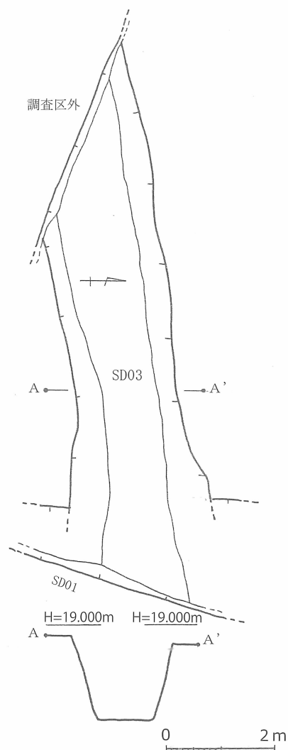
第9図 弥五郎遺跡2次1区SD03 実測図 (S=1/100)
