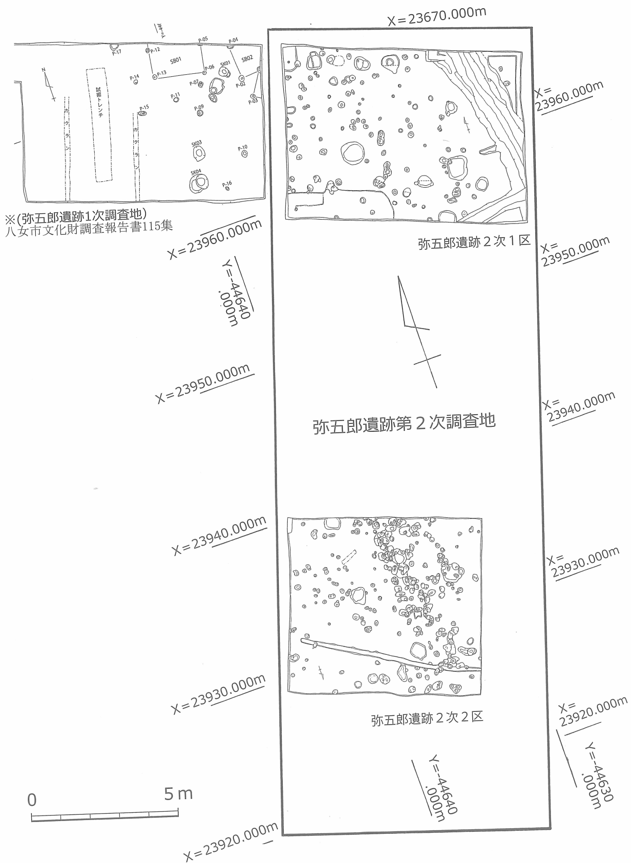
第3図 弥五郎遺跡調査区全体図 (S=1/500)
