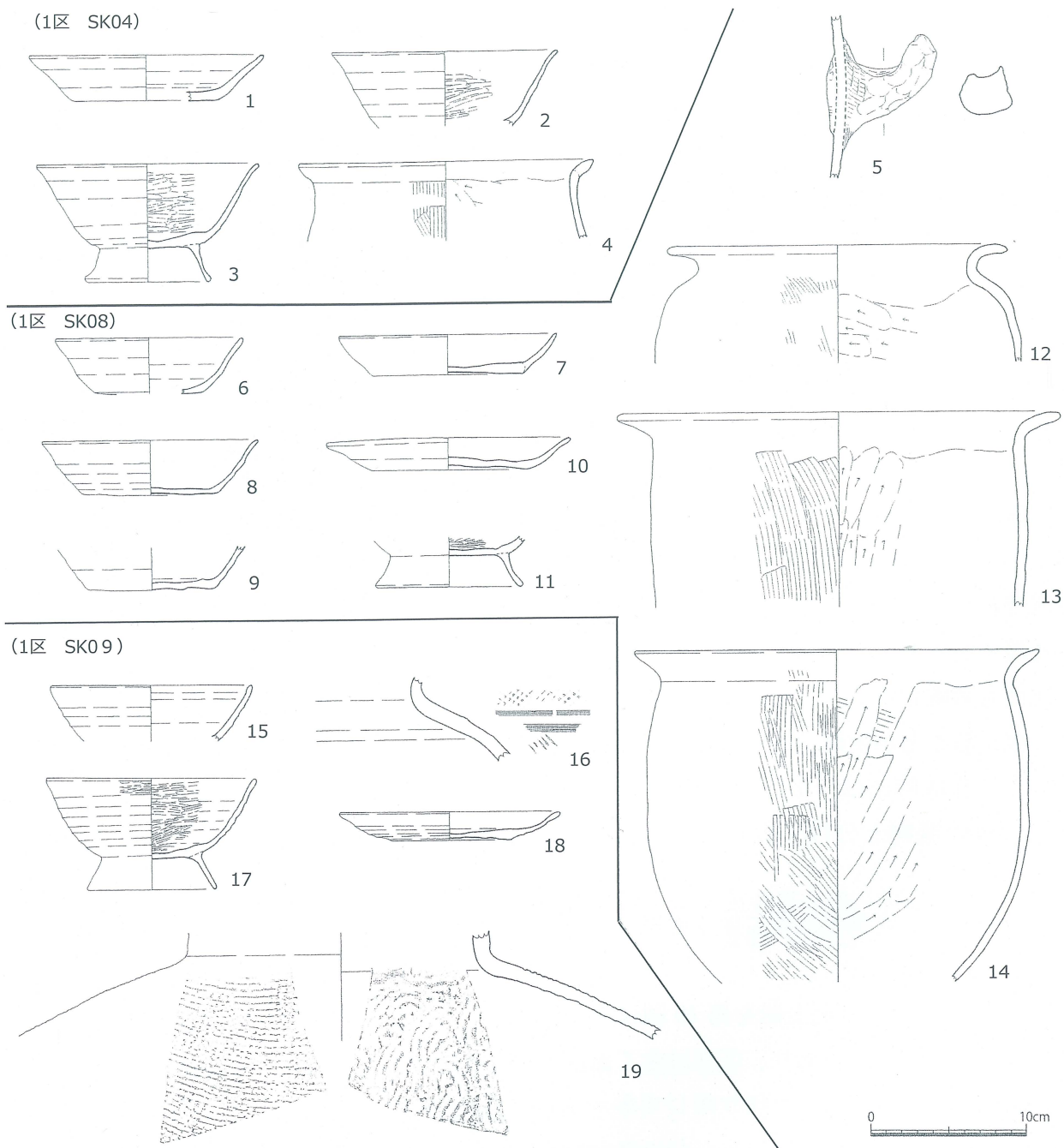
第17図 弥五郎遺跡2次1区SK04・SK08・SK09出土遺物 (S=1/4)
