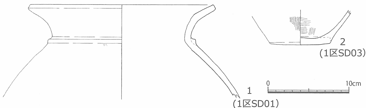
第7図 弥五郎遺跡2次1区SD01・SD03出土土器 (S=1/4)
