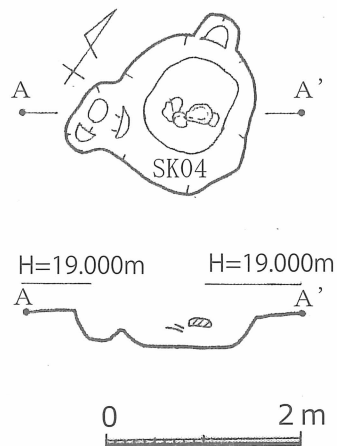
第 14 図 弥五郎遺跡 2 次 1 区 SK04 実測図 (S=1/80)
