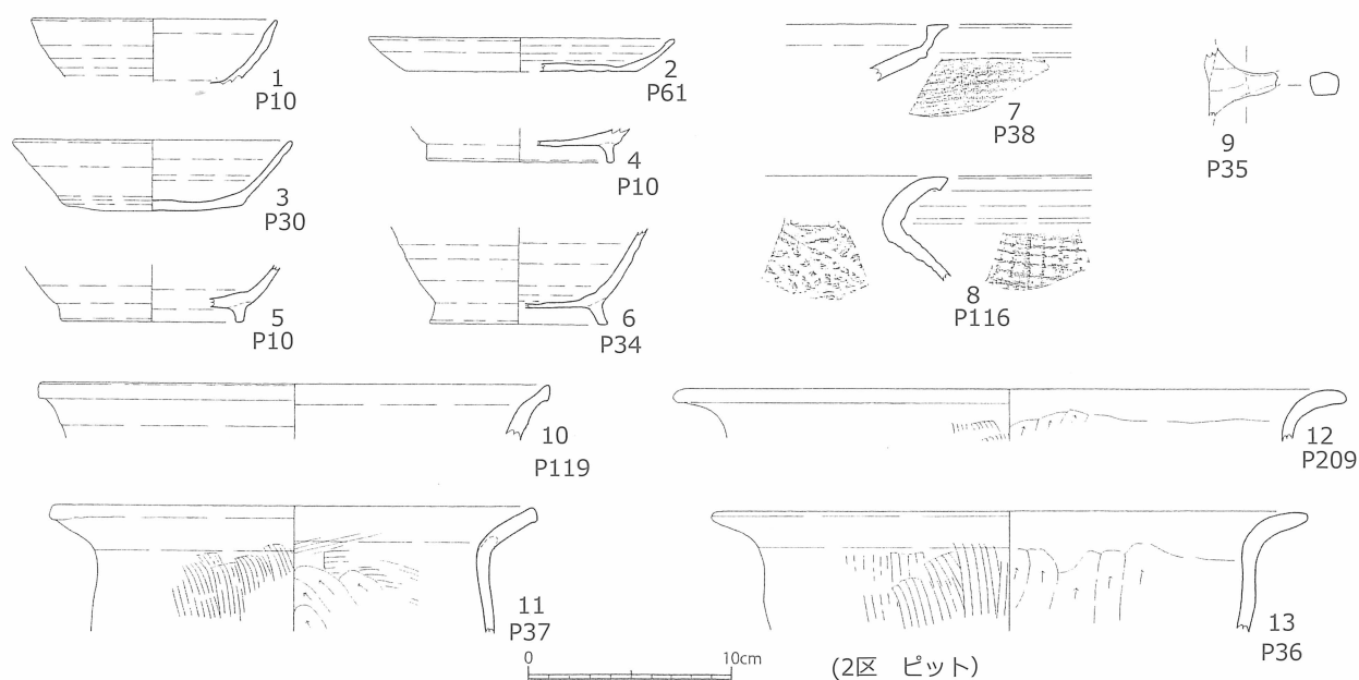
第25図 弥五郎遺跡2次2区ピット出土遺物実測図 (S=1/4)
