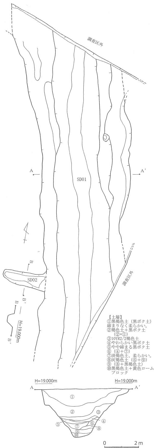
第8図 弥五郎遺跡2次1区SD01実測図（S=1/100）
