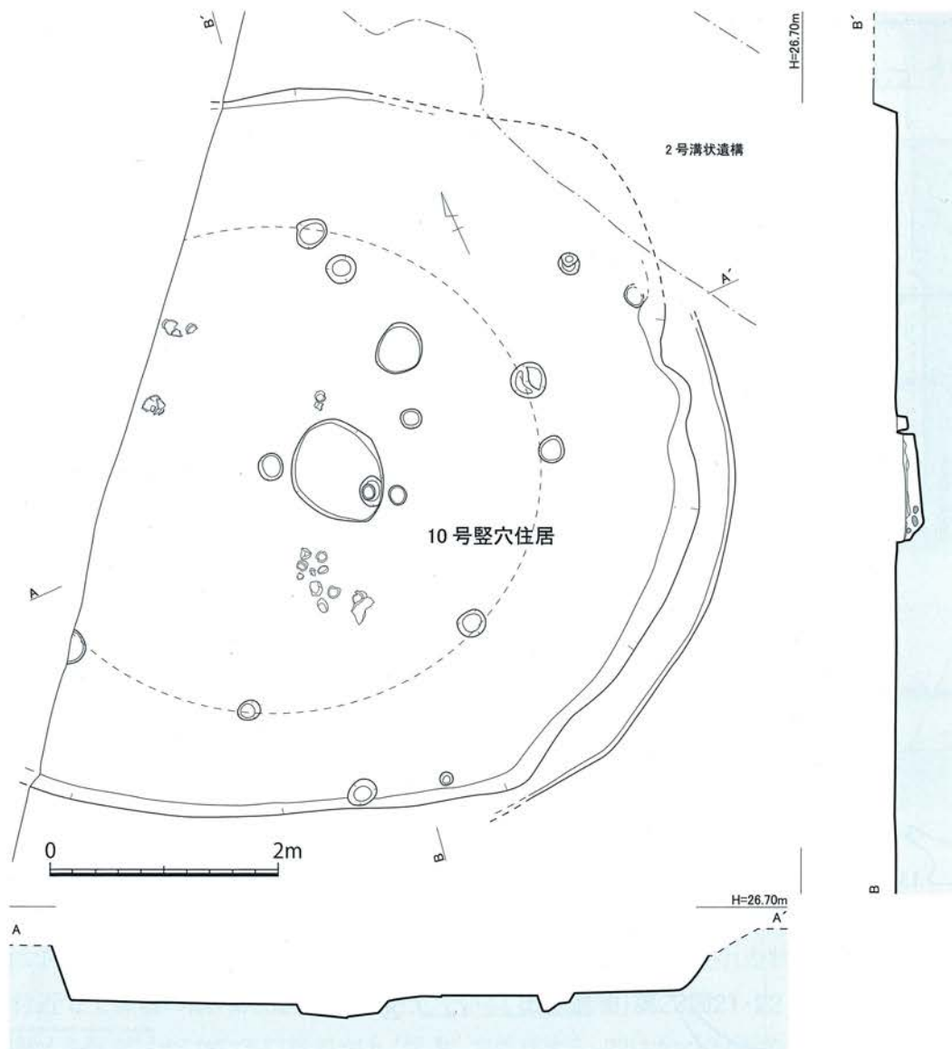
第16図 島田遺跡 10号竪穴住居(SB10) 実測図[1/60]
