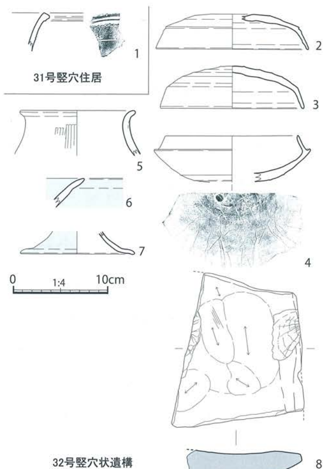
第45図 島田遺跡 31号竪穴住居、32号竪穴状遺構(SB31・32) 出土遺物実測図 [1/4]
