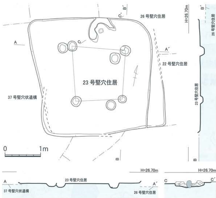
第33図 島田遺跡 23号竪穴住居 (SB23) 実測図 [1/60]
