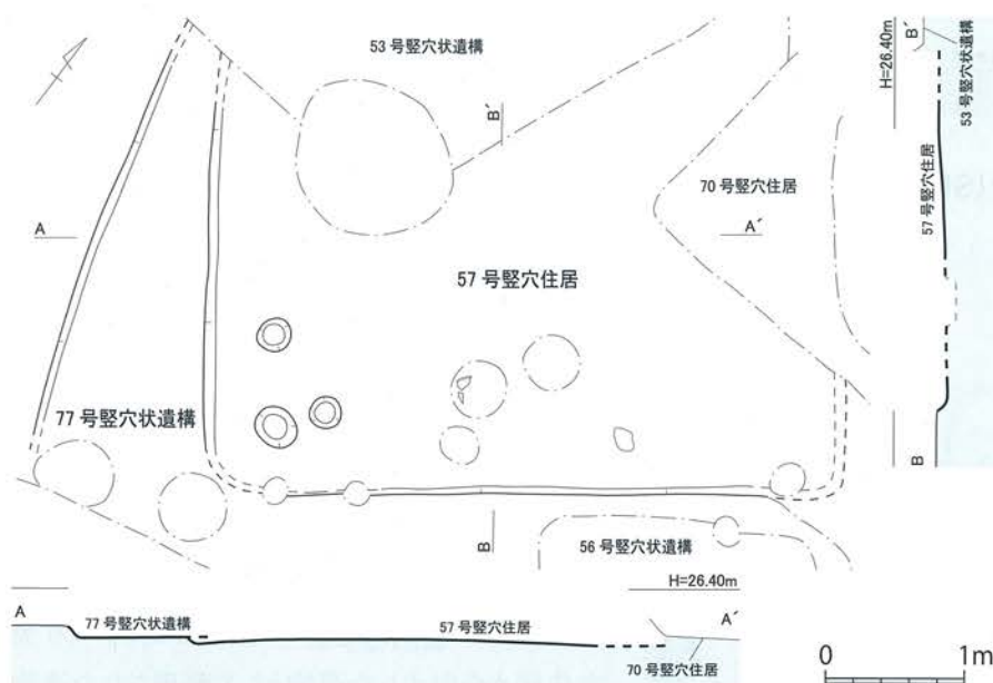
第71図 島田遺跡 57号堅穴住居、77号堅穴状遺構(SB57・77) 実測図[1/60]
