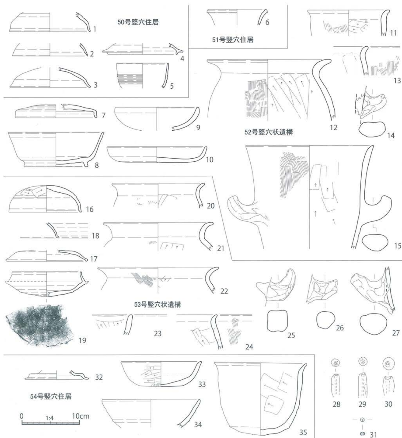
第 69 図 島田遺跡 50・51・54号竪穴住居、52・53号竪穴状遺構(SB50・51・52・53・54) 出土遺物実測図 [1/4]
