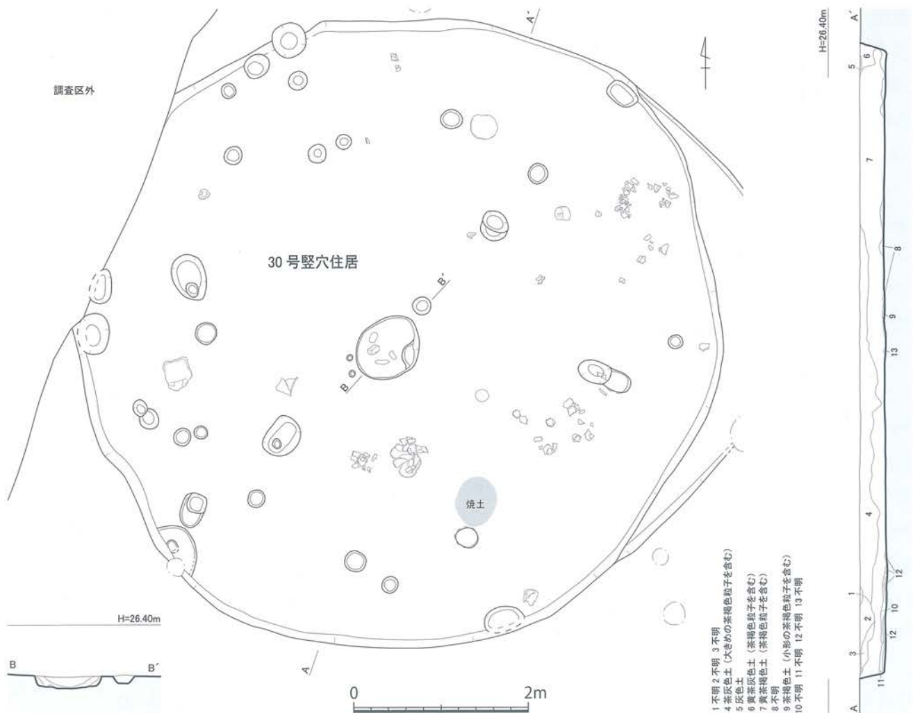
第41図 島田遺跡 30号竖穴住居(SB30) 実測図[1/60]
