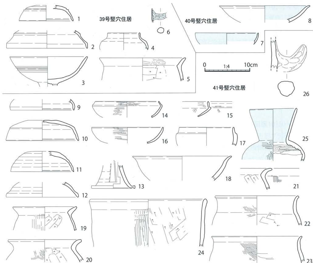
第 54 図 島田遺跡 39・40・41号竪穴住居(SB39・40・41) 出土遺物実測図[1/4]
