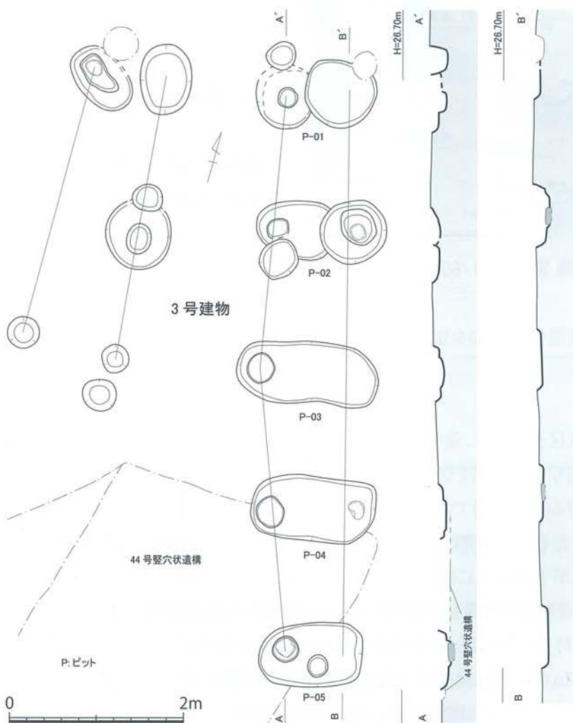
第96図 島田遺跡 3号建物 実測図[1/60]
