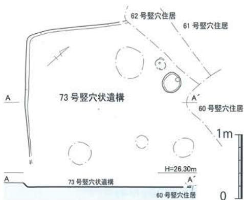
第 83 図 島田遺跡 73号竖穴状遺構 (SB73) 実測図 [1/60]
