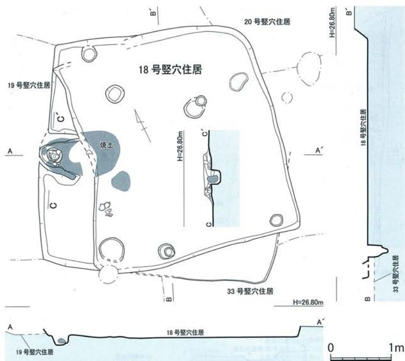
第26図 島田遺跡 18号竖穴住居(SB18) 実測図[1/60]
