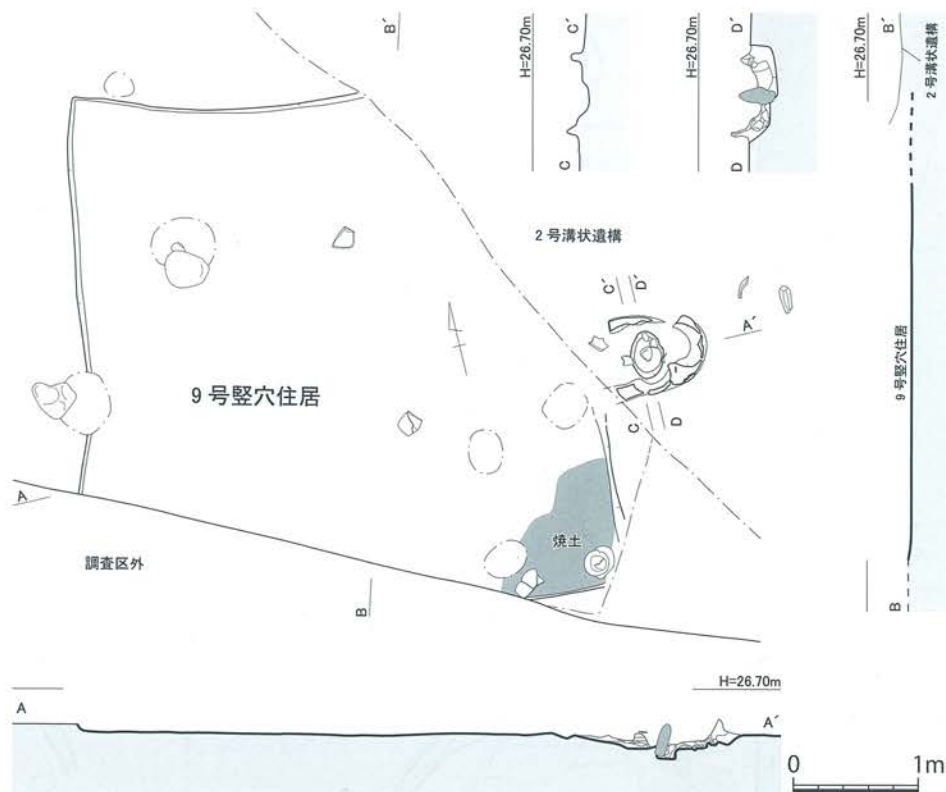
第14図 島田遺跡 9号竪穴住居(SB09) 実測図[1/60]
