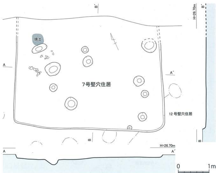
第12図 島田遺跡 7号竪穴住居 (SB07) 実測図 [1/60]
