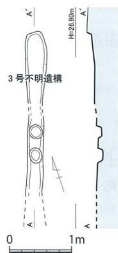
第111図 島田遺跡 3号不明遺構 実測図[1/60]
