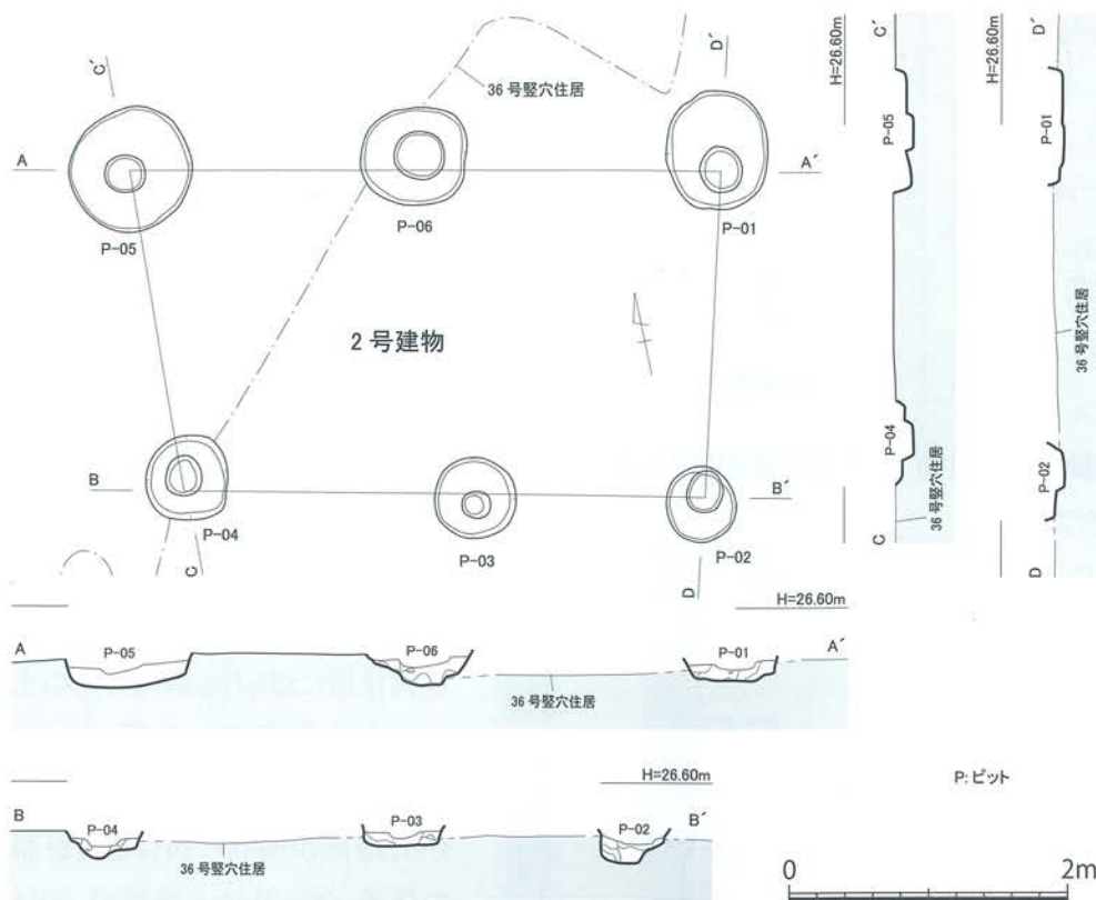
第95図 島田遺跡 2号建物 実測図[1/60]
