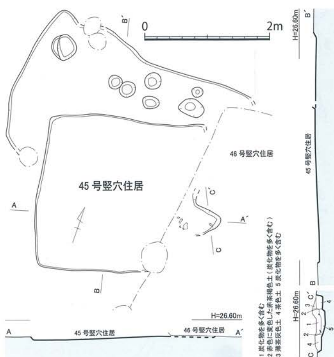
第59図 島田遺跡 45号竪穴住居 (SB45) 実測図[1/60]
