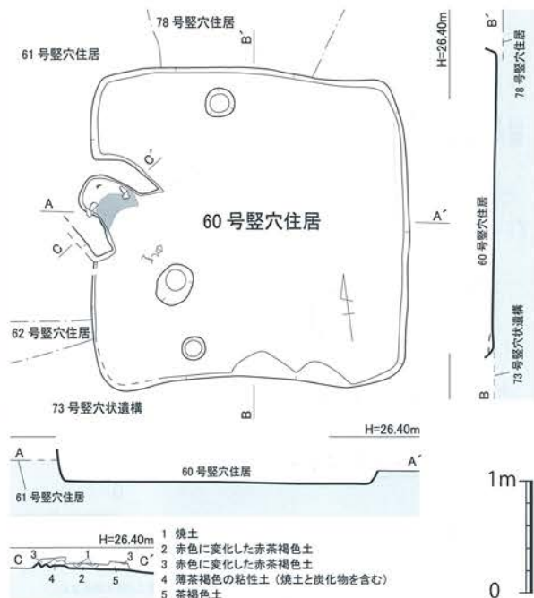
第75図 島田遺跡 60号竖穴住居(SB60) 実測図[1/60]
