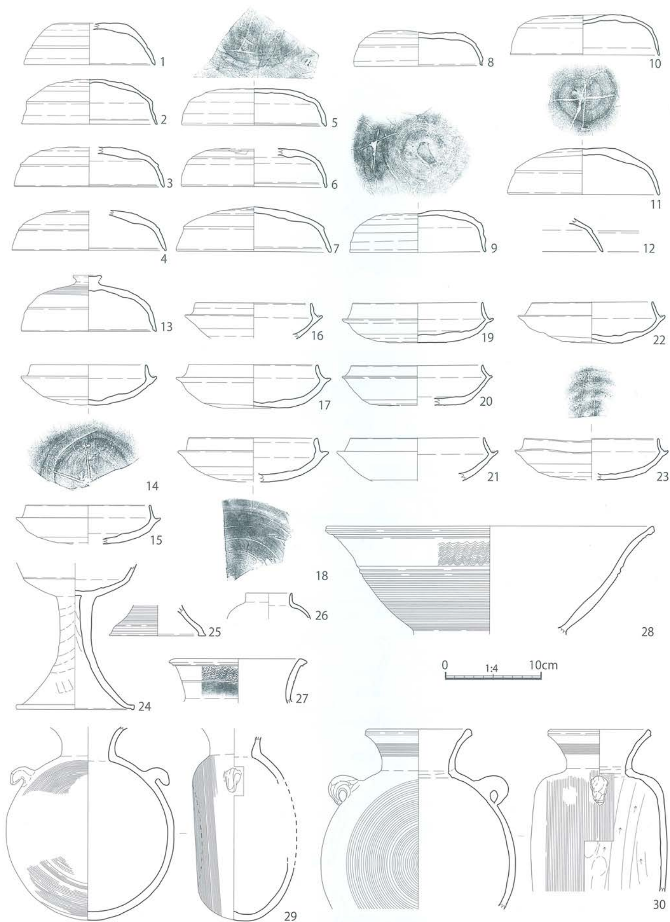
第 103 図 島田遺跡 2号溝状遺構(SD02) 出土遺物実測図① [1/4]
