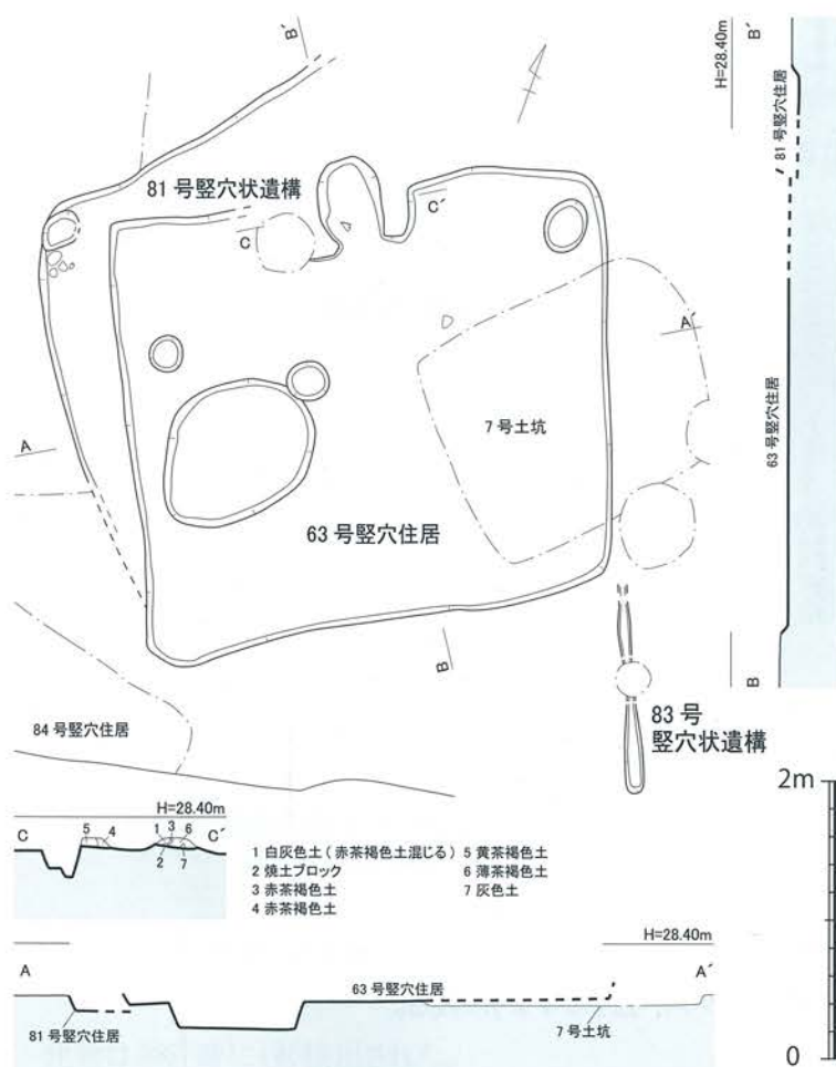
第77図 島田遺跡 63号竖穴住居、81・83号竖穴状遺構(SB63・81・83) 実測図[1/60]
