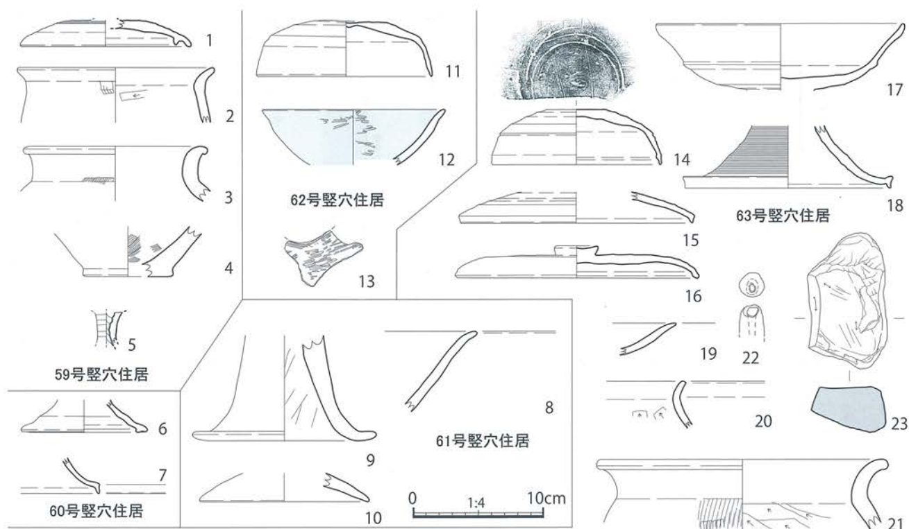
第 78 図 島田遺跡59~63号竖穴住居(SB59~63) 出土遺物実測図[1/4]
