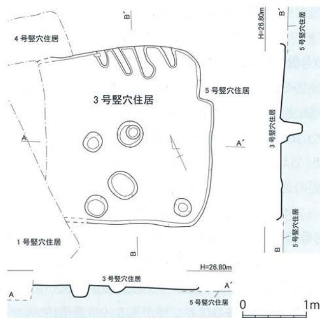
第8図 島田遺跡 3号竖穴住居(SB03) 実測図[1/60]
