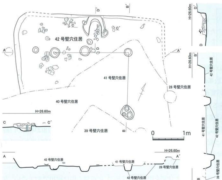
第 55 図 島田遺跡 42号竪穴住居(SB42) 実測図[1/60]
