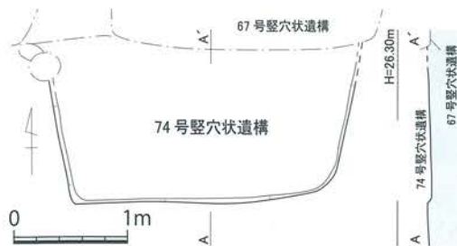
第 85 図 島田遺跡 74号竖穴状遺構 (SB74) 実測図 [1/60]
