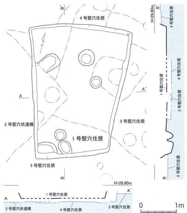
第5図 島田遺跡 1号竪穴住居 (SB01) 実測図 [1/60]
