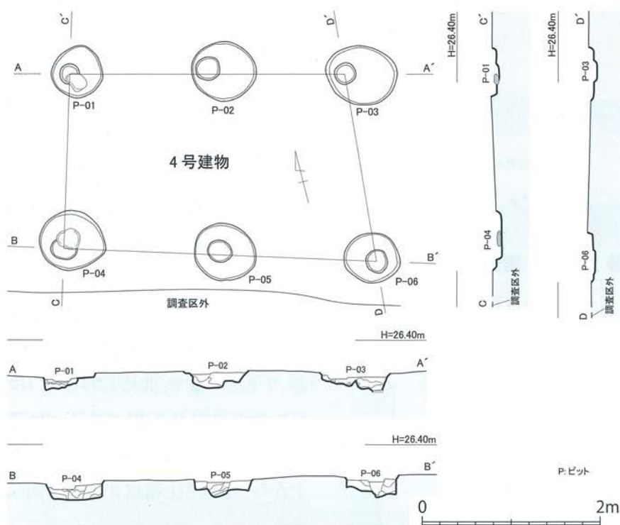
第 98 図 島田遺跡 4号建物 実測図[1/60]
