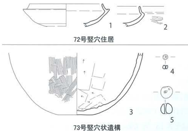
第 84 図 島田遺跡 72号竖穴住居、73号竖穴状遺構 (SB72・73) 出土遺物実測図 [1/4]
