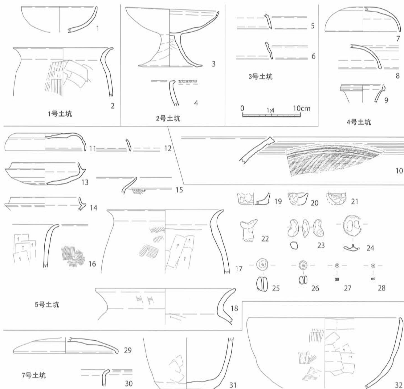
第100図 島田遺跡 土坑出土遺物実測図[1/4]
