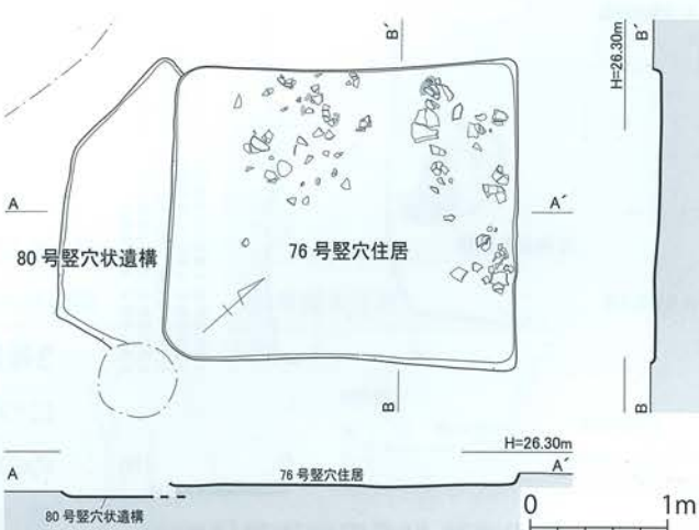
第 87 図 島田遺跡 76号竖穴住居、80号竖穴状遺構 (SB76・80) 実測図 [1/60]
