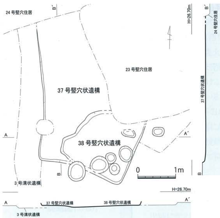
第 51 図 島田遺跡 37・38号竪穴状遺構 (SB37・38) 実測図 [1/60]
