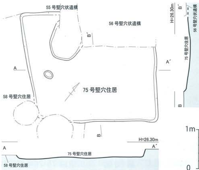
第 86 図 島田遺跡 75号竖穴住居 (SB75) 実測図 [1/60]
