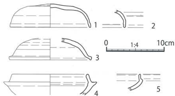
第72図 島田遺跡 57号堅穴住居(SB57) 出土遺物実測図[1/4]
