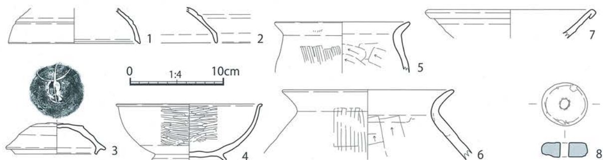
第 115 図 島田遺跡 その他の遺物 実測図[1/4]
