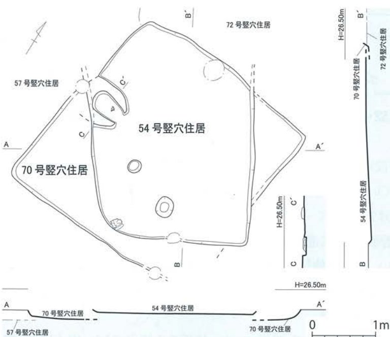
第 68 図 島田遺跡 54・70号竪穴住居(SB54・70) 実測図[1/60]
