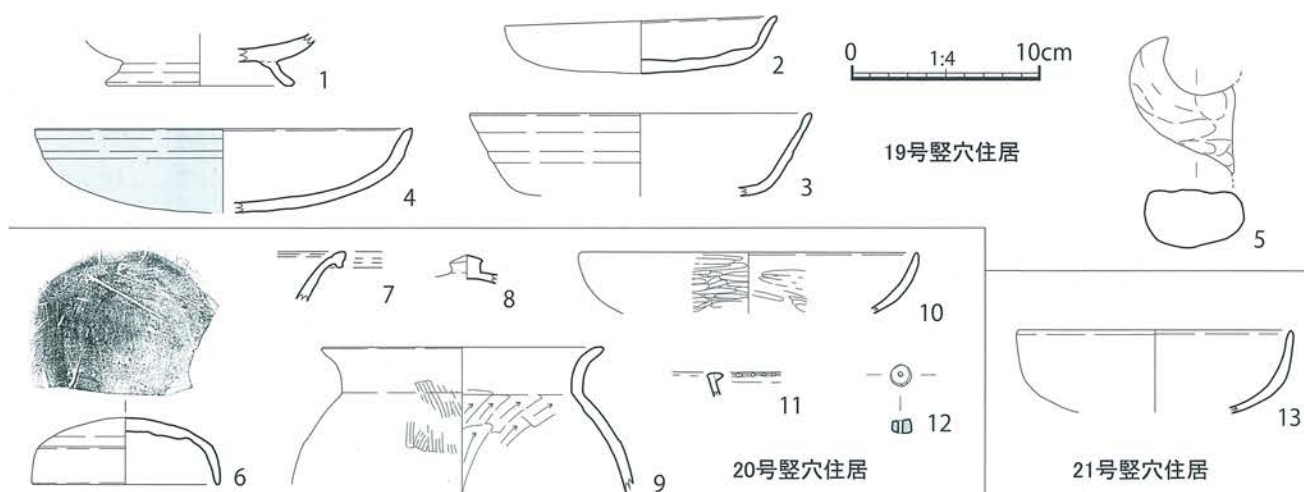
第31図 島田遺跡 19・20・21号竪穴住居(SB19・20・21) 出土遺物実測図[1/4]
