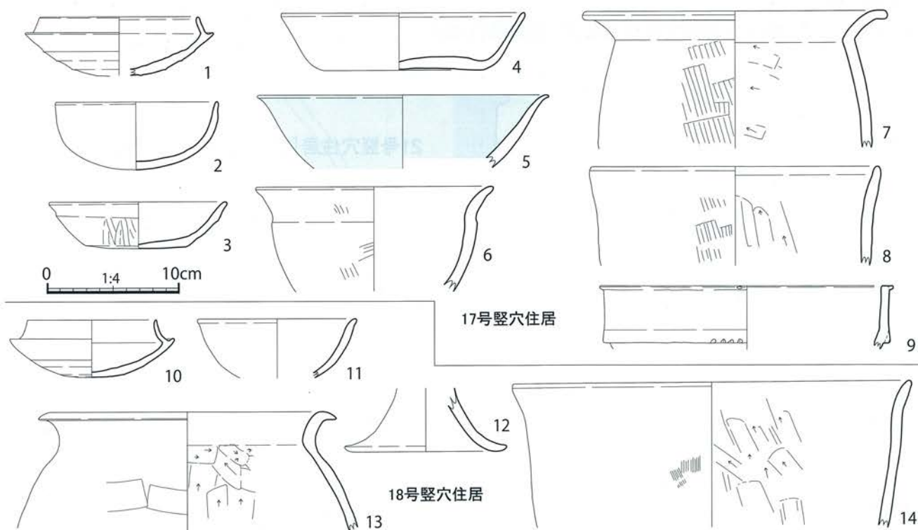
第27図 島田遺跡 17・18号竖穴住居(SB17・18) 出土遺物実測図[1/4]
