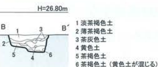
第99図 島田遺跡 1~7号土坑(SK01~07) 実測図[1/60]
