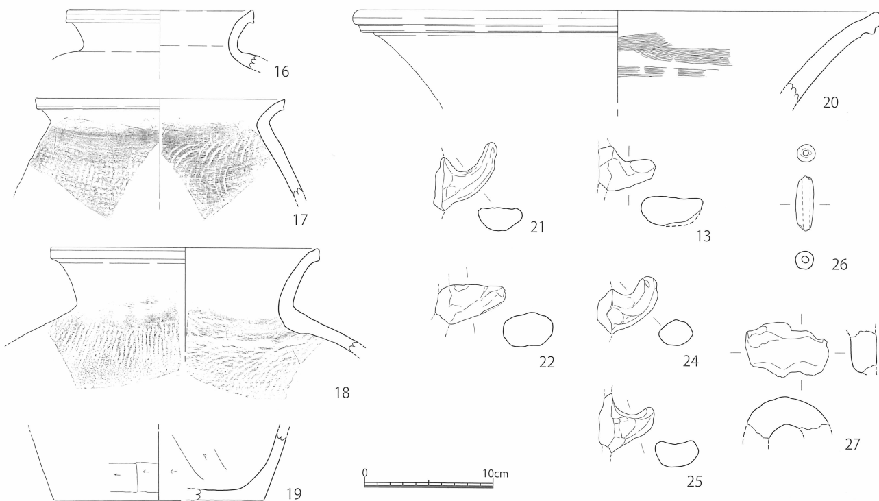
第 25 図 国伏遺跡 1号溝状遺構(SD01) 出土遺物実測図 [1/4]
