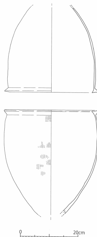
第 57 図 松ノ本遺跡B地点 8号甕棺実測図[1/8]
