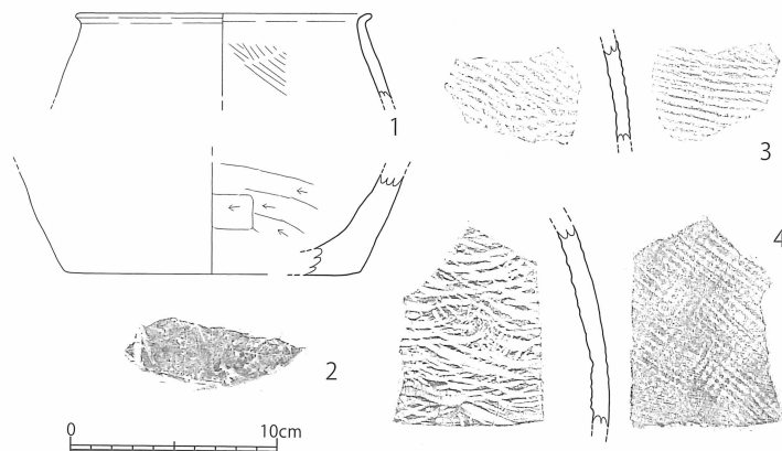
第 30 図 国伏遺跡 表採遺物実測図 [1/4]
