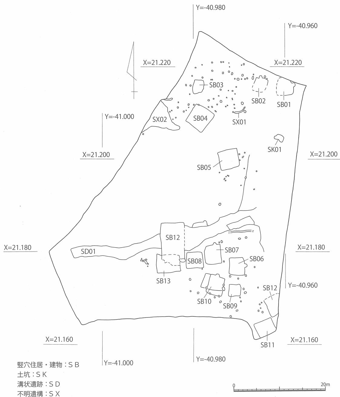
第 4 図 国伏遺跡 遺構配置図[1/500]
