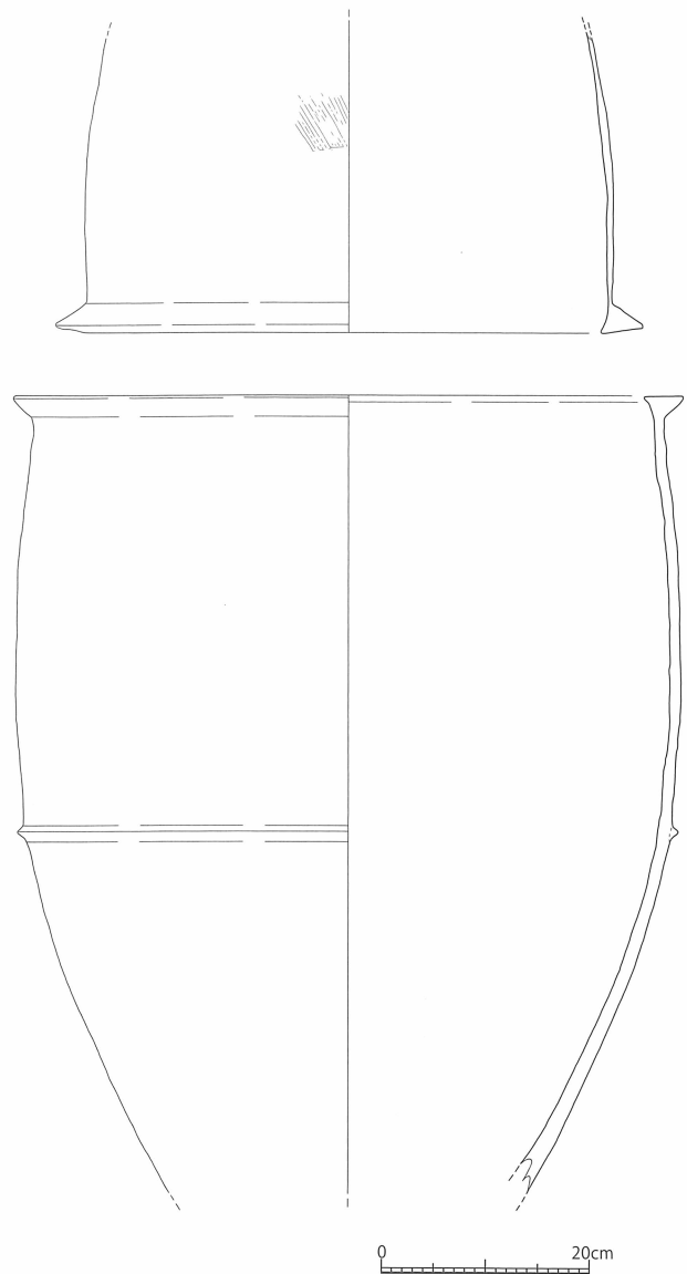
第59図 松ノ本遺跡B地点 9号甕棺実測図[1/8]
