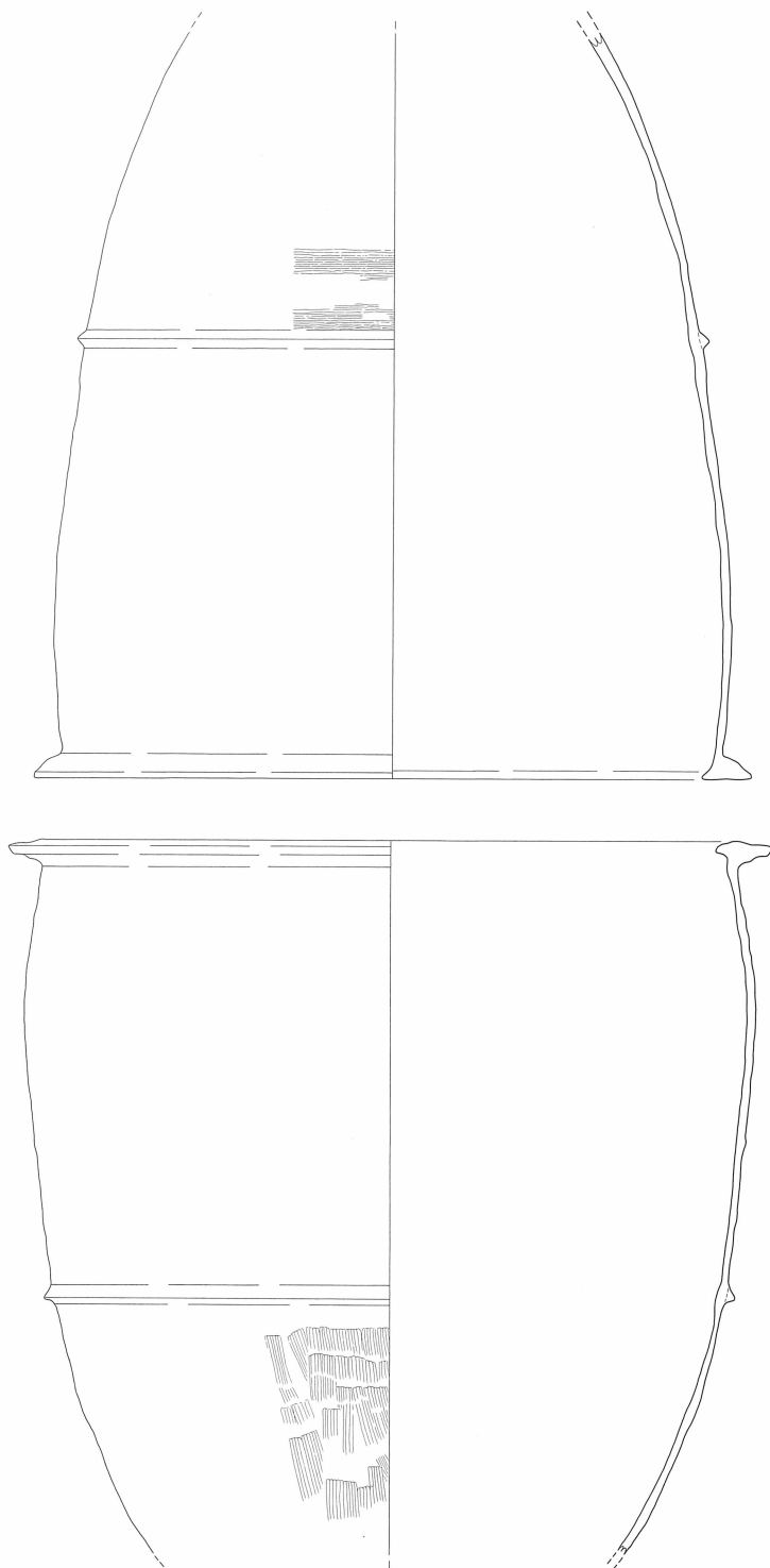
第 52 図 松ノ本遺跡B地点 3号甕棺実測図[1/8]
