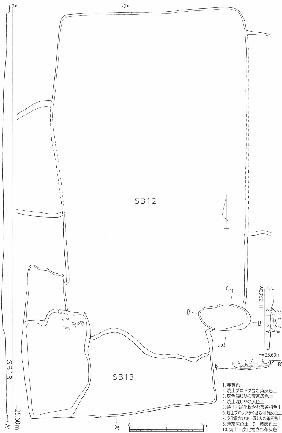
第 20 図 国伏遺跡 12・13号竪穴住居 (SB12・13) 実測図 [1/60]
