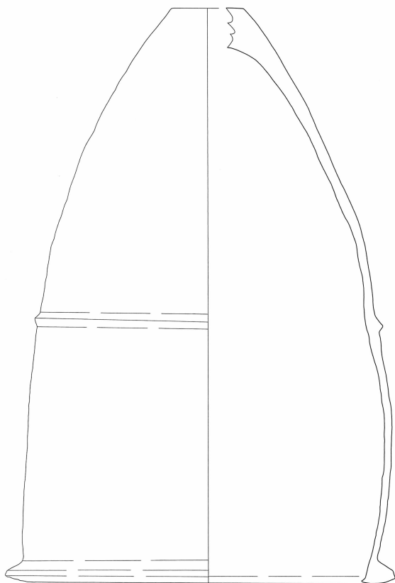
第 50 図 松ノ本遺跡B地点 2号甕棺出土遺物実測図 [1/4]
