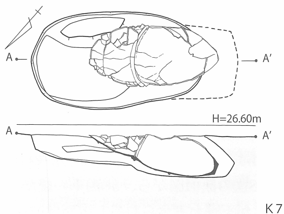
第 48 図 松ノ本遺跡B地点 1~8号甕棺墓(K01~08)実測図[1/40]
