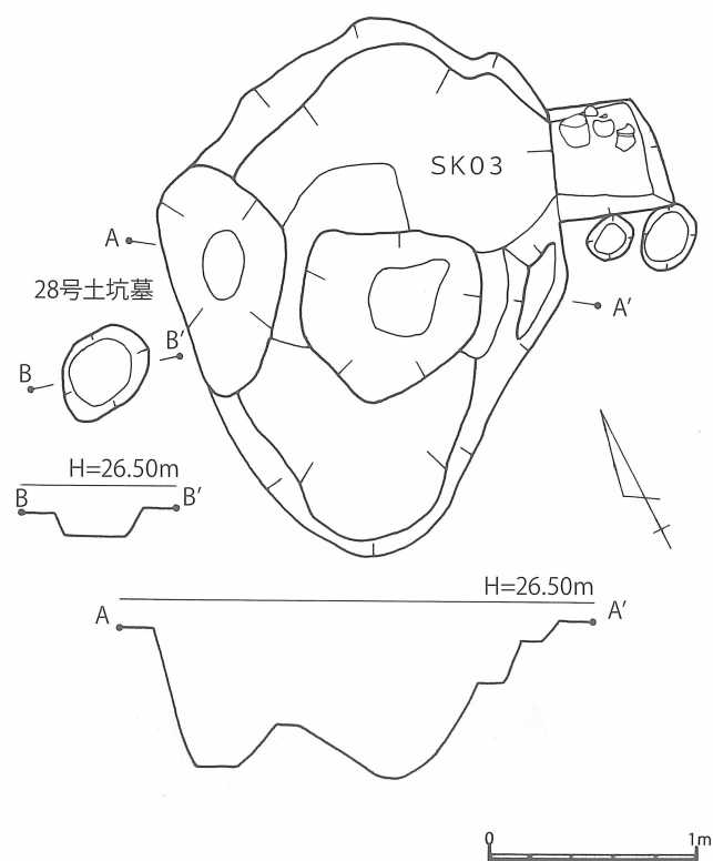
第 68 図 松ノ本遺跡B地点 28号土坑墓・3号不明遺構 (SX03) 実測図 [1/40]
