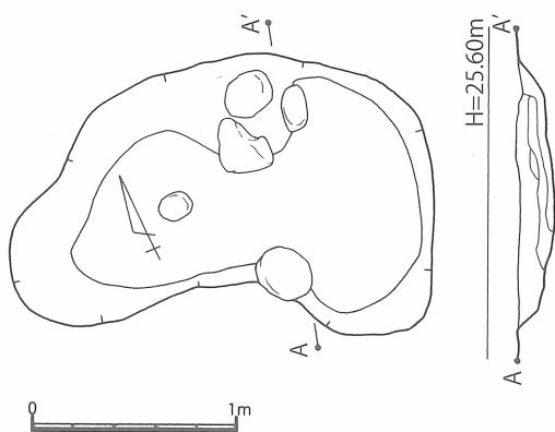
第 22 図 国伏遺跡 1号土坑(SK01)実測図[1/40]
