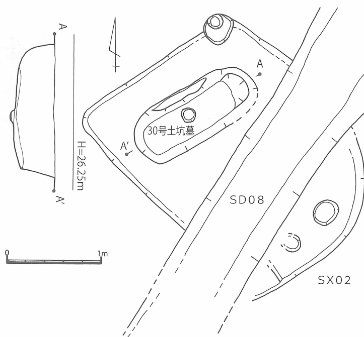
第 69 図 松ノ本遺跡B地点 30号土坑墓・8号溝状遺構 (SD08) ・2号不明遺構 (SX02) 実測図 [1/40]
