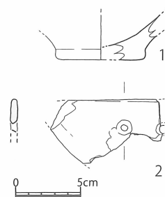
第 23 図 国伏遺跡 1号土坑(SK01) 出土遺物実測図[1/4]
