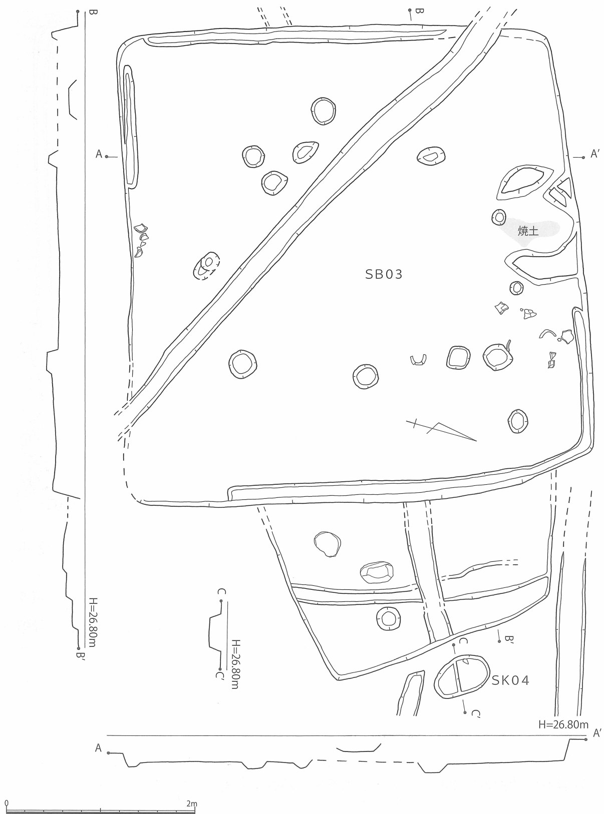
第 36 図 松ノ本遺跡A地点 3号竪穴住居 (SB03)、4号土坑 (SK04) 実測図 [1/40]
