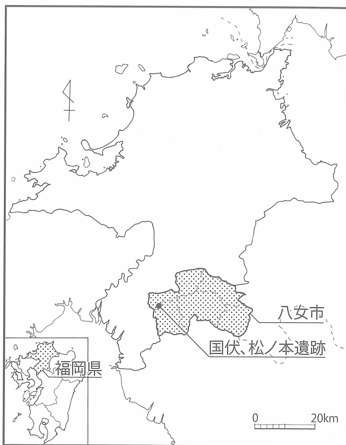
第1図 国伏遺跡・松ノ本遺跡 位置図 [1/125,000]
