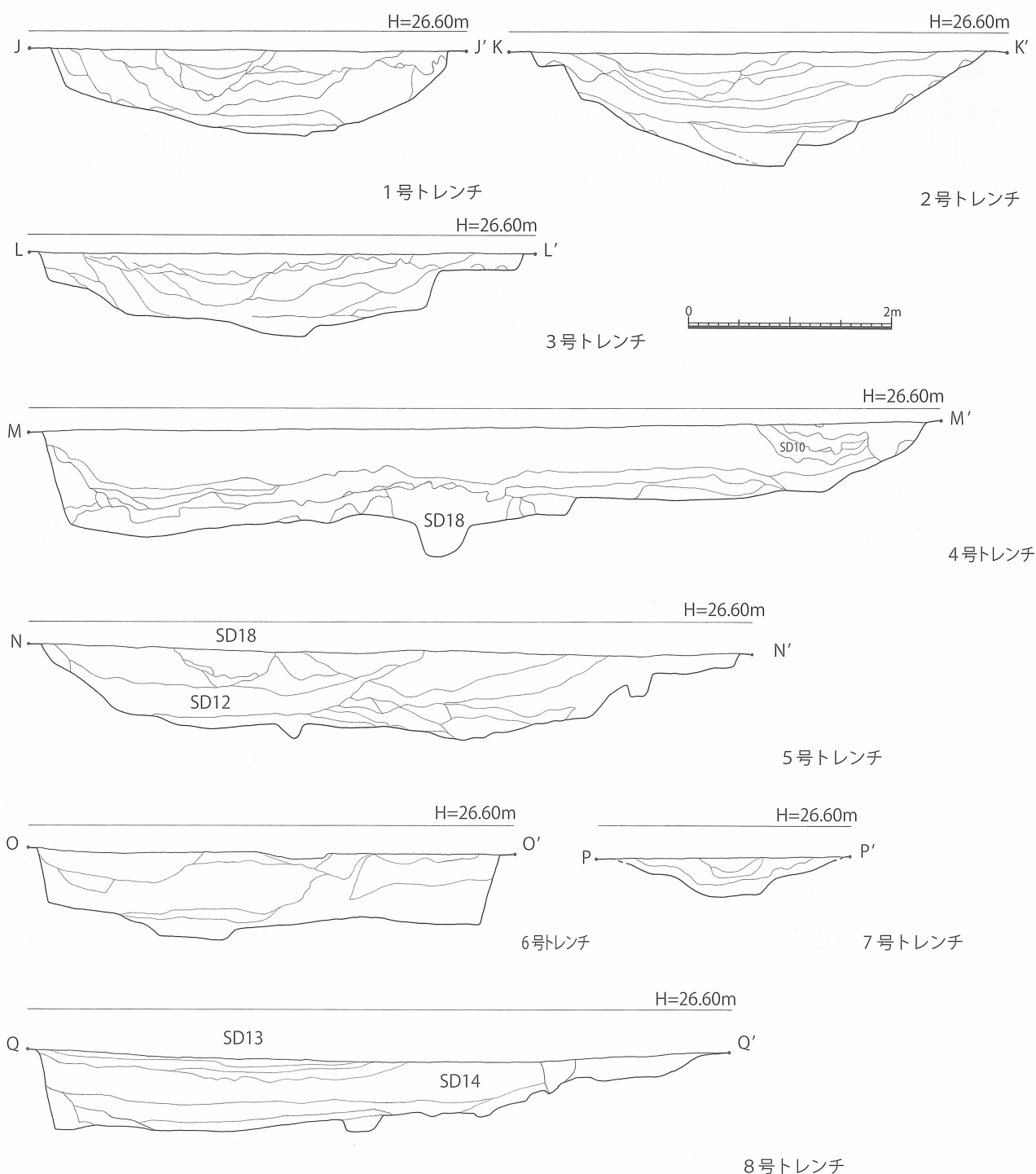
第 75 図 松ノ本遺跡B地点 1～8号トレンチ土層図[1/60]
