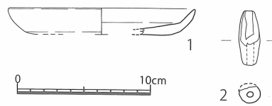
第 29 図 国伏遺跡 ピット出土遺物実測図 [1/4]
