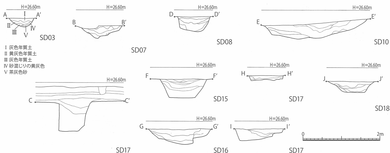
第 72 図 松ノ本遺跡B地点 3・7・8・10・15～18号溝状遺構(SD03・07・08・10・15～18)土層図〔1/60〕
