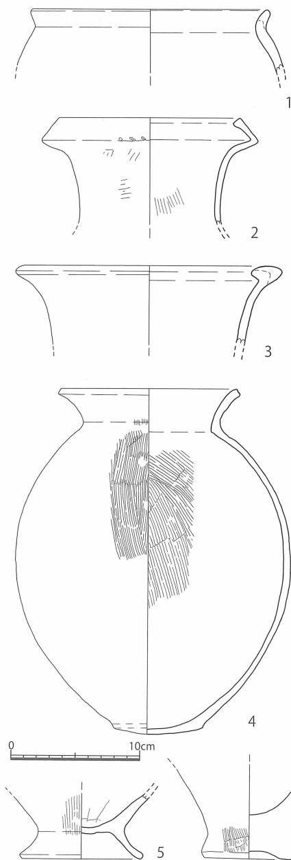
第 42 図 松ノ本遺跡A地点11号 溝状遺構 (SD11) 出土遺物実測図 [1/4]
