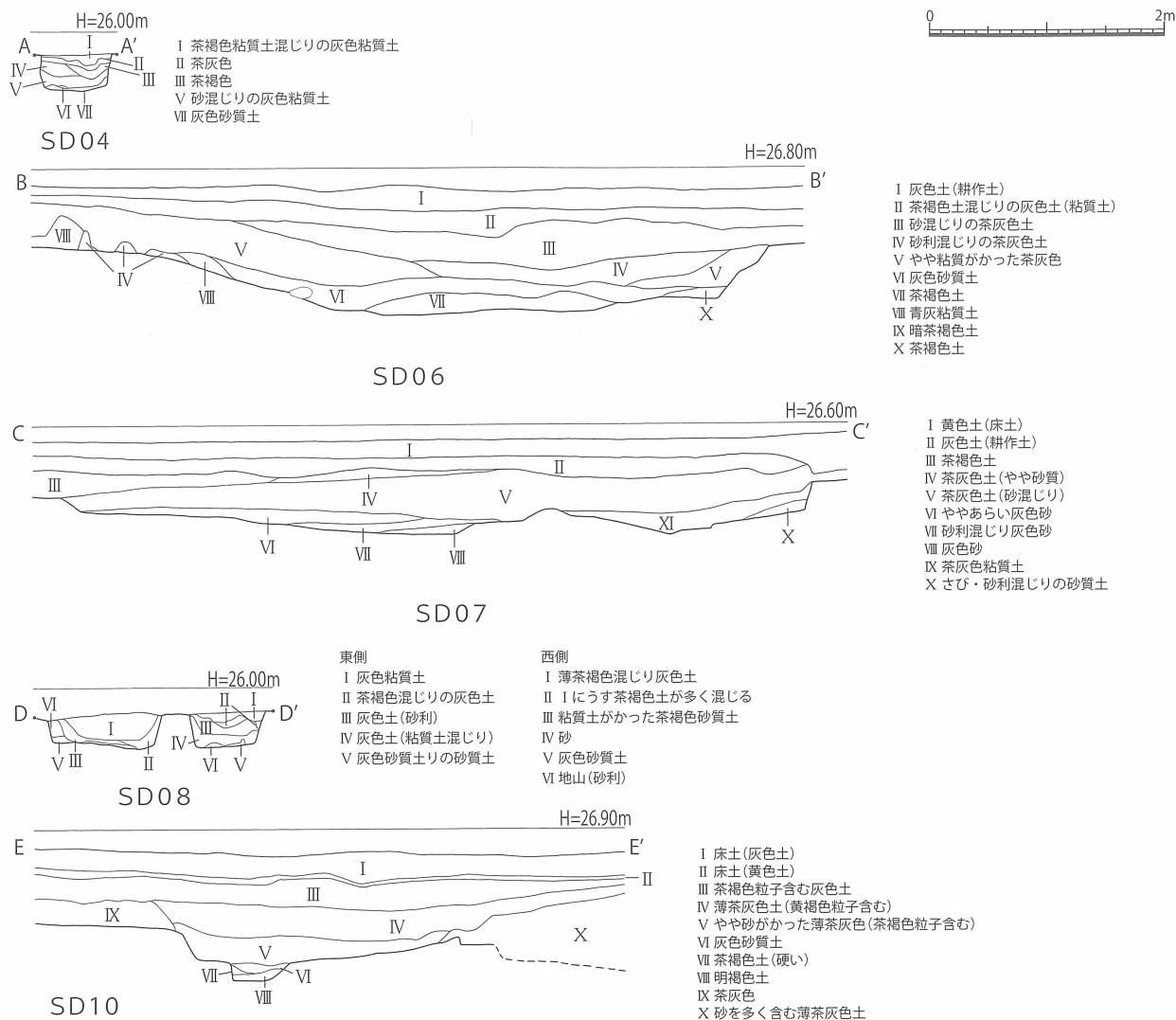
第 40 図 松ノ本遺跡A地点4・6・7・8・10号溝状遺構(SD04・06・07・08・10)実測図 [1/60]
