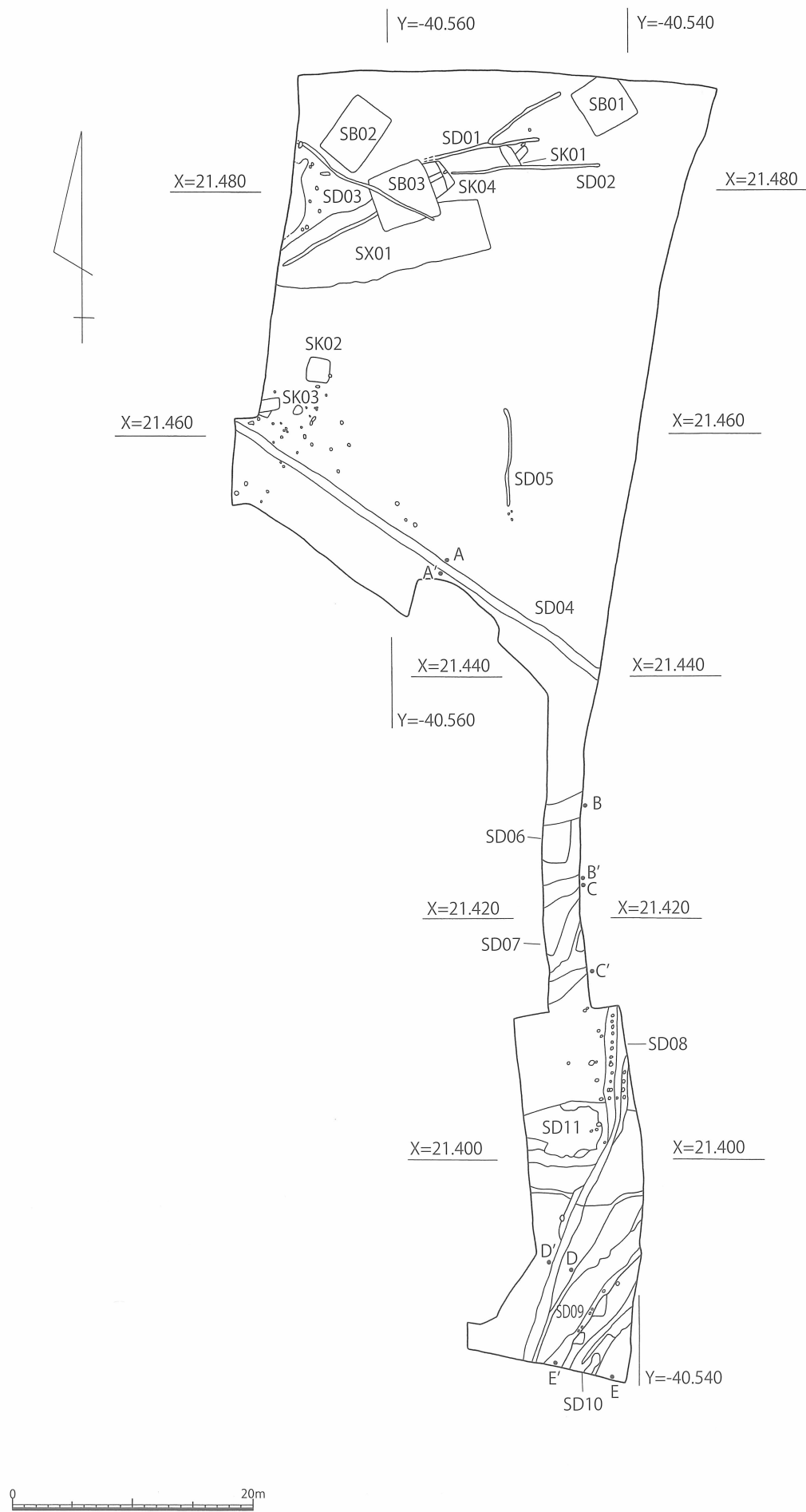
第 31 図 松ノ本遺跡A地点 遺構配置図 [1/500]
