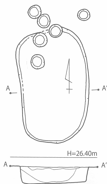
第 85 図 松ノ本遺跡E地点 1号土坑 (SK01)実測図 [1/40]
