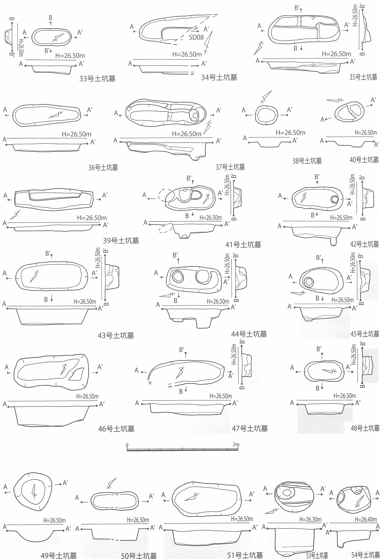
第 70 图 松ノ本遺跡B地点 33~51, 53, 54号土坑墓実測図[1/40]
