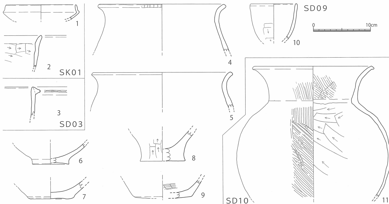
第 41 図 松ノ本遺跡A地点 1号土坑(SK01)、3・9・10号溝状遺構(SD03・09・10)出土遺物実測図 [1/4]
