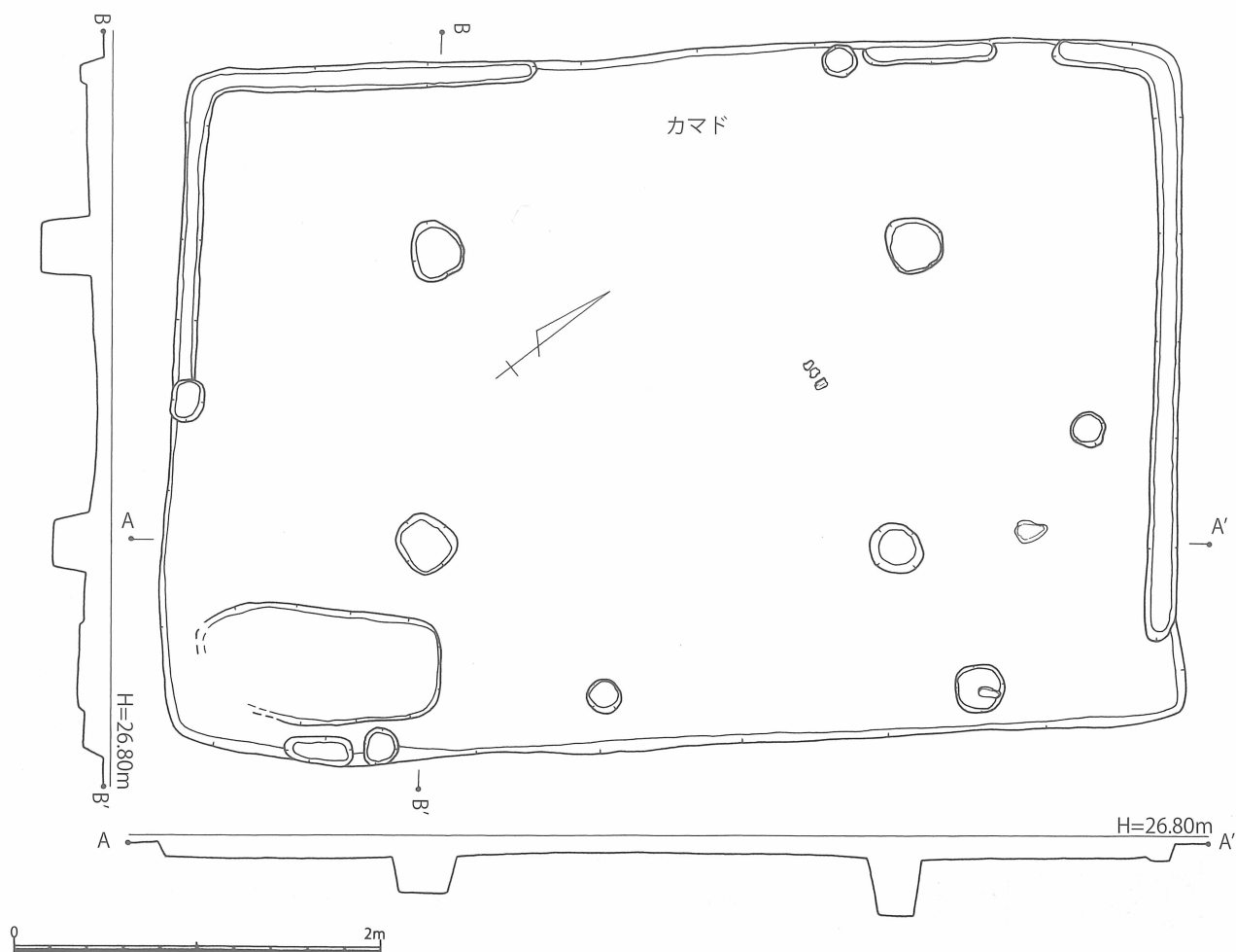
第 35 図 松/本遺跡A地点 2号竪穴住居 (SB02) 実測図 [1/40]
