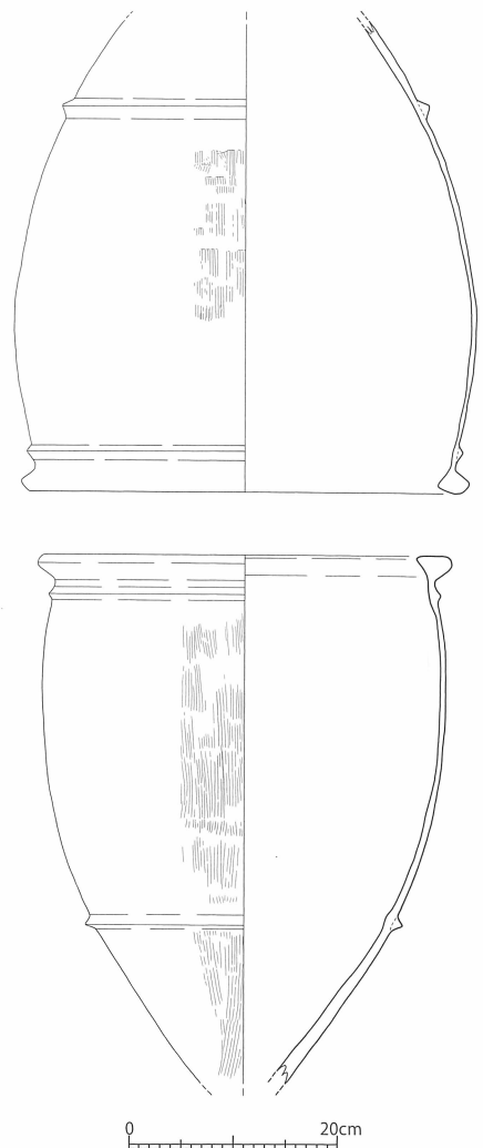
第 54 図 松ノ本遺跡B地点 4号甕棺 実測図[1/8]
