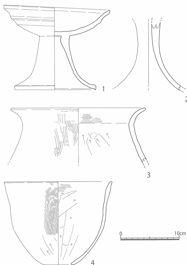
第 33 図 松ノ本遺跡A地点 1号竪穴住居 (SB01) 出土遺物実測図 [1/4]
