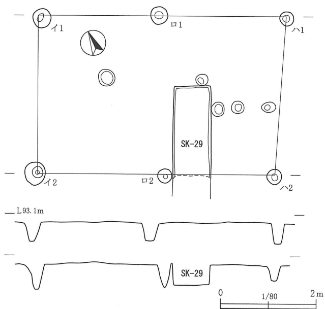
第 168 图 第 11 号掘立柱建物跡、第 29 号土坑
