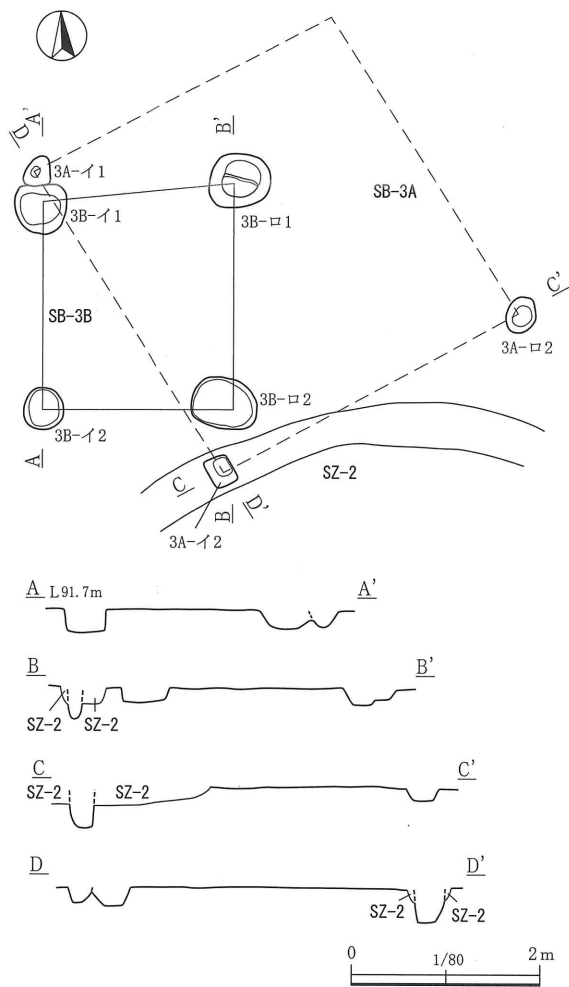
第160図 第3A・3B号掘立柱建物跡
