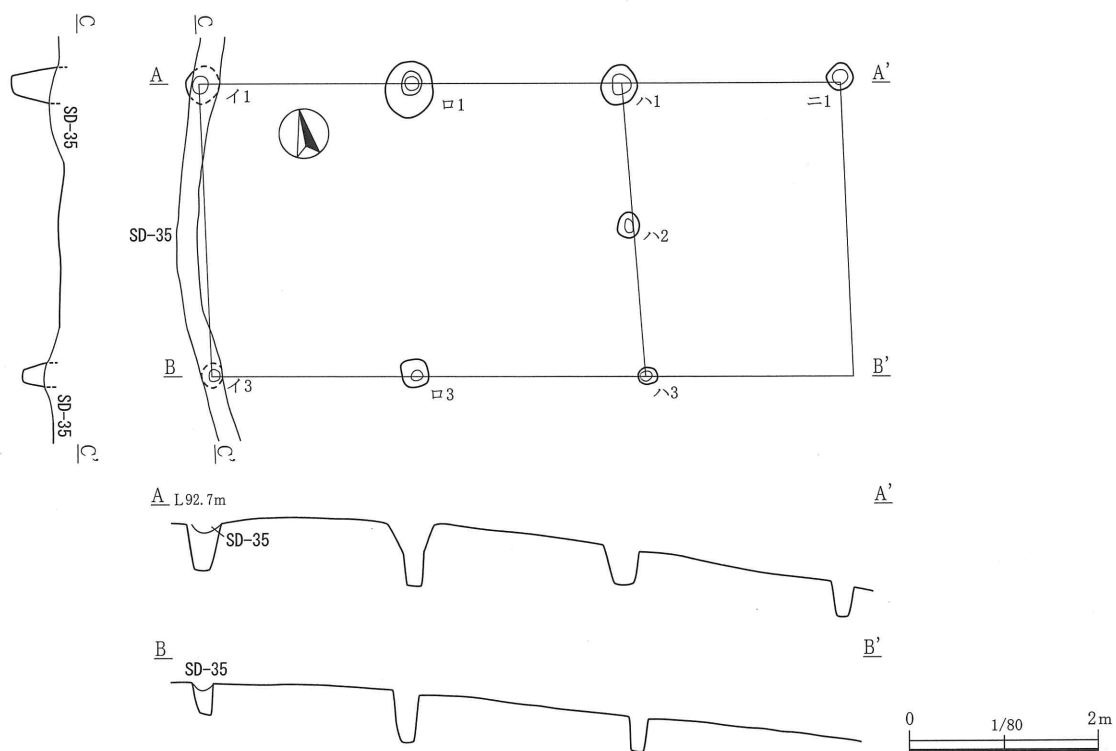
第178図 第25号掘立柱建物跡
