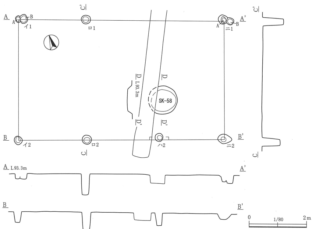
第180图 第27号掘立柱建物迹、第58号土坑
