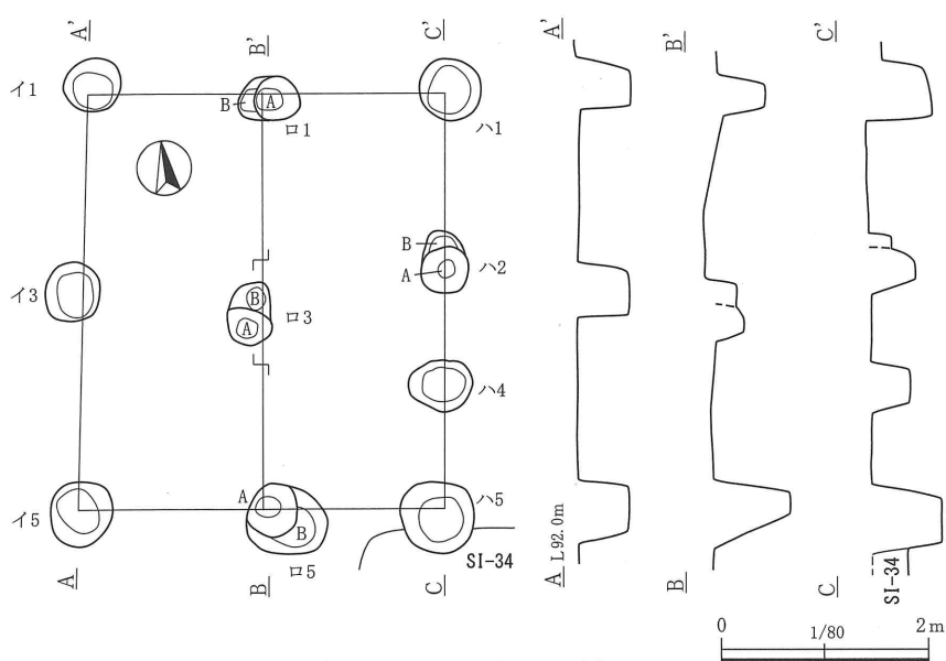
第164图 第7号掘立柱建物跡
