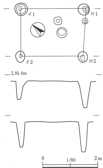
第167图 第13号掘立柱建物跡
