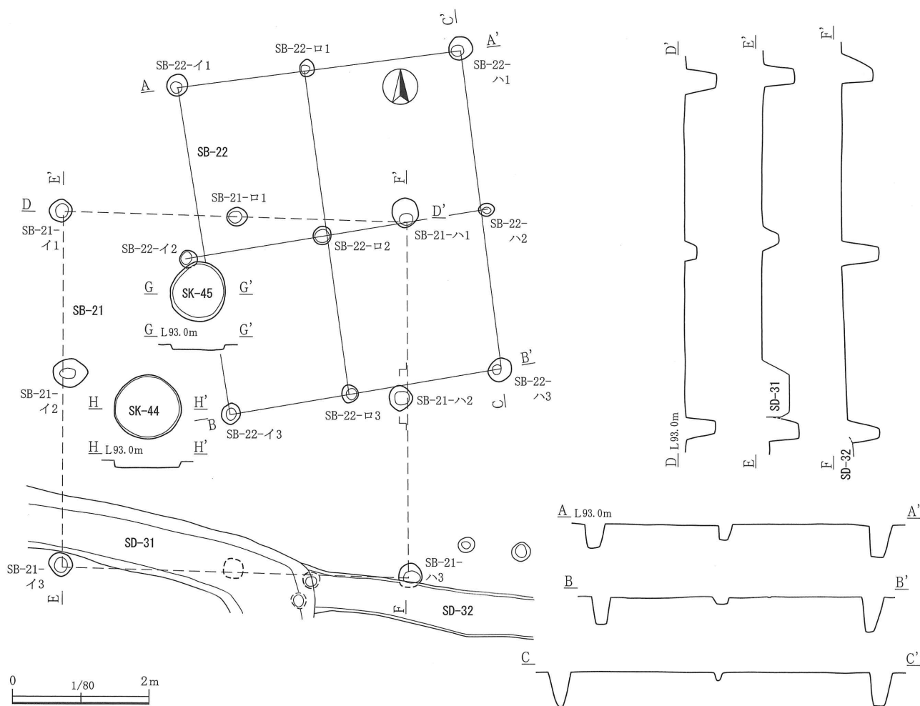
第 175 図 第 21・22 号掘立柱建物跡、第 44・45 号土坑
