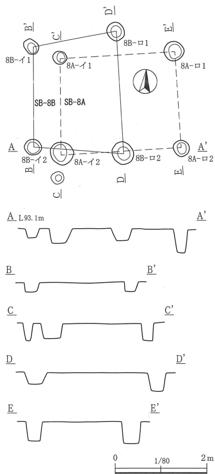
第165图 第8A・8B号掘立柱建物跡
