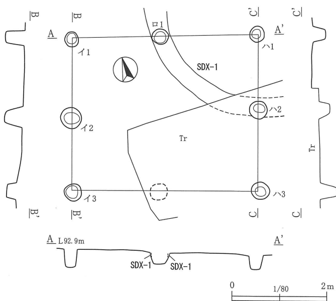
第 169 图 第 12 号掘立柱建物跡
