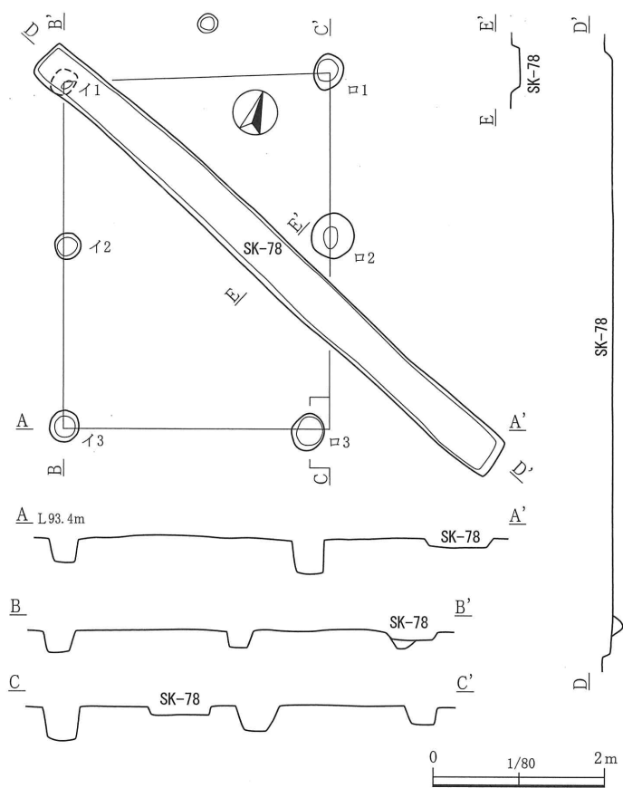
第 183 图 第 29 号掘立柱建物迹、第 78 号土坑
