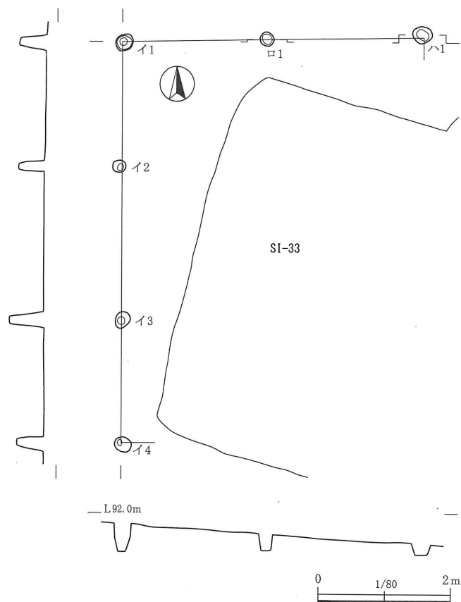
第 172 图 第 18 号掘立柱建物跡
