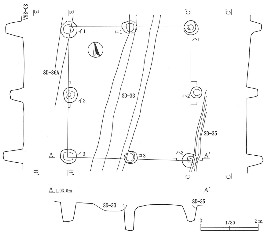
第 176 図 第 23 号掘立柱建物跡
