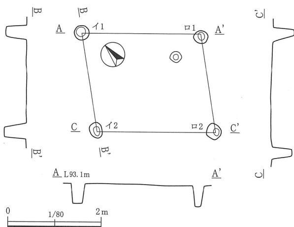
第 170 图 第 14 号掘立柱建物跡
