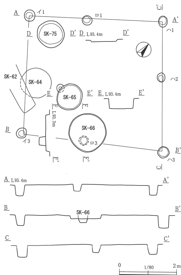
第181图 第30号掘立柱建物迹、第65·66·75号土坑
