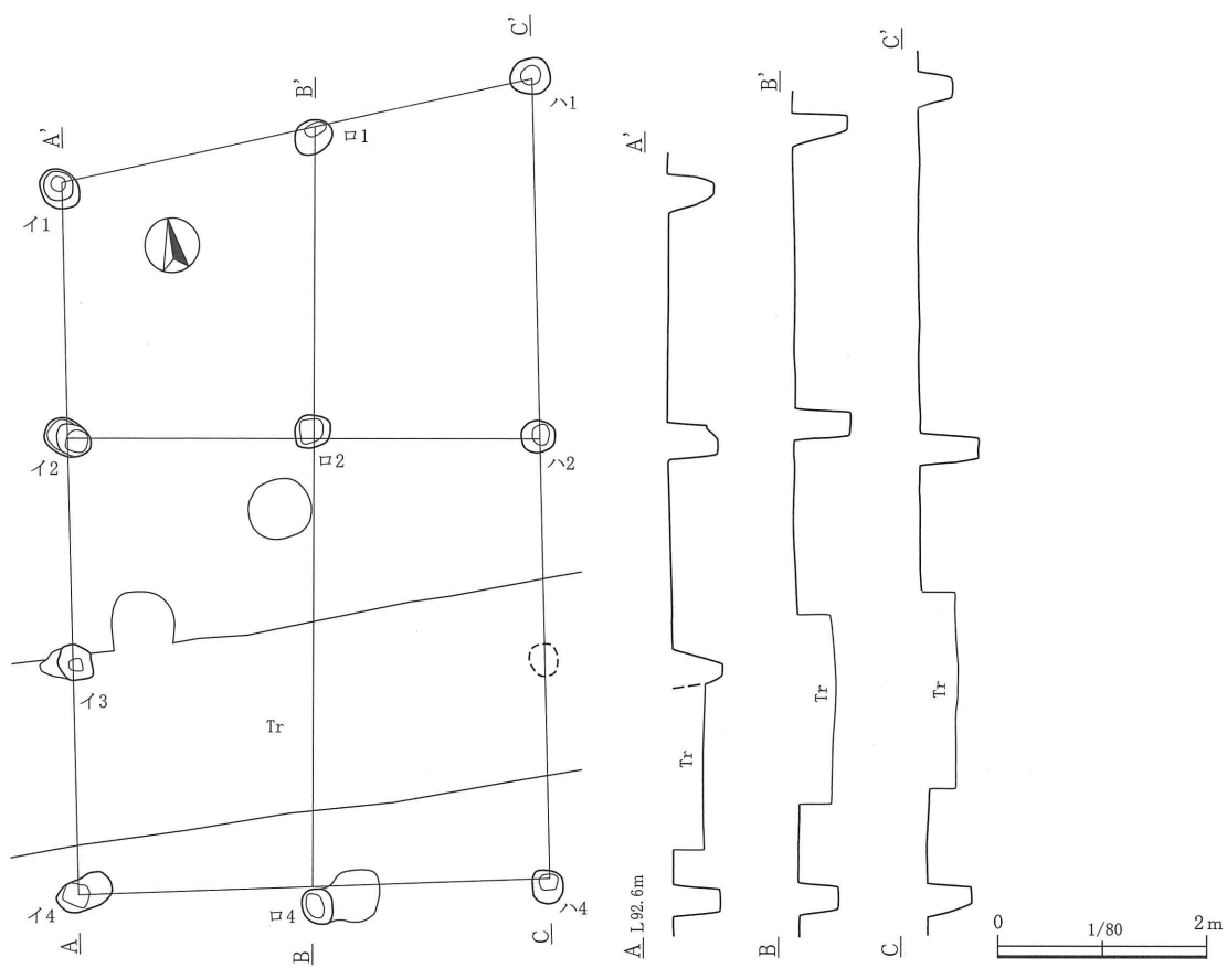
第 163 図 第 6 号掘立柱建物跡
