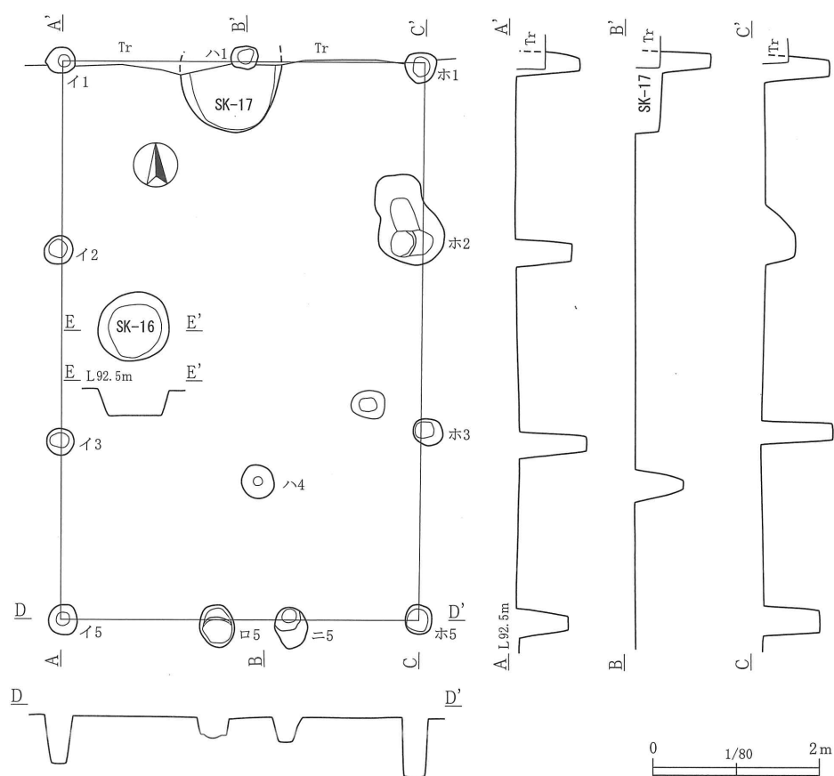
第 162 図 第 5 号掘立柱建物跡、第 16・17 号土坑
