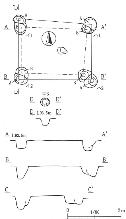
第 185 图 第 36 号掘立柱建物迹
