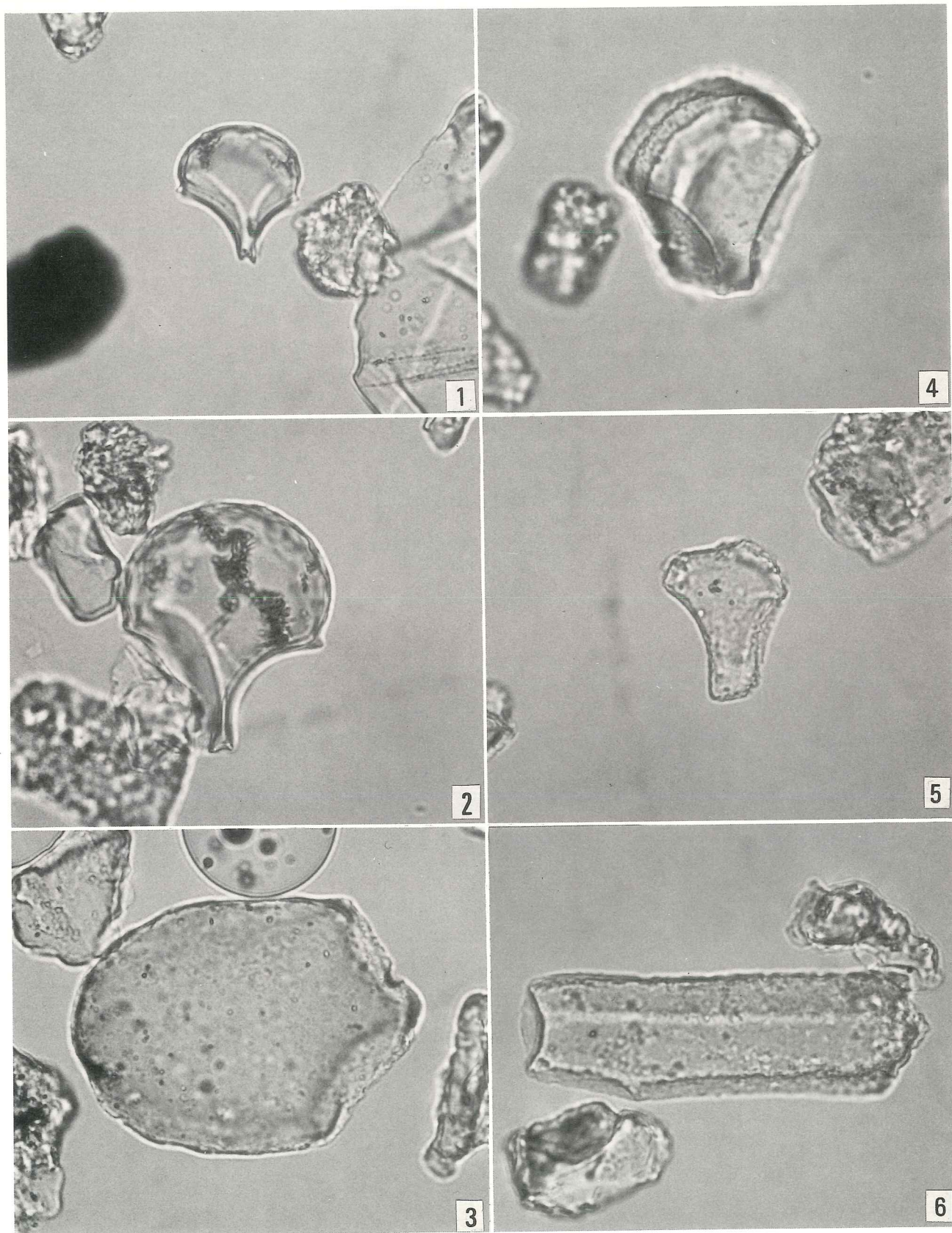
検出されたプラント・オパール顕微鏡写真 ※倍率はすべて400倍
