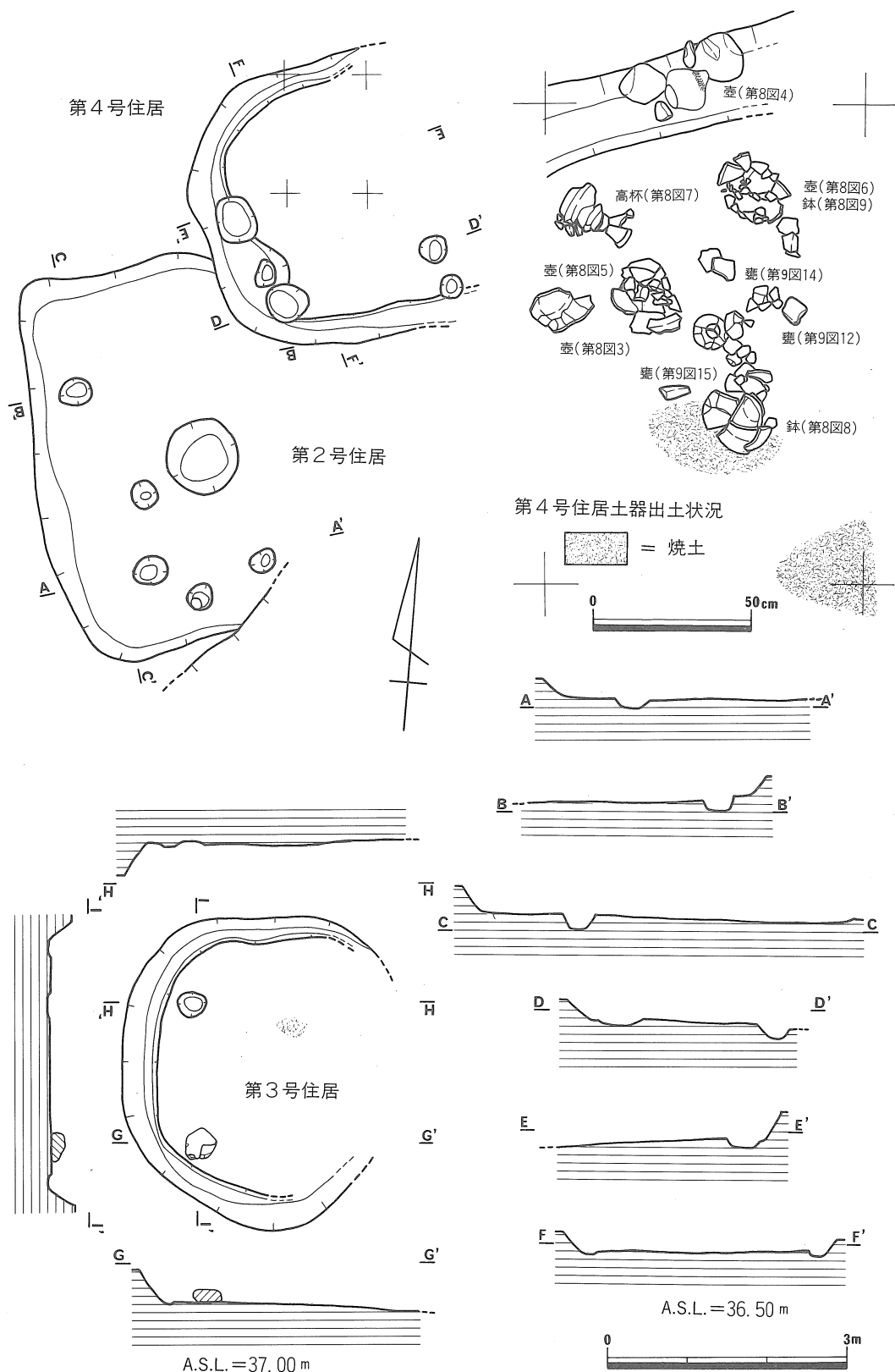
第4図 第2～4号住居実測図
