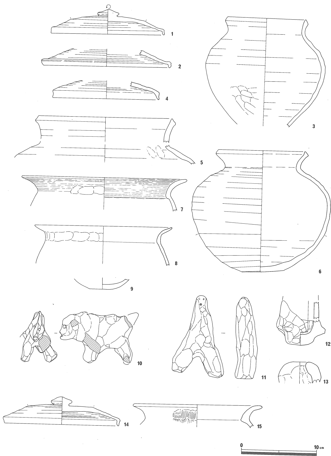
第12図 遺物実測図(4)
