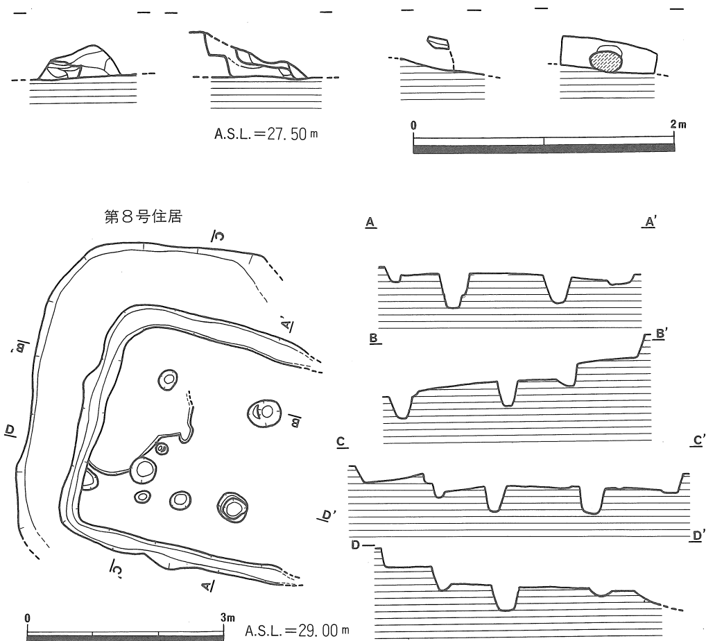
第5图 第6~8号住居实测图
