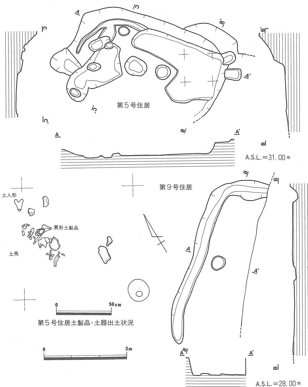
第6図 第5・9号住居実測図
