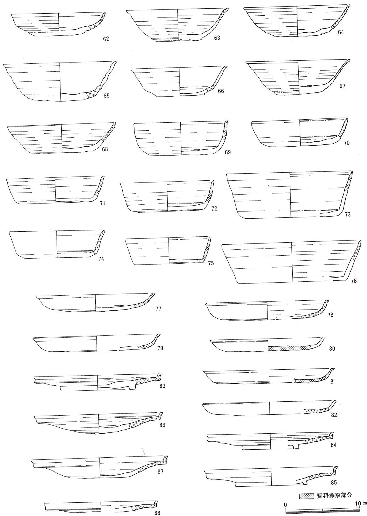
第3図 胎土分析資料土器実測図(3)
