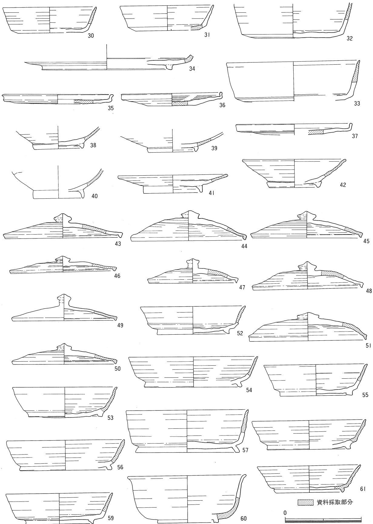
第2図 胎土分析資料土器実測図(2)
