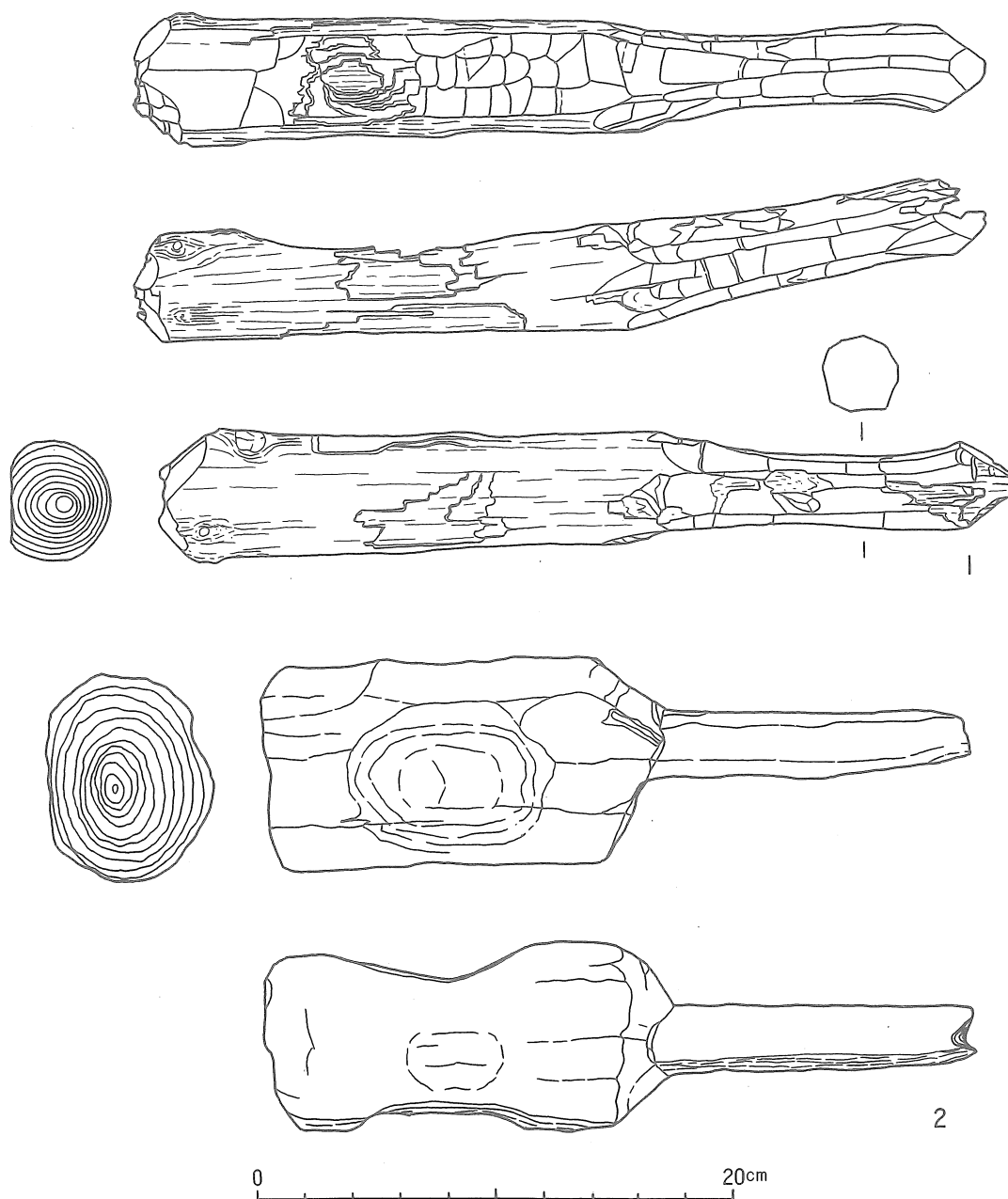
第10図 ヨコヅチ実測図
