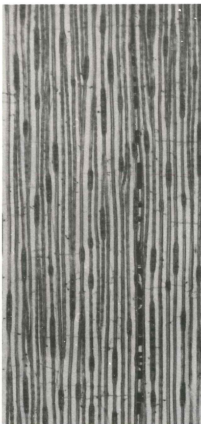
接線断面 75×
