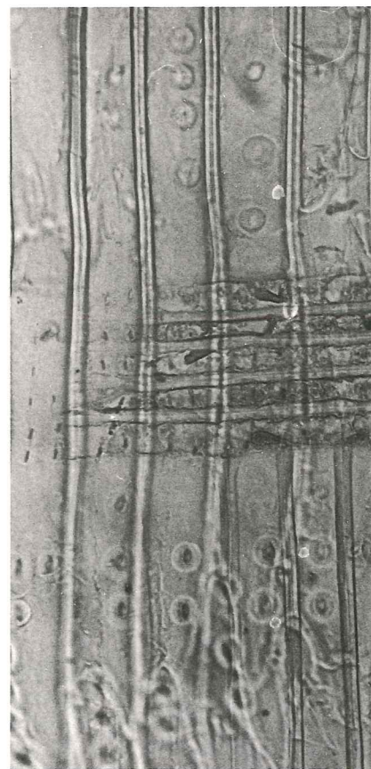
放射断面 375×
