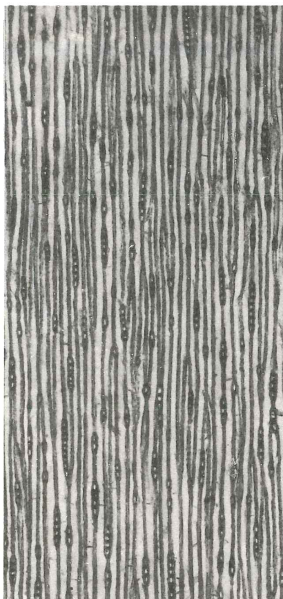
接線断面 75×
