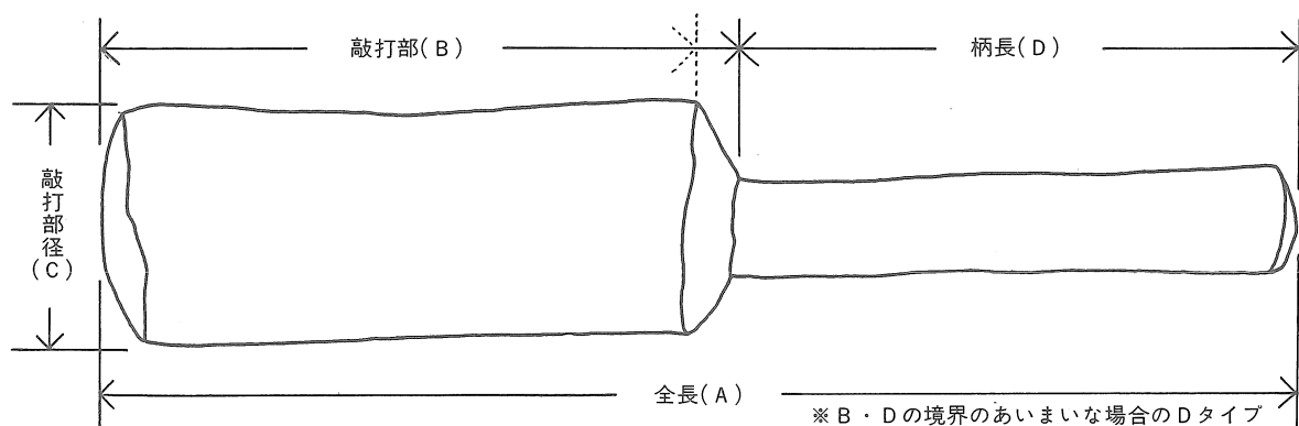
第7図 ヨコヅチの計測部位
