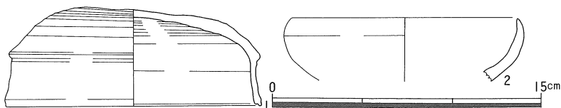
第5図 SD 1 出土土器実測図
