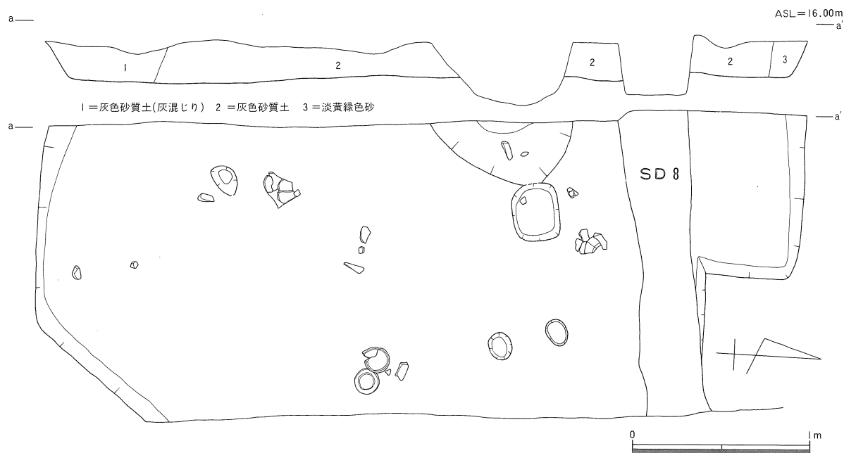
第12図 SI 1 実測図
