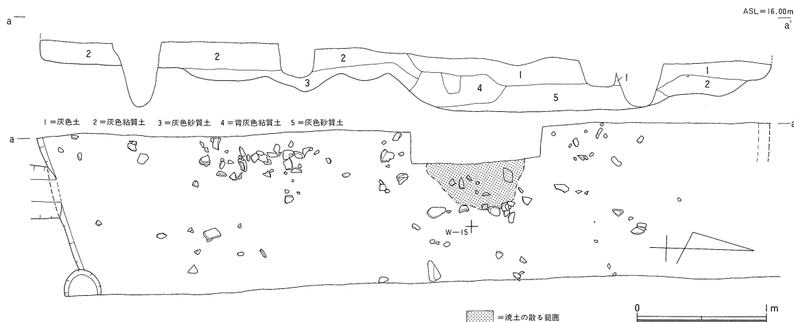
第24図 SI 8 実測図
