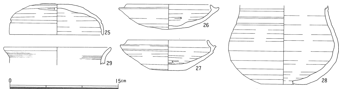
第13図 S I 1 出土土器実測図
