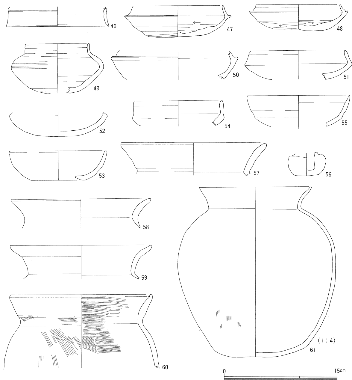
第18図 S I 5 出土土器実測図
