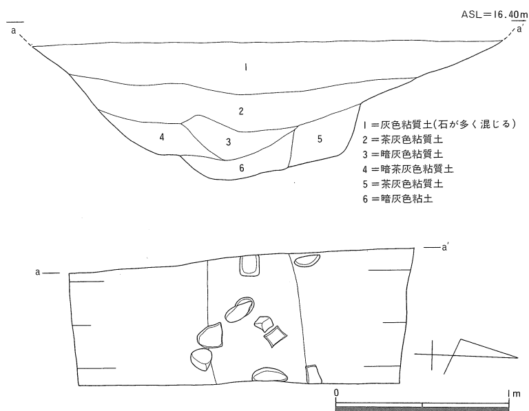
第28図 S D11実測図および出土土器実測図
