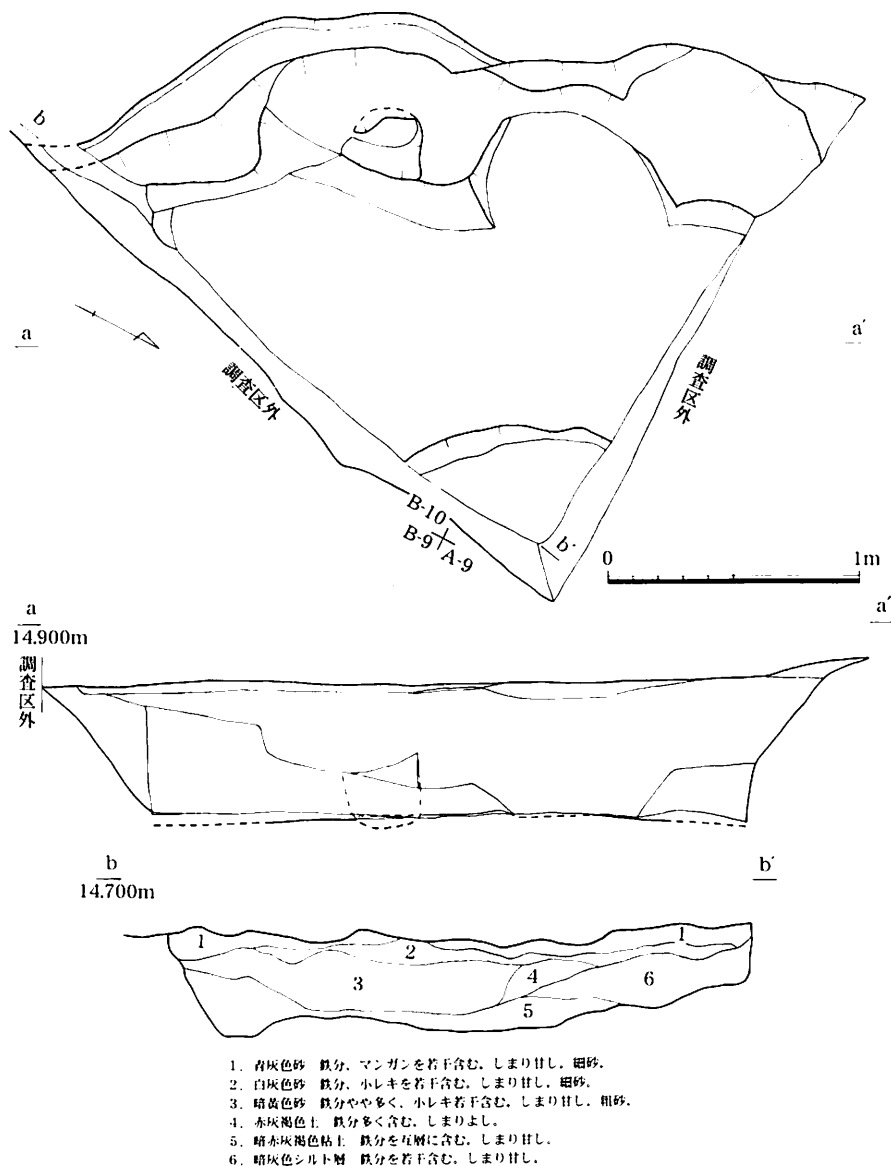
第111図 第1号溝状遺構平・断面図(1/30)
