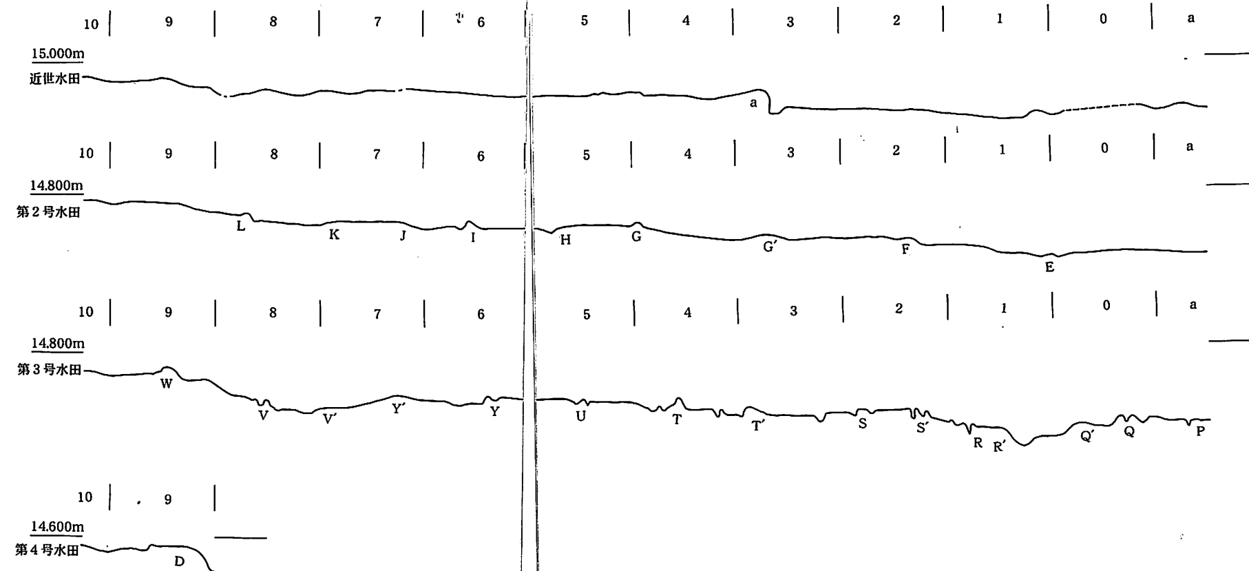
第129図 IIb区の水田の垂直的変遷(1/200, 断面1/40)
