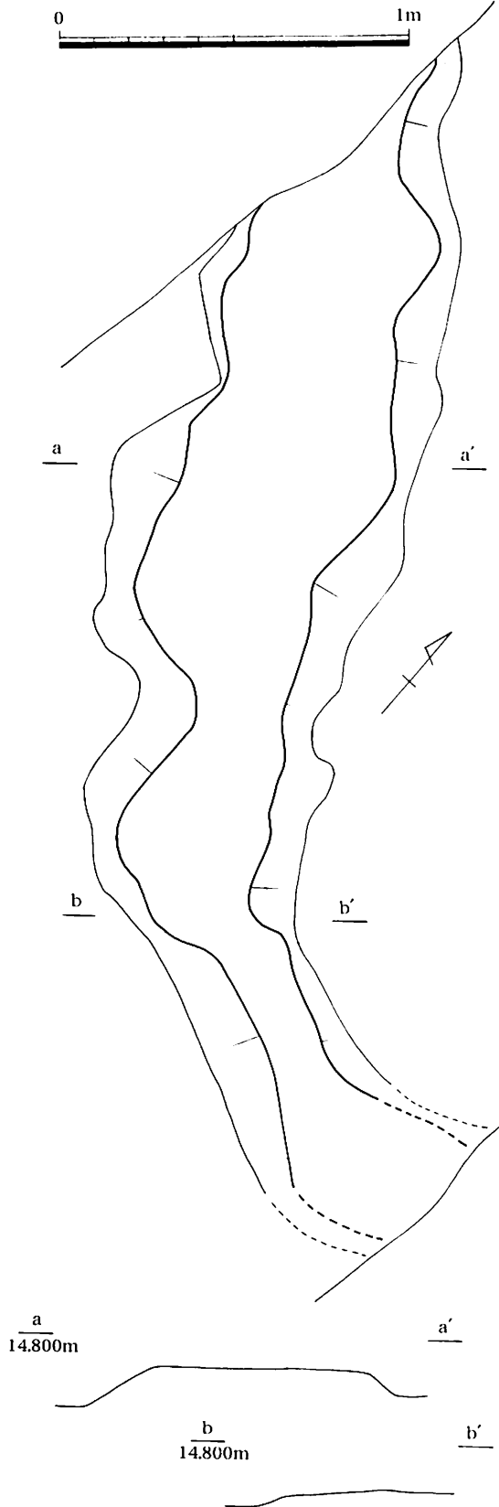
第81図 第3号水田A畦畔平・断面図(1/20)
