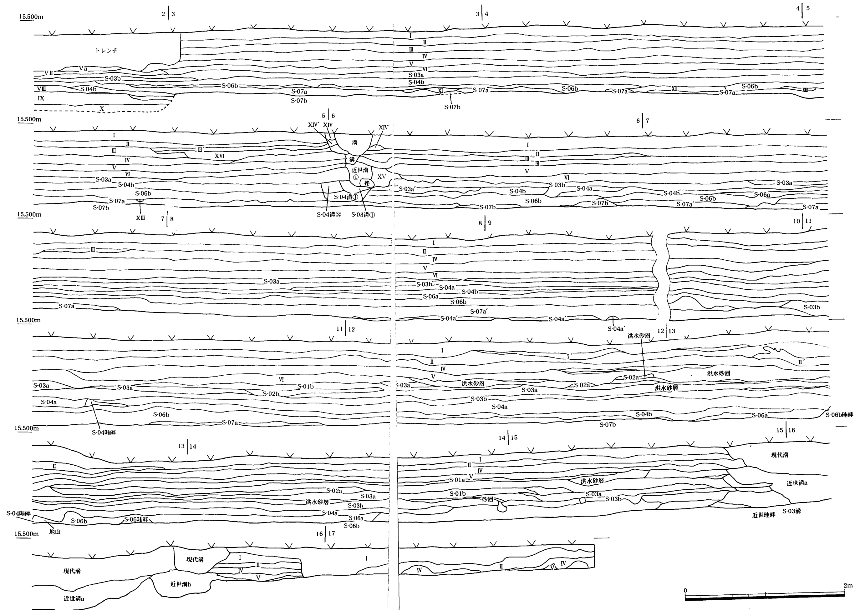
調査区北壁土層断面図(1/30)
