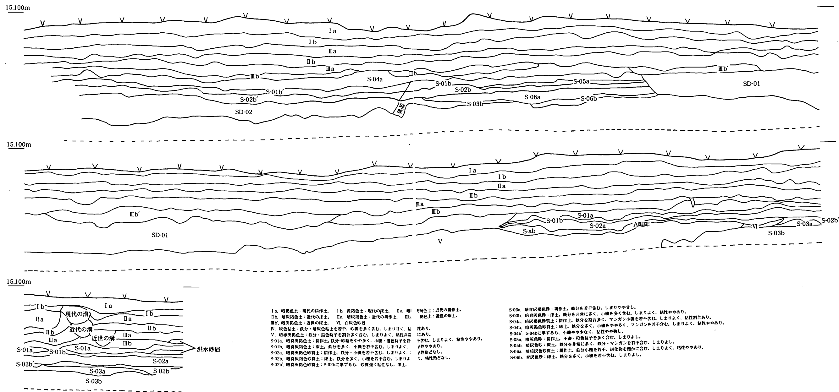
第61図 第I調査区 南壁土層断面図(1/30)
