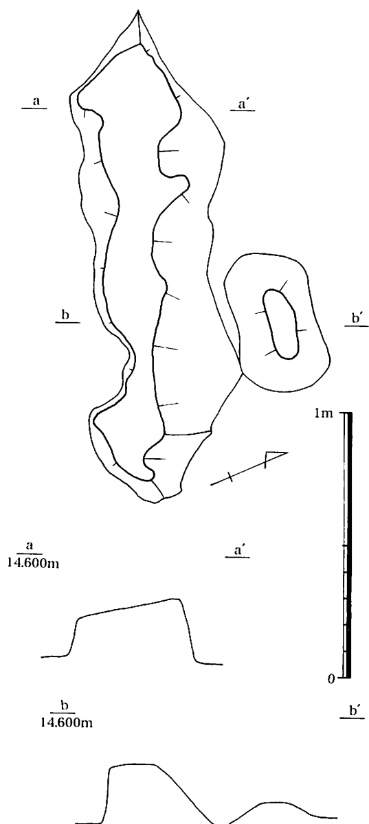
第115図 第4号水田C畦畔平・断面図 (1/20)
