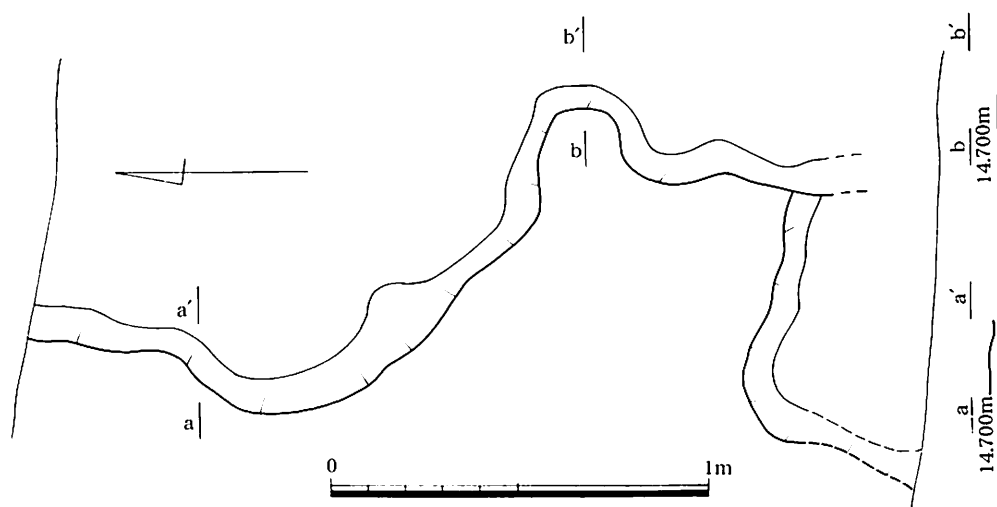
第119図 第4号水田H畦畔平・断面図(1/20)
