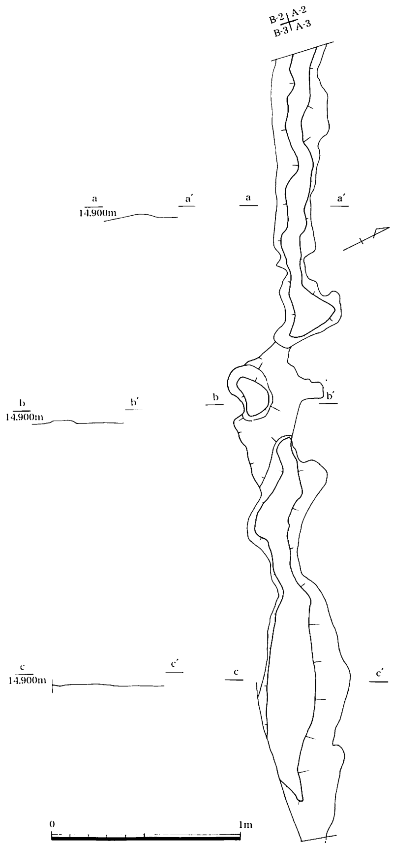
第11図 第3号水田A畦畔平・断面図 (1/20)
