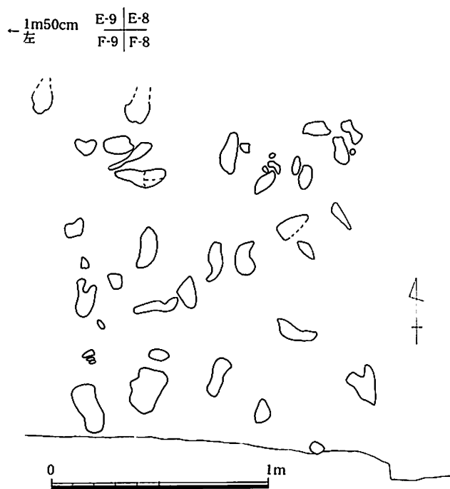
第107図 第3号水田直下牛・人の足跡平面図②(1/25)
