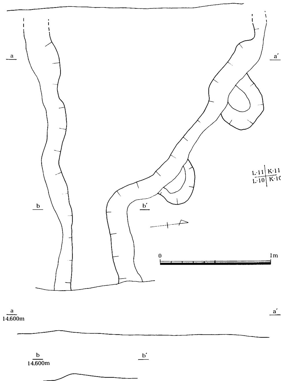
第87図 第3号水田G畦畔平・断面図(1/20)
