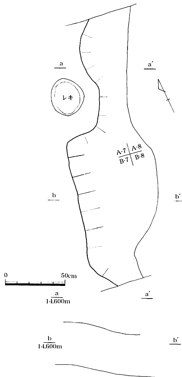
第29図 第6号水田D畦畔平・断面図 (1/20)
