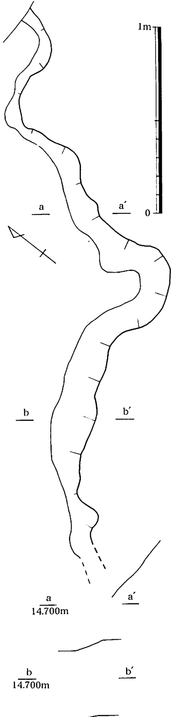
第101図 第 3 号水田Y畦畔平・断面図(1/20)
