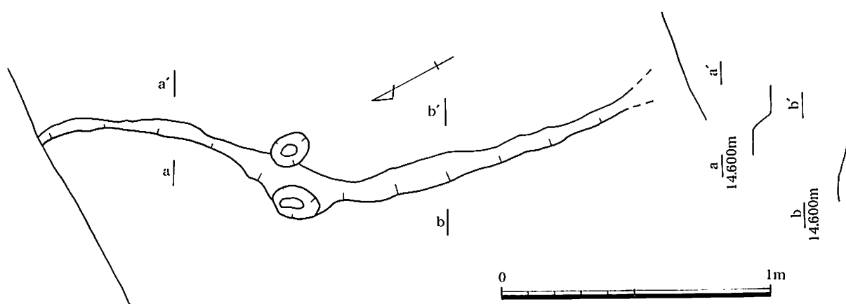
第99図 第3号水田U畦畔平・断面図(1/20)
