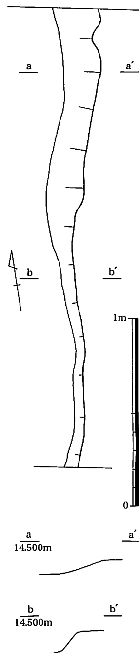
第41图 第7号水田C畦畔平·断面图(1/20)
