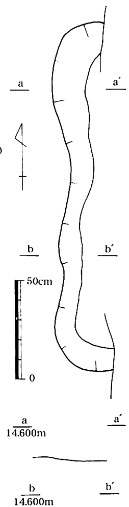
第88図 第3号水田H畦畔平・断面図(1/20)
