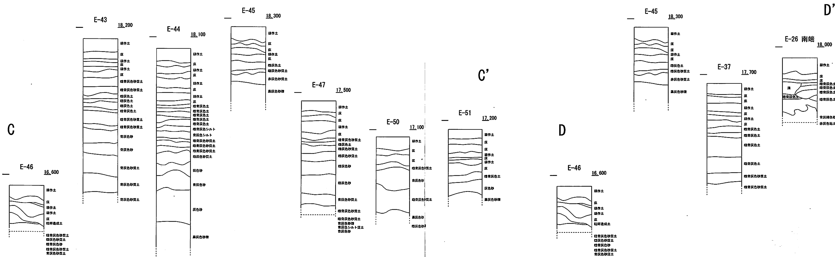
第138图 C-C' 土層断面柱状图
