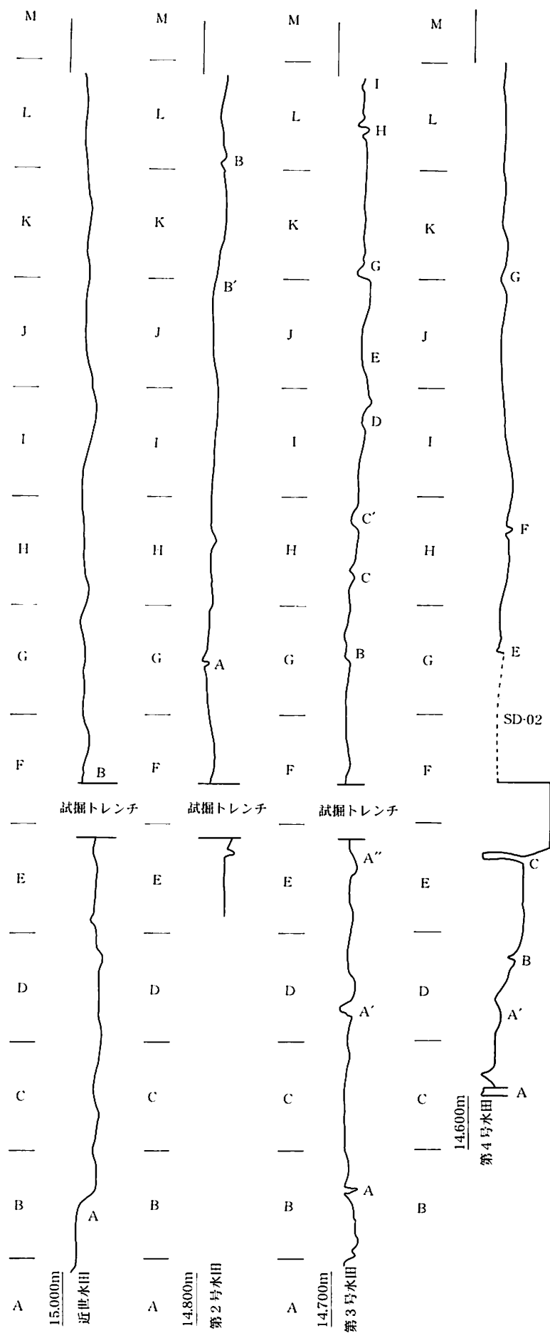
第127図 第Ⅱ調査区の水田の垂直的変遷(1/200, 断面1/40)
