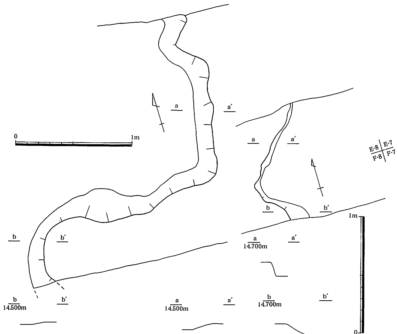
第102図 第3号水田S畦畔平・断面図(1/20)
