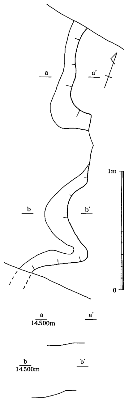
第97図 第3号水田R畦畔平・断面図(1/20)
