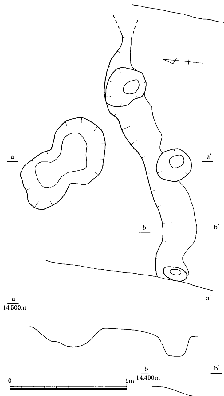
第116図 第4号水田B畦畔平・断面図(1/20)
