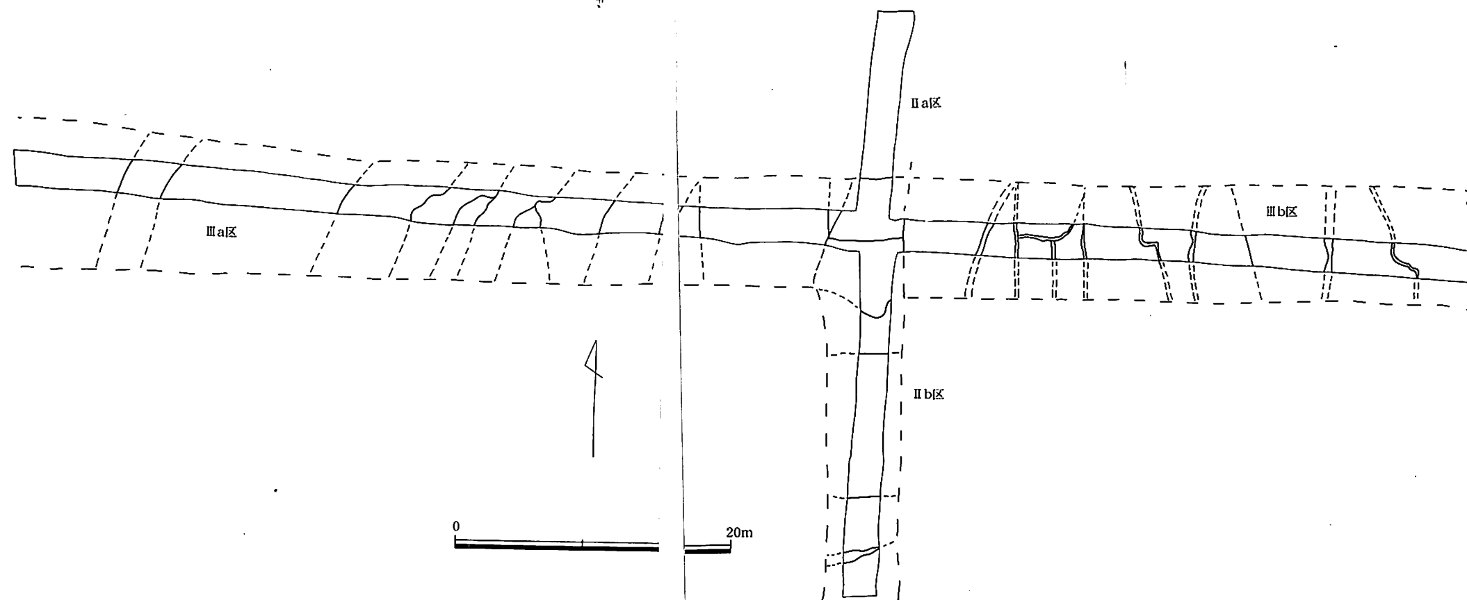
第132図 第4号水田の平面形の復原(1/400)
