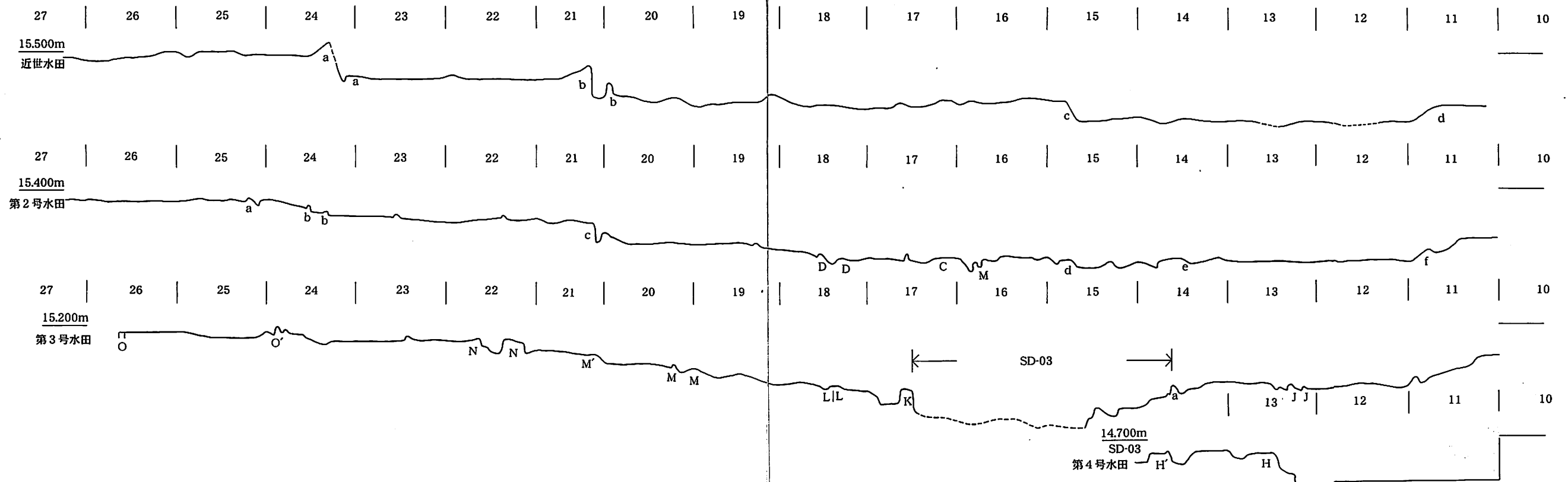
第128図 IIIa区の水田の垂直的変遷(1/200, 断面1/40)
