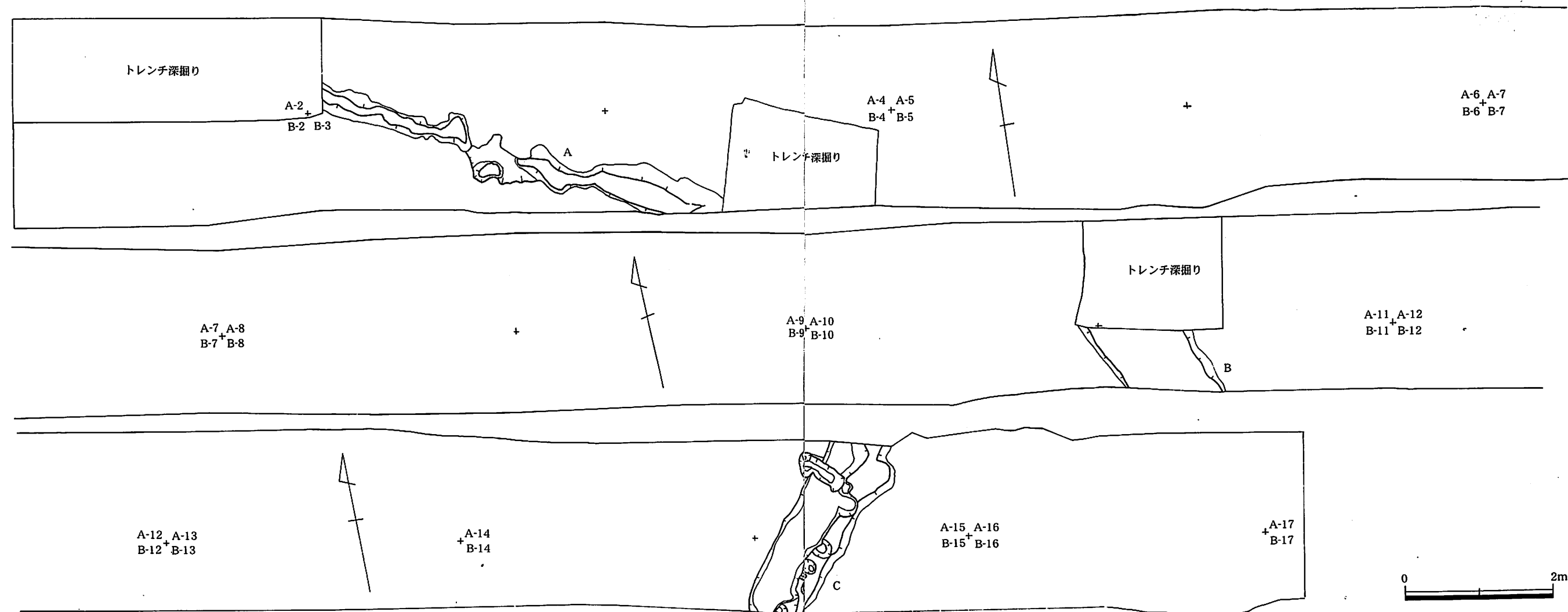
第10図 第3号水田平面図(1/60)
