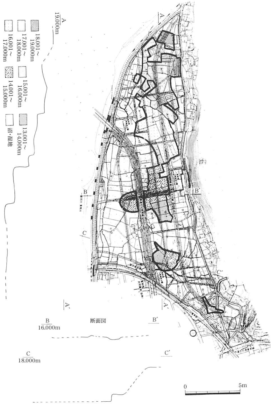
第143図 中世水田の範囲と水田上面の標高(平面図1/8000、断面図1/200)
