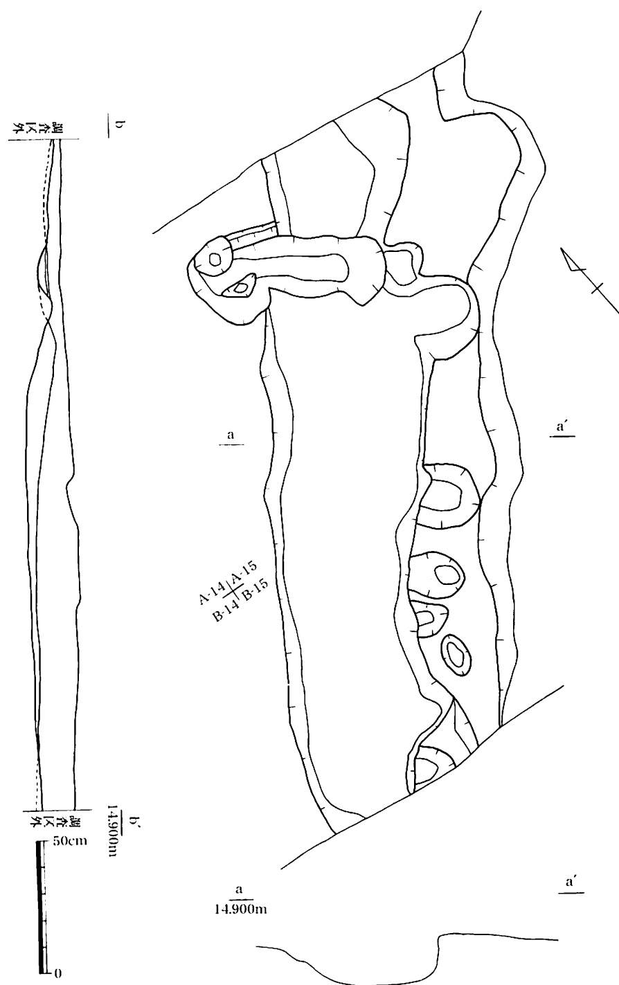
第14図 第3号水田C畦畔平・断面図(1/20)
