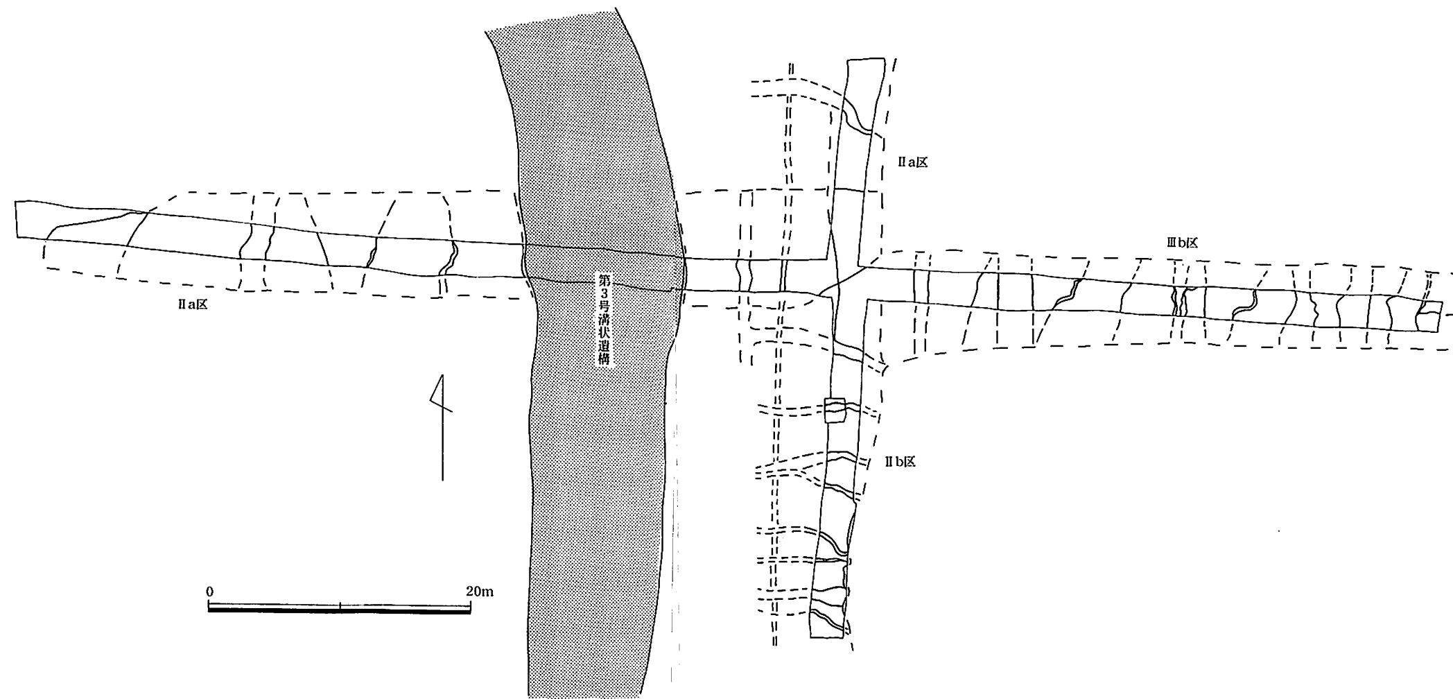
第131図 第3号水田の平面形の復原(1/400)
