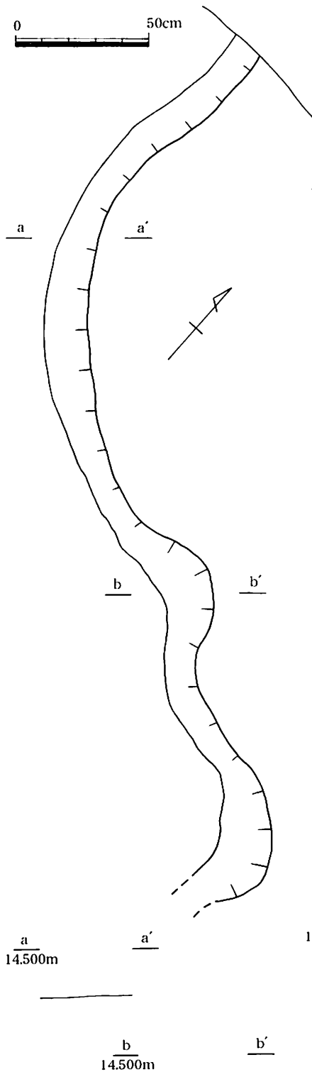
第71図 第2号水田E畦畔平・断面図 (1/20)
