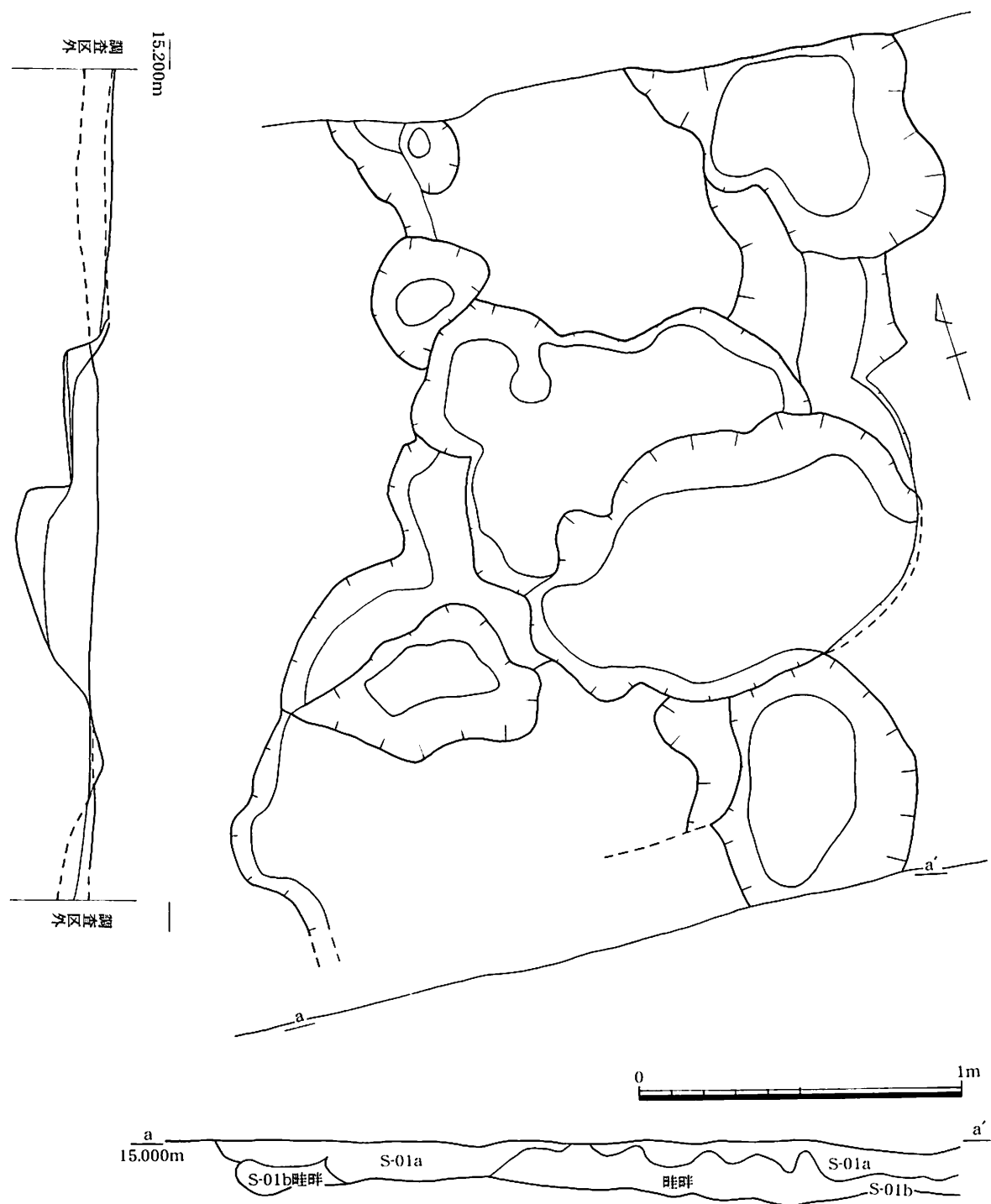
第95図 第3号水田N畦畔平・断面図(1/20)
