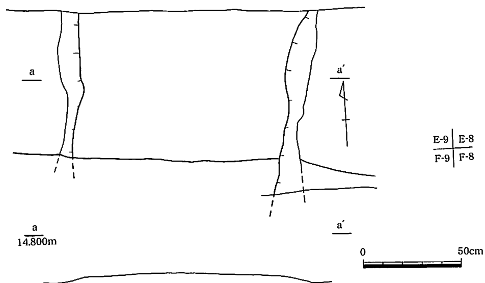
第104図 第3号水田W畦畔平・断面図(1/20)
