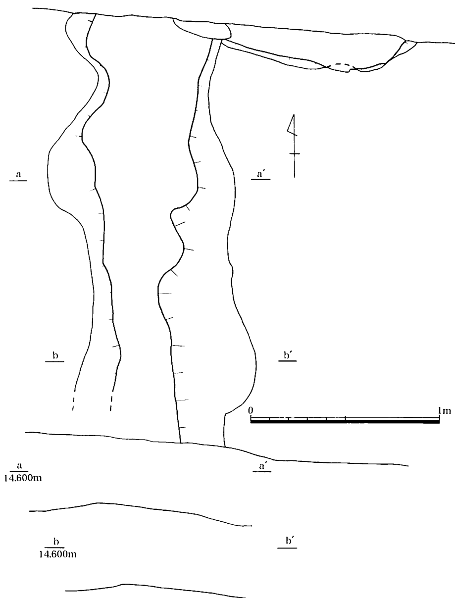
第105図 第3号水田T畦畔平・断面図(1/20)
