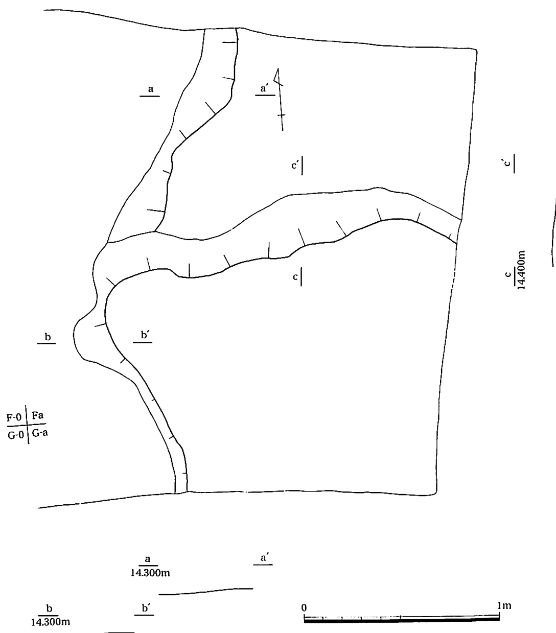
第98図 第3号水田P畦畔平・断面図(1/20)
