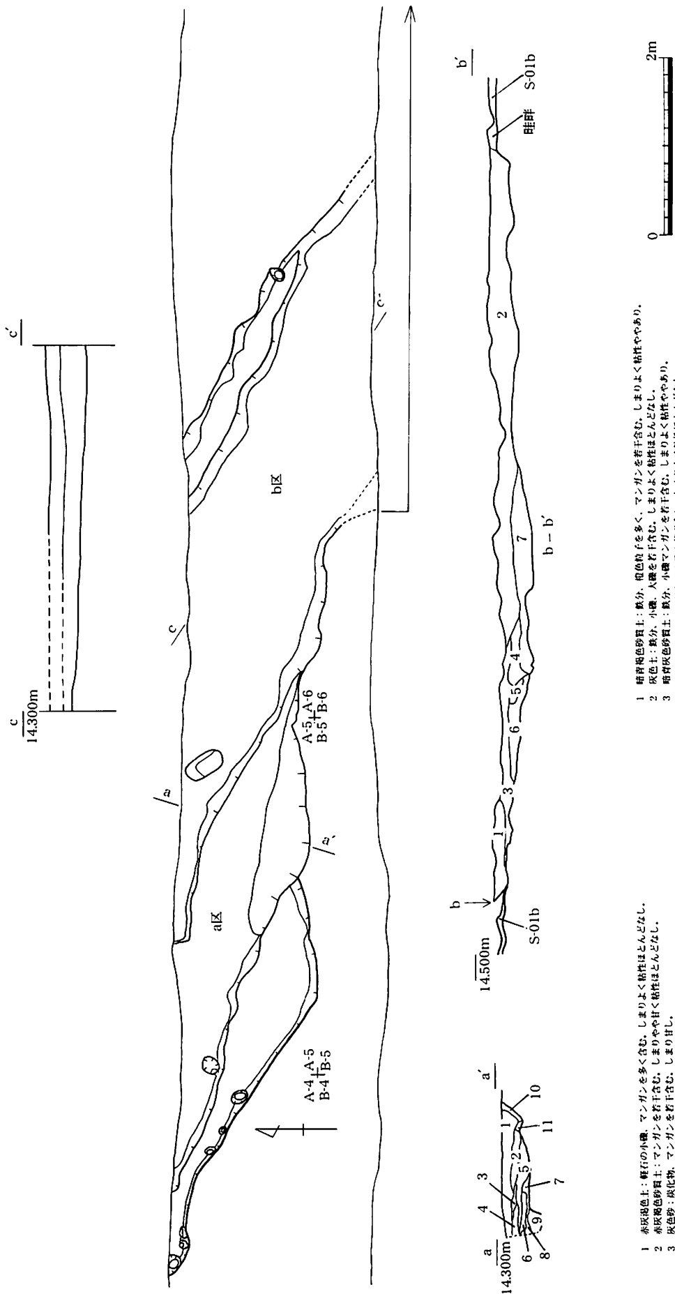
第54図 第1号溝状遺構平・断面図 (1/30)
