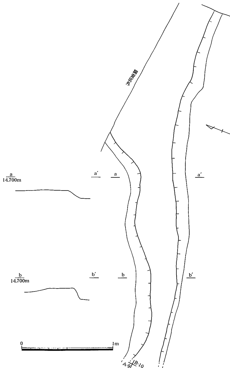
第24図 第4号水田E畦畔平・断面図(1/20)
