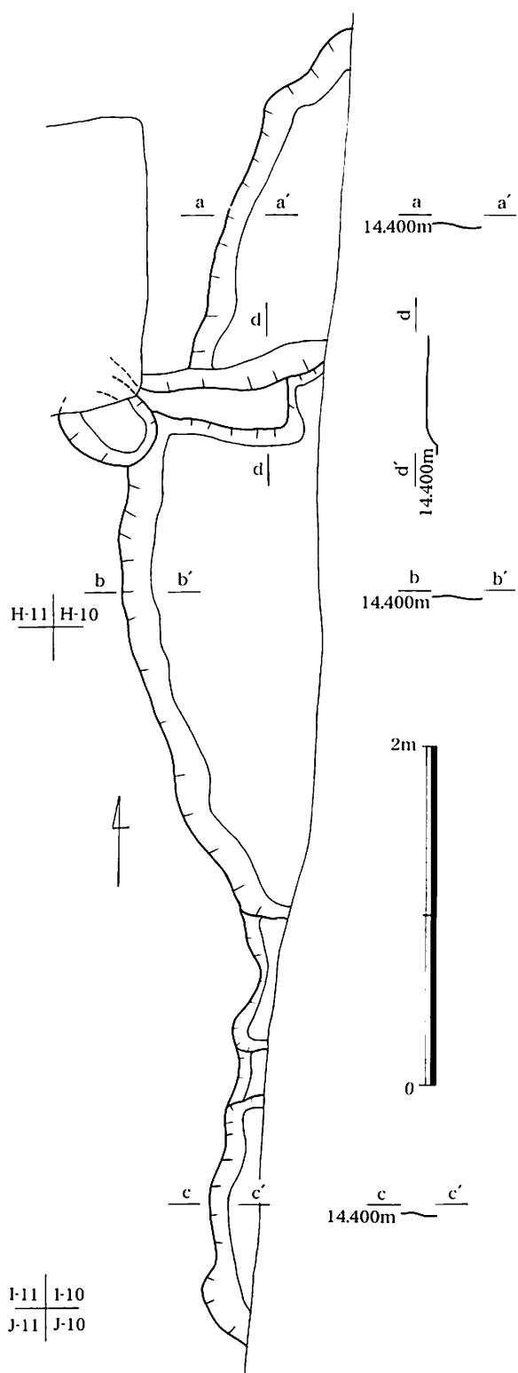
第120図 第4号水田F畦畔平・断面図(1/40)
