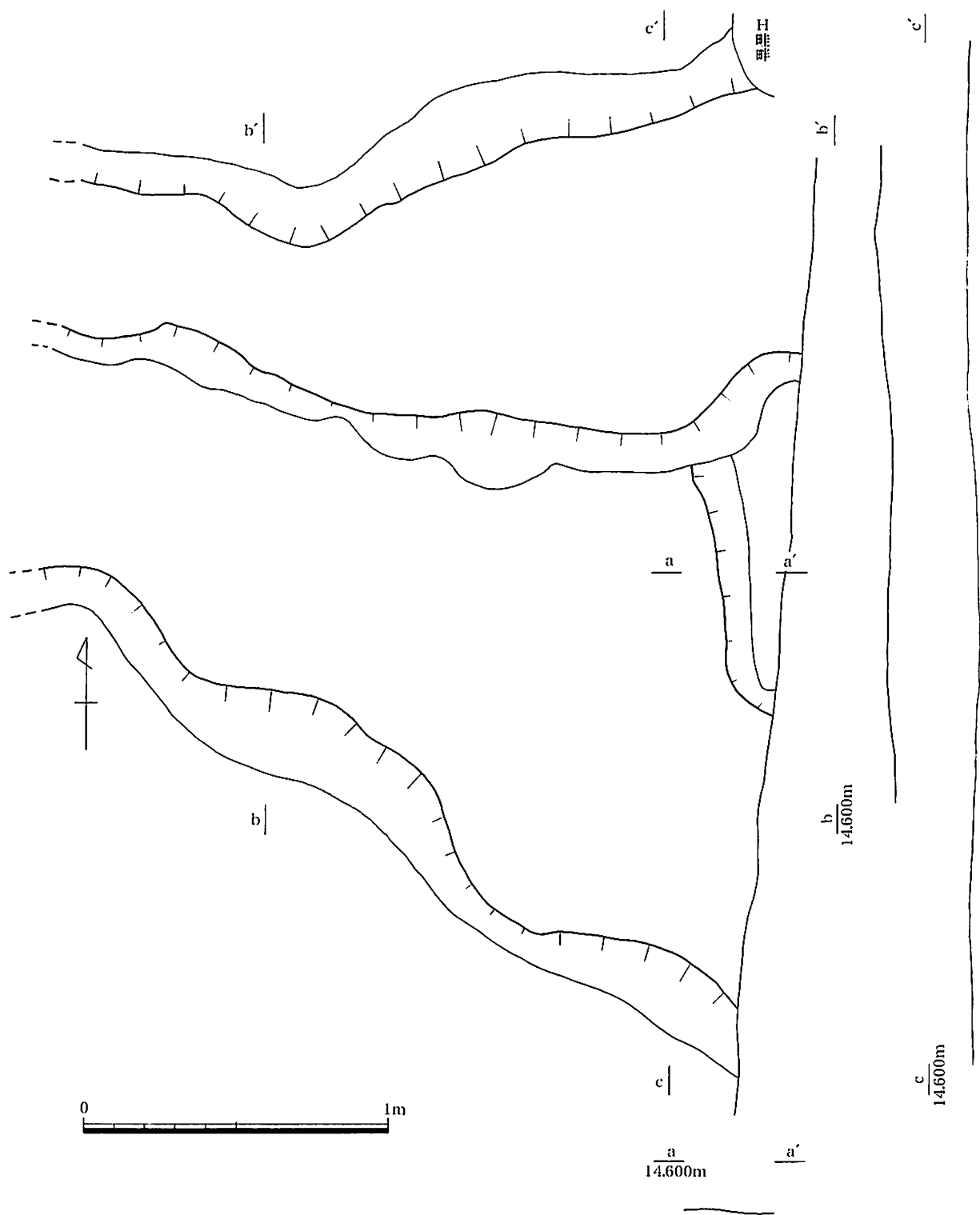
第89図 第3号水田 I 畦畔平・断面図 (1/20)
