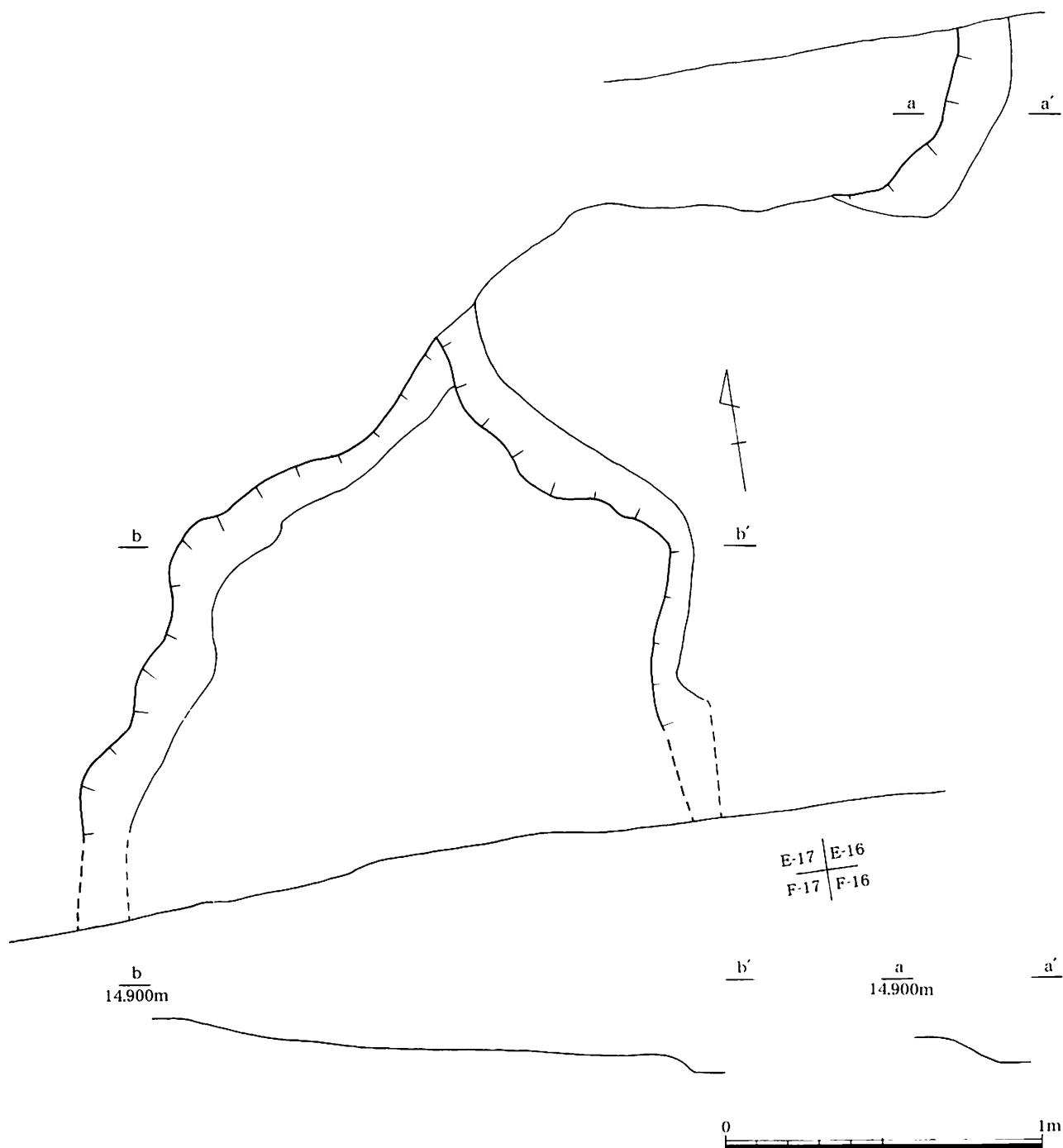
第68図 第2号水田M畦畔平・断面図(1/20)
