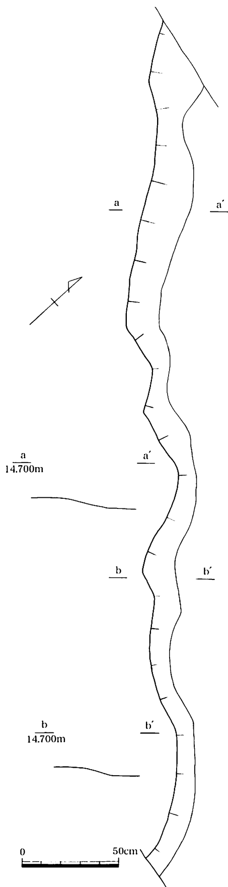
第28図 第6号水田C畦畔平・断面図 (1/20)
