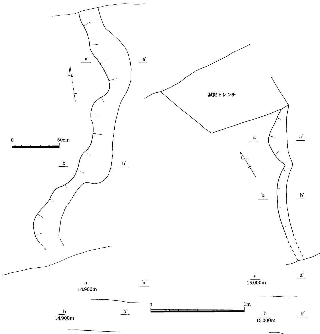
第93図 第3号水田L畦畔平・断面図(1/20)
