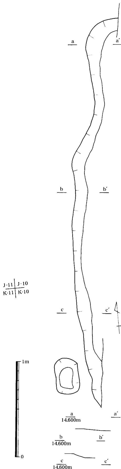
第86図 第3号水田F畦畔平・断面図 (1/20)
