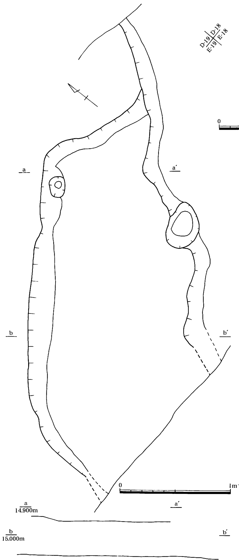
第69図 第2号水田C畦畔平・断面図(1/20)
