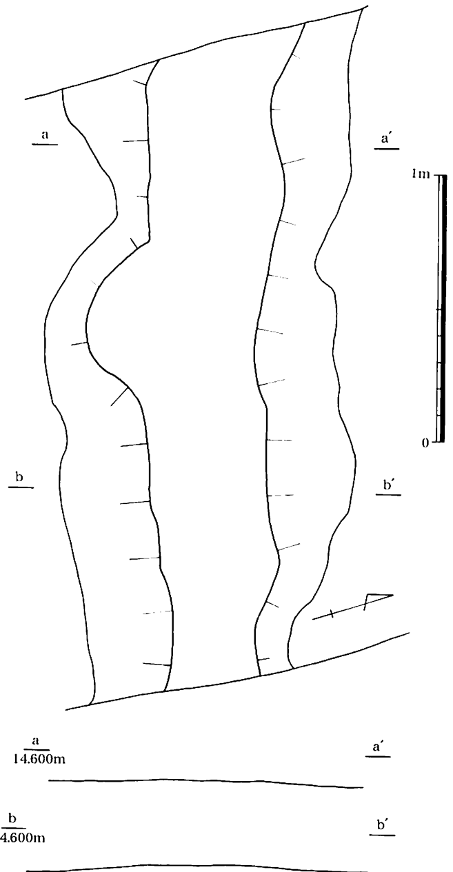
第82図 第3号水田B畦畔平・断面図(1/20)
