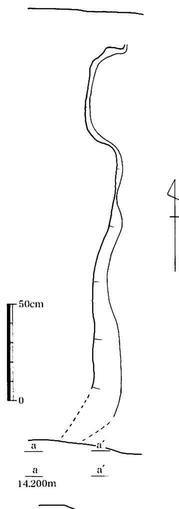
第59-2図 第3号水田A畦畔平・断面図(1/20)
