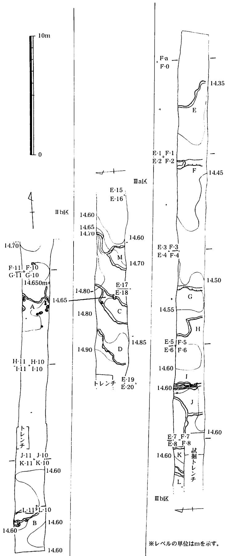
第65図 第Ⅱ・Ⅲ調査区第2号水田面遺構配置図 (1/200)
