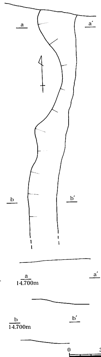
第73図 第2号水田G畦畔平・断面図 (1/20)
