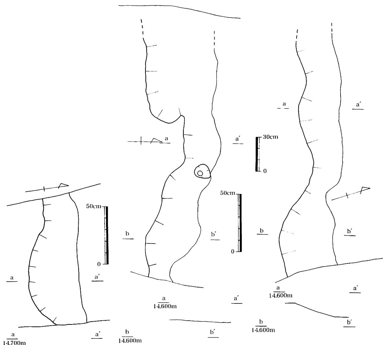
第83図 第3号水田C畦畔 平・断面図(1/20)
