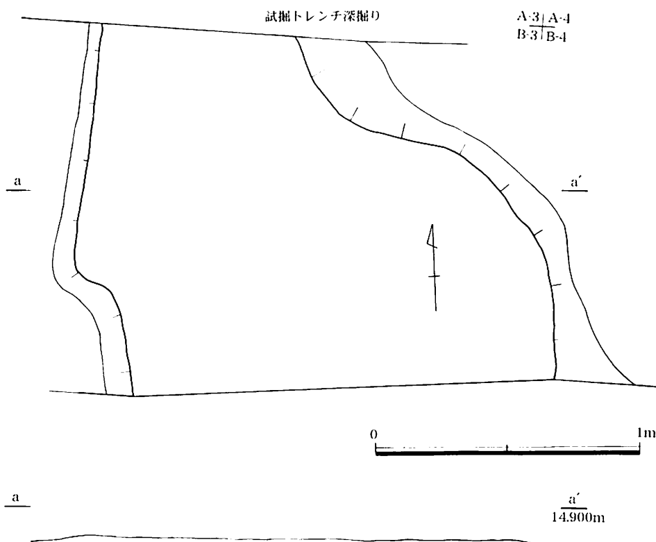
第20図 第4号水田A畦畔平・断面図(1/20)
