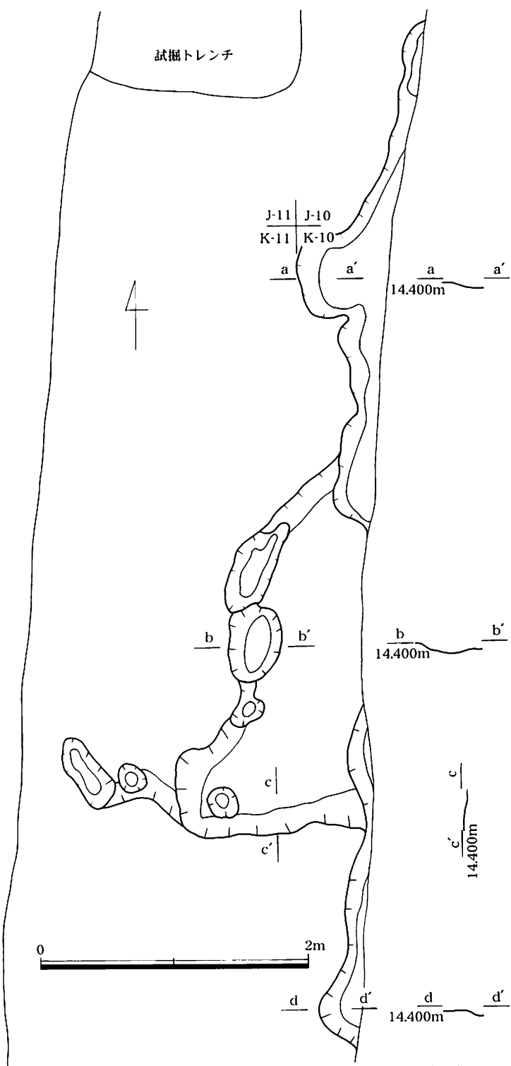
第121図 第4号水田G畦畔平・断面図(1/40)
