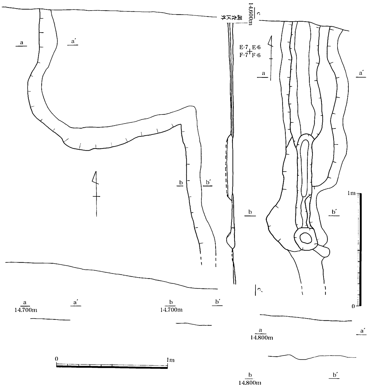
第74図 第2号水田H畦畔平・断面図(1/20)
