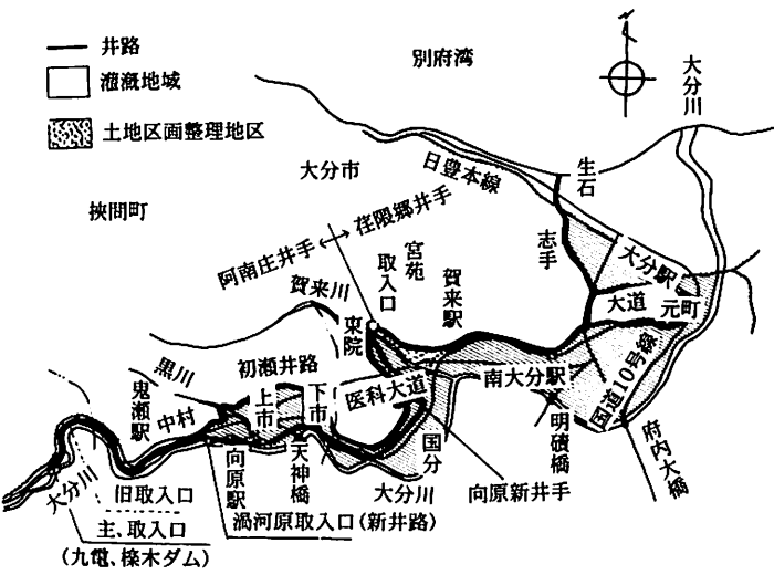
第146図 初瀬井路の水路現況模式図(秦1987文献第15図一部改)
