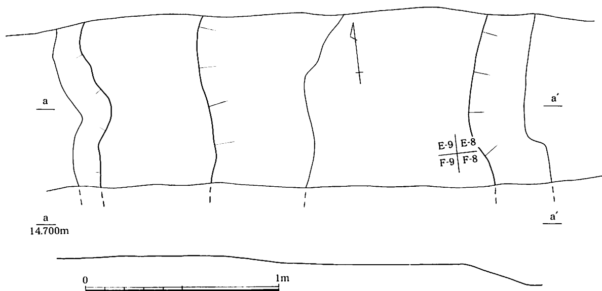
第118図 第4号水田D畦畔平・断面図(1/20)
