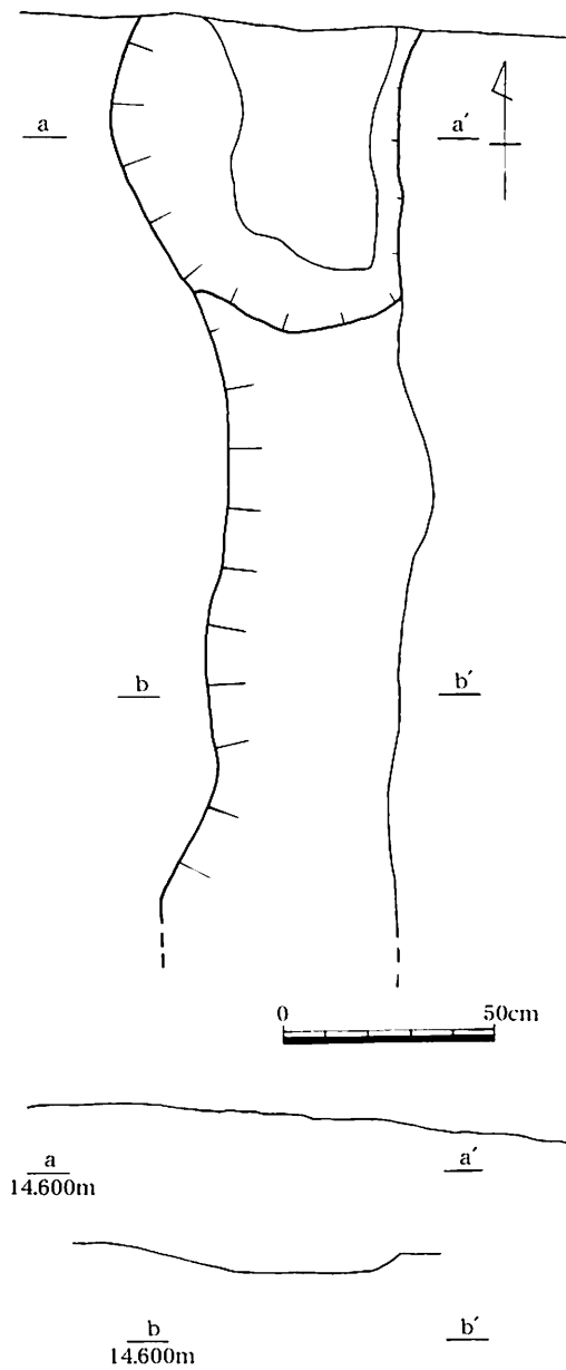
第72図 第2号水田F畦畔平・断面図 (1/20)
