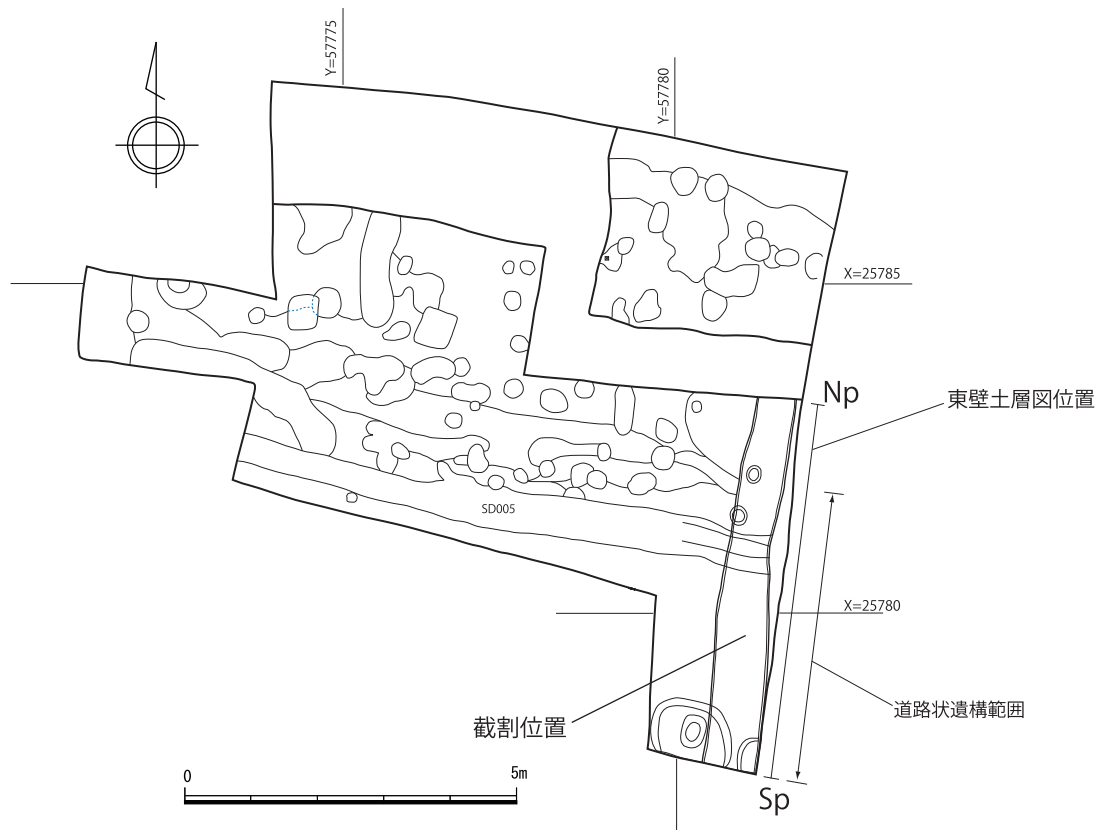
第11図 遺構配置図 (1/100)
