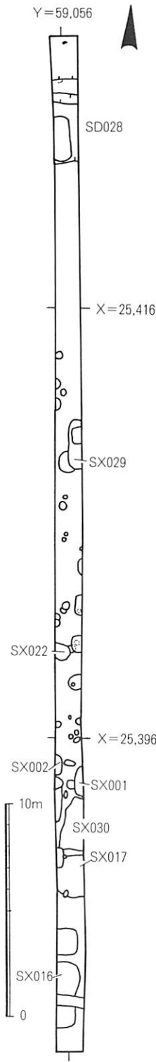
第40図 遺構配置図(1/250)
