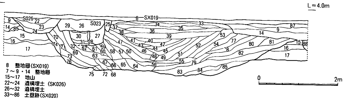
第105図 土塁跡 (SX020) 土層図 (1/60)
