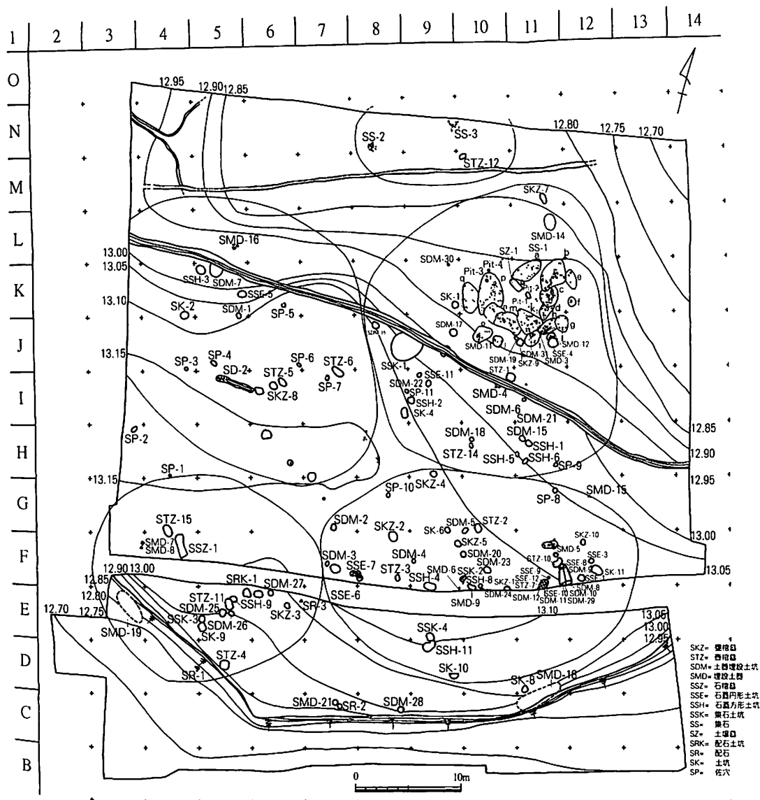
第150図 Ⅲ調査区遺構配置図（1/500）
