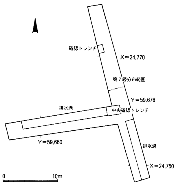
第55図 遺構配置図 (1/400)
