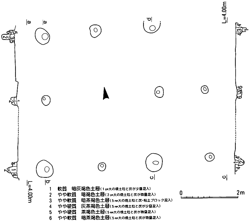
第106図 掘立柱建物跡 (SB001) 平面・断面図 (1/80)
