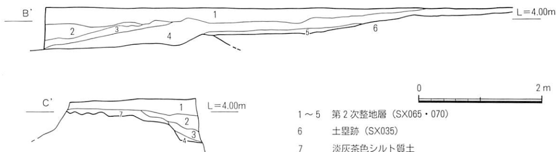
第150図 第2次整地層 (SX065・070) 土層図 (1/60)
