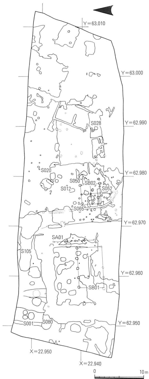
第82図 遺構配置図 (1/400)
