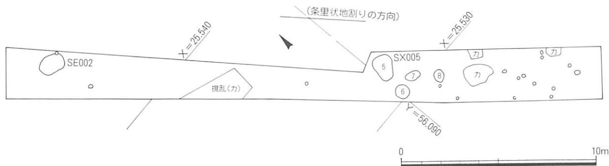
第169図 遺構配置図 (1/200)
