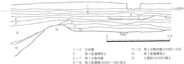
第147図 調査区南側壁土層図 (1/60)
