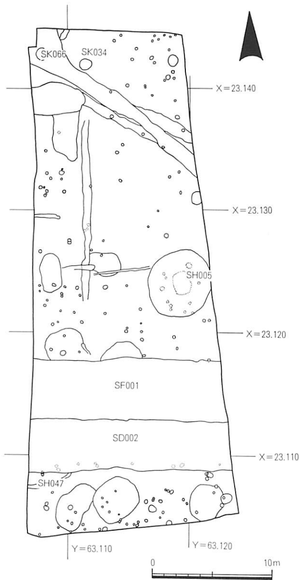
第86図 遺構配置図 (1/300)
