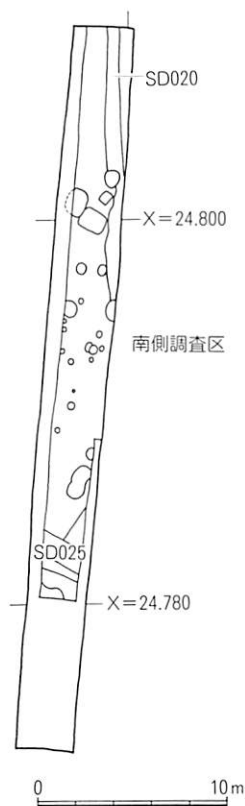
第51図 遺構配置図(1/400)
