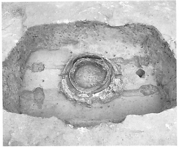
第111図 鑄造坑全景
