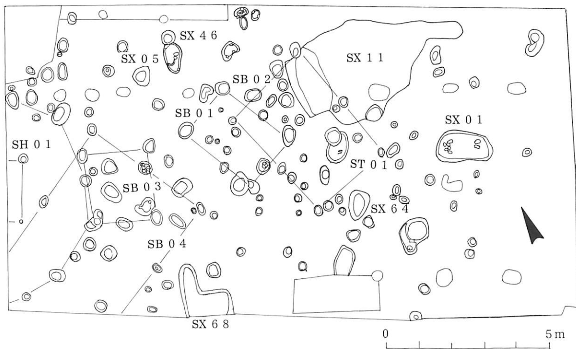
第165図 遺構配置図
