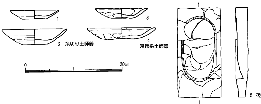
第125図 SX061出土遺物実測図（1/4）
