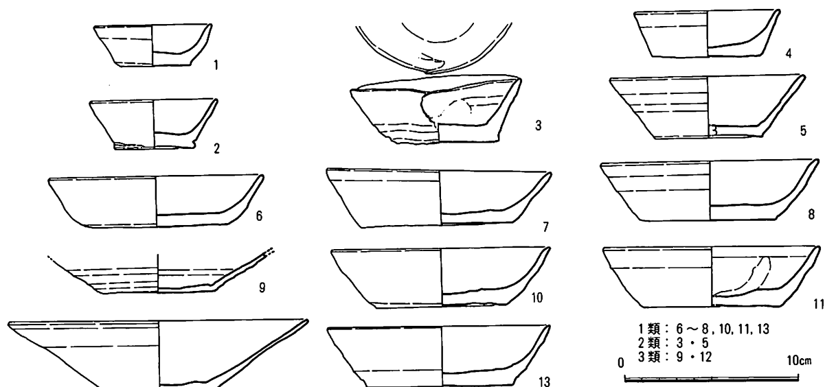
第136図 S008出土土器実測図 (1/3)
