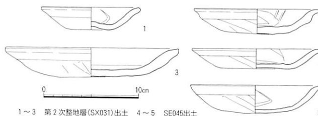
第151図 SX031・SE045出土遺物実測図 (1/4)
