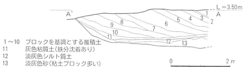
第155図 土塁跡 (SX035) 土層図 (1/80)
