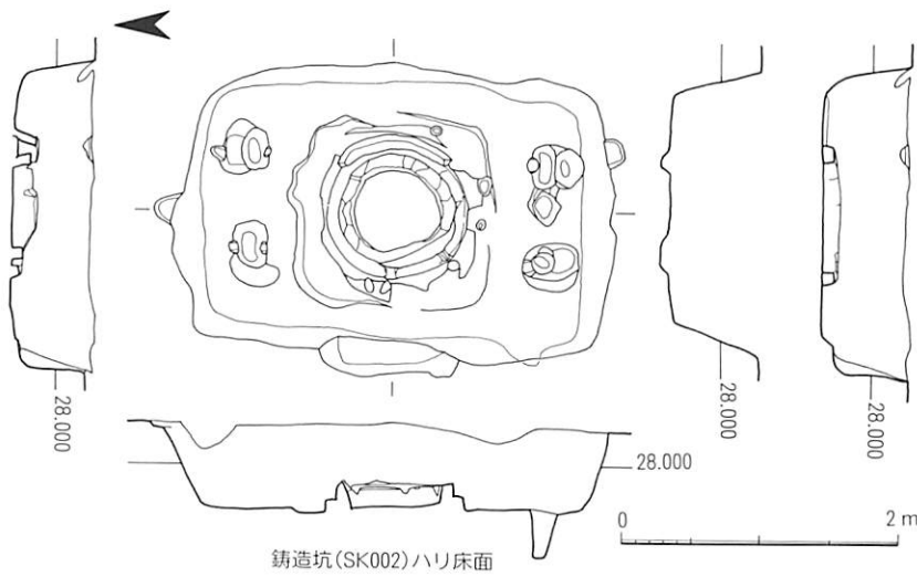
第112図 梵鐘鑄造遺構実測図 (1/60)
