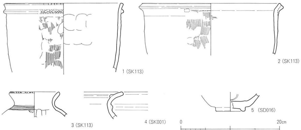
第13図 貯蔵穴 (SK)・溝 (SD) 出土遺物実測図 (1/4)
