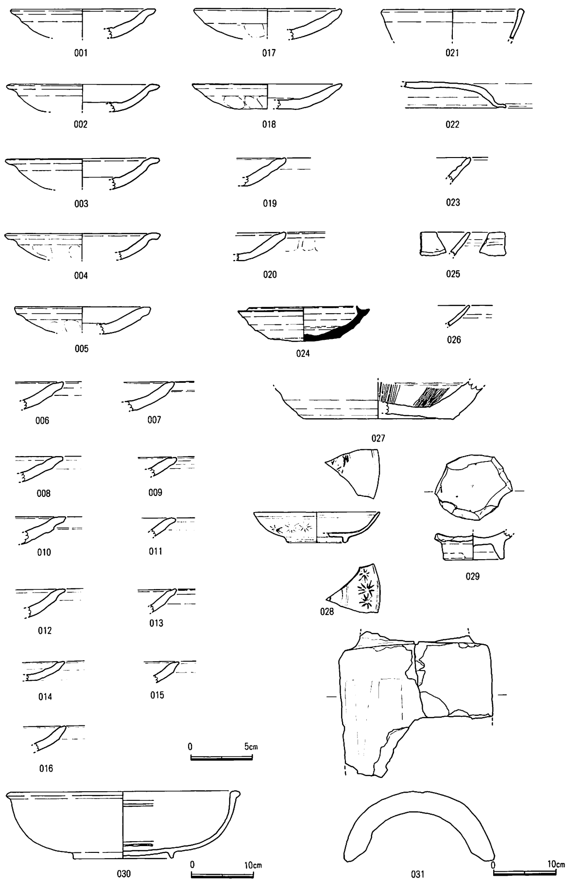
第106図 出土遺物実測図 (1/3・1/6)
