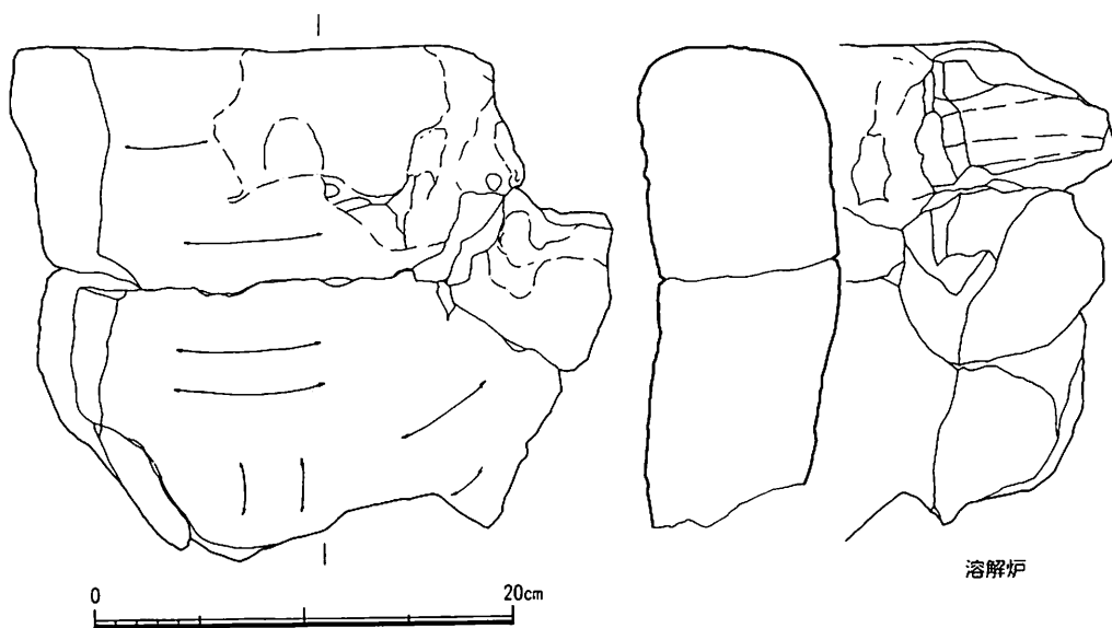
第114図 梵鏡鑄造遺構出土遺物実測図 (1/4)
