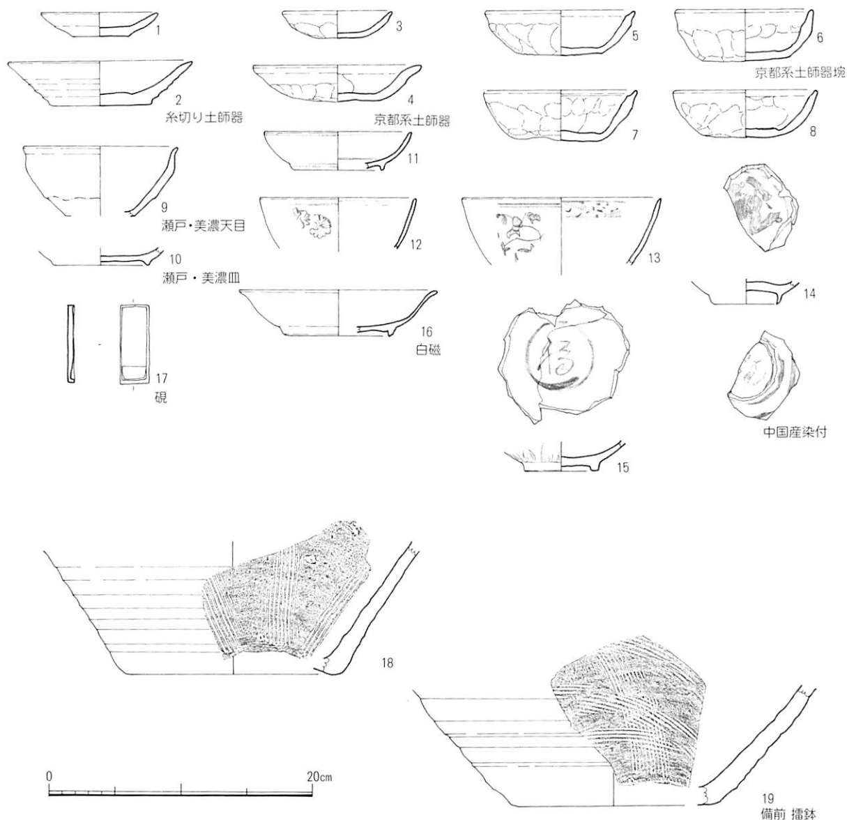
第124図 SK160出土遺物実測図（1/4）
