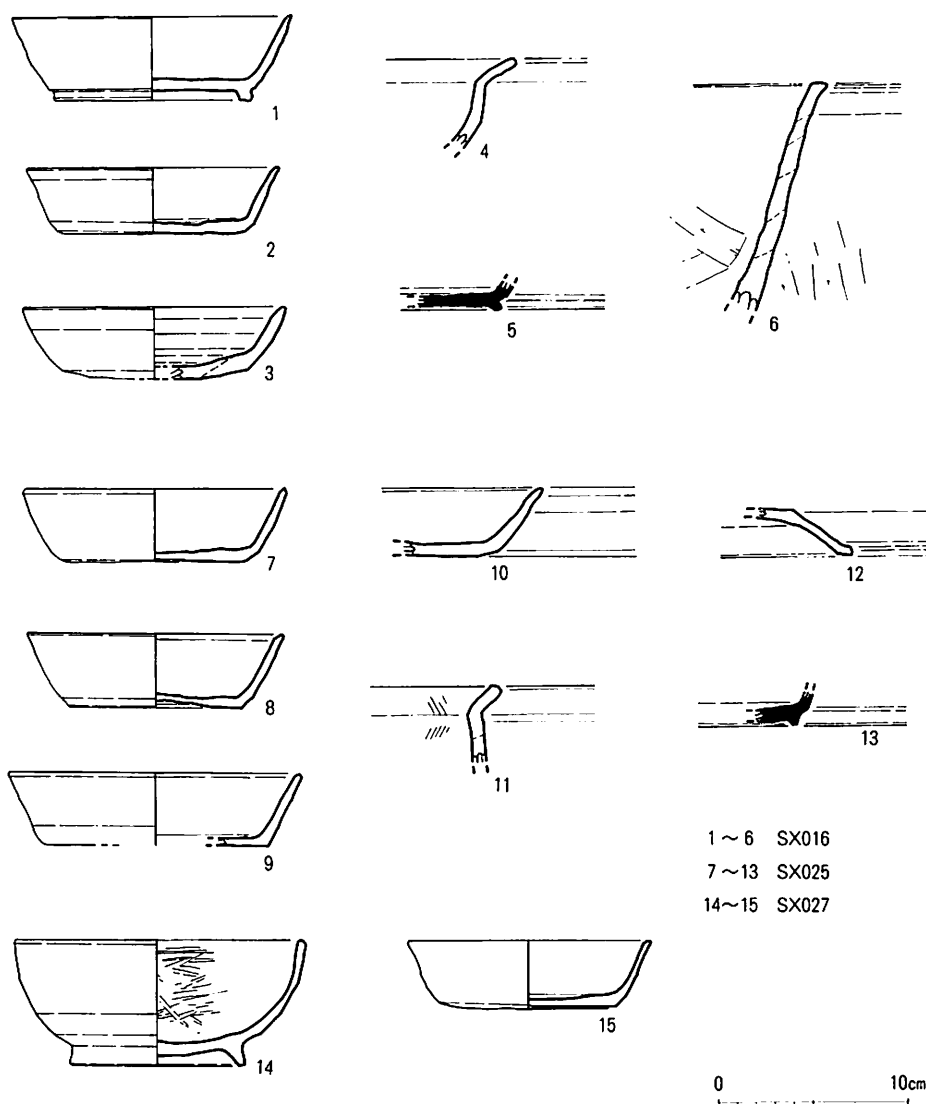
第25図 出土遺物実測図（1/4）
