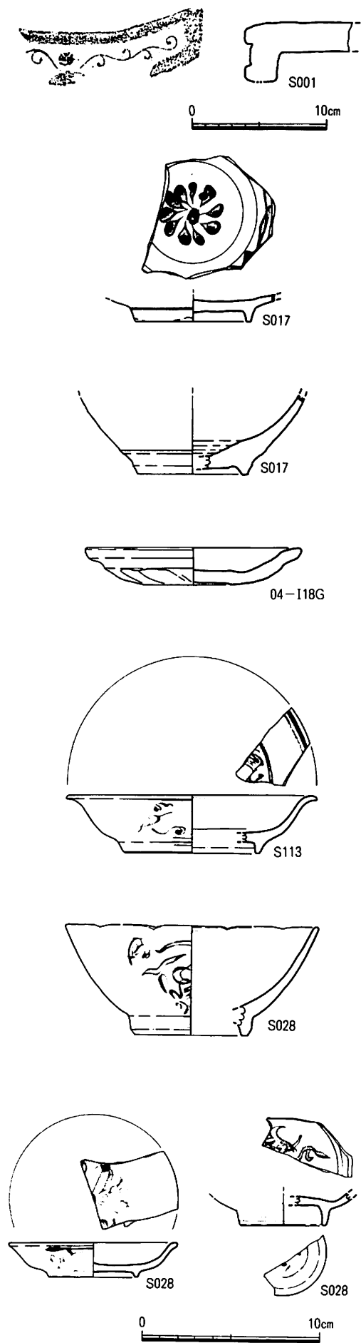
第79図 出土遺物実測図 (1/4・1/3)
