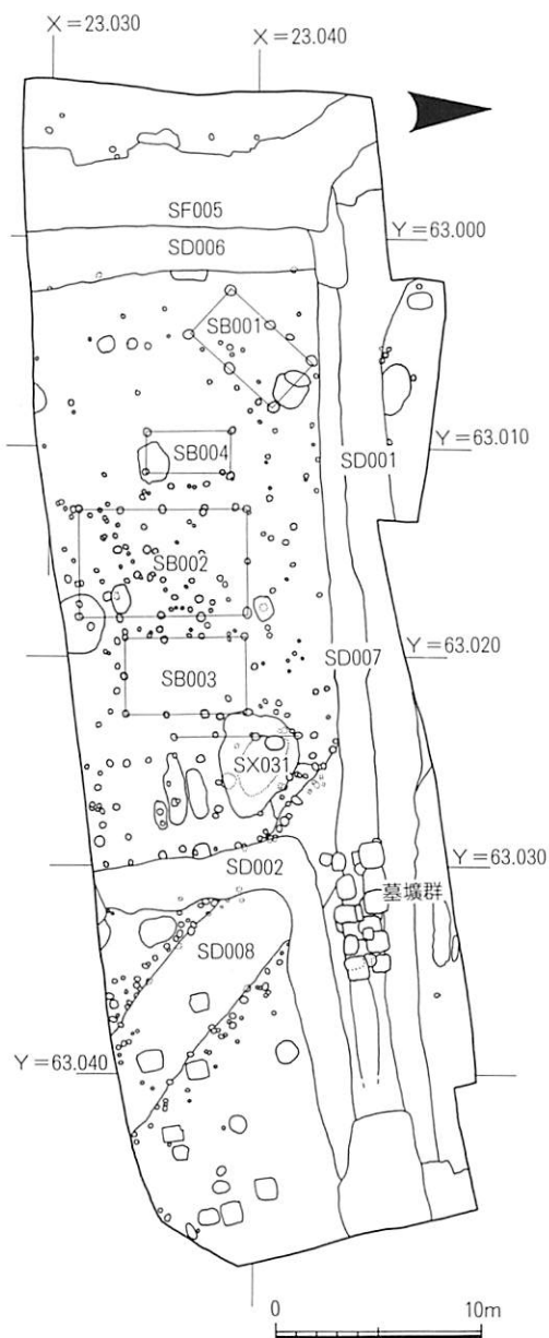
第69図 遺構配置図 (1/400)
