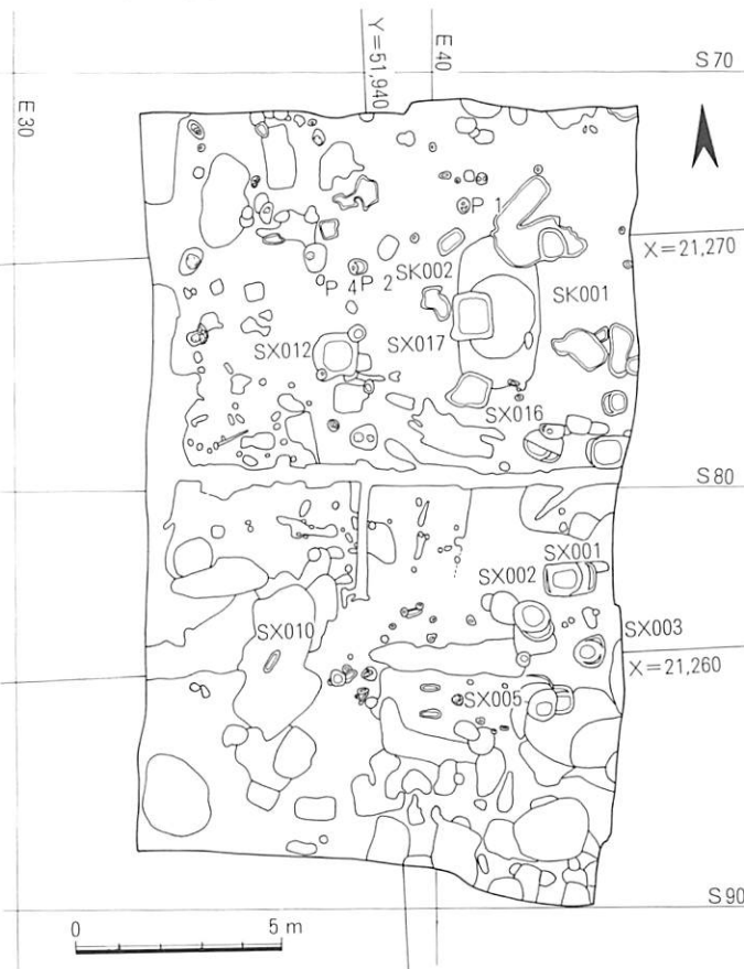
第109図 遺構配置図 (1/200)
