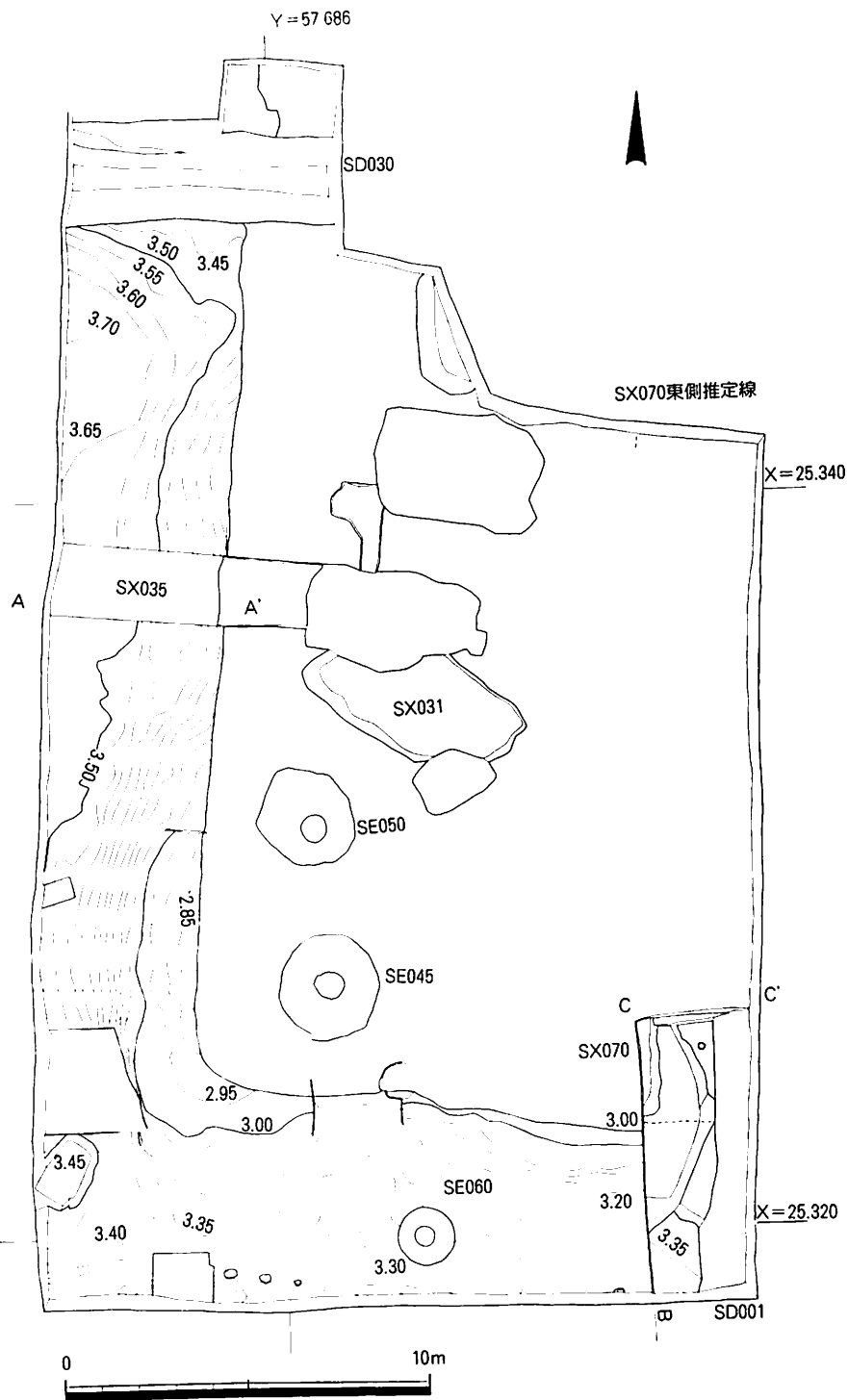
第152図 第3面遺構配置図 (1/200)
