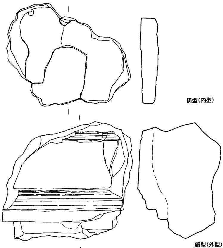
第113図 梵鏡鑄造遺構出土遺物実測図 (1/4)
