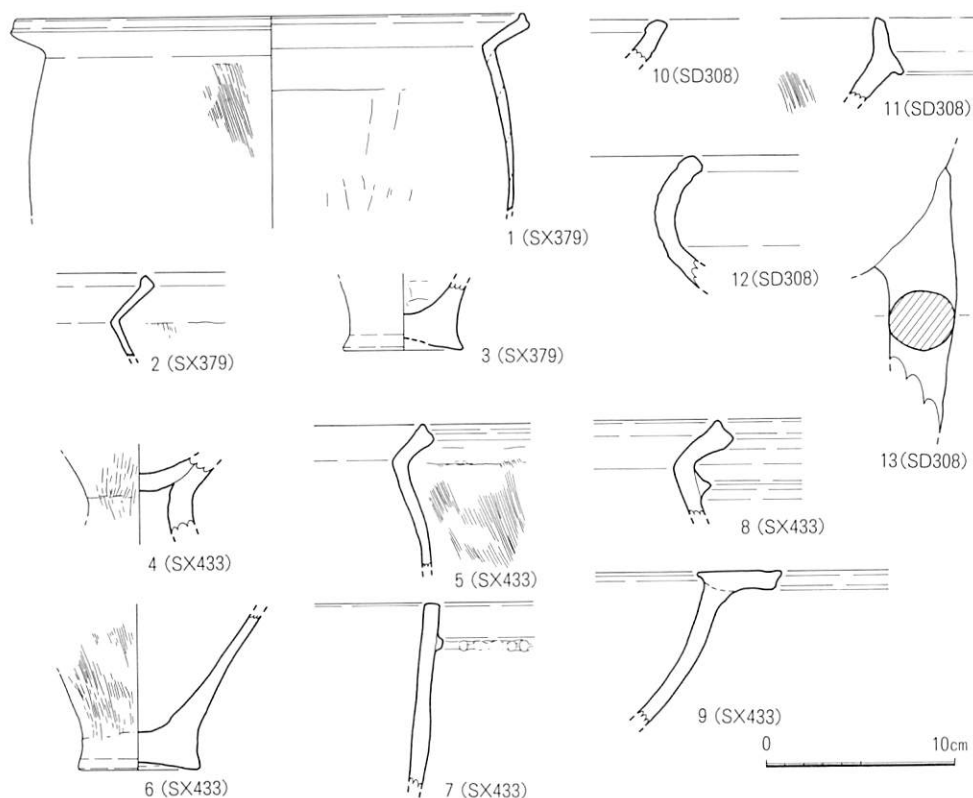
第57図 出土遺物実測図 (1/4)
