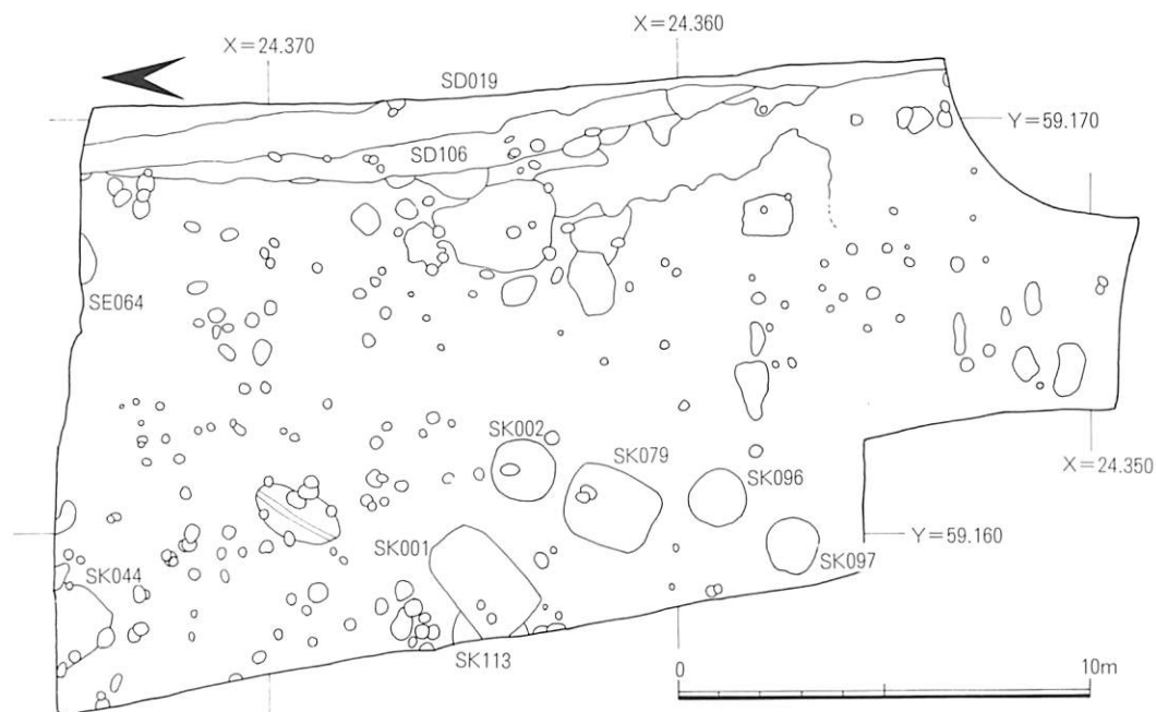
第11図 遺構配置図 (1/200)
