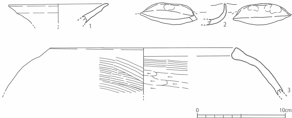
第 13 図 弥五郎遺跡 SK03 出土遺物 (S = 1 / 2)
