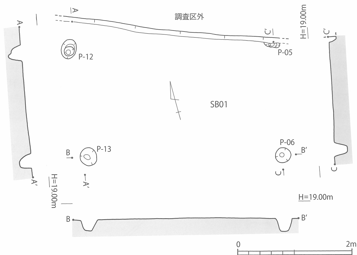
第 4 図 弥五郎遺跡 SB01 実測図（S = 1 / 40）
