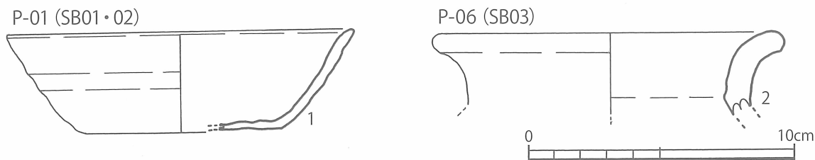
第7図 弥五郎遺跡 SB 出土遺物 (S = 1 / 2)
