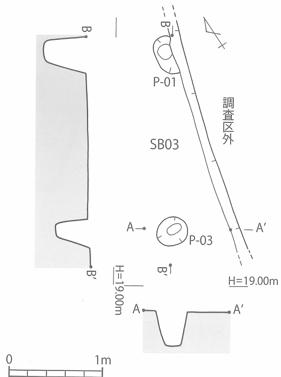
第6図 弥五郎遺跡 SB03 実測図 (S=1/40)
