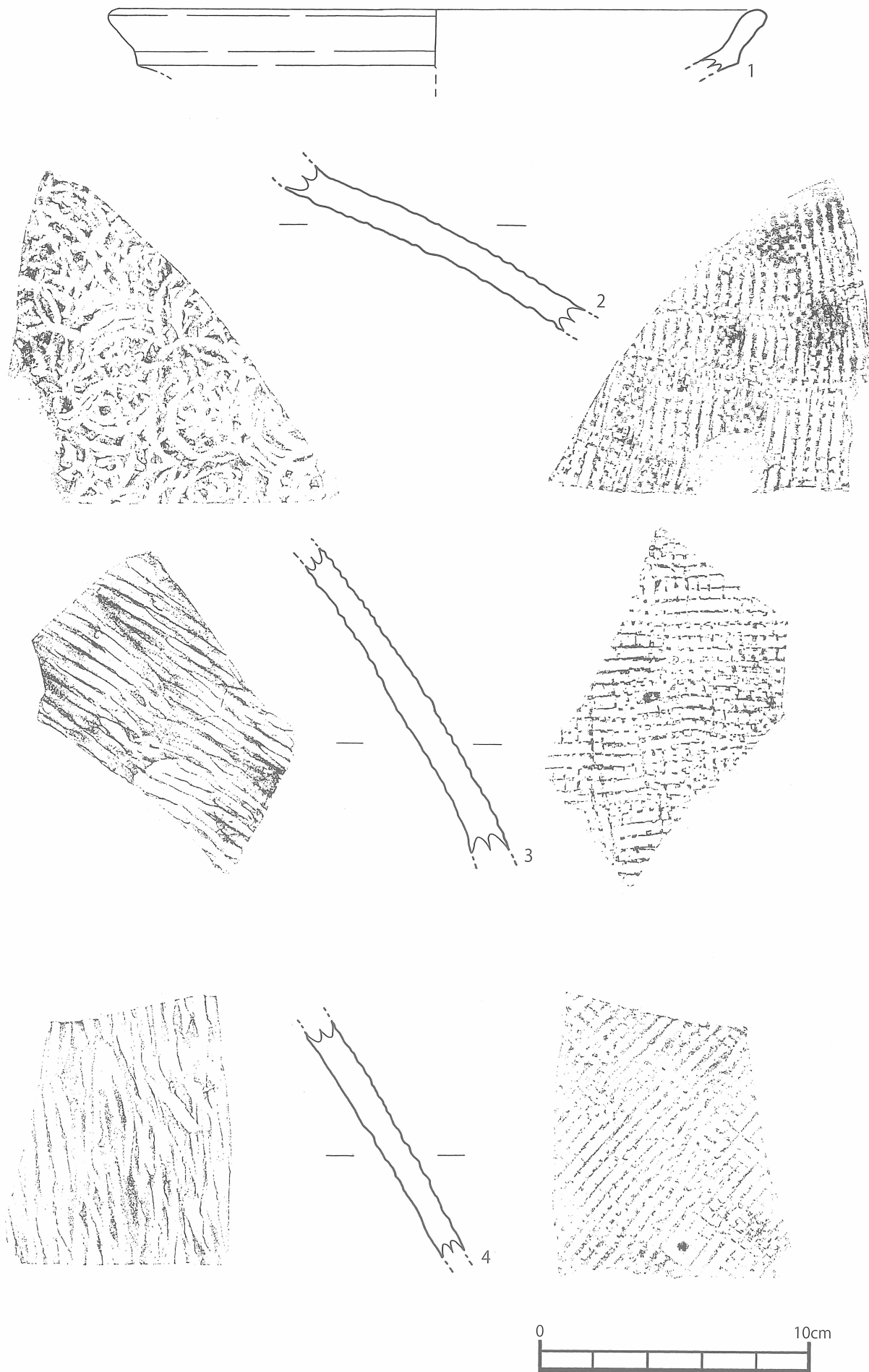
第 11 図 弥五郎遺跡 SK02 出土遺物 2 (S=1 / 2)
