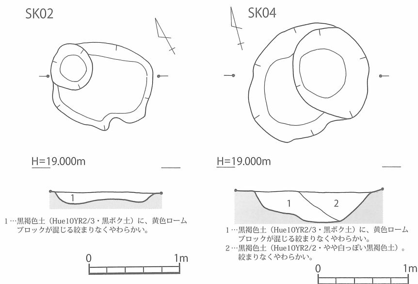
第8図 弥五郎遺跡 SK02 実測図 (S = 1 / 40)
