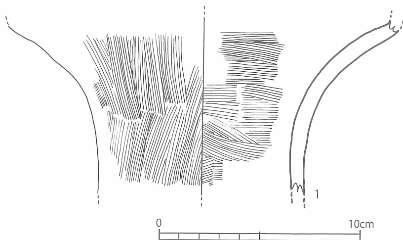
第 15 図 弥五郎遺跡表土層出土遺物 (S = 1 / 2)
