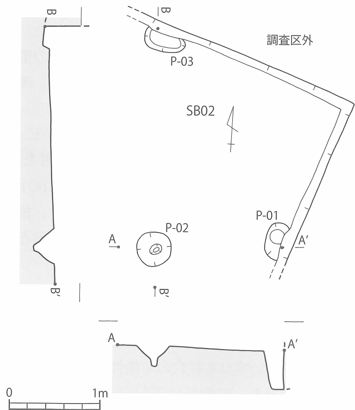
第5図 弥五郎遺跡 SB02 実測図 (S=1/40)
