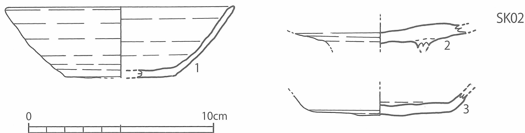
第10図 弥五郎遺跡 SK02 出土遺物 1 (S = 1 / 2)
