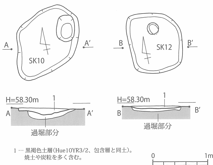
第 19 図 中甸遺跡 SK10・12 実測図 (S=1/40)
