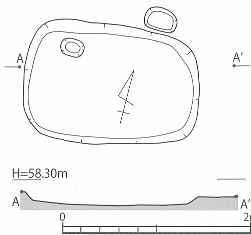
第11図 中甸遺跡SK01実測図 (S=1/40)
