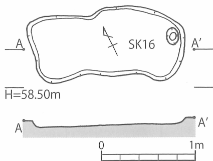
第25図 中甸遺跡SK16実測図 (S=1/40)
