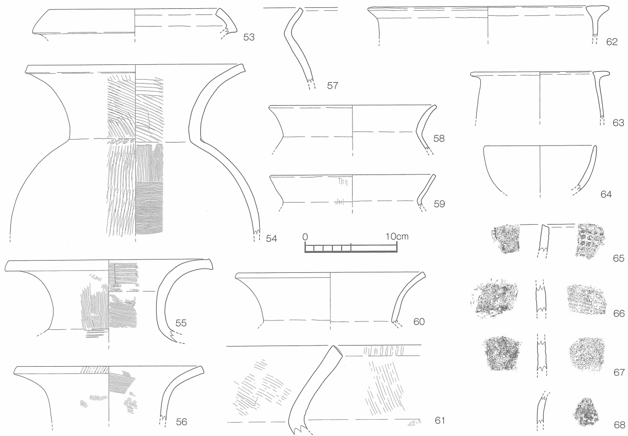
第 1 2 図 原ノ前遺跡 6号竪穴住居 (SB-06) 出土遺物実測図 [1/4]
