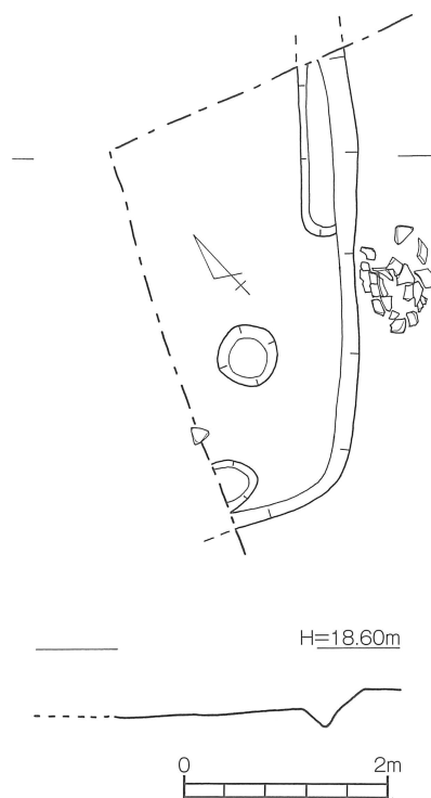
第 15 図 原ノ前遺跡 8 号竪穴住居 (SB-08) 実測図 [1/40]
