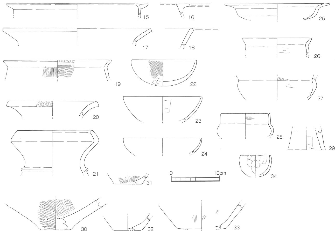
第6図 原ノ前遺跡 2号竪穴住居 (SB-02) 出土遺物実測図 [1/4]
