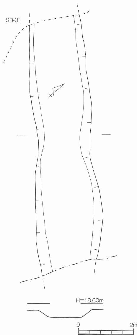
第23図 原ノ前遺跡 1号溝状遺構 (SD-01) 実測図 [1/40]
