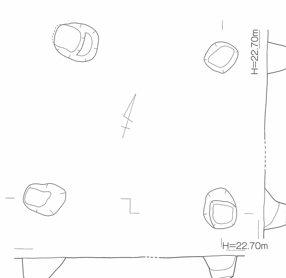
第35図 松本遺跡 7号掘立柱建物 (SB07) 実測図 [1/80]
