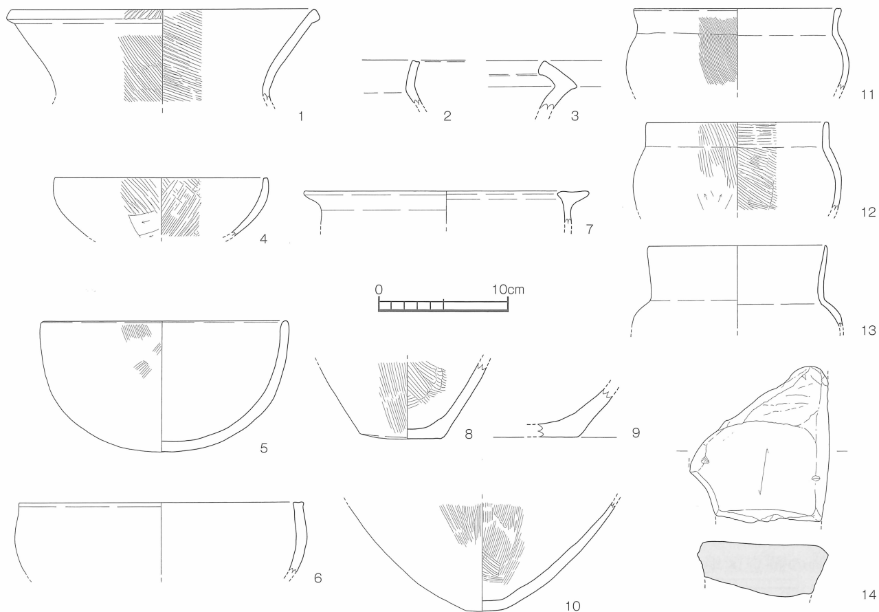
第5図 原ノ前遺跡 1号竪穴住居 (SB-01) 出土遺物実測図 [1/4]
