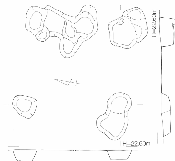
第45図 松本遺跡 17号掘立柱建物 (SB 17) 実測図 [1/80]
