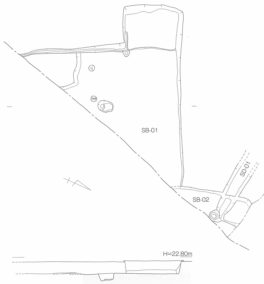
第30図 松本遺跡 1, 2号竪穴住居 (SB01, 02) 実測図 [1/80]
