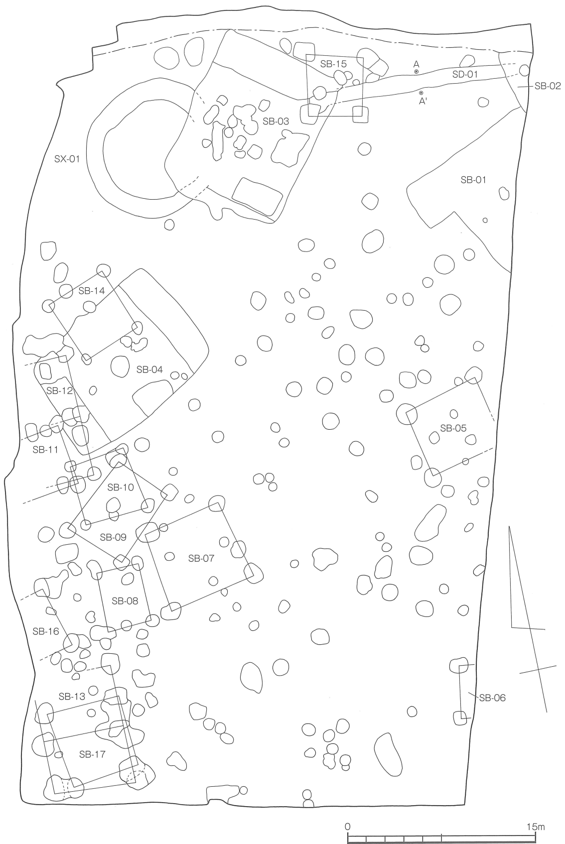
第29図 松本遺跡遺構配置図 [1/150]
