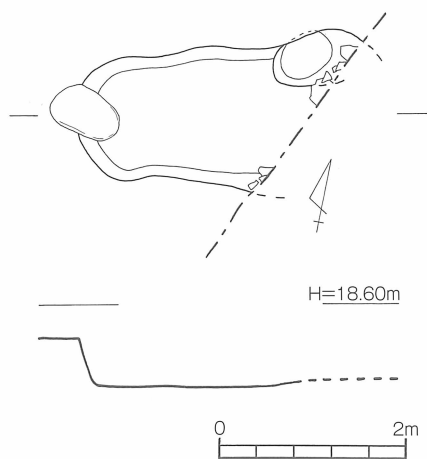
第21図 原ノ前遺跡 3号土坑 (SK-03) 実測図 [1/40]
