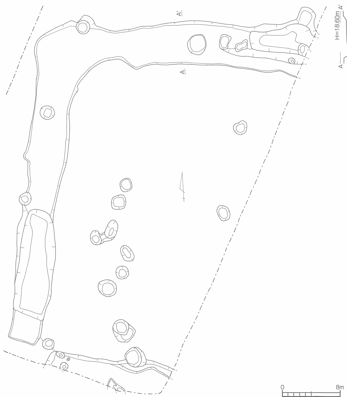
第26図 原ノ前遺跡 2号不明遺構 (SX-02) 実測図 [1/80]
