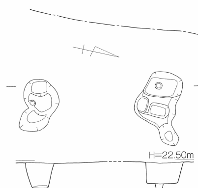
第44図 松本遺跡 16号掘立柱 建物 (SB16) 実測図 [1/80]
