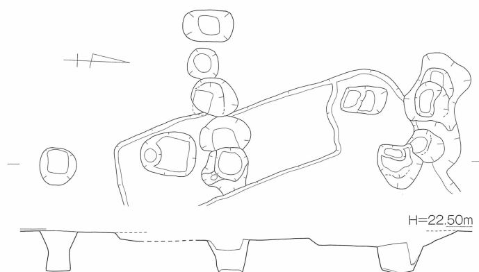
第40図 松本遺跡 12号掘立柱建物 (SB12) 実測図 [1/80]
