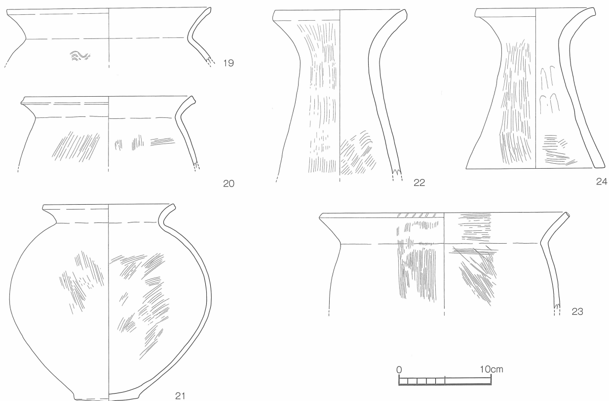
第49図 松本遺跡 13, 14号掘立柱建物 (SB13, 14)・1号不明遺構 (SX01)・ピット出土土器実測図 [1/4]
