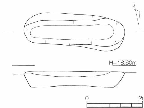
第25図 原ノ前遺跡 1号不明遺構 (SX-01) 実測図 [1/40]
