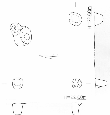
第38図 松本遺跡 10号掘立柱建物 (SB10) 実測図 [1/80]
