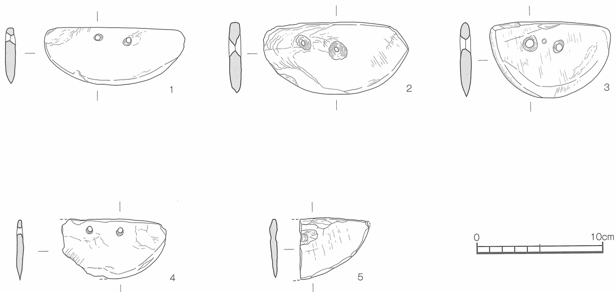
第50図 松本遺跡 3, 4号竪穴住居 (SB03, 04) 出土石製品実測図 [1/3]
