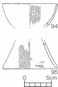
第19図 原ノ前遺跡 1号土坑 (SK-01) 出土遺物実測図 [1/4]
