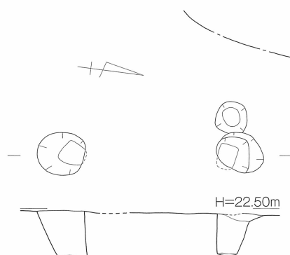
第39図 松本遺跡 11号掘立柱建物 (SB11) 実測図 [1/80]
