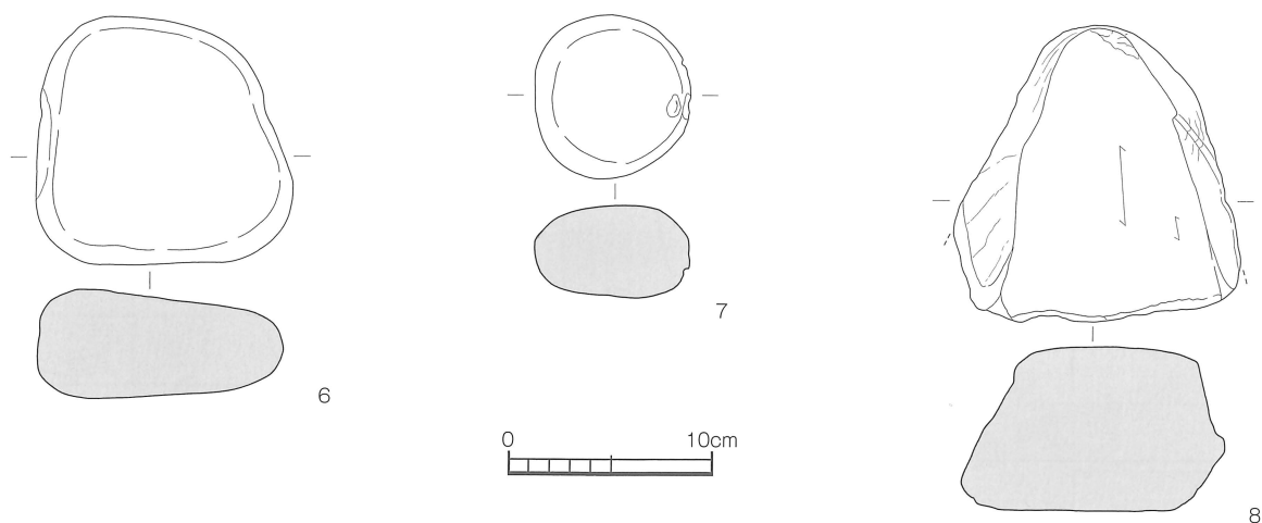
第51図 松本遺跡 4号竪穴住居（SB04）出土石製品実測図〔1／4〕
