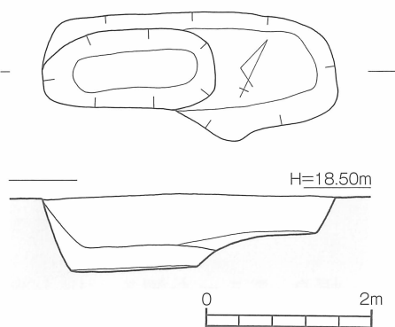
第20図 原ノ前遺跡 2号土坑 (SK-02) 実測図 [1/40]
