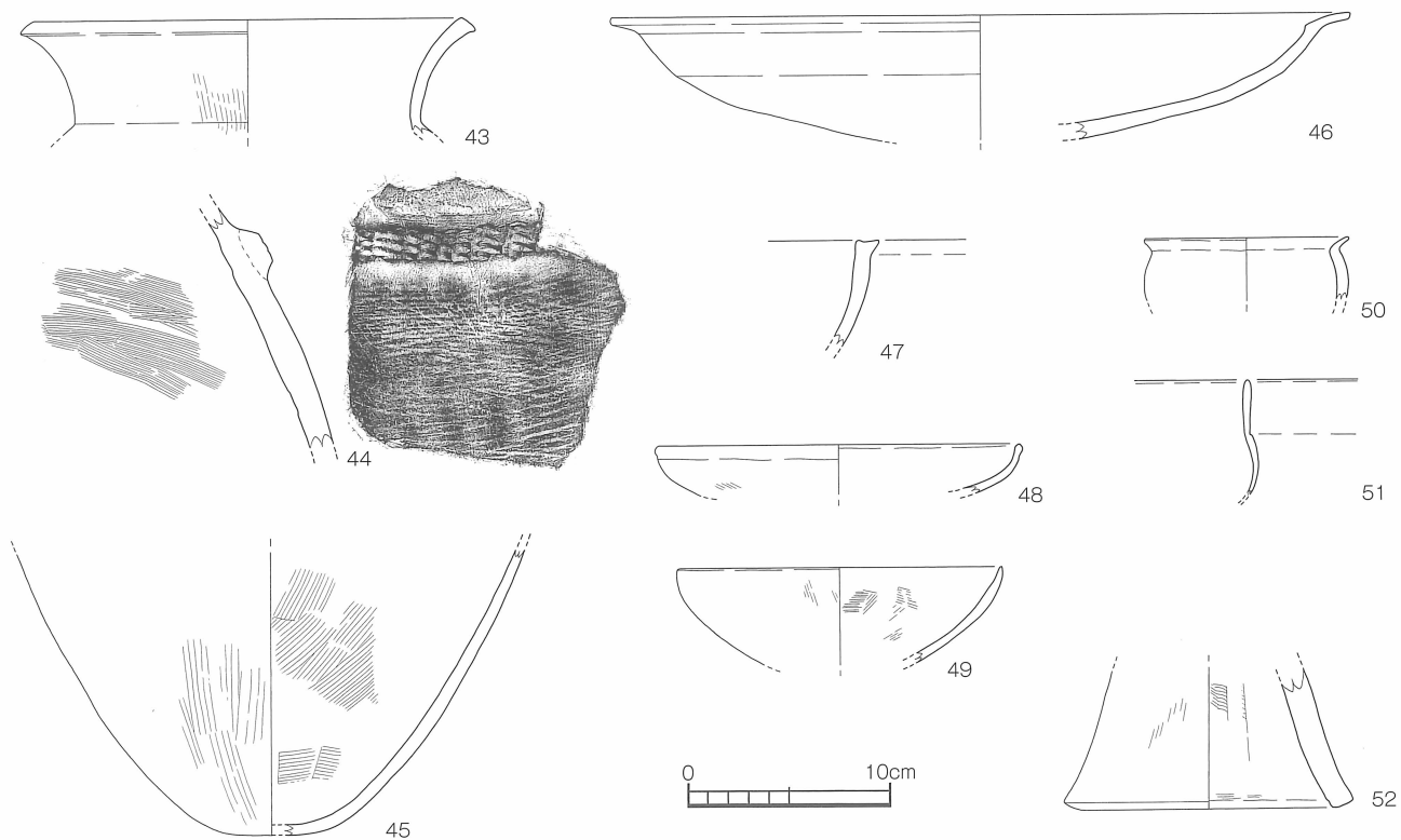
第 1 1 図 原ノ前遺跡 5号竪穴住居 (SB-05) 出土遺物実測図 [1/4]
