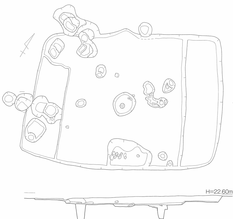
第32図 松本遺跡 4号竪穴住居 (SB04) 実測図 [1/80]
