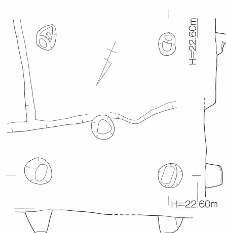
第42図 松本遺跡 14号掘立柱 建物 (SB14) 実測図 [1/80]
