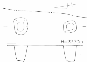
第34図 松本遺跡 6号掘立柱建物 (SB06) 実測図 [1/80]
