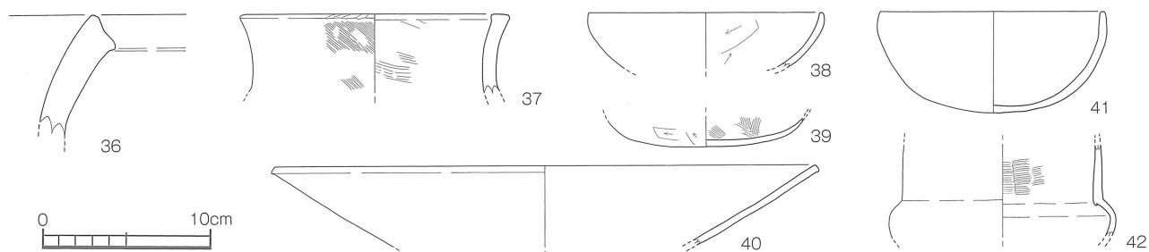
第9図 原ノ前遺跡 4号竪穴住居 (SB-04) 出土遺物実測図 [1/4]
