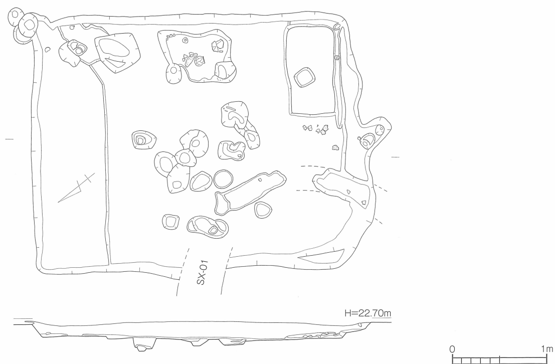
第31図 松本遺跡 3号竪穴住居 (SB03) 実測図 [1/80]
