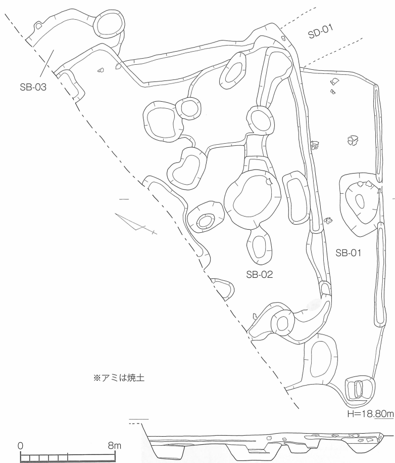
第4図 原ノ前遺跡 1, 2, 3号竪穴住居 (SB-01, 02, 03) 実測図 [1/80]
