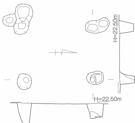
第36図 松本遺跡 8号掘立柱建物 (SB08) 実測図 [1/80]
