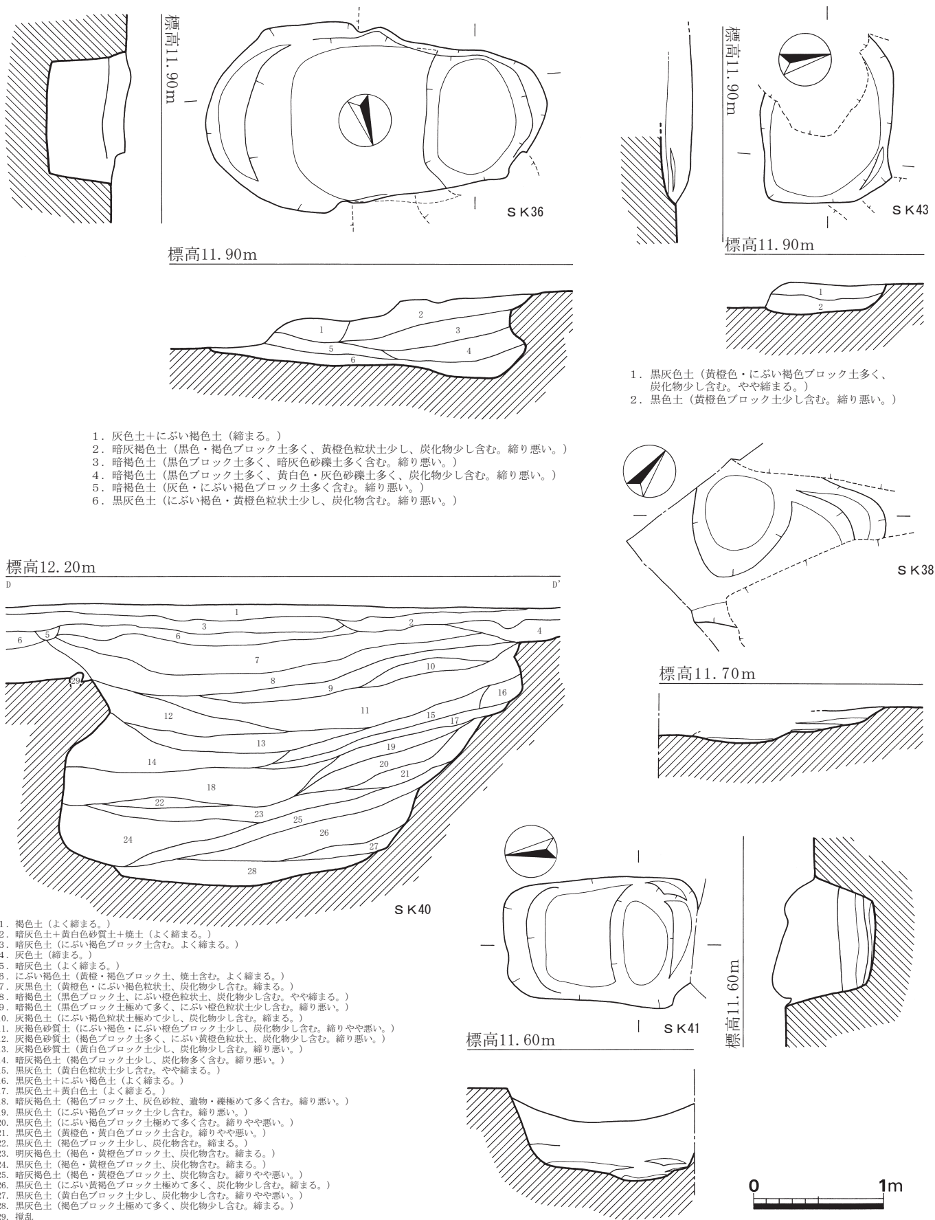
第11図 SK36・38・41・43 実測図、SK40 土層図 (1/40)
