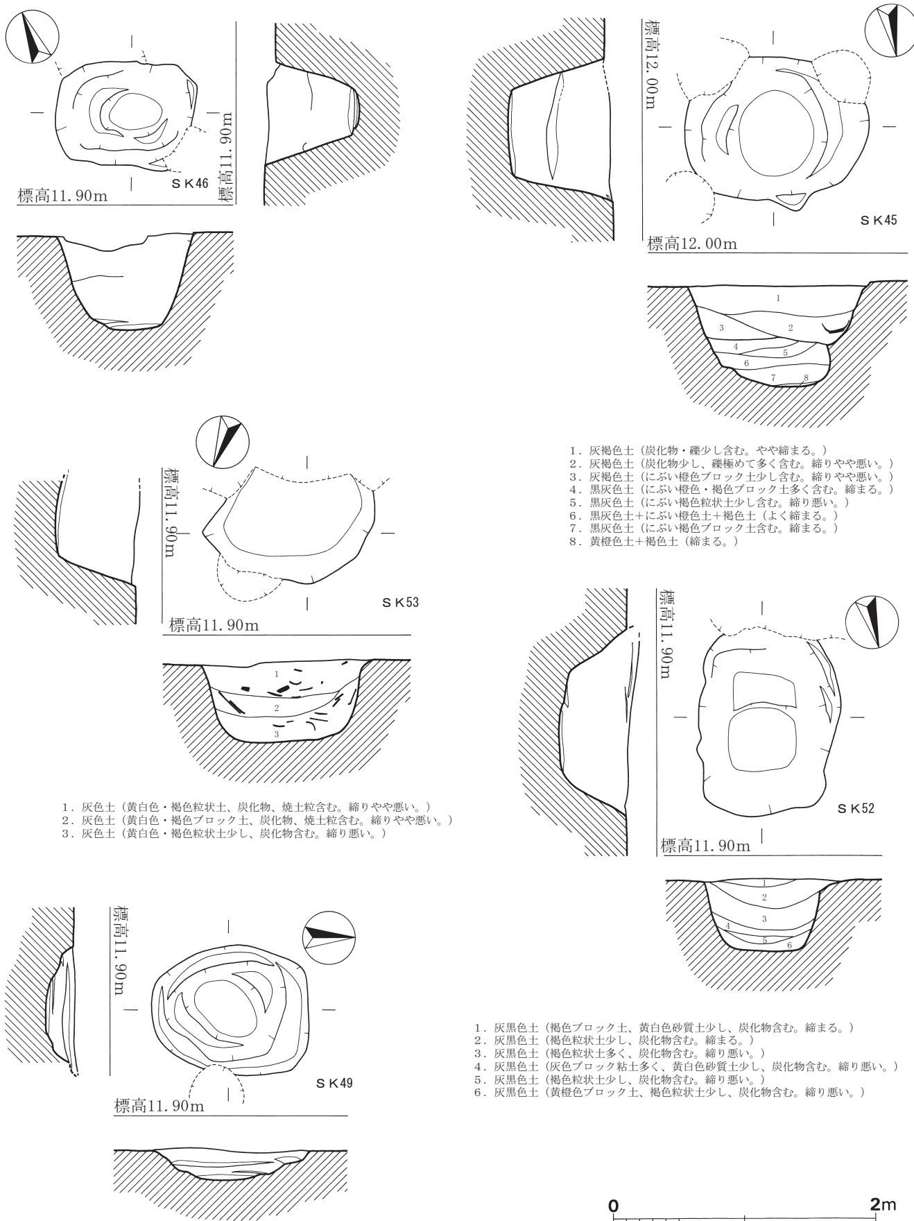
第12図 SK45・46・49・52・53実測図 (1/40)
