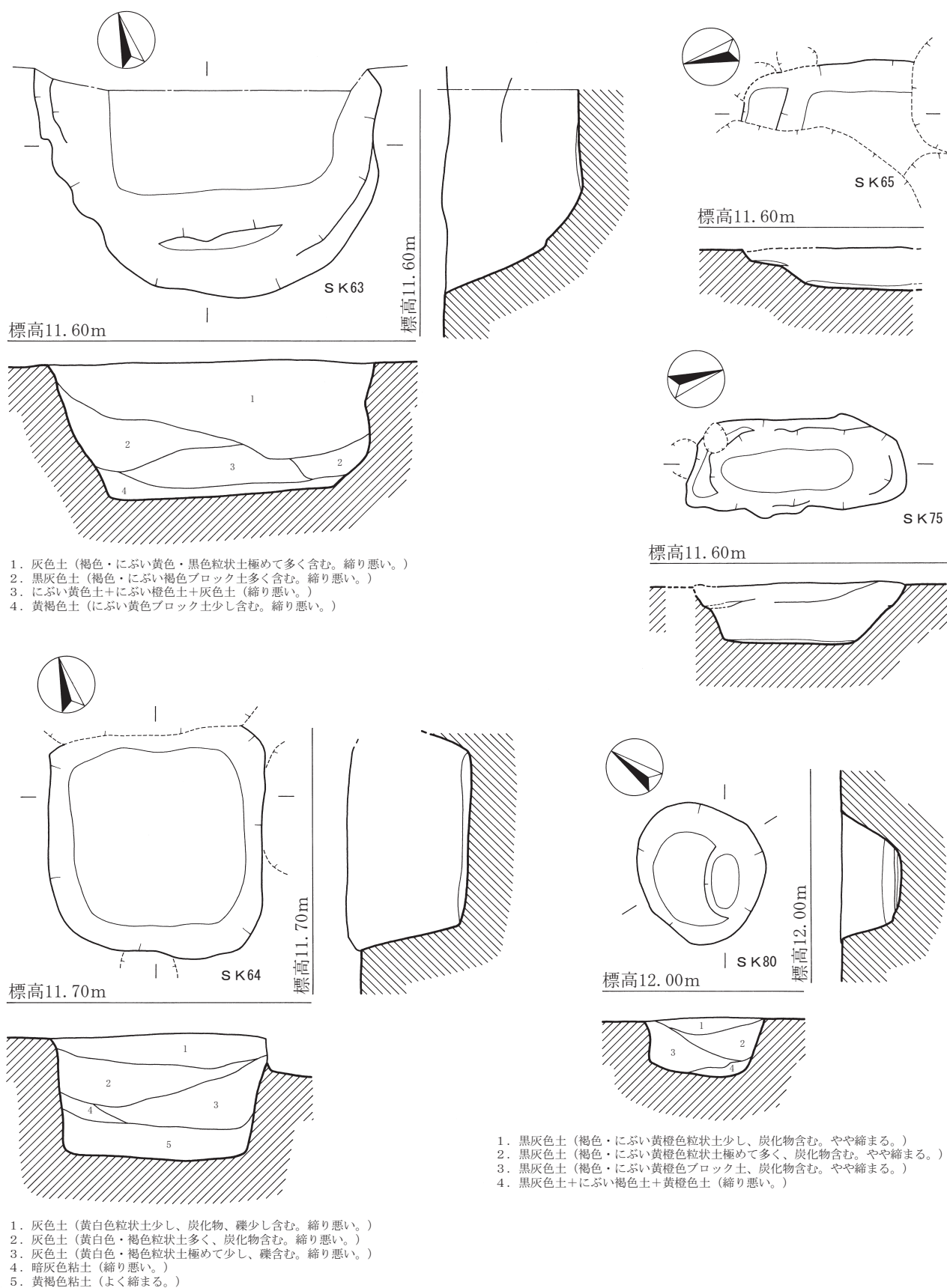
第14図 S K63・64・65・75・80 実測図 (1/40)
