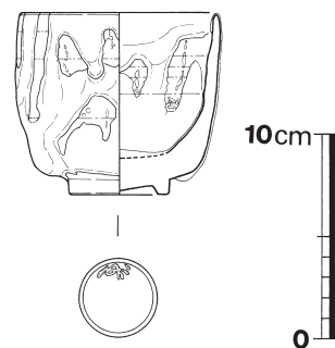
第17図 遺物実測図 (1/4)
