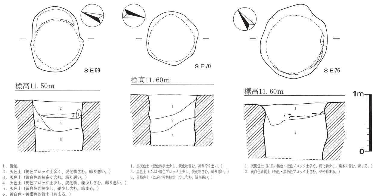
第9図 SE69・70・76 実測図（1/40）
