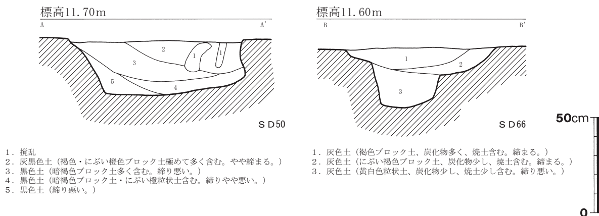
第8図 SD50・66 土層図 (1/20)
