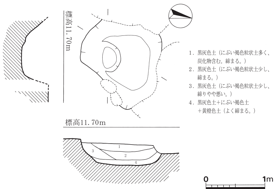
第16図 SK90 実測図 (1/40)
