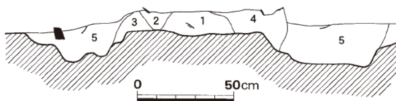
第5図 S I 10カマド実測図 (1/20)
