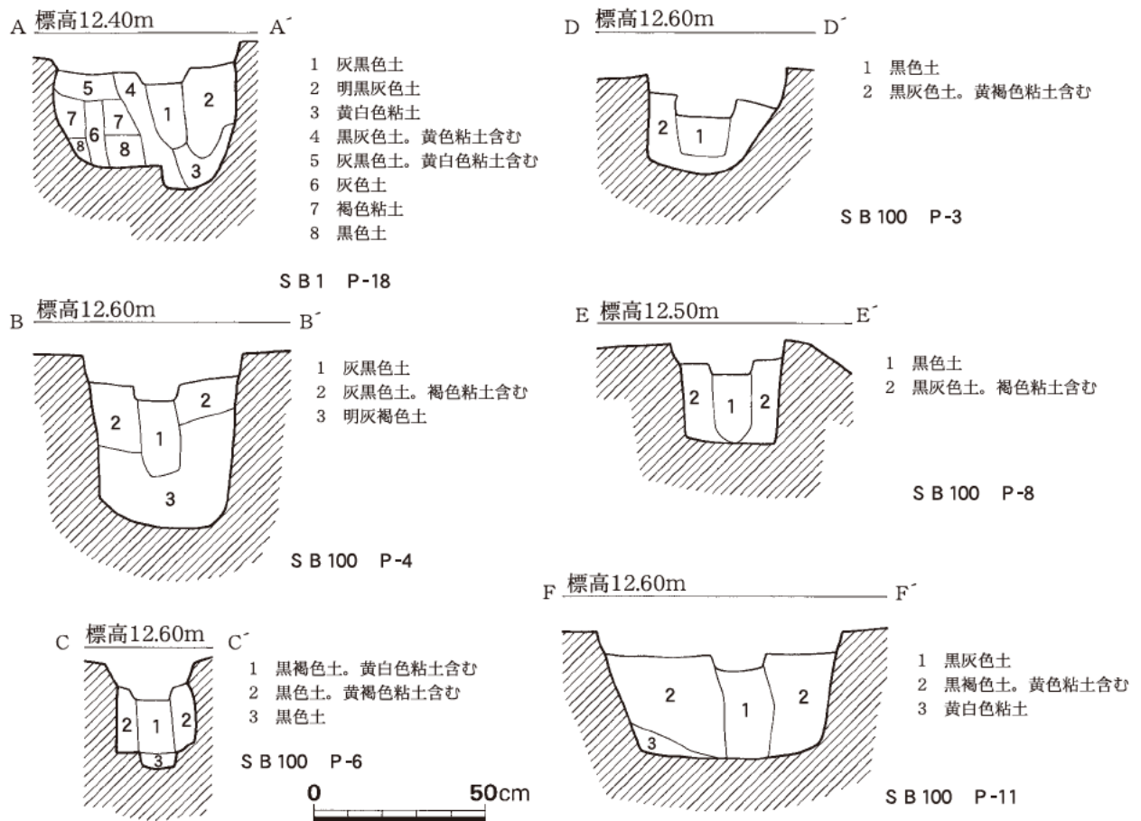
第10図 S B 1・100柱穴土層断面図 (1/20)
