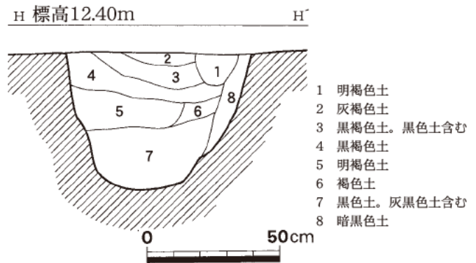
第19図 SD20土層断面図（1/20）
