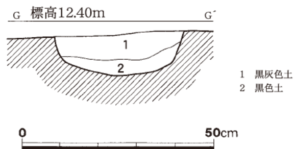
第16図 SD 5 土層断面図 (1/10)
