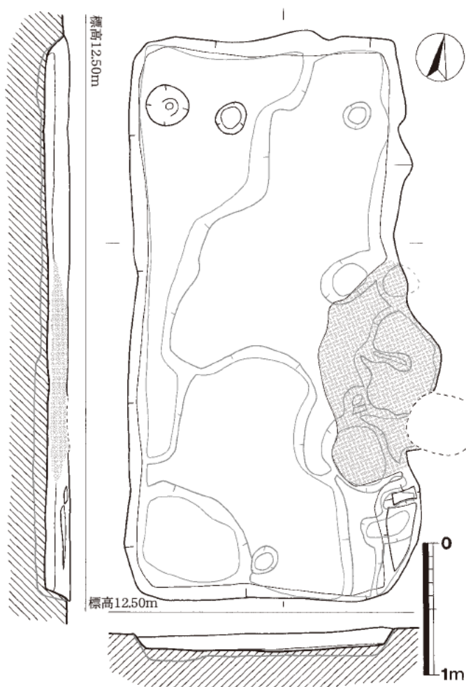
第3図 S I 10実測図（1/40）
