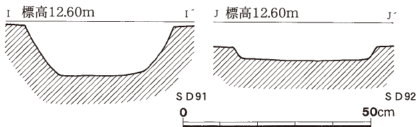
第23図 SD91・92断面図（1/10）
