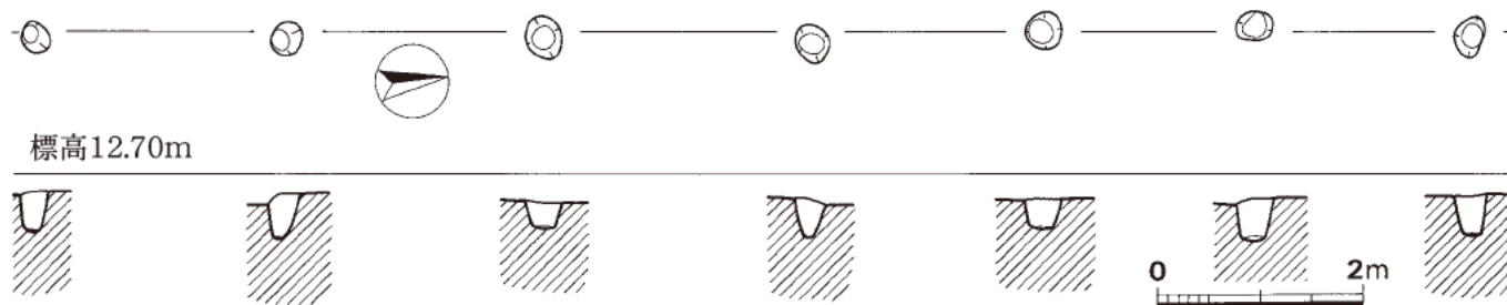
第15図 SA129実測図 (1/80)
