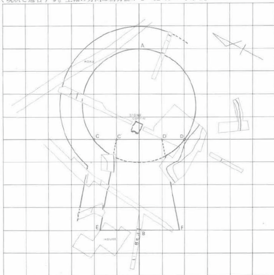
第13図 木塚古墳復元推定図(1/600)
