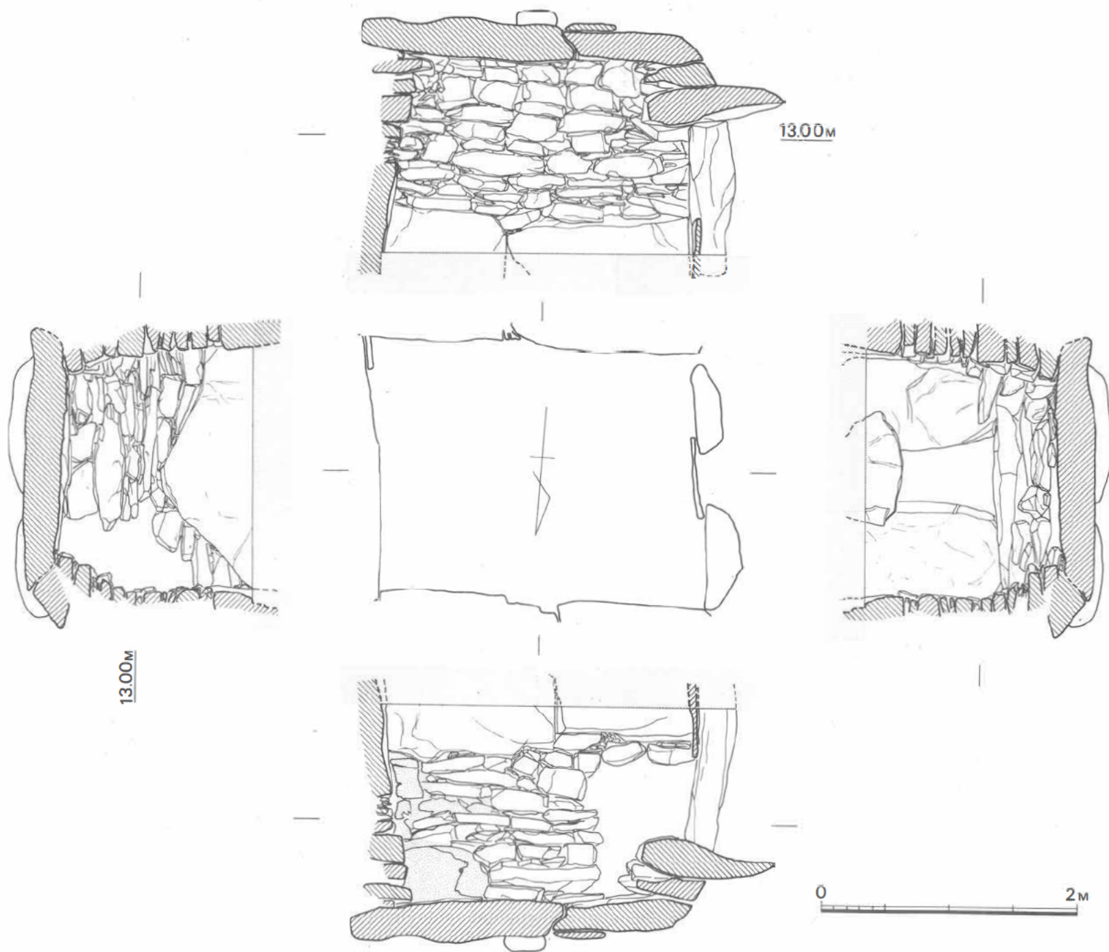
第11図 木塚古墳石室実測図(40)
