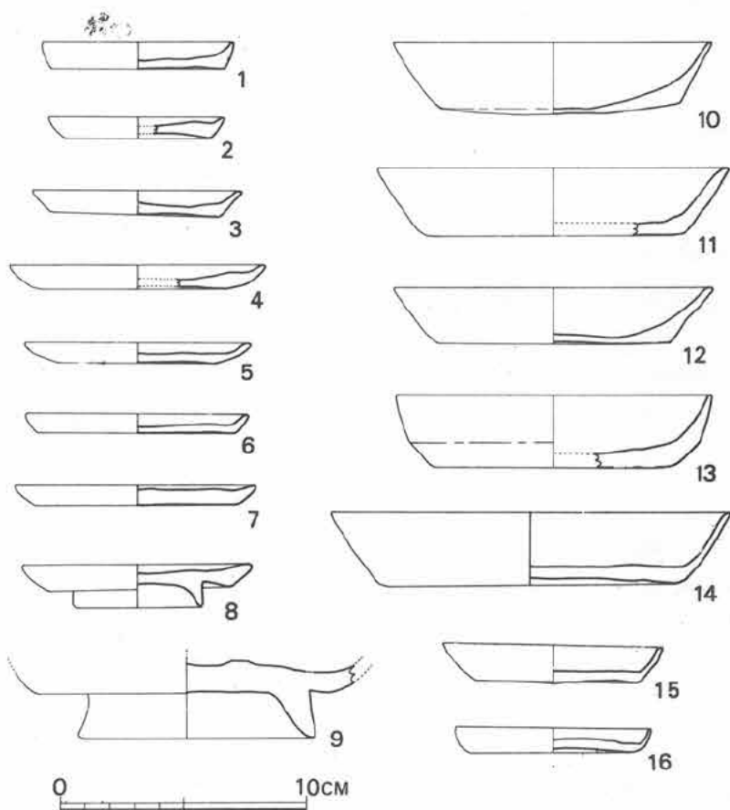
第58図 IV区出土土師器実測図 (1/3)
