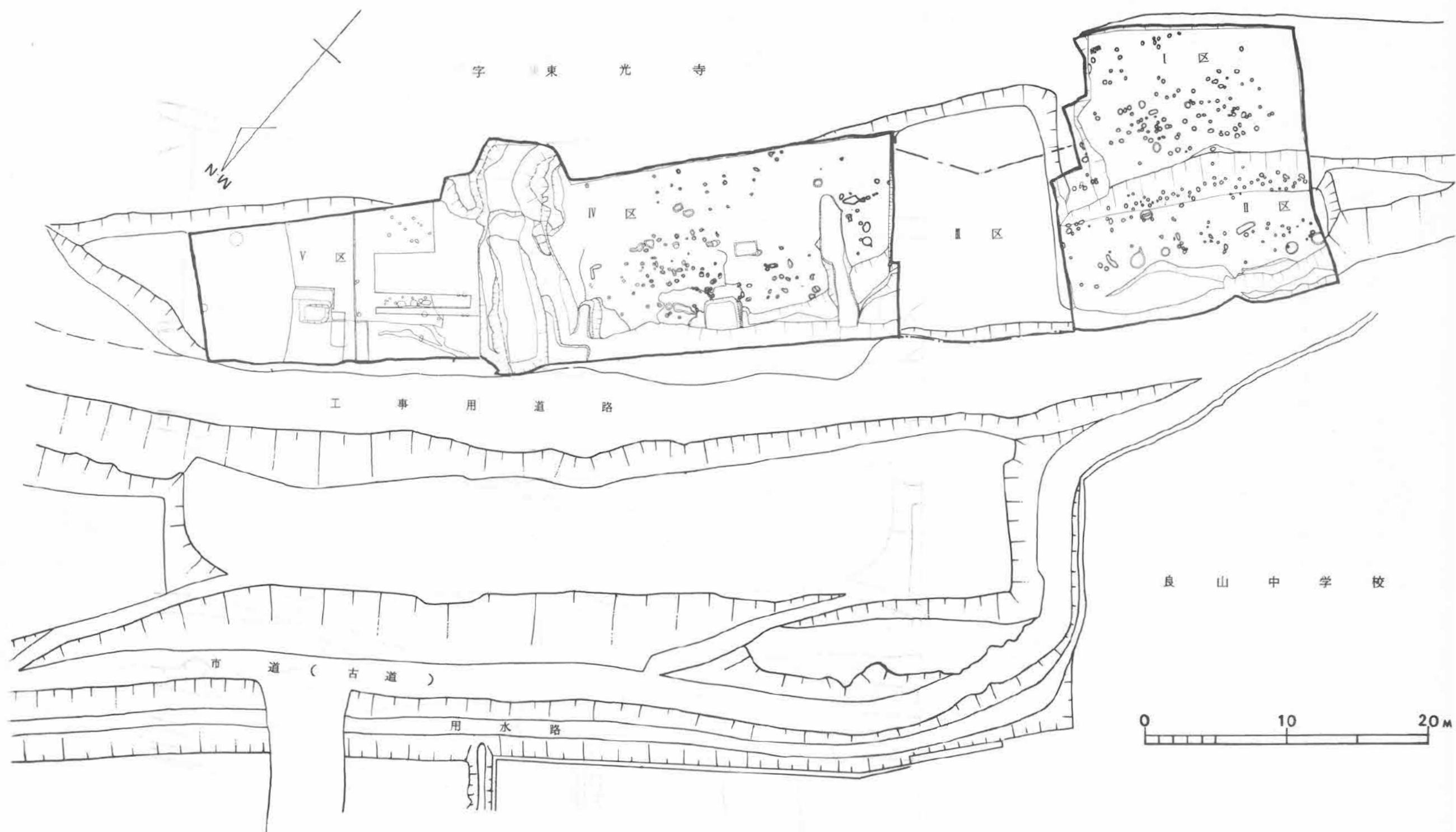
第41図 東光寺遺構全体図 (1/300)
