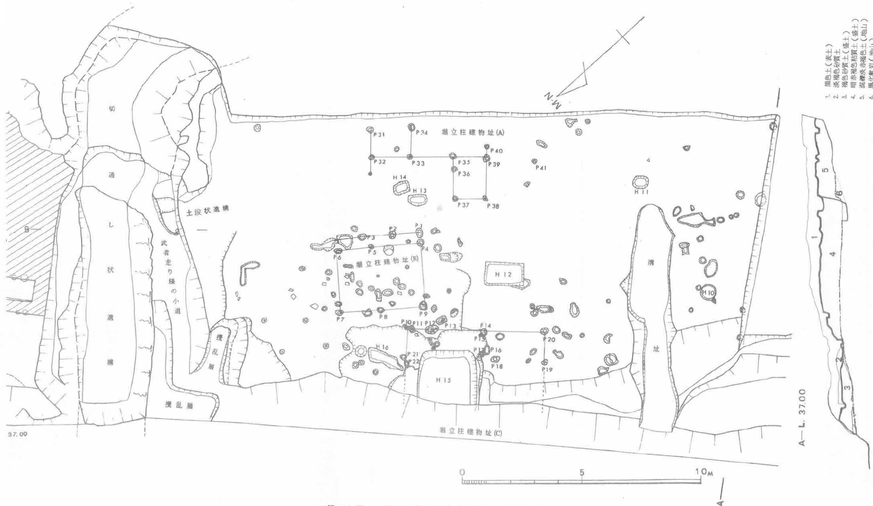
第44図 N区遺構実測図 (1/100)
