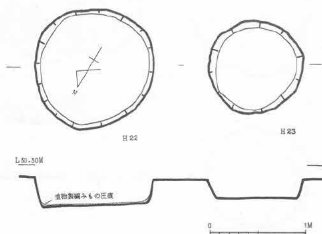
第10図 VI 区土壇実測図 (1/40)
