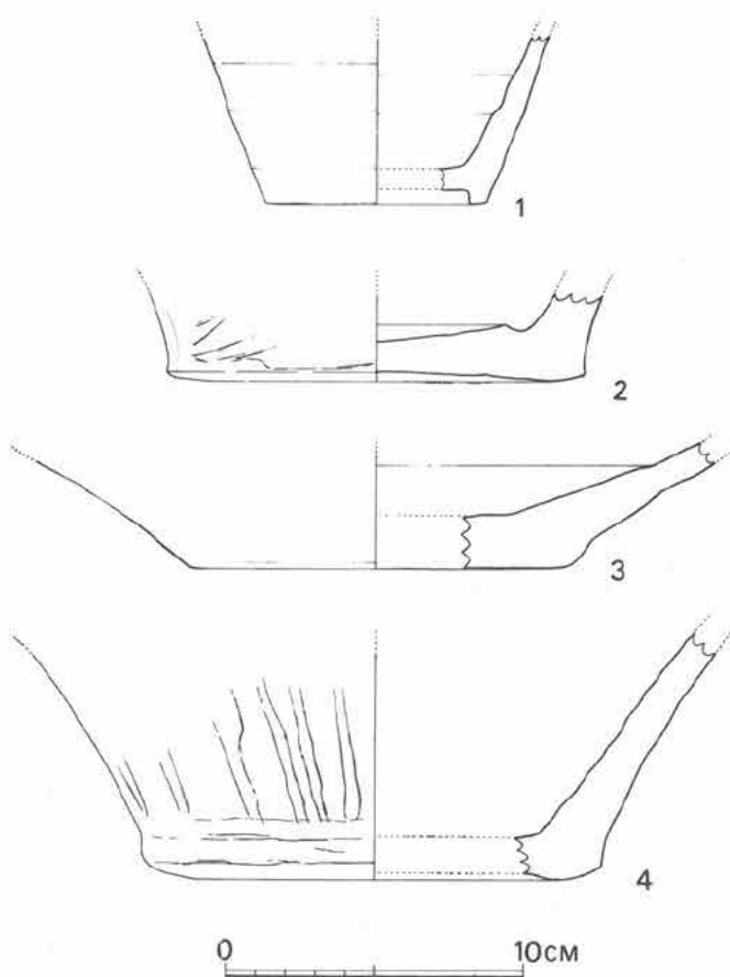
第60図 IV区出土陶器実測図 (1/3)
