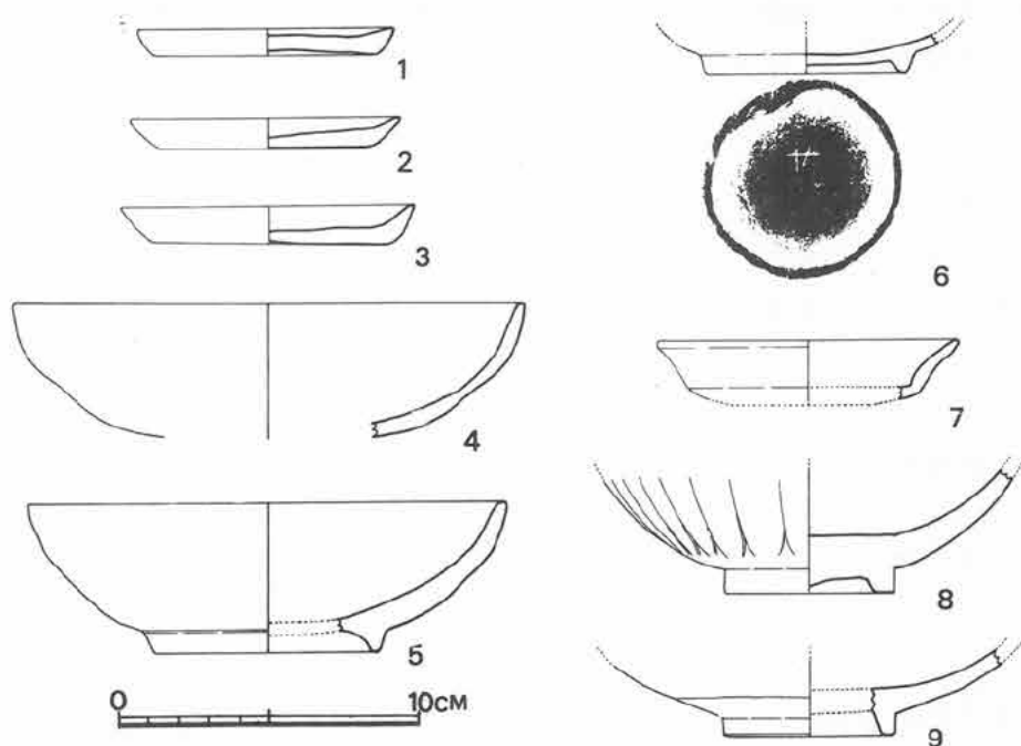
第64図 V区出土遺物実測図 (1/3)
