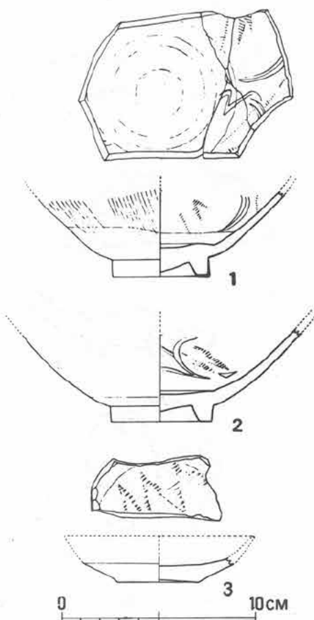
第19図 V区出土青磁実測図 (1/3)
