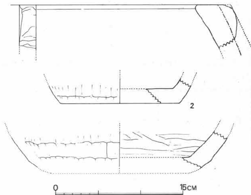
第51図 I区出土石鍋実測図 (1/3)
