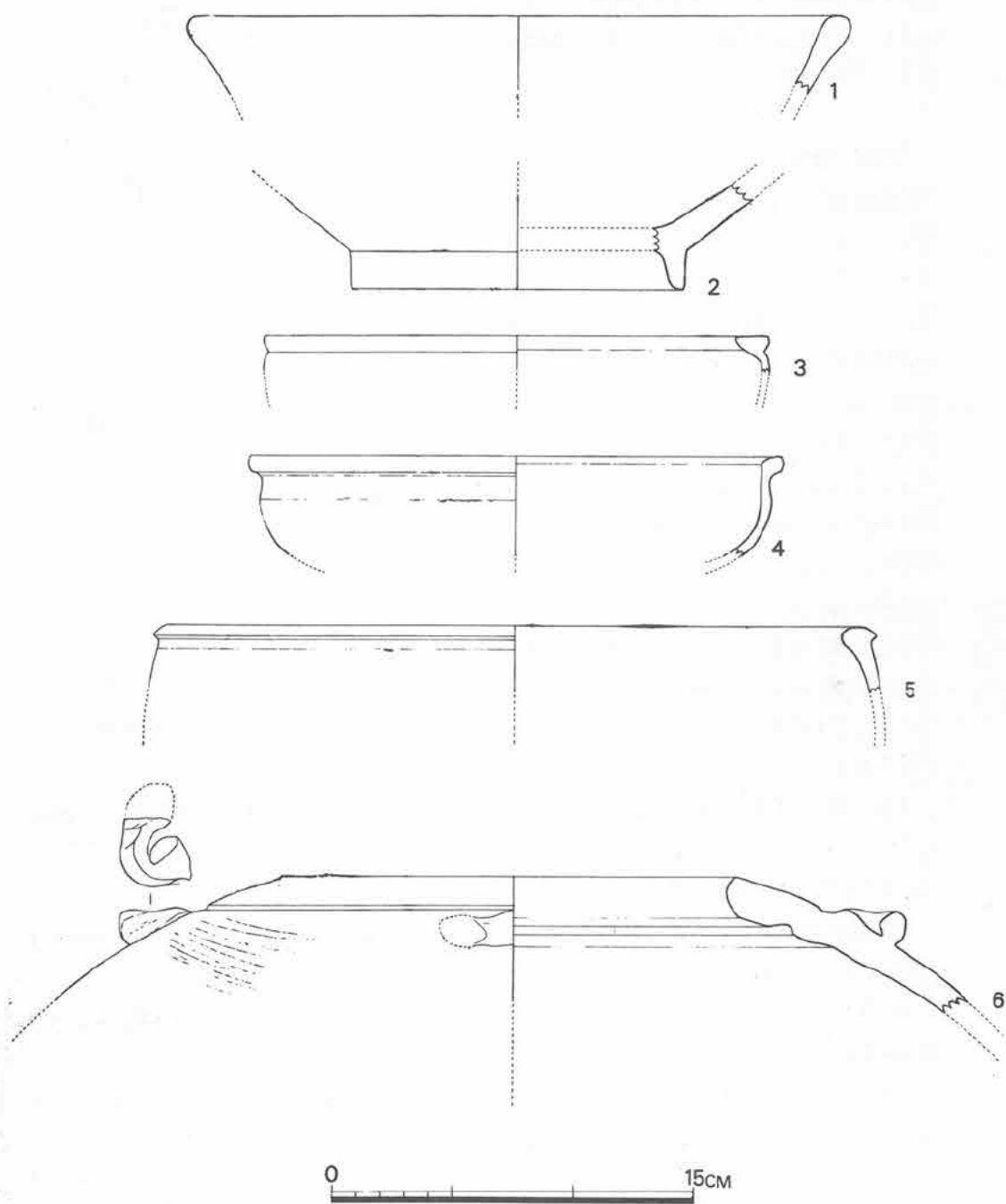
第 26 图 V 区出土陶器实测图 (1/3)
