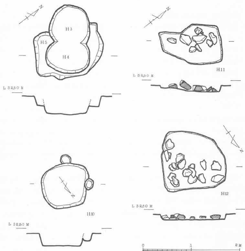
第7図 V 区 上 段 土 坑 実 測 図 (1/40)
