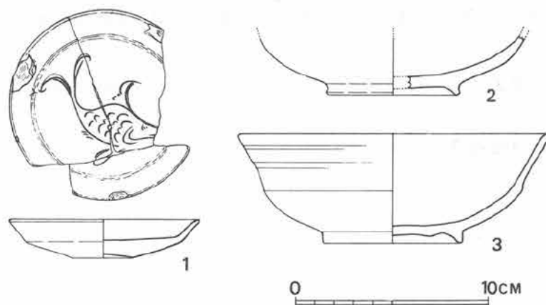
第65図 V区出土遺物実測図 (1/3)
