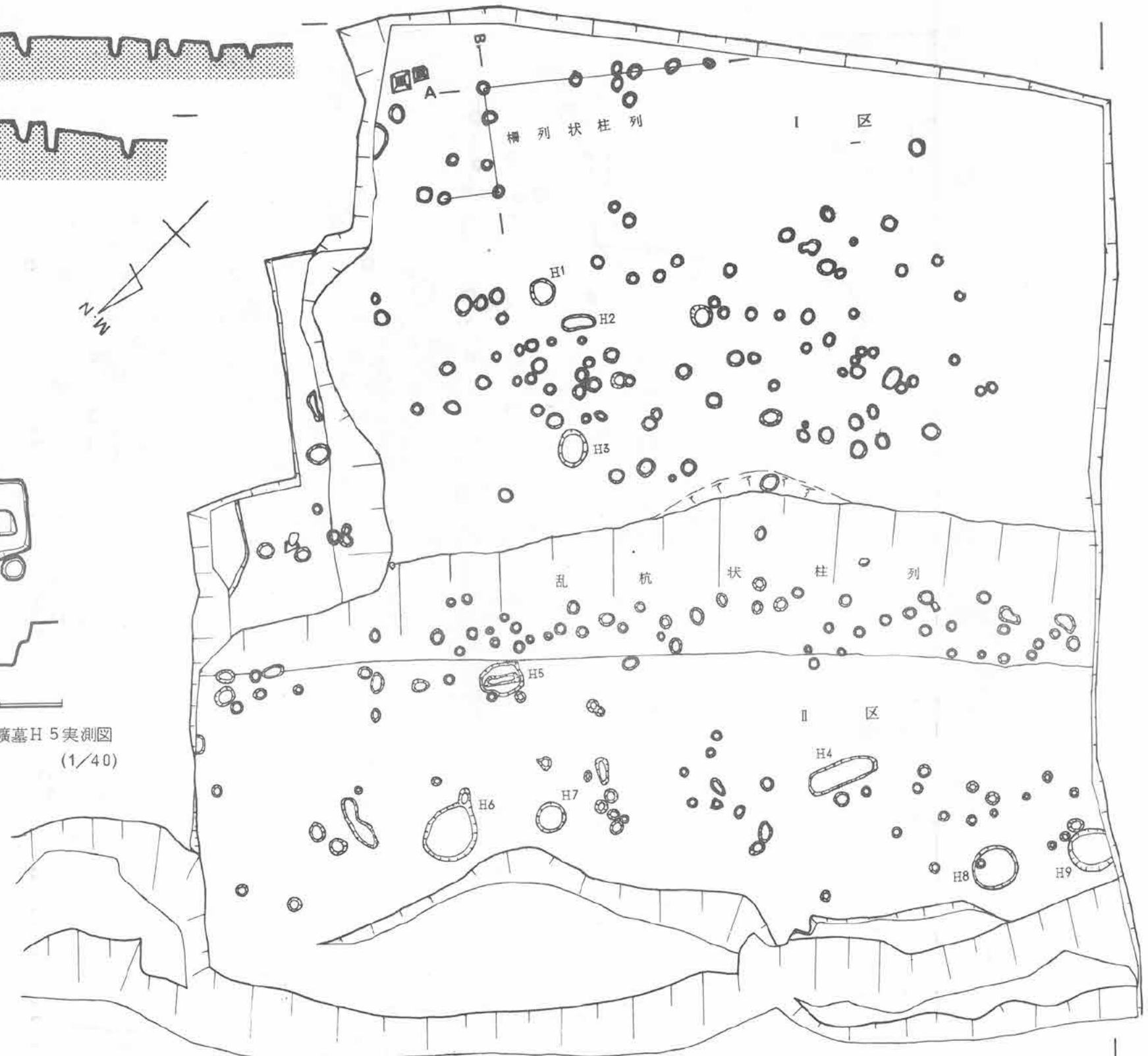
第 42 图 I 区・II 区遺構实测图 (1/100)
