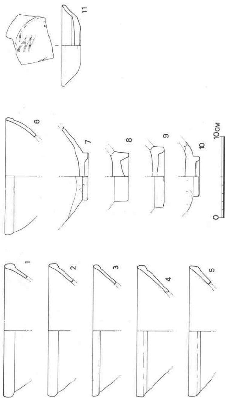
第49图 I区出土青磁·白磁夹测图 (1/3)
