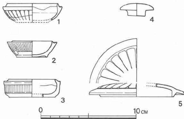
第24図 V区出土青白磁実測図 (1/3)
