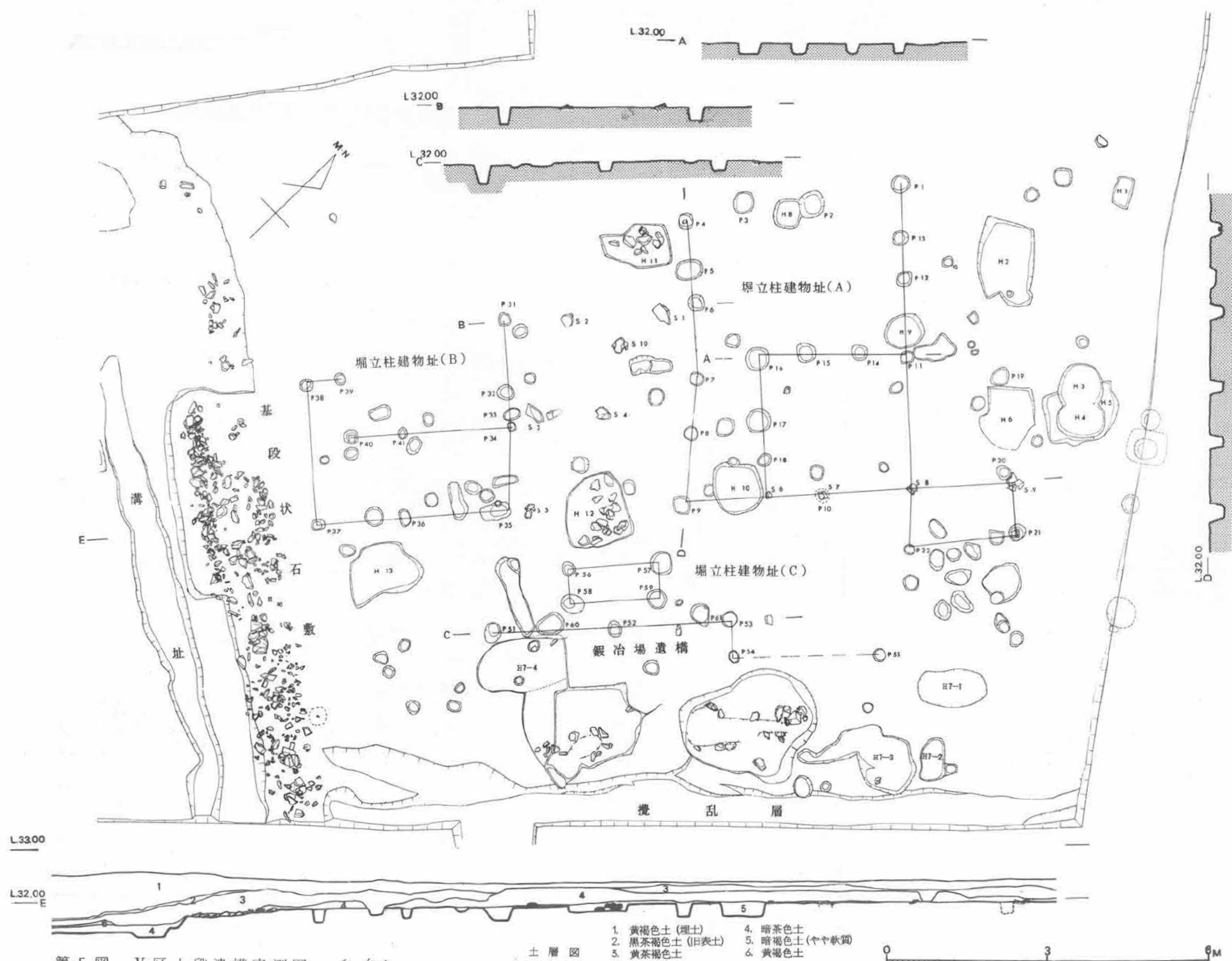
第5図 V区上段遺構実測図 (1/80)
