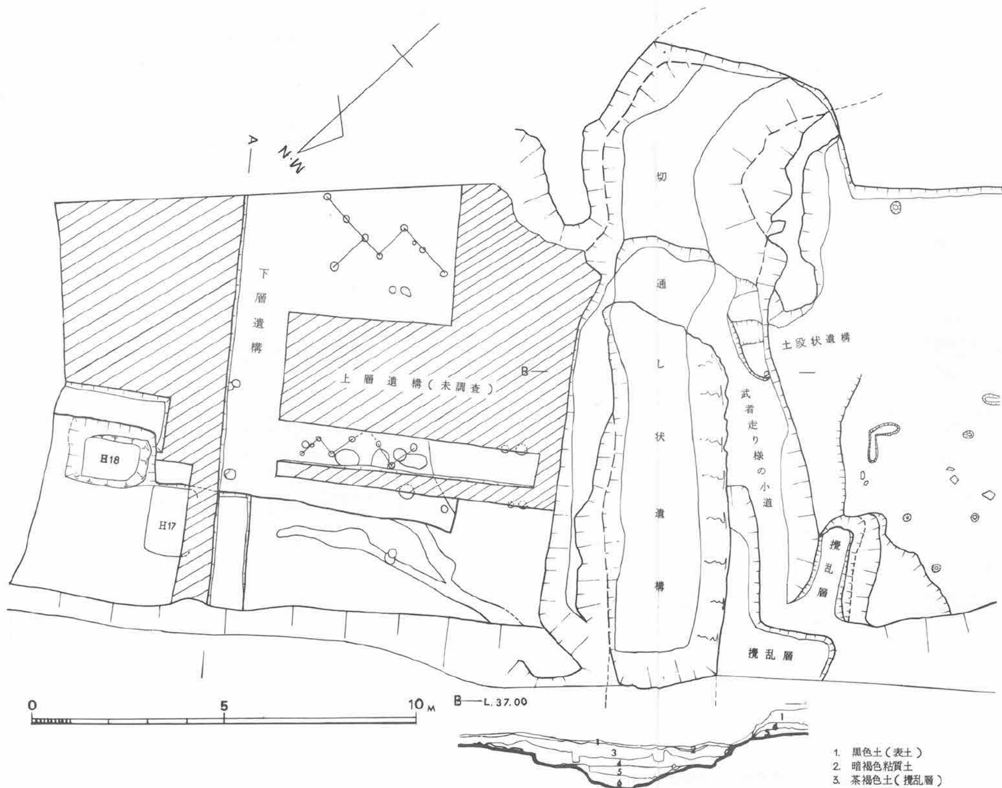
第47図 V区下層遺構実測図 (1/100)
