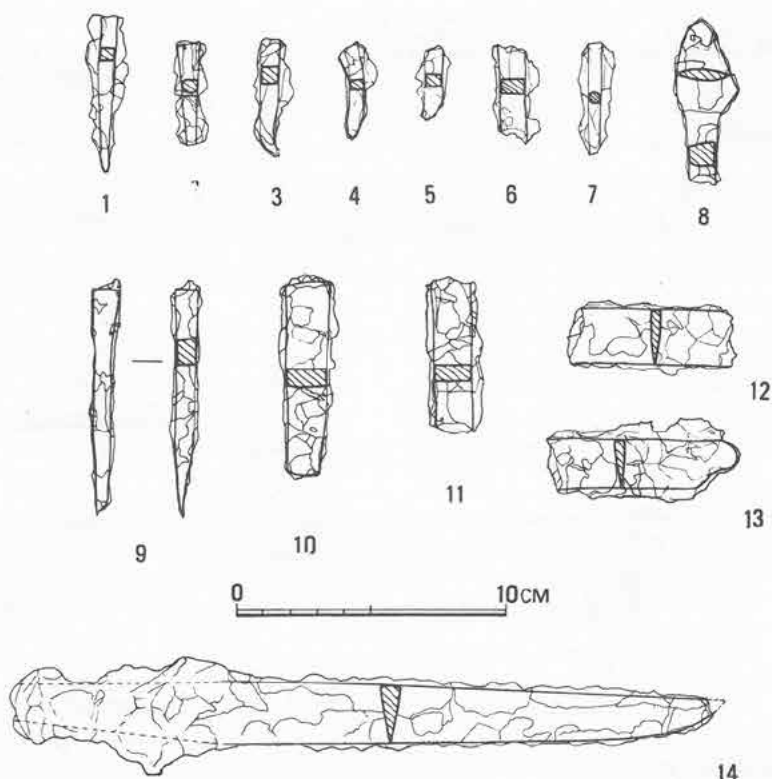
第 33 図 V 区出土鉄器実測図 (1/3)
