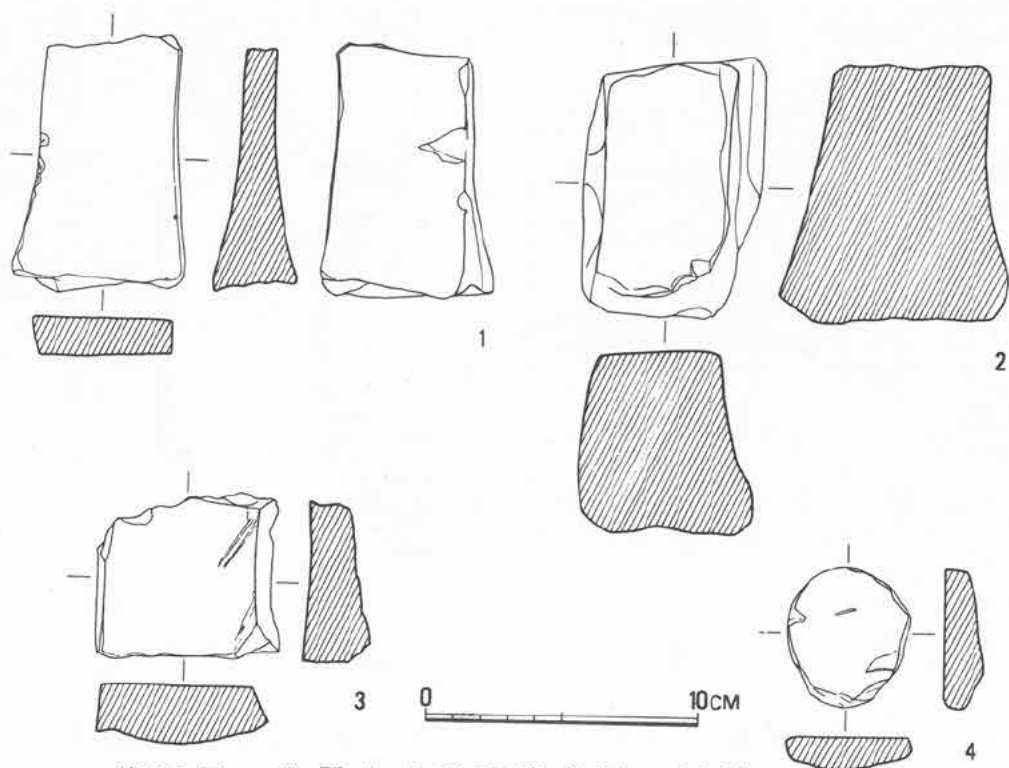
第30图 V区出土石鉢実測図 (1/3)
