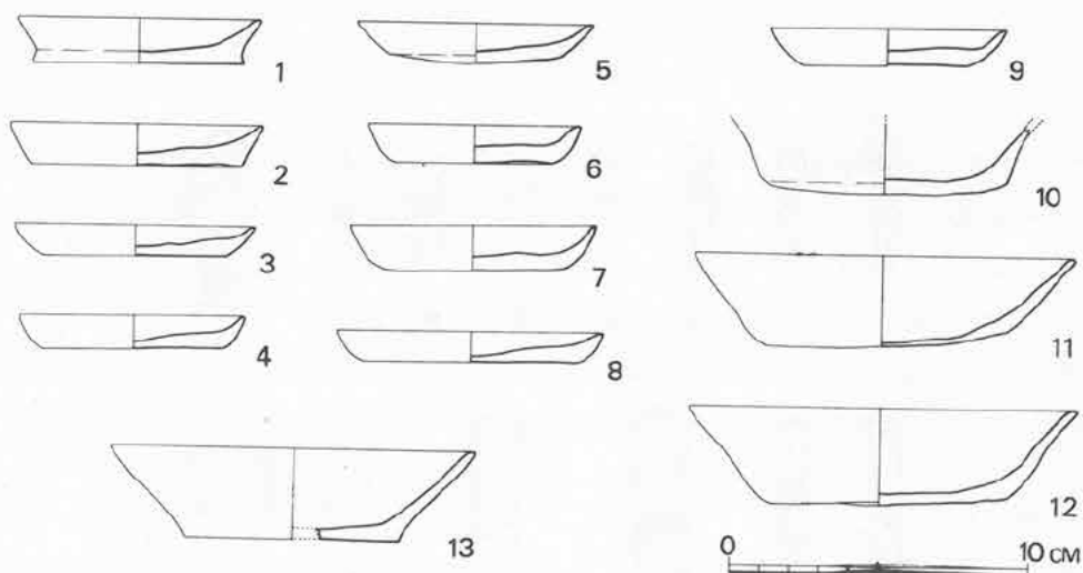
第35图 VI区出土土師器実測図 (1/3)
