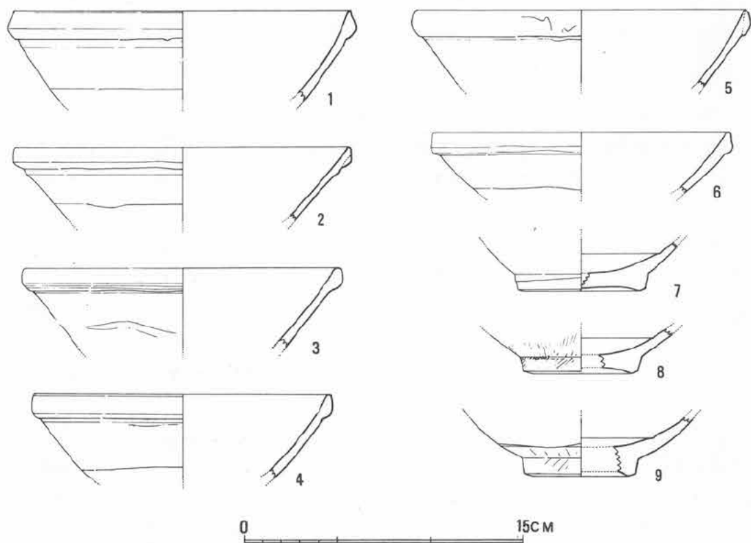
第21图 V区出土白磁夹测图 (1/3)
