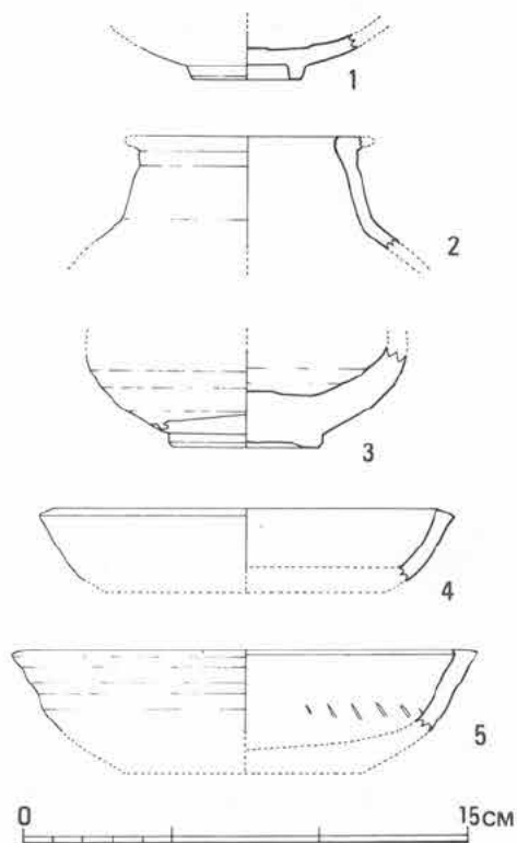
第27図 V区出土陶器実測図（1/3）
