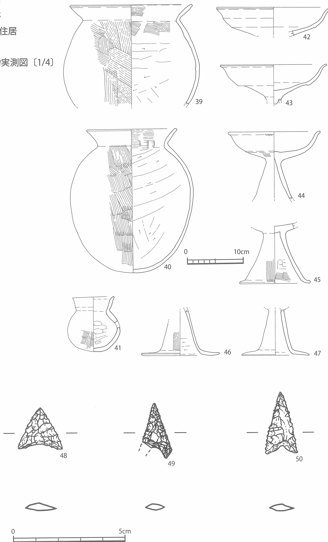
第17図 川原遺跡 2,4号竪穴住居 (SB-02,04) 出土石製品実測図〔1/1〕
