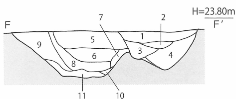
第60図 打越遺跡3地点 17号溝状遺構 (SD-17) 土層断面図 [1/40]
