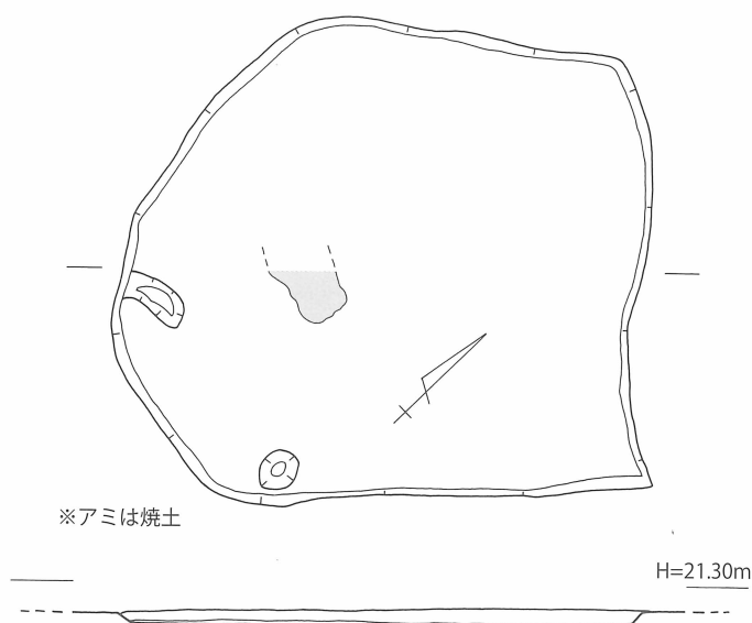
第10図 川原遺跡 1号土坑 (SK-01) 実測図 [1/40]
