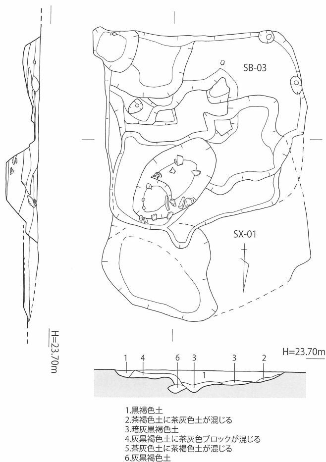
第24図 新替遺跡 3号竪穴住居(SB-03)
