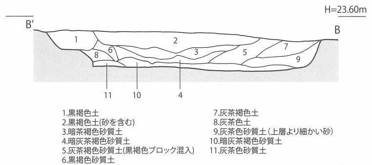
第33図 新替遺跡 1号溝状遺構 (SD-01) 東側土層断面図〔1/40〕
