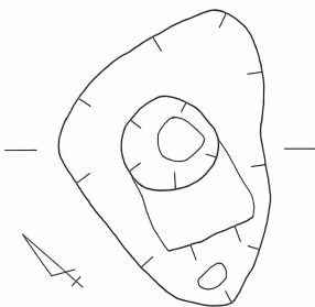
第30図 新替遺跡 3号土壙 (SK-03) 実測図〔1/40〕
