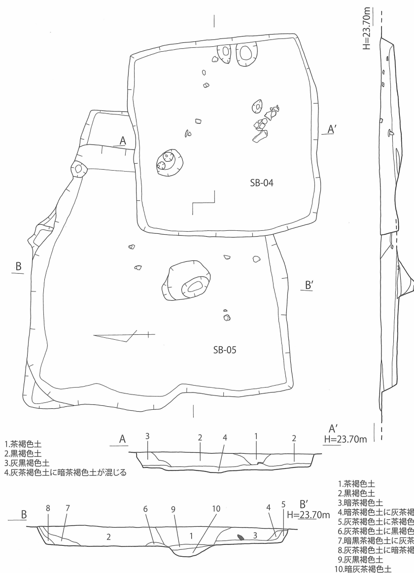
第25図 新替遺跡 4,5号竪穴住居 (SB-04,05) 実測図 [1/60]
