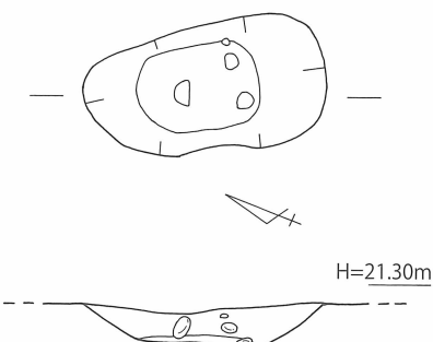
第12図 川原遺跡 3号土坑 (SK-03) 実測図 [1/40]
