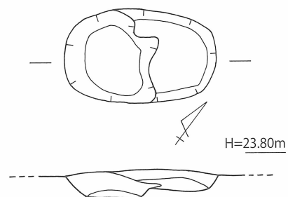
第48図 打越遺跡3地点 1号土壙 (SK-01) 実測図 [1/40]
