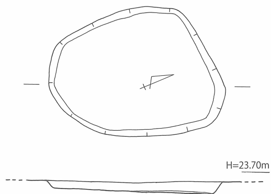
第50図 打越遺跡3地点 3号土壙 (SK-03) 実測図 [1/40]
