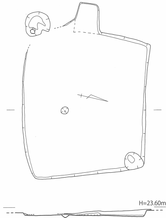
第21図 新替遺跡 1号竪穴住居 (SB-01) 実測図〔1/60〕
