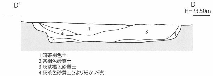
第33図 新替遺跡 1号溝状遺構 (SD-01) 東側土層断面図〔1/40〕
