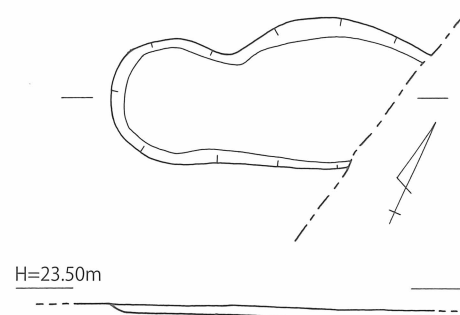
第41図 打越遺跡2地点 1号 不明遺構(SX-01)実測図〔1/40〕
