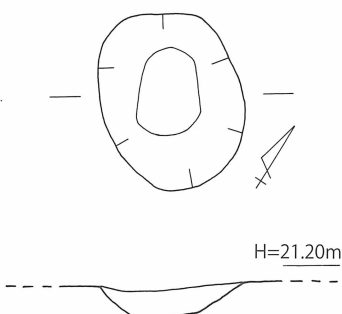
第13図 川原遺跡 4号土坑 (SK-04) 実測図 [1/40]
