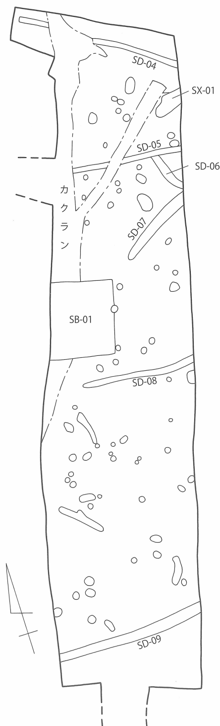
第38図 打越遺跡2地点 遺構配置図 [1/200]
