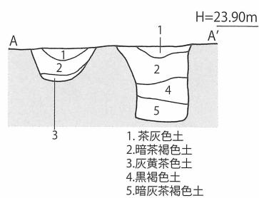
第54図 打越遺跡3地点 6号土壌 (SK-06) 実測図〔1/40〕
