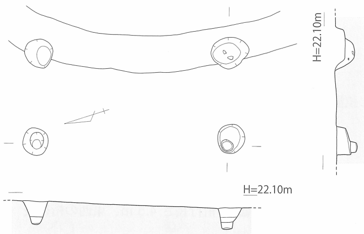
第40図 大坪・前田遺跡4地点 掘立柱建物 (S B 1 5) 実測図 [1/80]
