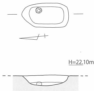
第72図 大坪・前田遺跡4地点 土壇 (SK23) 実測図
