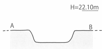
第4図 上島町・日津町遺跡 溝A—B (S D 0 1) 断面図 〔1 / 4 0〕
