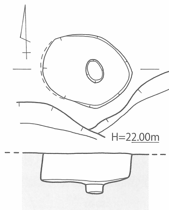
第29図 大坪・前田遺跡2地点 土壌(SK04)実測図 [1/40]
