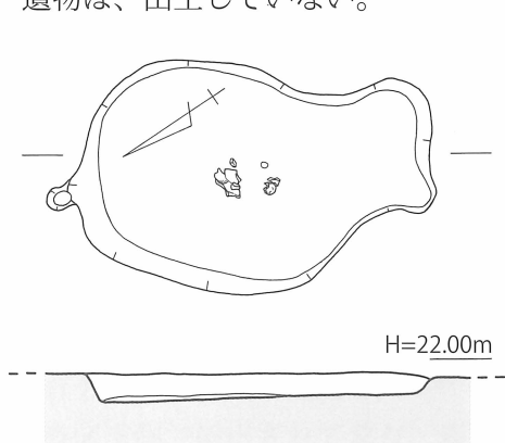
第26図 大坪・前田遺跡2地点 土壌(SK01)実測図 [1/40]
