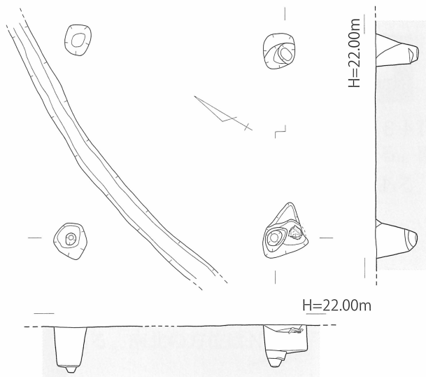
第 5 0 図 大坪・前田遺跡 4 地点 掘立柱建物 (S B 3 4) 実測図〔1/80〕
