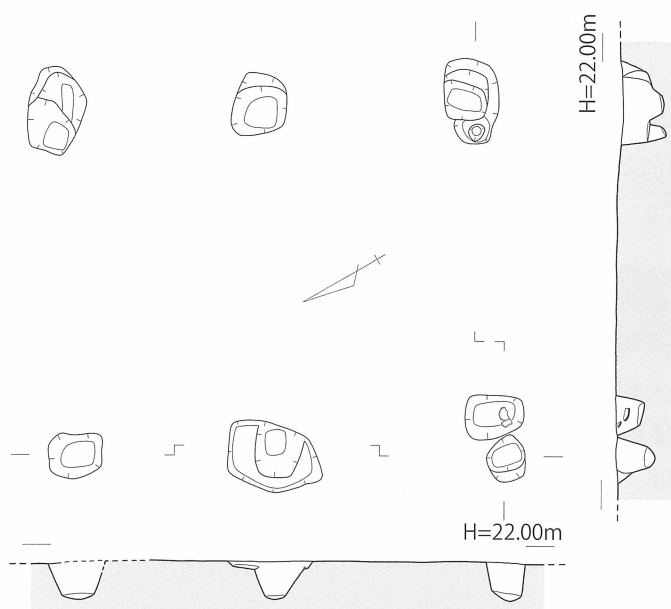
第46図 大坪・前田遺跡4地点 掘立柱建物 (SB29) 実測図 [1/80]
