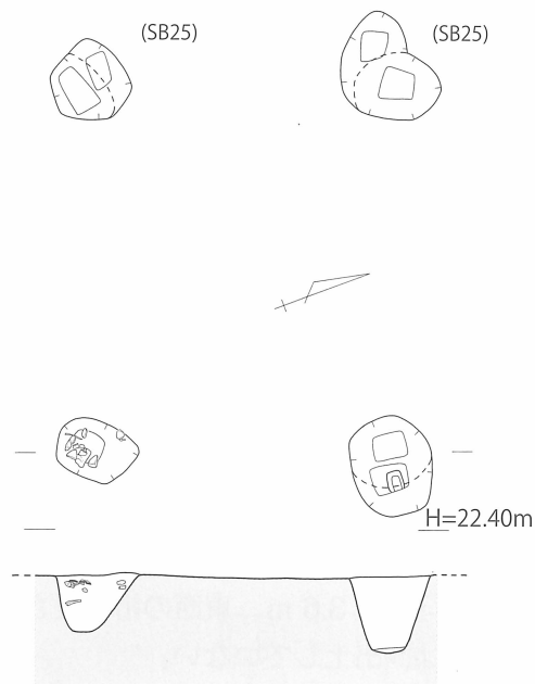
第42図 大坪・前田遺跡4地点 掘立柱建物 (S B 2 4) 実測図 [1/80]
