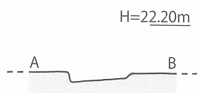
第17図 上島町・日津町遺跡 溝A—B (SD10) 断面図 〔1/40〕
