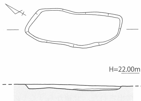
第73図 大坪・前田遺跡4地点 土壇 (SK25) 実測図 [1/40]
