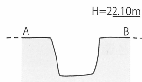
第18図 上島町・日津町遺跡 溝A—B (SD11) 断面図 〔1/40〕
