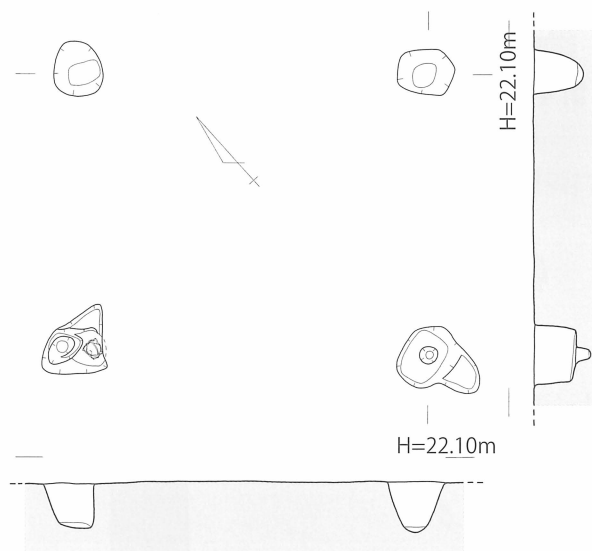
第 5 1 図 大坪・前田遺跡 4 地点 掘立柱建物 (S B 3 5) 実測図〔1/80〕
