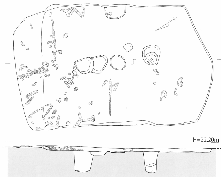
第58図 大坪・前田遺跡4地点竪穴住居 (SB 42) 実測図〔1/80〕
