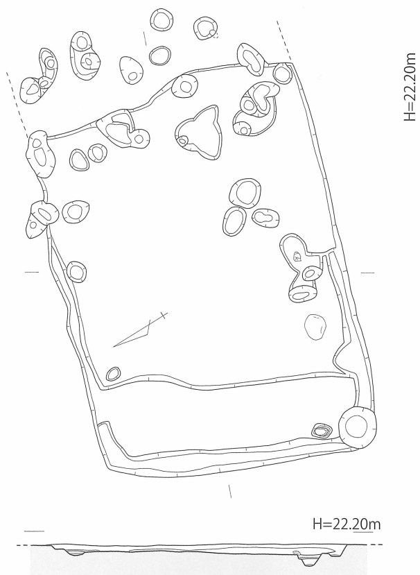
第55図 大坪・前田遺跡4地点竪穴住居 (SB38) 実測図 [1/80]
