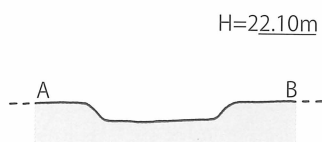
第16図 上島町・日津町遺跡 溝A—B (SD09) 断面図 〔1/40〕
