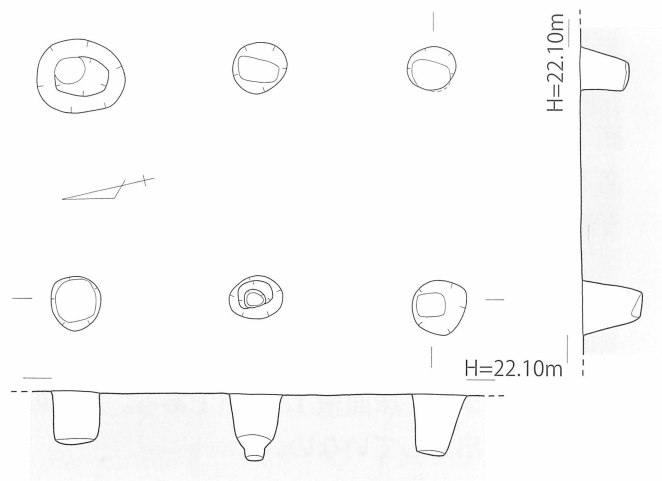
第39図 大坪・前田遺跡4地点 掘立柱建物 (S B 1 4) 実測図 [1/80]
