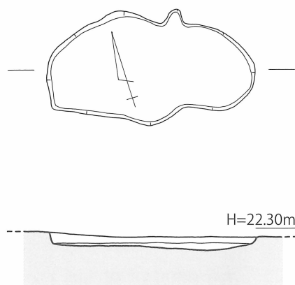
第27図 大坪・前田遺跡2地点 土壌(SK02)実測図 [1/40]
