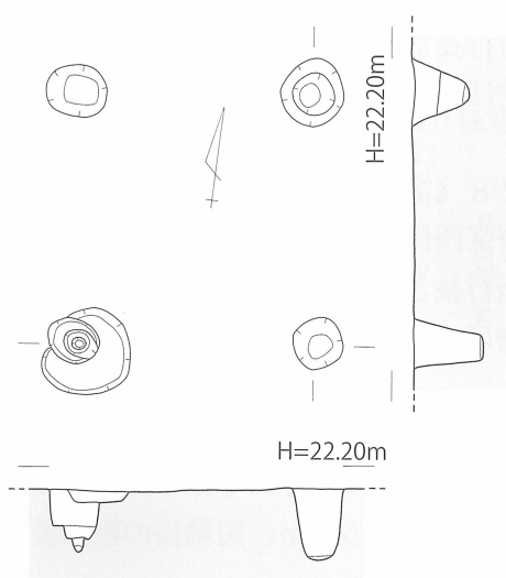
第41図 大坪・前田遺跡4地点 掘立柱建物 (S B 2 2) 実測図 [1/80]
