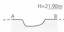
第15図 上島町・日津町遺跡 溝A—B (SD08) 断面図 〔1/40〕
