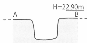
第7図 上島町・日津町遺跡 溝A—B (S D 0 3) 断面図 〔1 / 4 0〕
