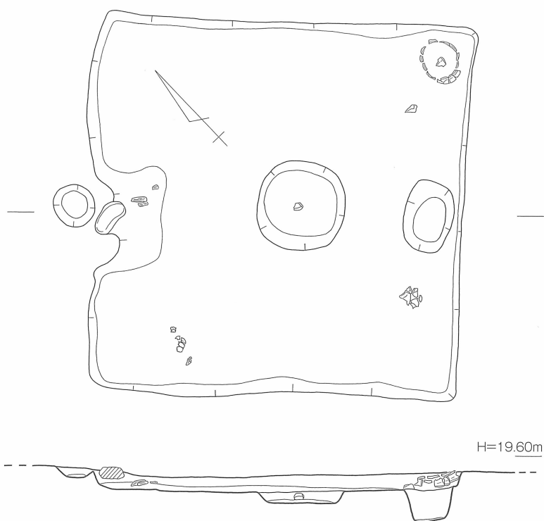
第 6 図 吉書田遺跡 1 地点 3 号竪穴住居 〔1/40〕
