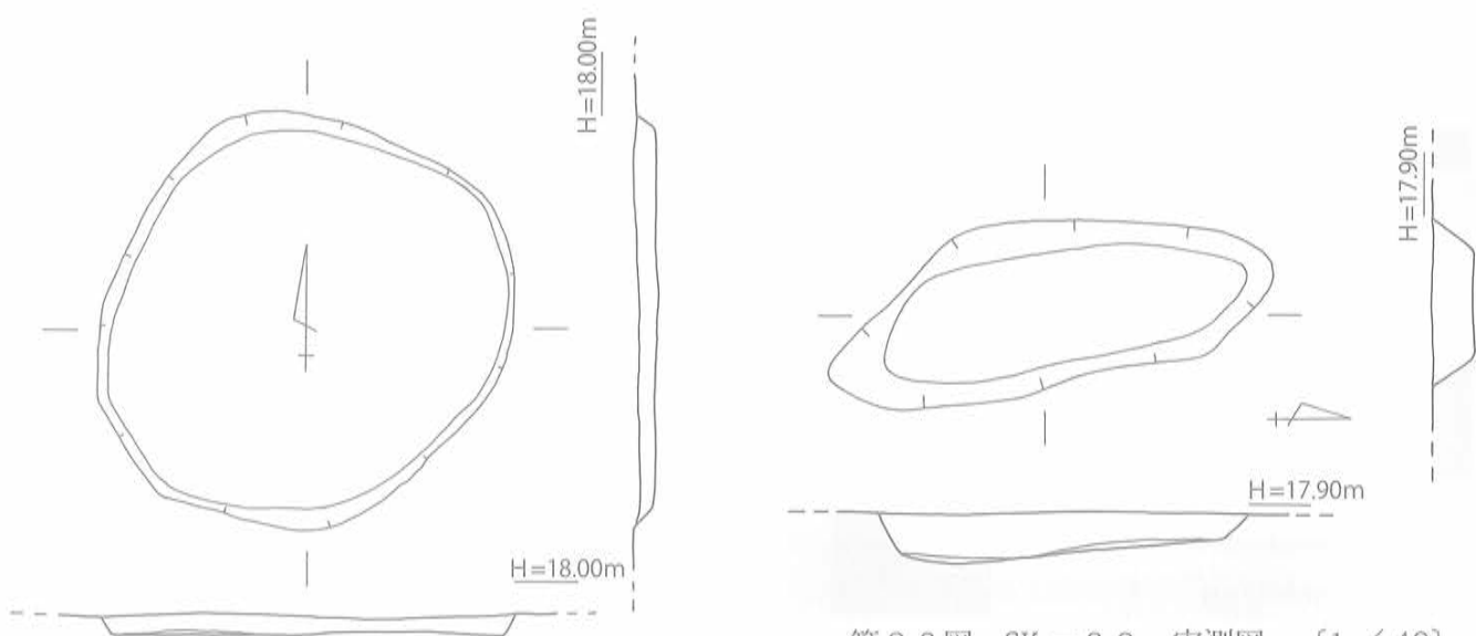
第86図 SK-60 実測図 [1/40]
