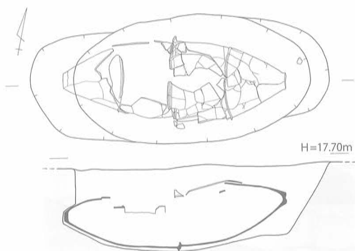
第128図 K-54 実測図 [1/30]
