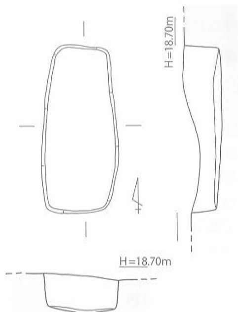
第105図 SK-123 実測図 [1/40]
