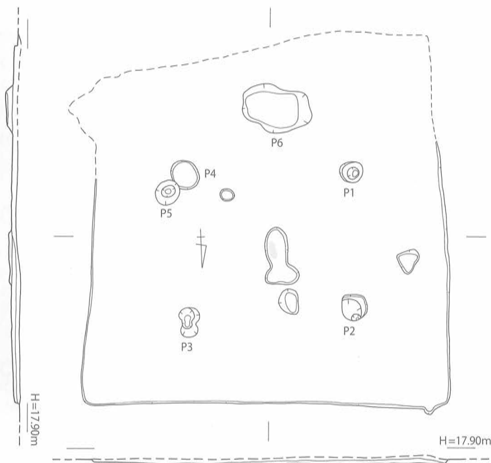
第9図 SB-06 実測図 [1/80]
