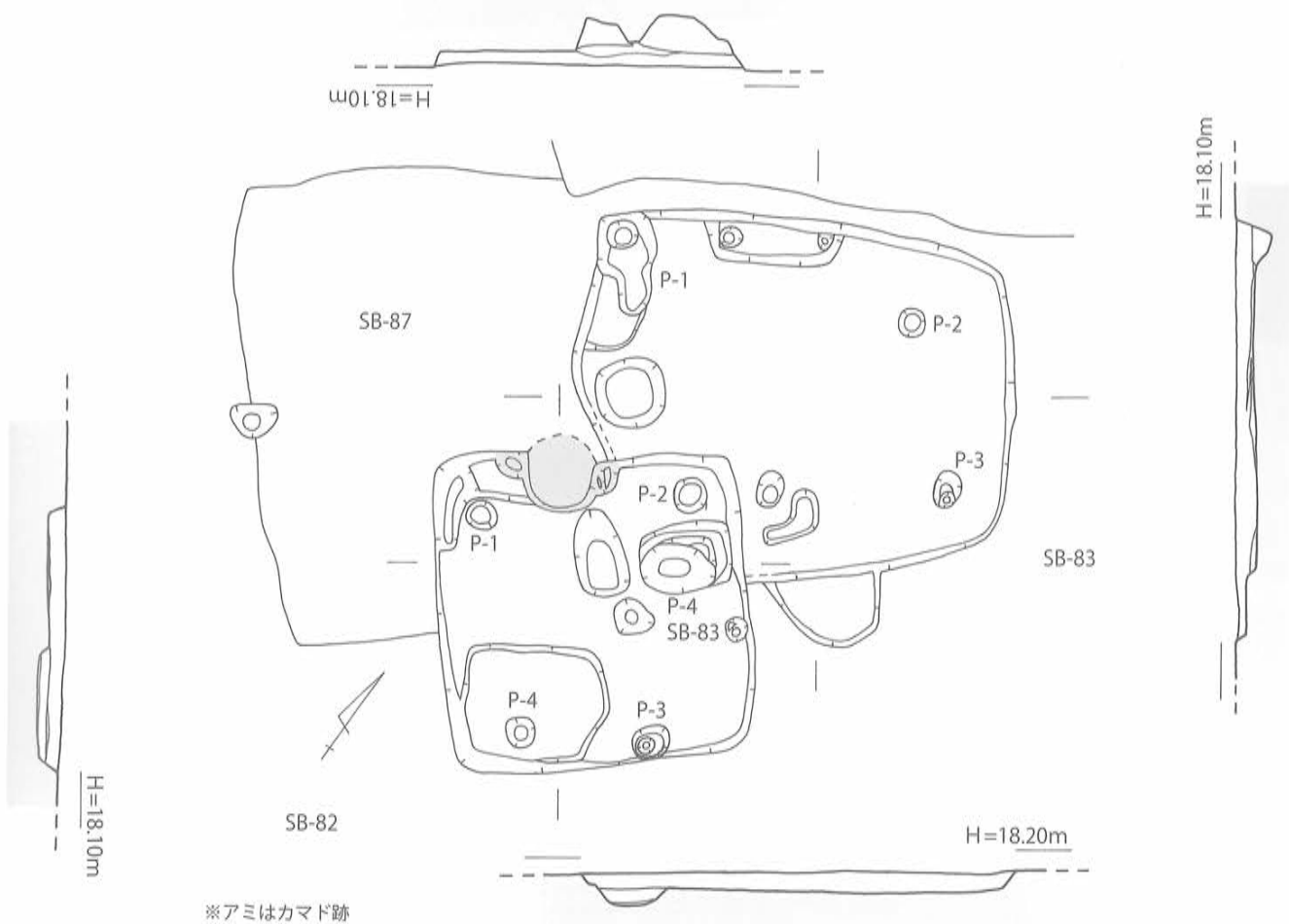
第41図 SB-82・83 実測図 [1/80]
