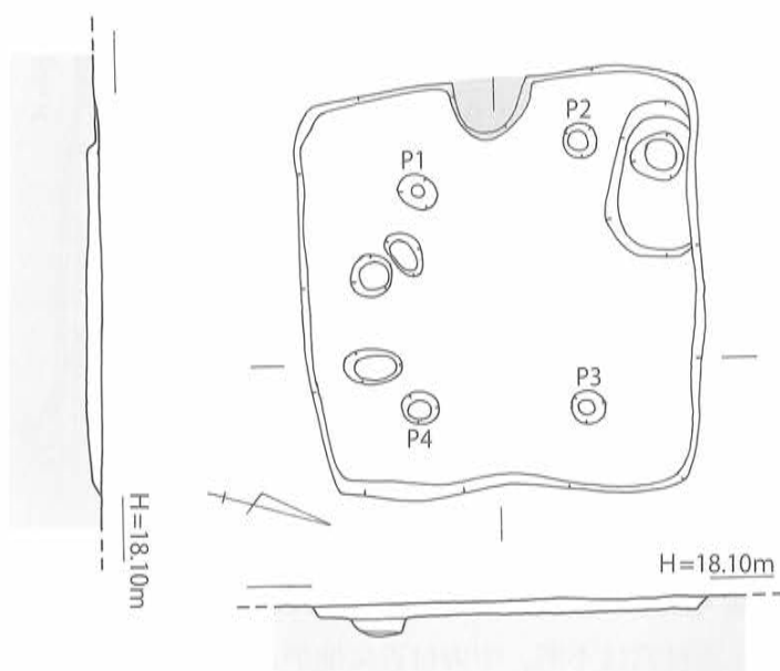
第30図 SB-45 実測図 [1/80]
