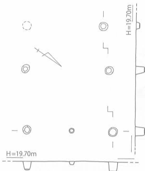
第141図 SB-06 実測図 [1/80]
