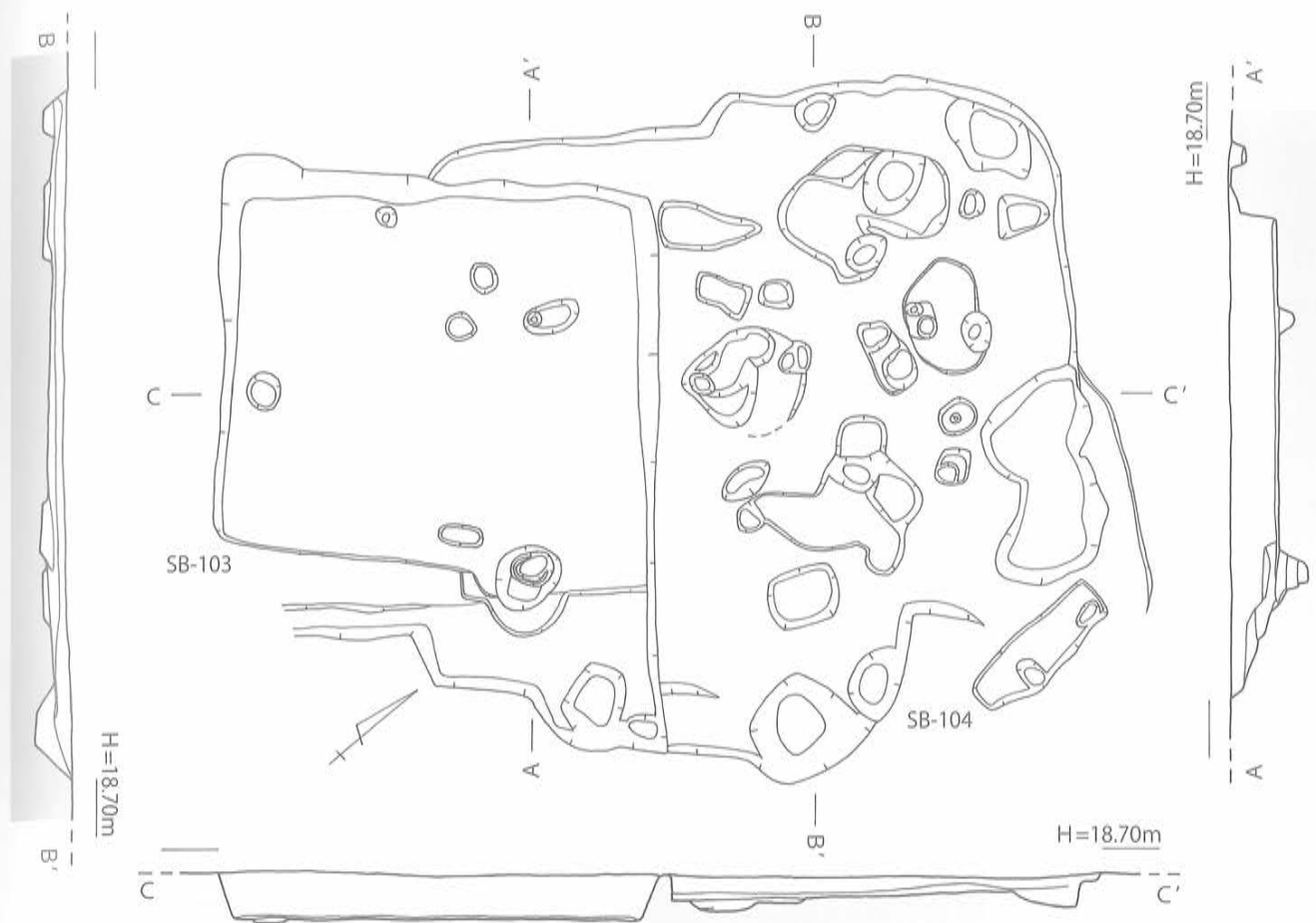
第52図 SB-103・104 実測図 [1/80]
