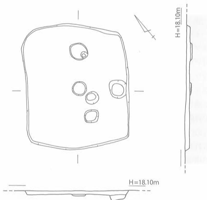
第32図 SB-50 実測図 [1/80]
