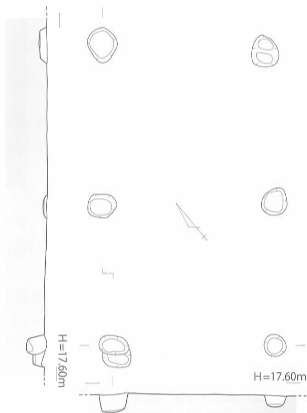
第62図 掘立柱建物 A 実測図 [1/80]
