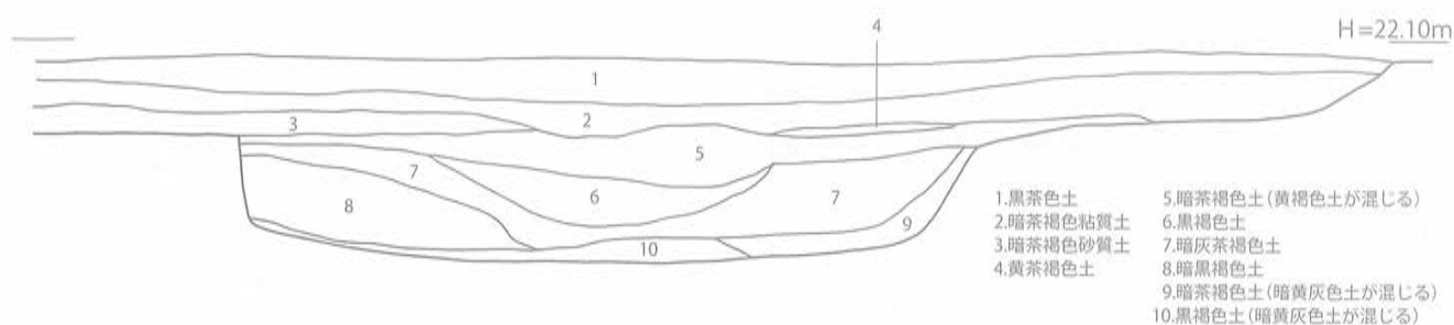
第159図 SD-01 H土層 断面実測図 [1/40]
