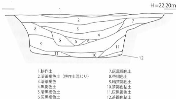
第162図 SD-11 土層断面実測図 [1/40]
