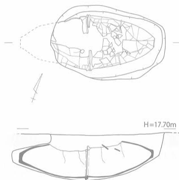
第118図 K-11 実測図 [1/30]
