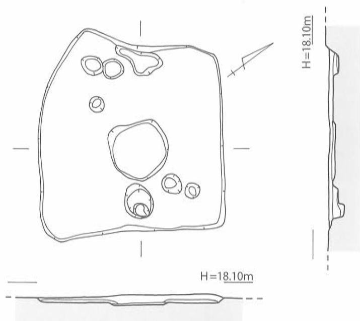
第25図 SB-38 実測図 [1/80]
