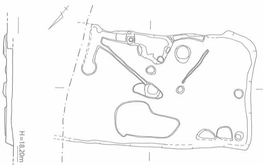
第38図 SB-75 実測図 [1/80]
