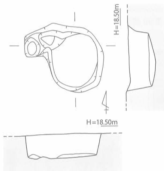
第98図 SK-107 実測図 [1/40]
