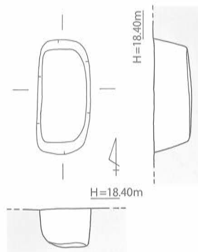
第96図 SK-100 実測図 [1/40]
