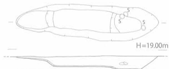
第 150 図 SK-01 実測図 [1/80]
