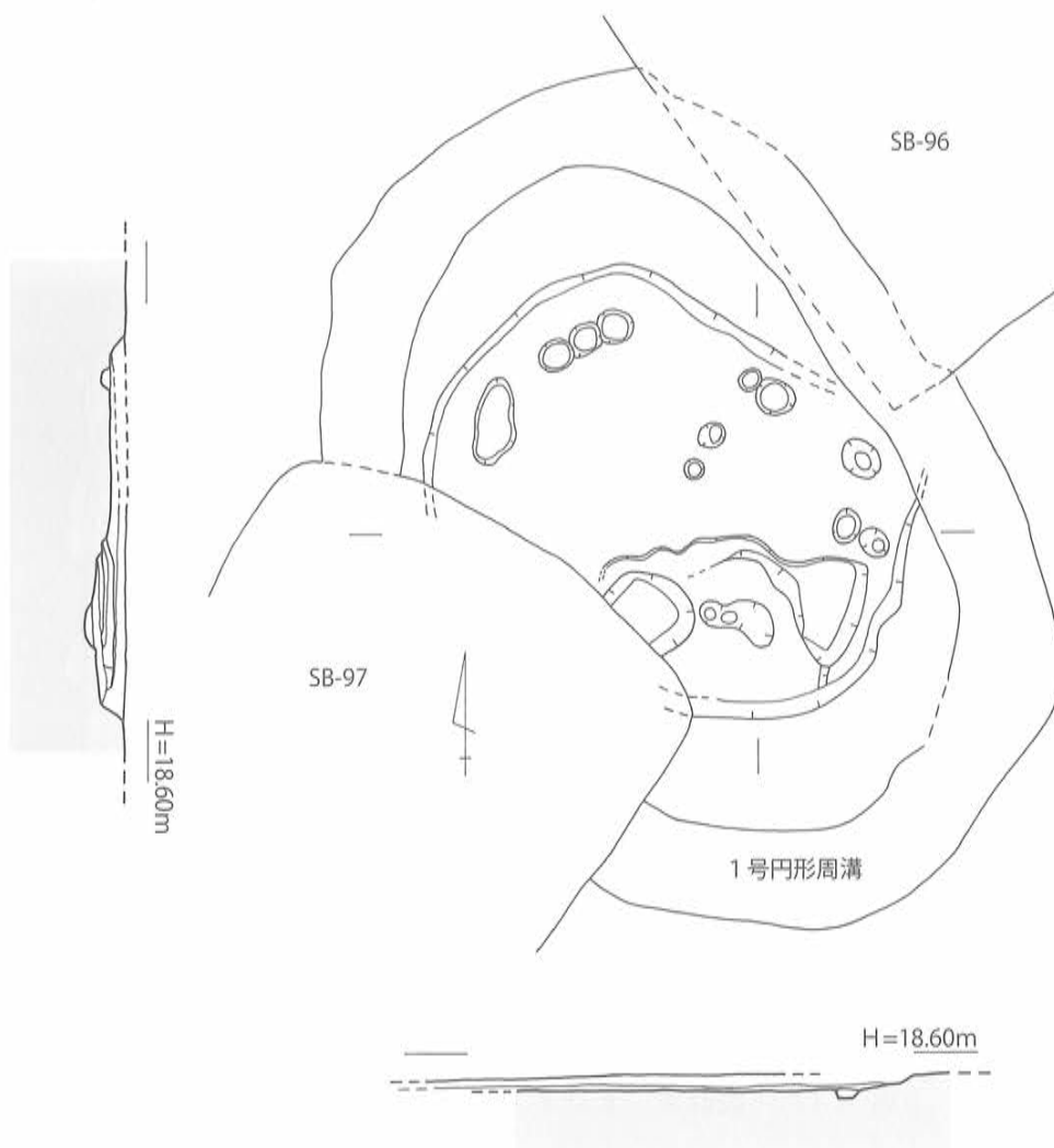
第48図 SB-98実測図 [1/80]
