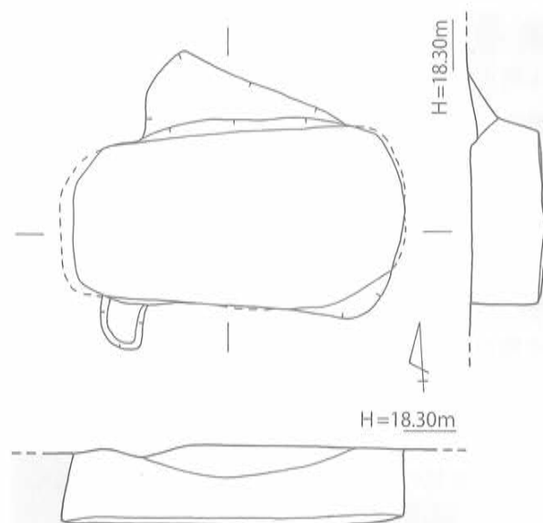
第103図 SK-120 実測図 [1/40]
