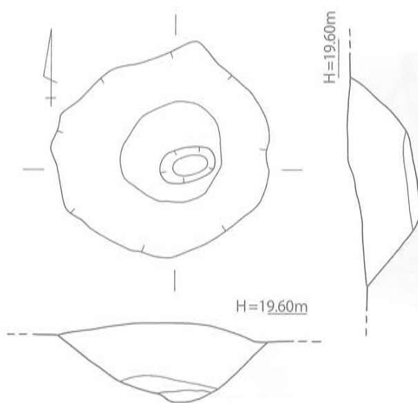
第58図 SB-122・123 実測図 [1/80]
