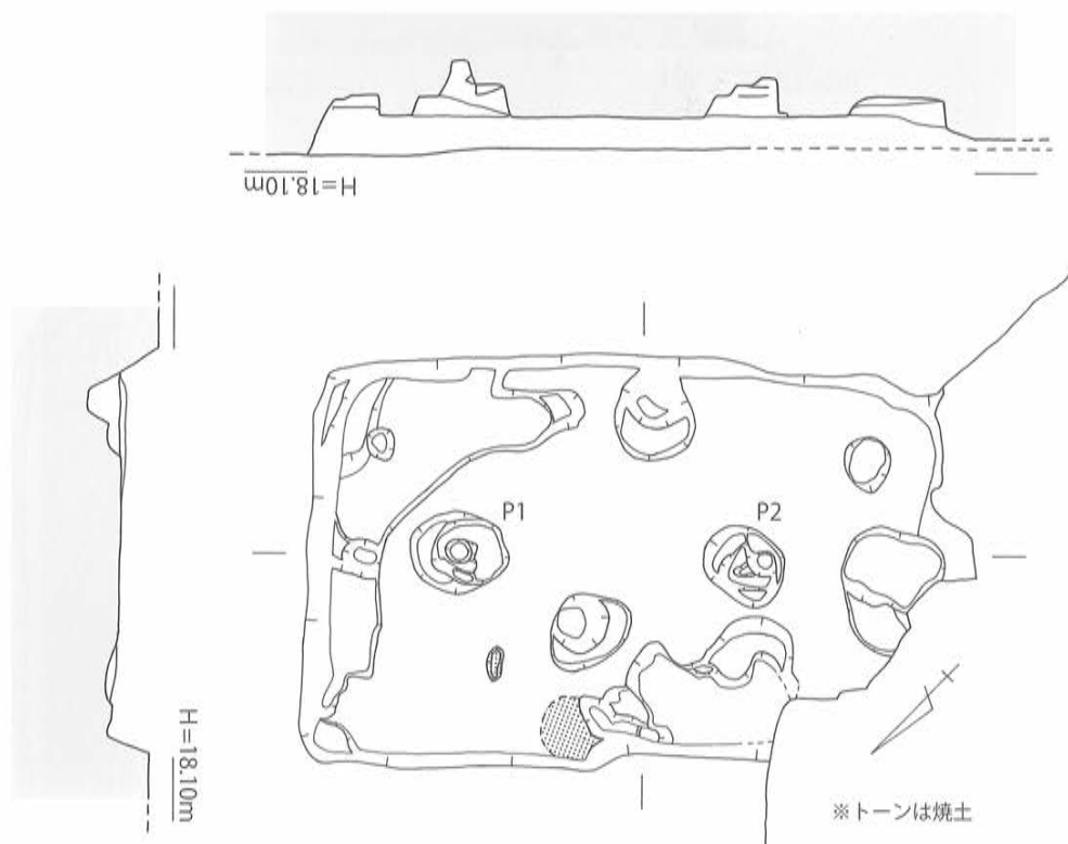
第31図 SB-49 実測図 [1/80]
