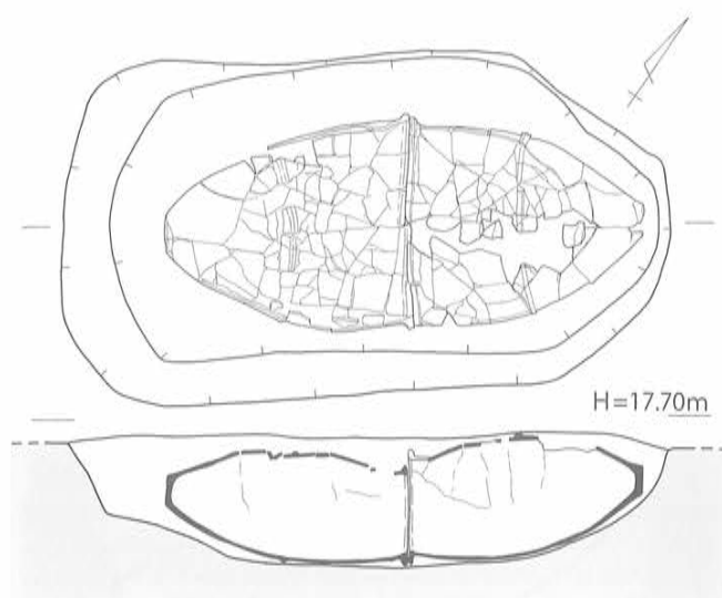
第124図 K-41 実測図 [1/30]
