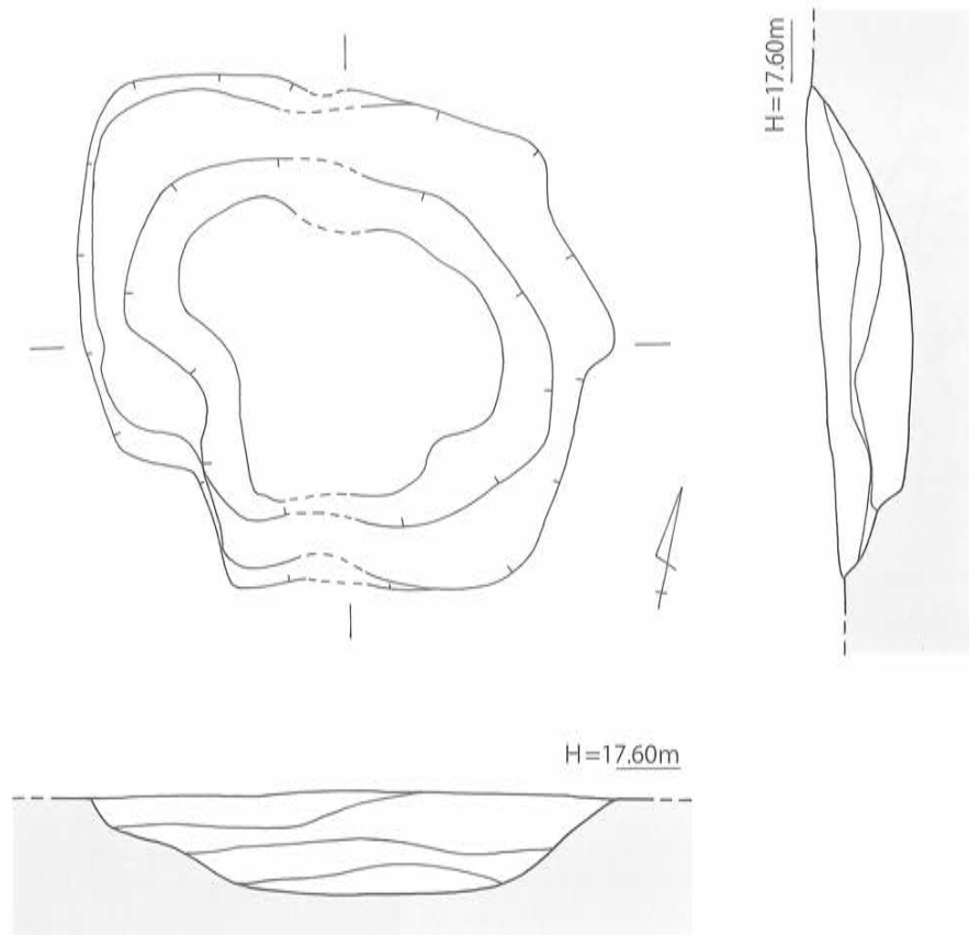
第 8 1 図 SK - 3 2 実測図 [1 / 40]
