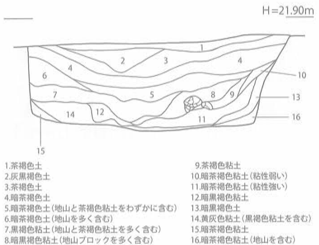
第157図 SD-01 D土層 断面実測図 [1/40]
