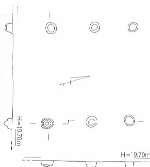
第139図 SB-04 実測図 [1/80]
