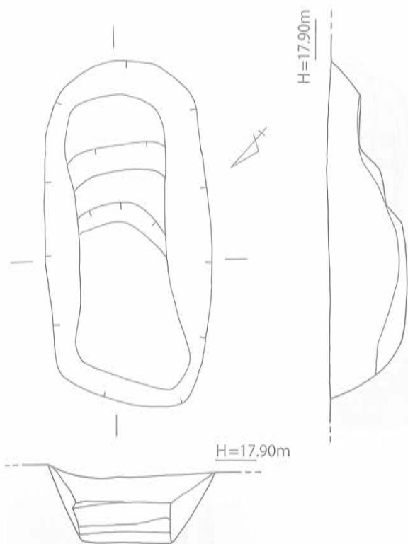
第87図 SK-62 実測図 [1/40]
