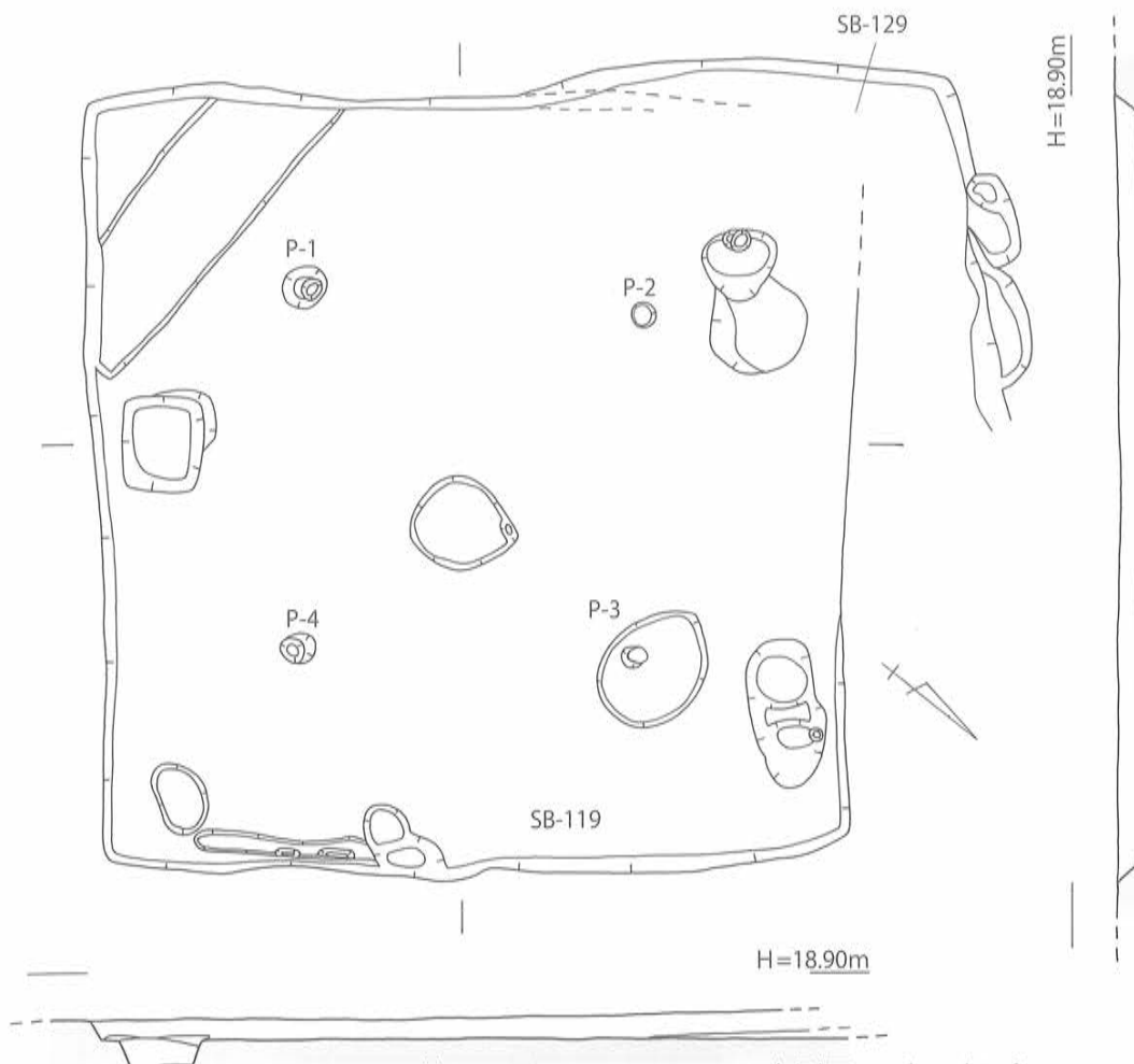
第57図 SB-119 実測図 [1/80]
