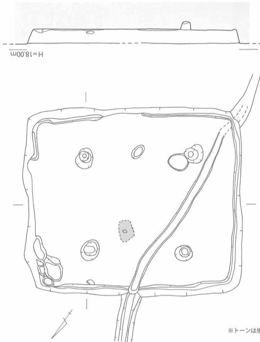
第19図 SB - 28 実測図 [1 / 80]
