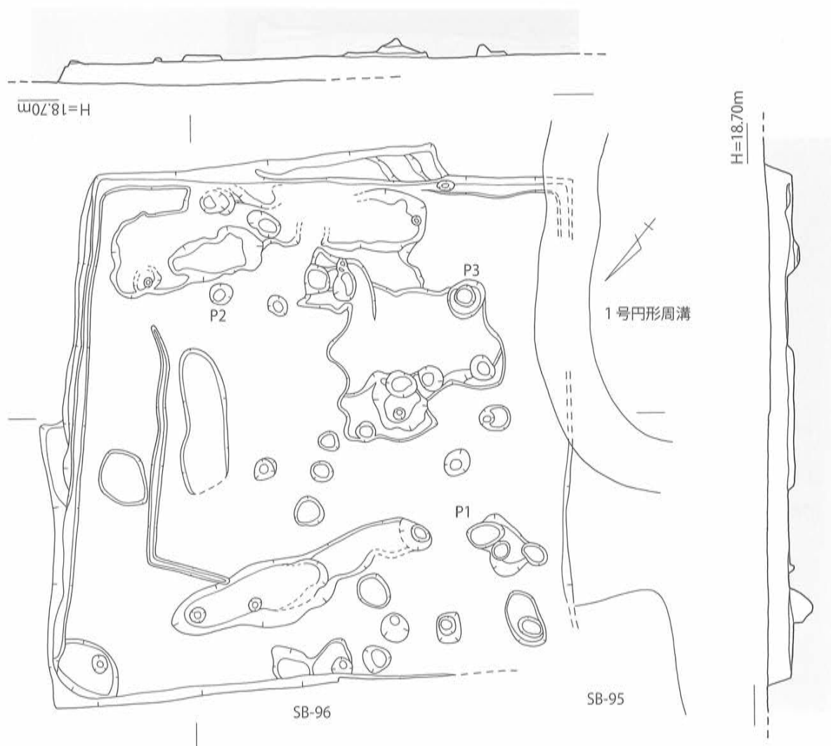
第46図 SB-96 実測図 [1/80]
