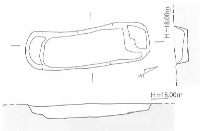
第95図 SK-88 実測図 [1/40]
