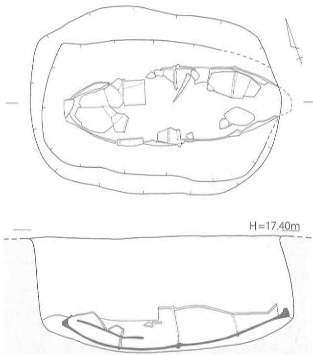
第132図 K-77 実測図 [1/30]
