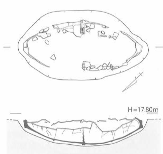
第123図 K-35 実測図 [1/30]
