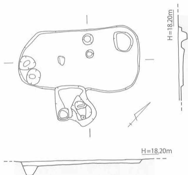
第40図 SB-80 実測図 [1/80]
