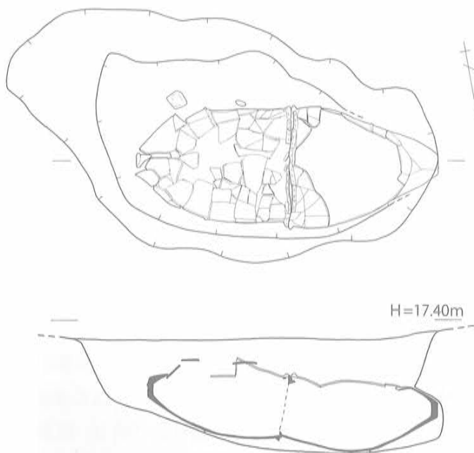
第131図 K-76 実測図 [1/30]
