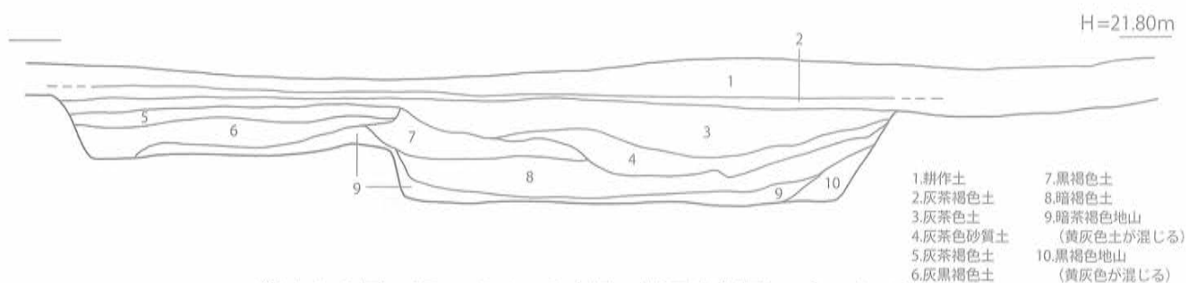
第160図 SD-01 J土層 断面実測図 [1/40]
