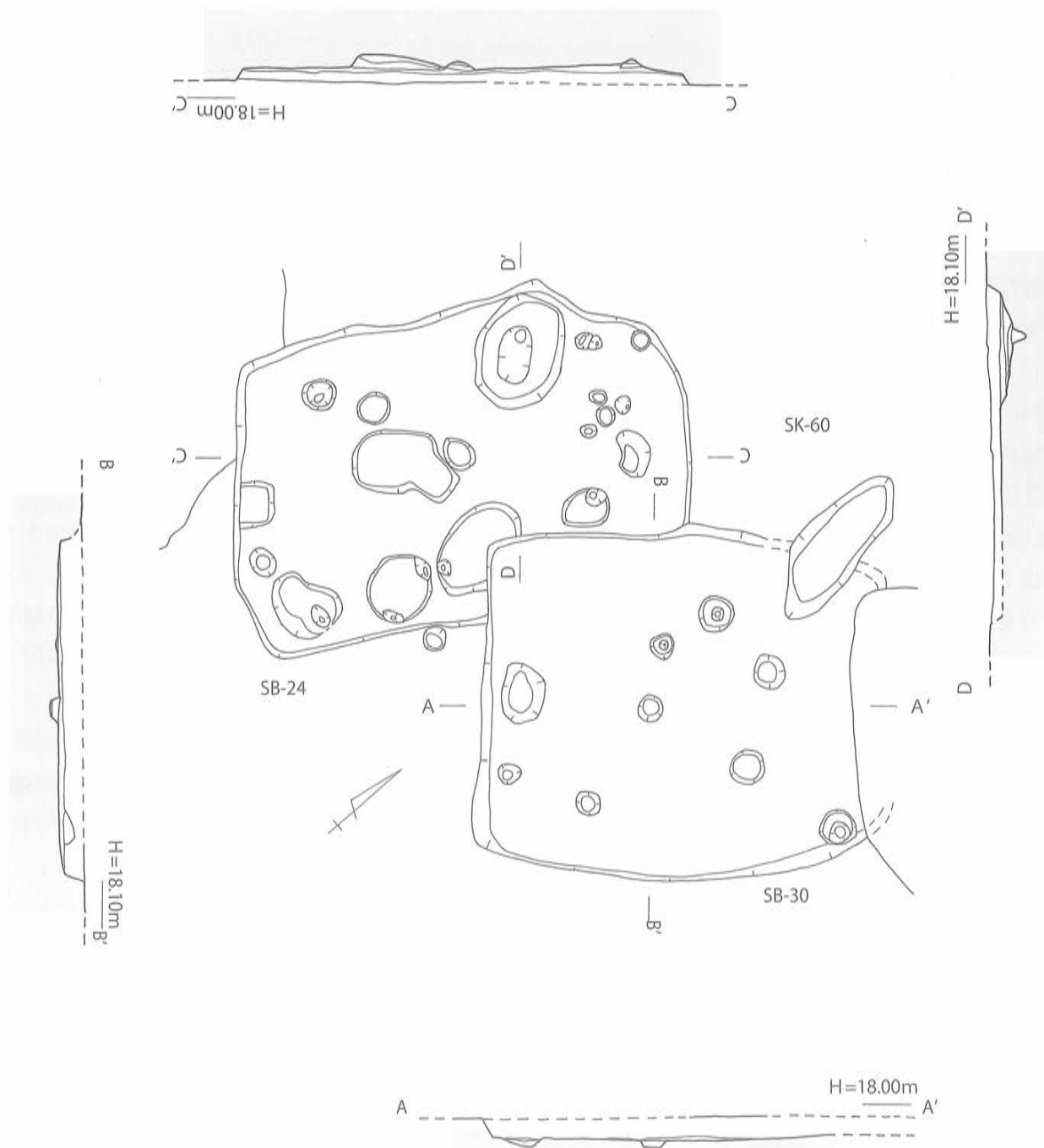
第16図 SB-24・30 実測図 [1/80]
