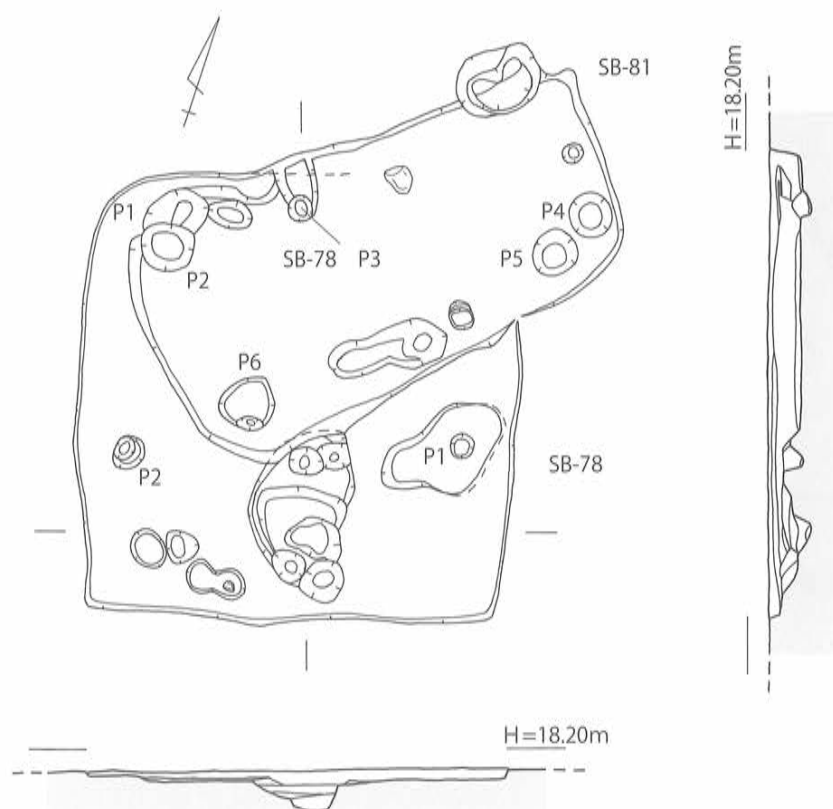
第39図 SB-78・81 実測図 [1/80]
