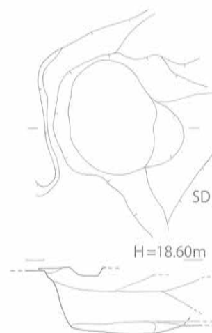
第 151 図 SK-02 実測図 [1/80]
