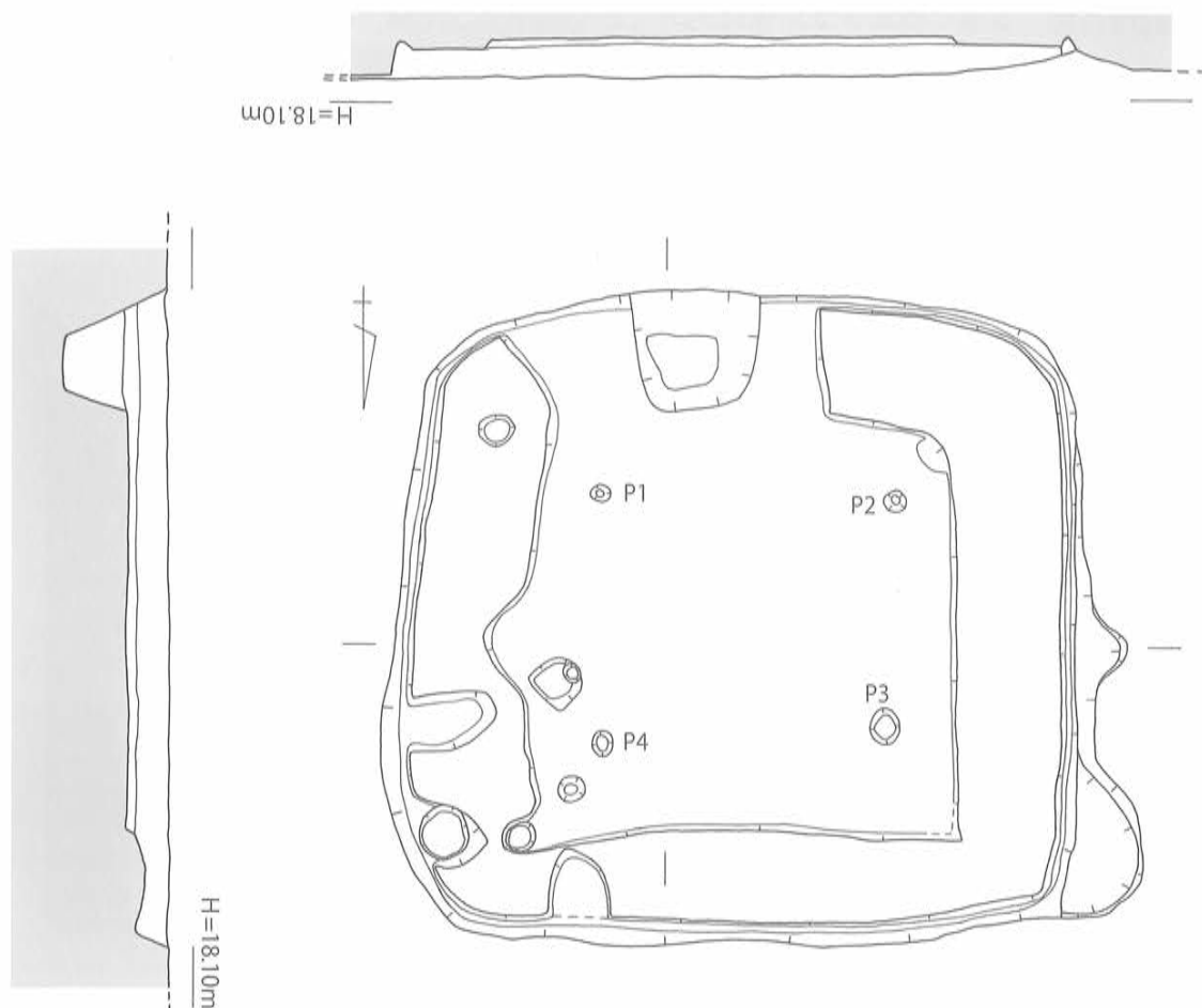
第29図 SB-43 実測図 [1/80]
