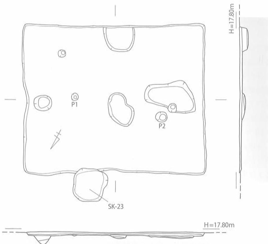
第10図 SB-07 実測図 [1/80]
