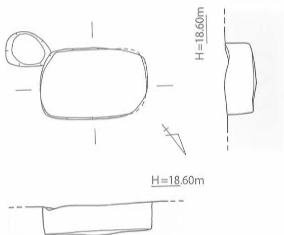
第70図 SK-03 実測図 [1/40]
