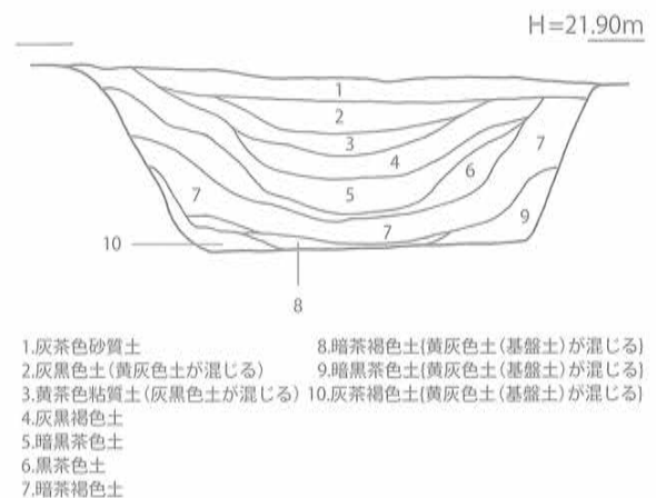
第158図 SD-01 E土層 断面実測図 [1/40]
