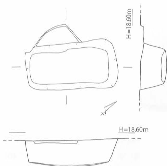
第102図 SK-114 実測図 [1/40]
