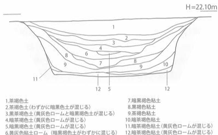
第155図 SD-01 B土層 断面実測図
