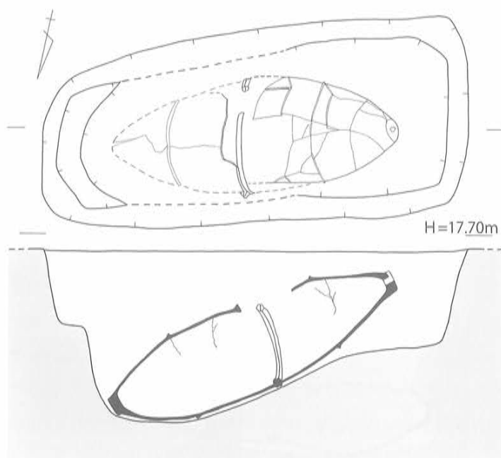
第126図 K-47 実測図 [1/30]
