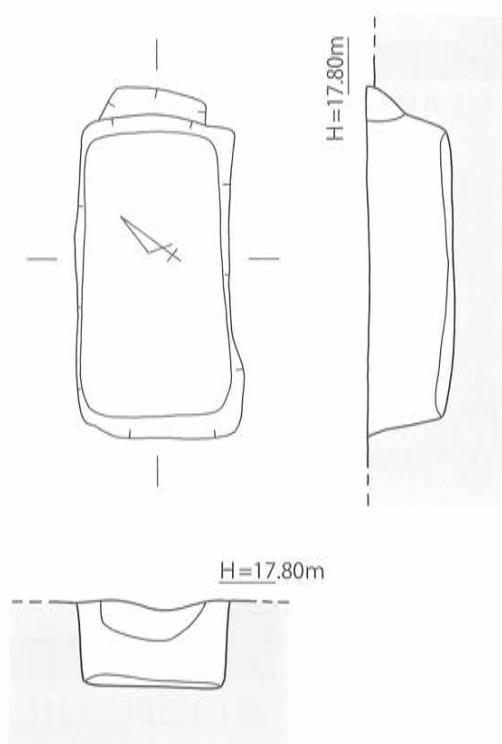
第112図 11号土壙墓 実測図 [1 / 40]
