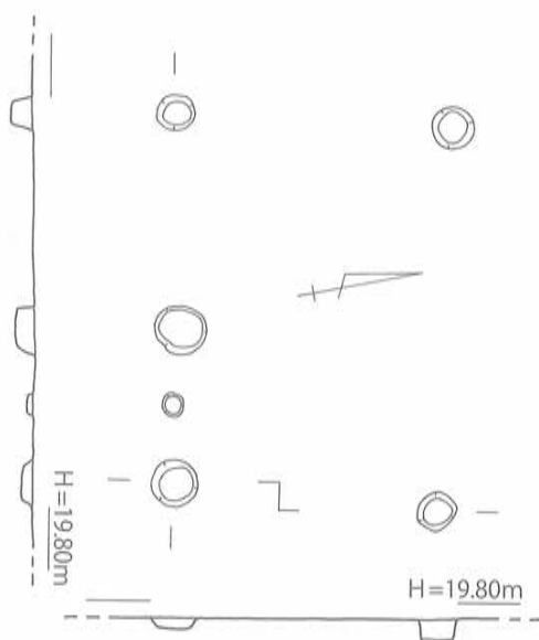
第137図 SB-02 実測図 [1/80]
