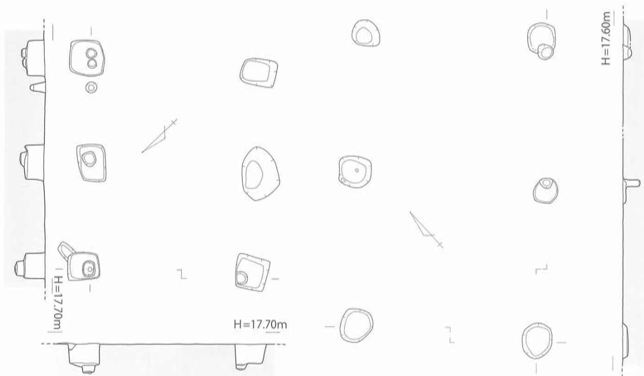
第63図 掘立柱建物B 実測図 [1/80]
