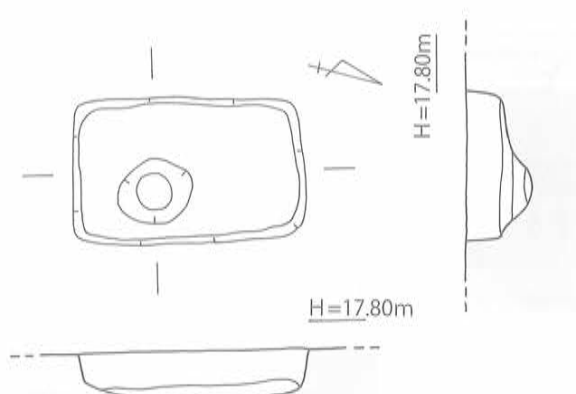
第77図 SK-16 実測図 [1/40]
