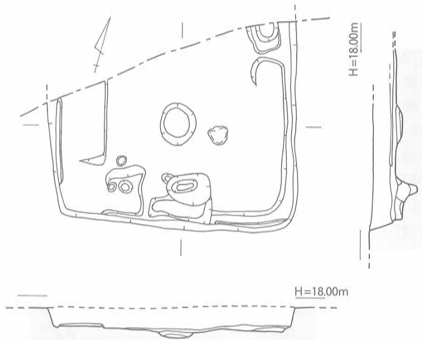
第20図 SB-29 実測図 [1/80]
