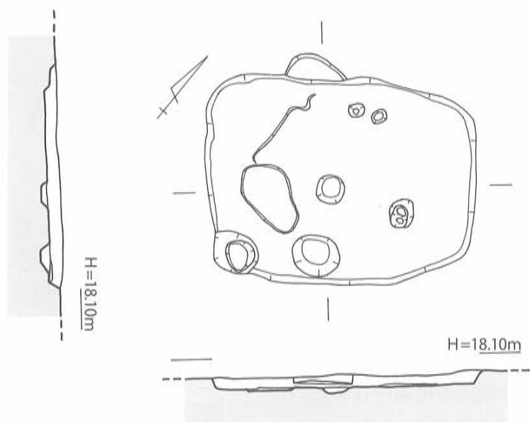
第24図 SB-37 実測図 [1/80]
