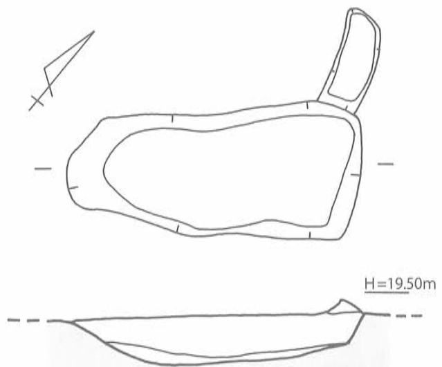
第147図 SK-07 実測図 [1/40]
