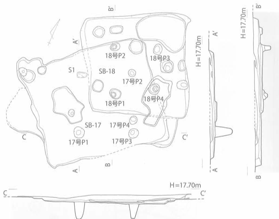
第14図 SB-17・18 実測図 [1/80]
