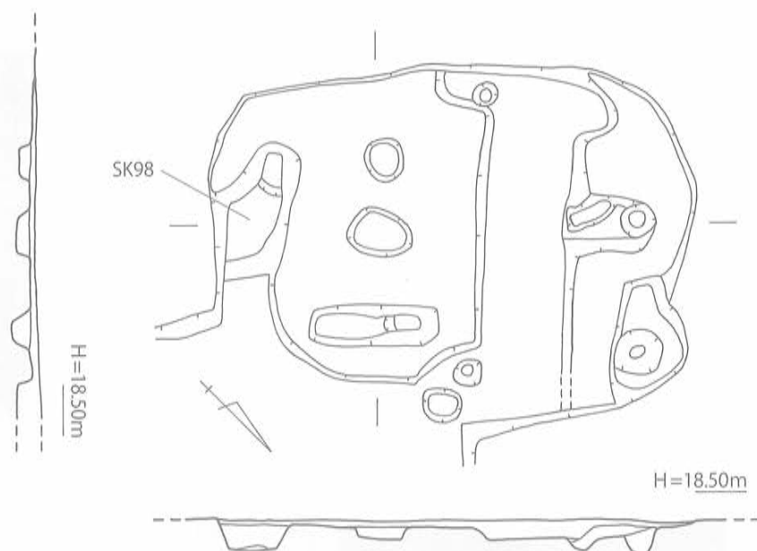
第 4 4 図 SB - 9 2 実測図 [1 / 80]
