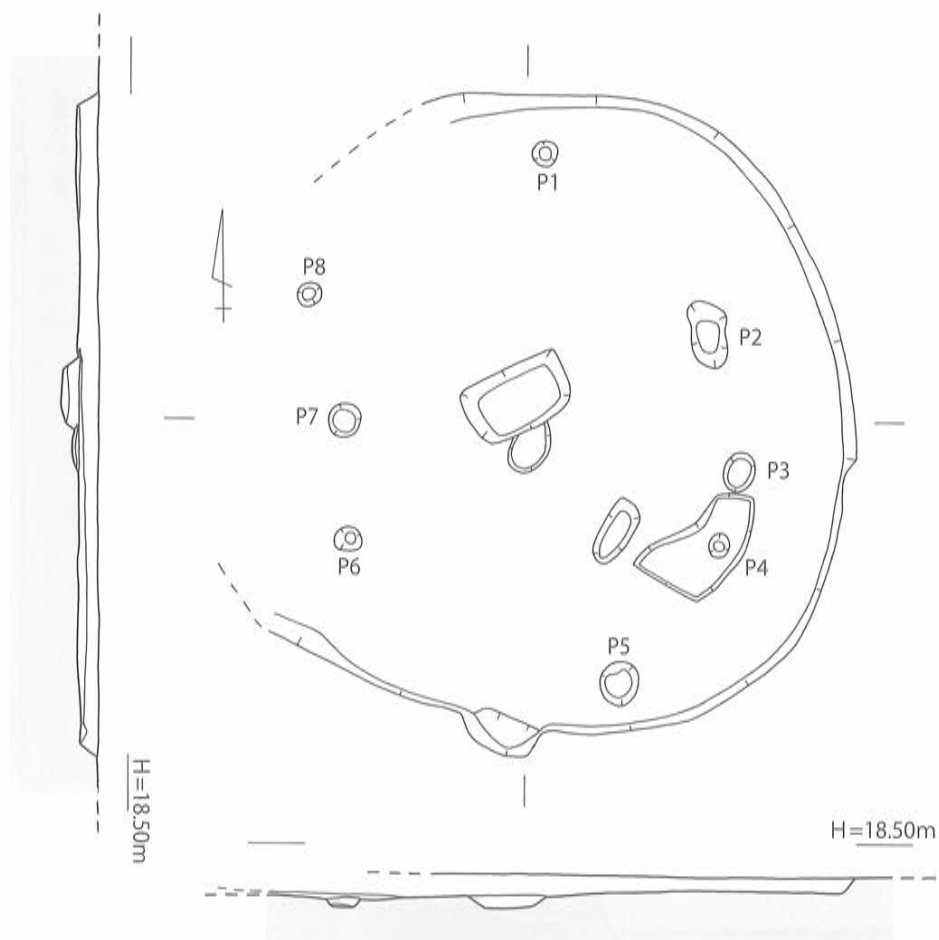
第 5 5 図 SB - 1 1 2 実測図 [1 / 80]
