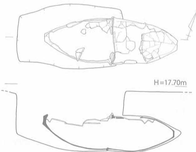
第130図 K-63 実測図 [1/30]
