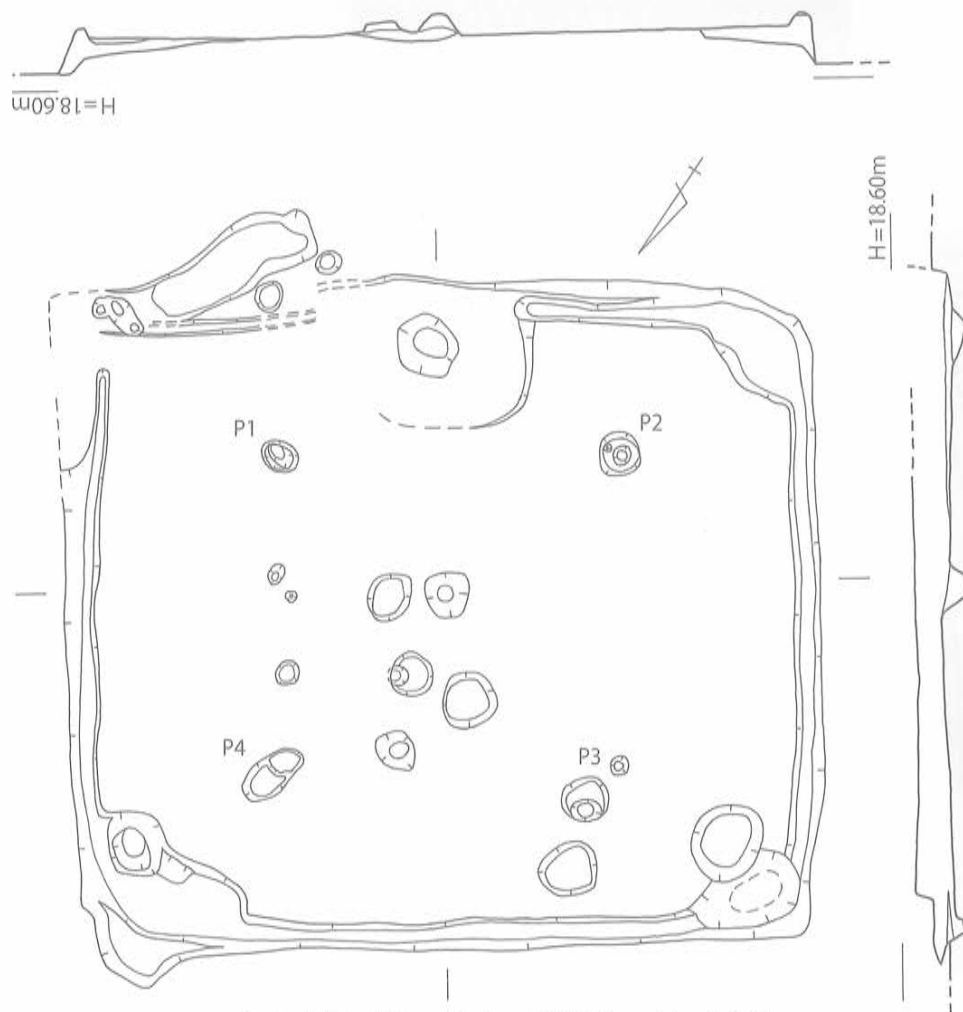
第45図 SB-94 実測図 [1/80]
