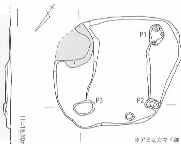
第27図 SB-41 実測図 [1/80]
