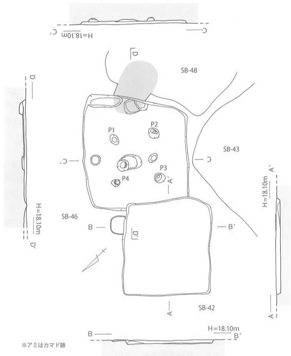
第28図 SB-42・46 実測図 [1/80]
