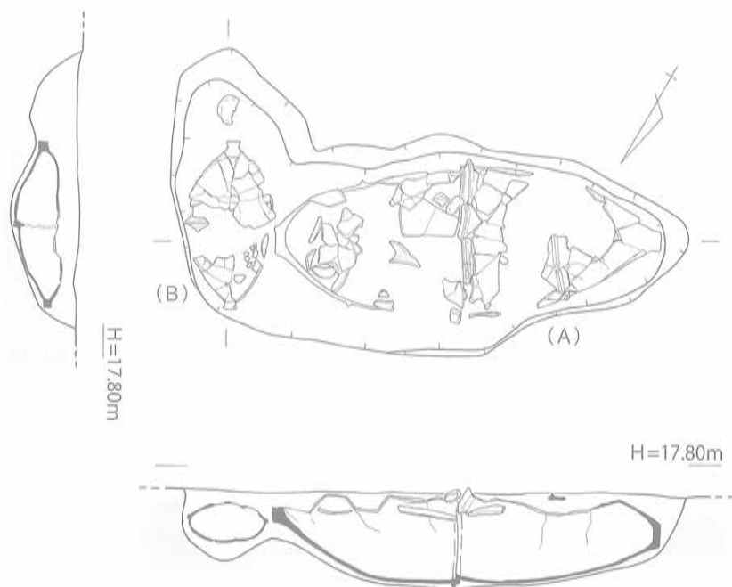
第116図 K-3 (A・B) 実測図 [1/30]
