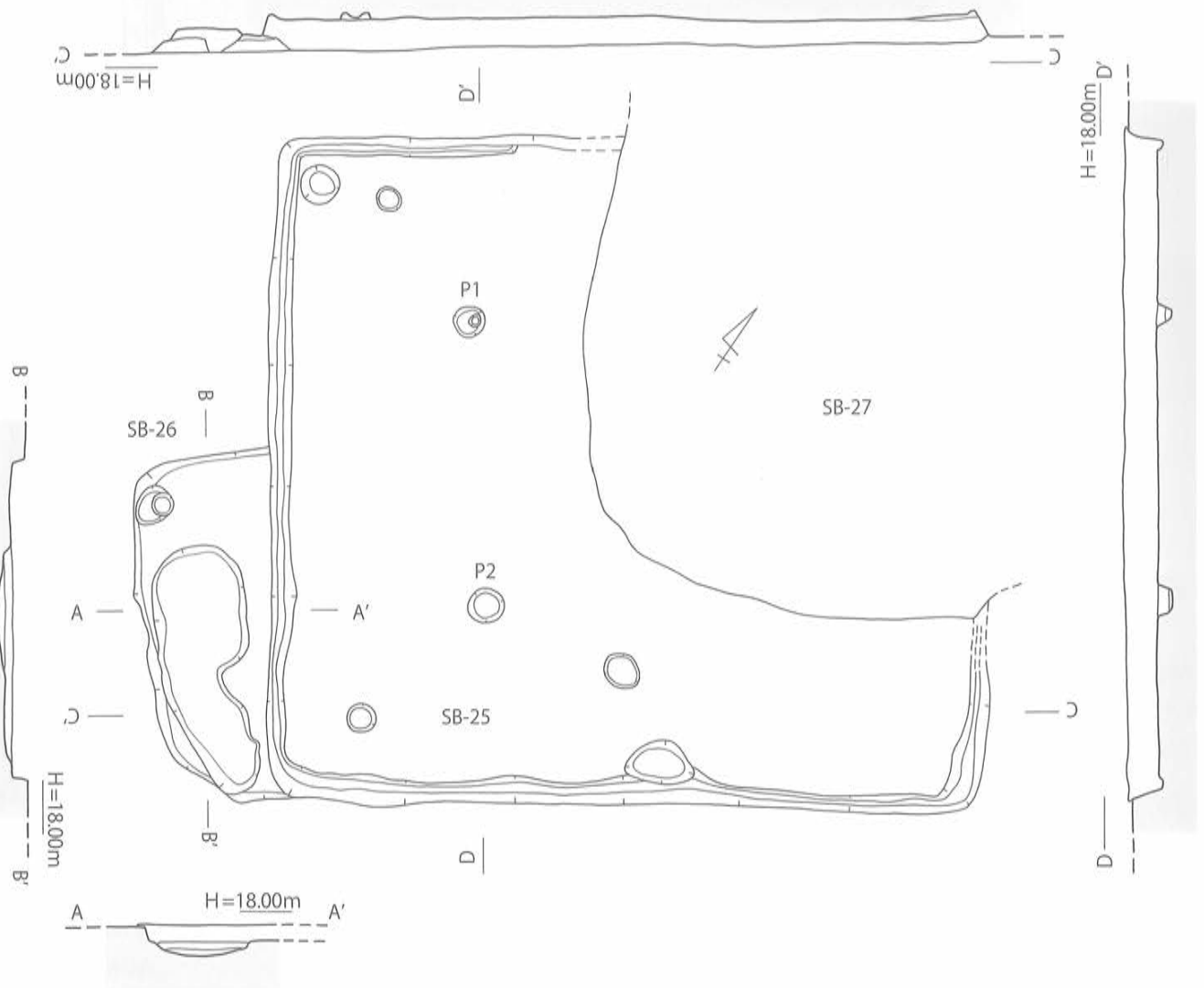
第17図 SB-25・26 実測図 [1/80]
