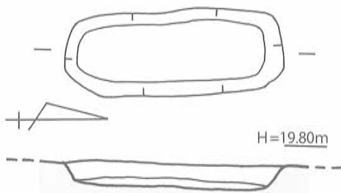
第145図 SK-05 実測図 [1/40]
