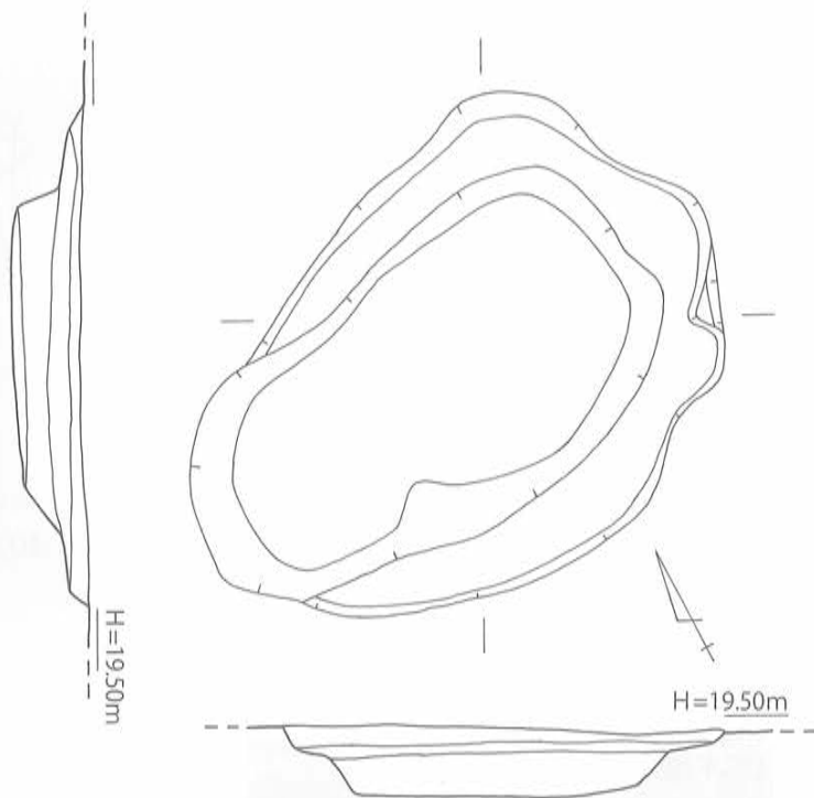
第146図 SK-06 実測図 [1/80]
