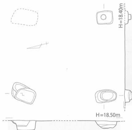
第67図 8号掘立柱建物 実測図 [1/80]
