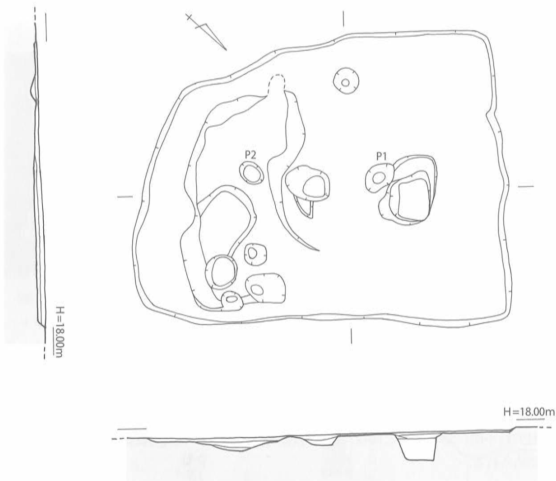
第23図 SB-36 実測図 [1/80]
