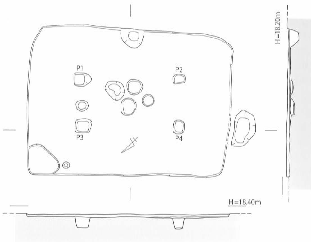
第6図 SB-01 実測図 [1/80]
