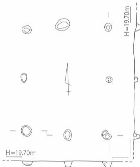
第140図 SB-05 実測図 [1/80]
