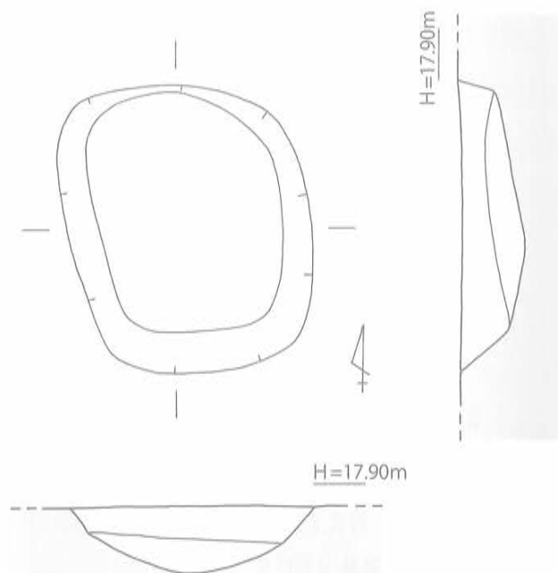
第89図 SK-68 実測図 [1/40]
