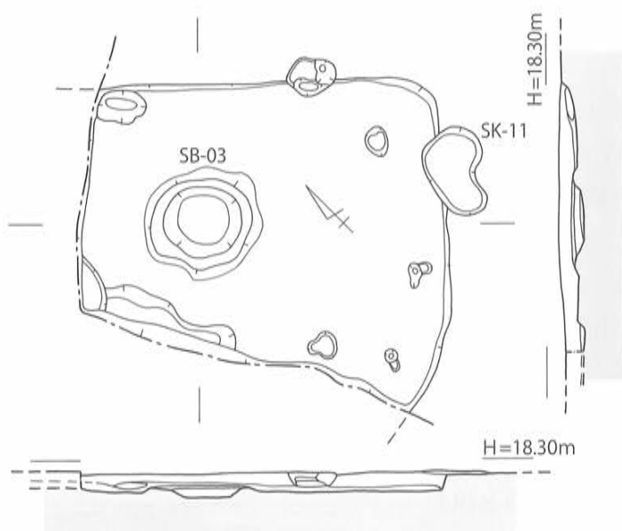
第7図 SB-03、SK-11 実測図 [1/80]
