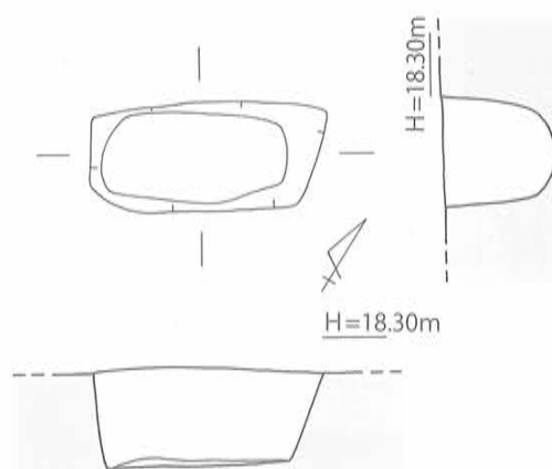
第100図 SK-109 実測図 [1/40]
