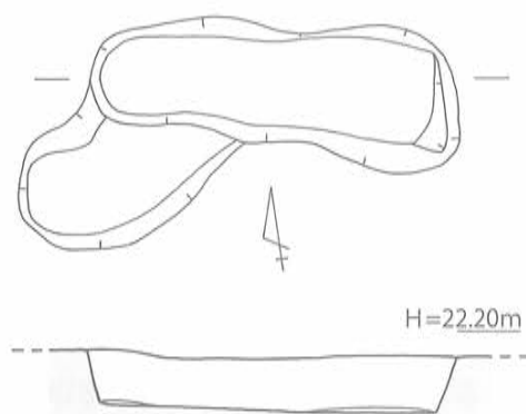
第164図 SK-03 実測図 [1/40]
