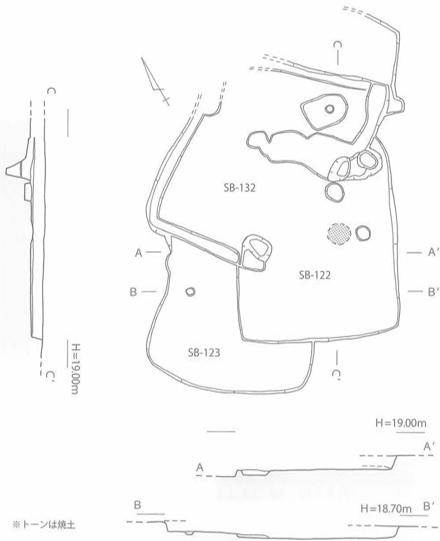
第58図 SB-122・123 実測図 [1/80]
