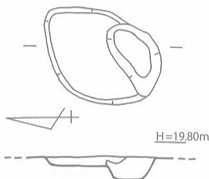
第143図 SK-03 実測図 [1/40]
