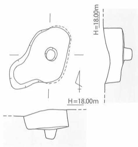
第93図 SK-86 実測図 〔1/40〕
