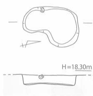
第74図 SK-11 実測図 [1/40]
