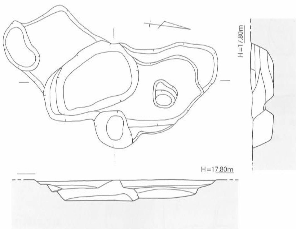
第78図 SK-25 実測図 [1/40]
