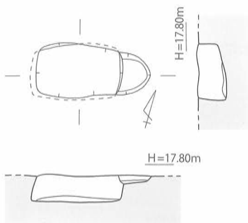
第109図 4号土壙墓 実測図 [1 / 40]
