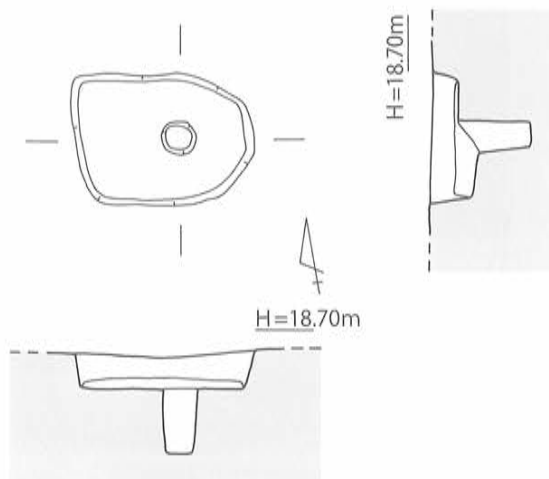
第106図 SK-124 実測図 [1/40]
