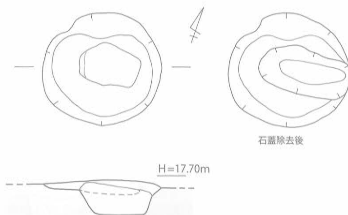
第115図 1号石蓋土墳墓 実測図 [1 / 40]
