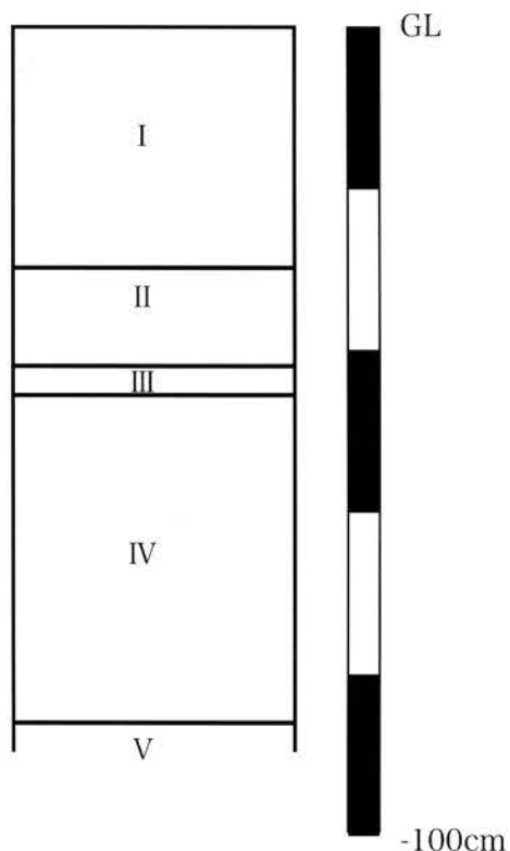
常入遺跡群土層柱状図
