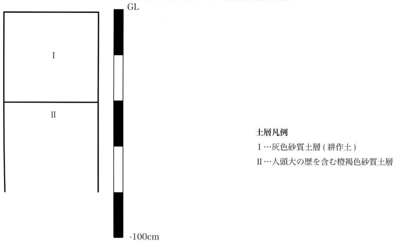
中村Ⅱ遺跡土層柱状図
