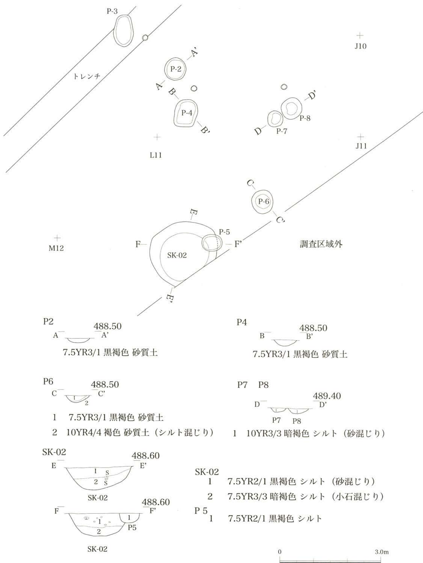
図9 遺構実測図2
