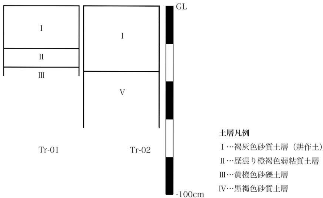
清水坂遺跡土層柱状図
