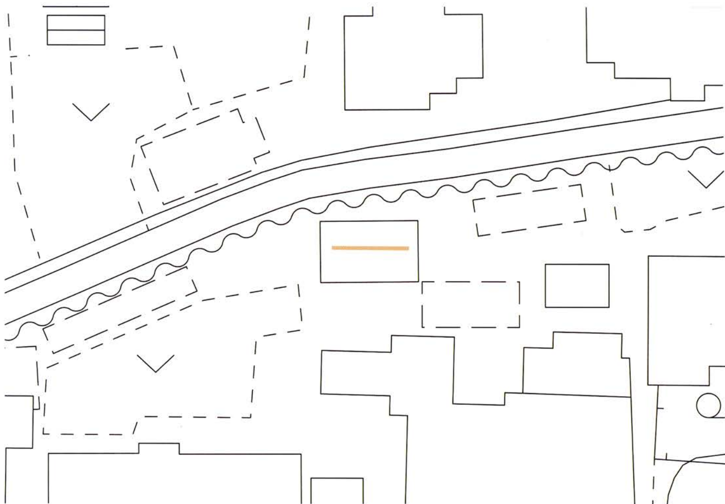
下久根遺跡試掘調査トレンチ設定図 (1/1000)
