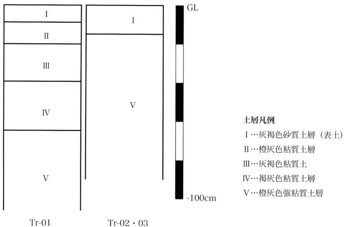
依田条里的遺構・三角遺跡土層柱状図
