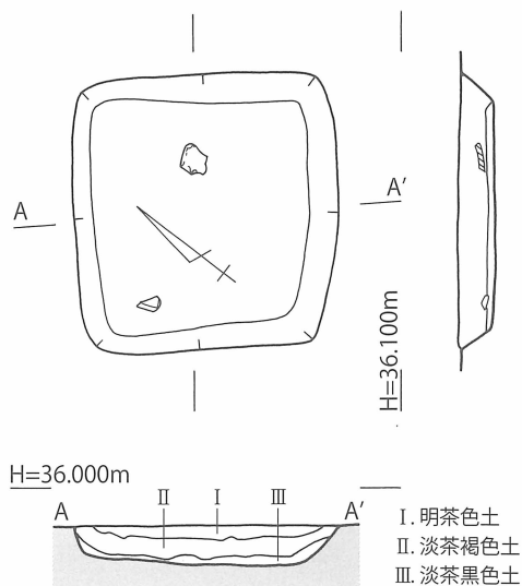
第11図 高島遺跡（5次調査） 12号土壙〔1／40〕
