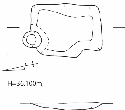
第10図 高島遺跡（5次調査） 11号土壙〔1／40〕
