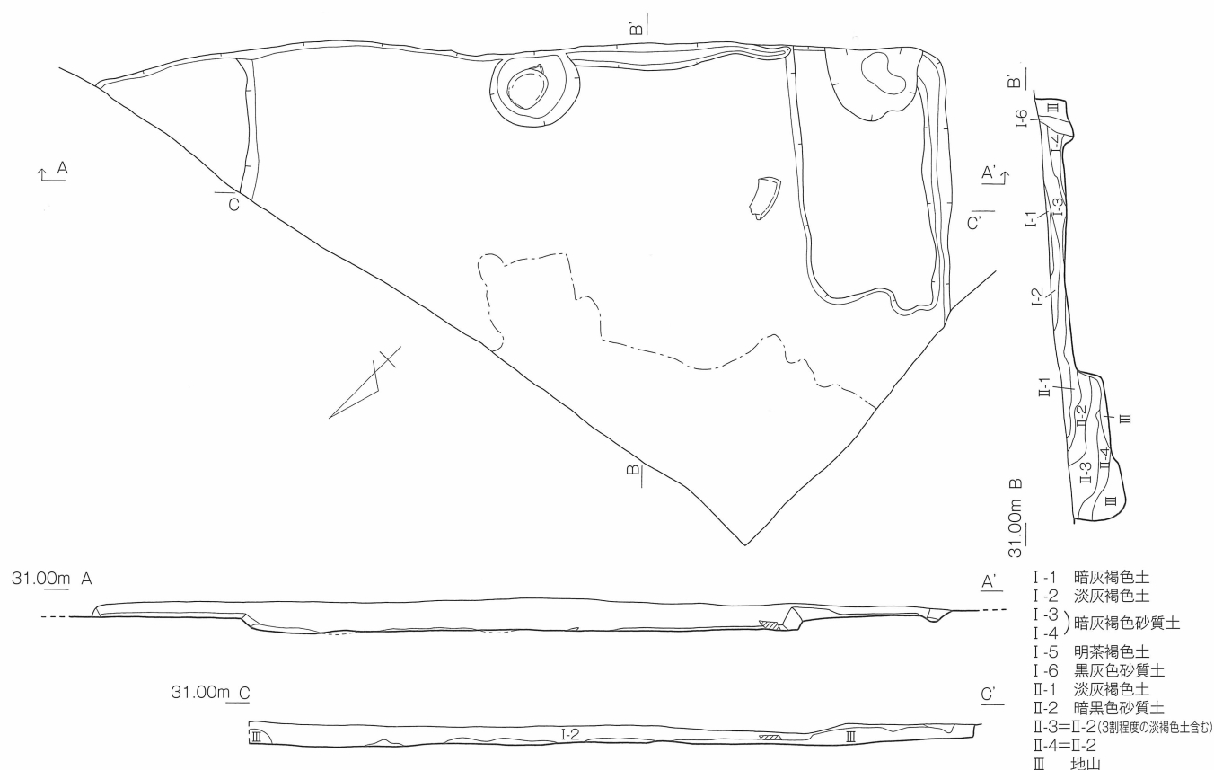
第13図 1号竖穴住居 実測図〔1/60〕
