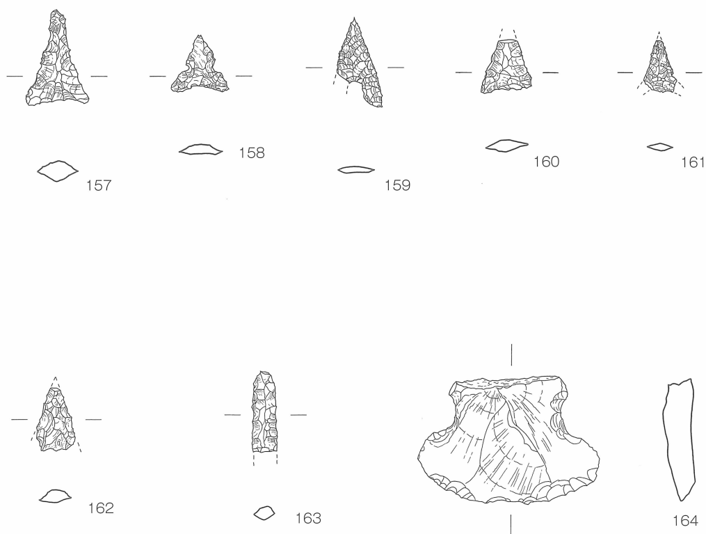
第29図 1～4号竪穴住居，1号不明遺構 出土石製品実測図〔1／2〕
