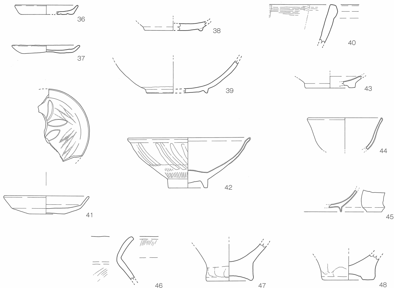
第 11 図 3・4号溝状遺構 出土遺物実測図〔1／3〕
