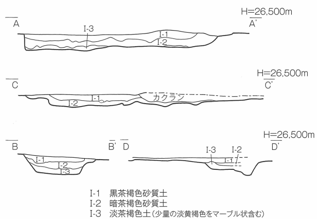
第8図 4号溝状遺構 土層図〔1/60〕
