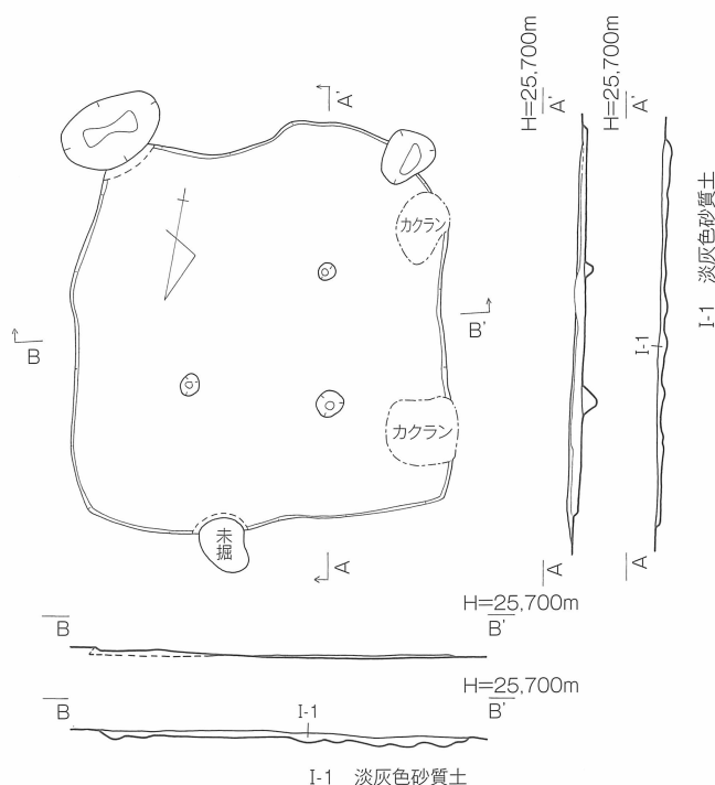
第4図 1号竪穴住居 実測図〔1/60〕
