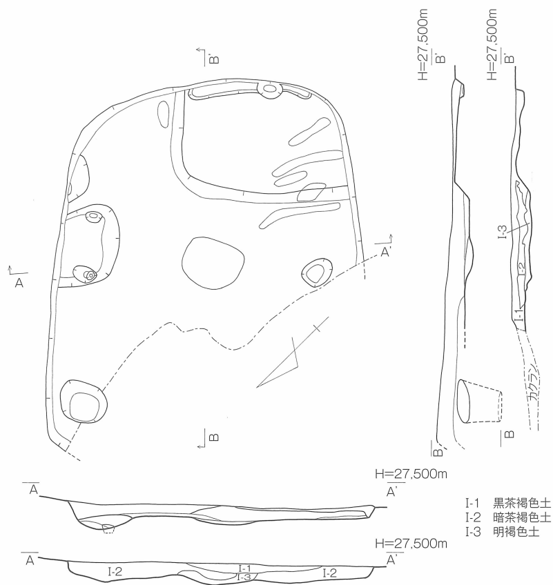
第5図 5号縦穴住居 実測図〔1/60〕
