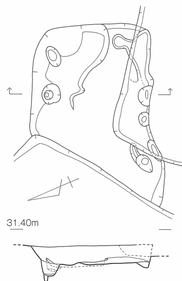
第18図 6号竖穴建物 実測図 〔1/60〕
