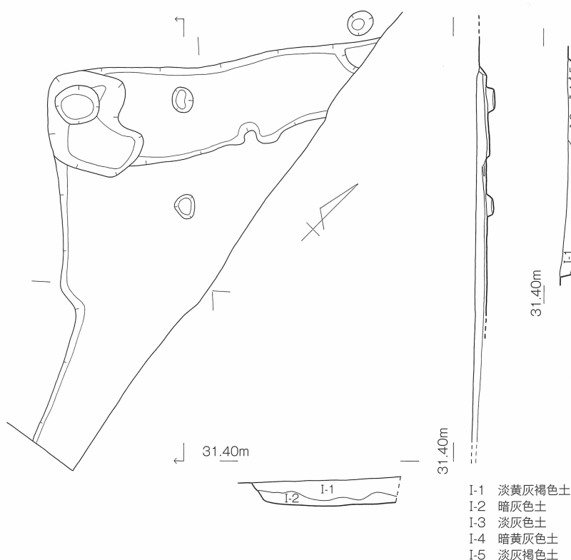
第17図 5号竖穴建物 実測図〔1/60〕
