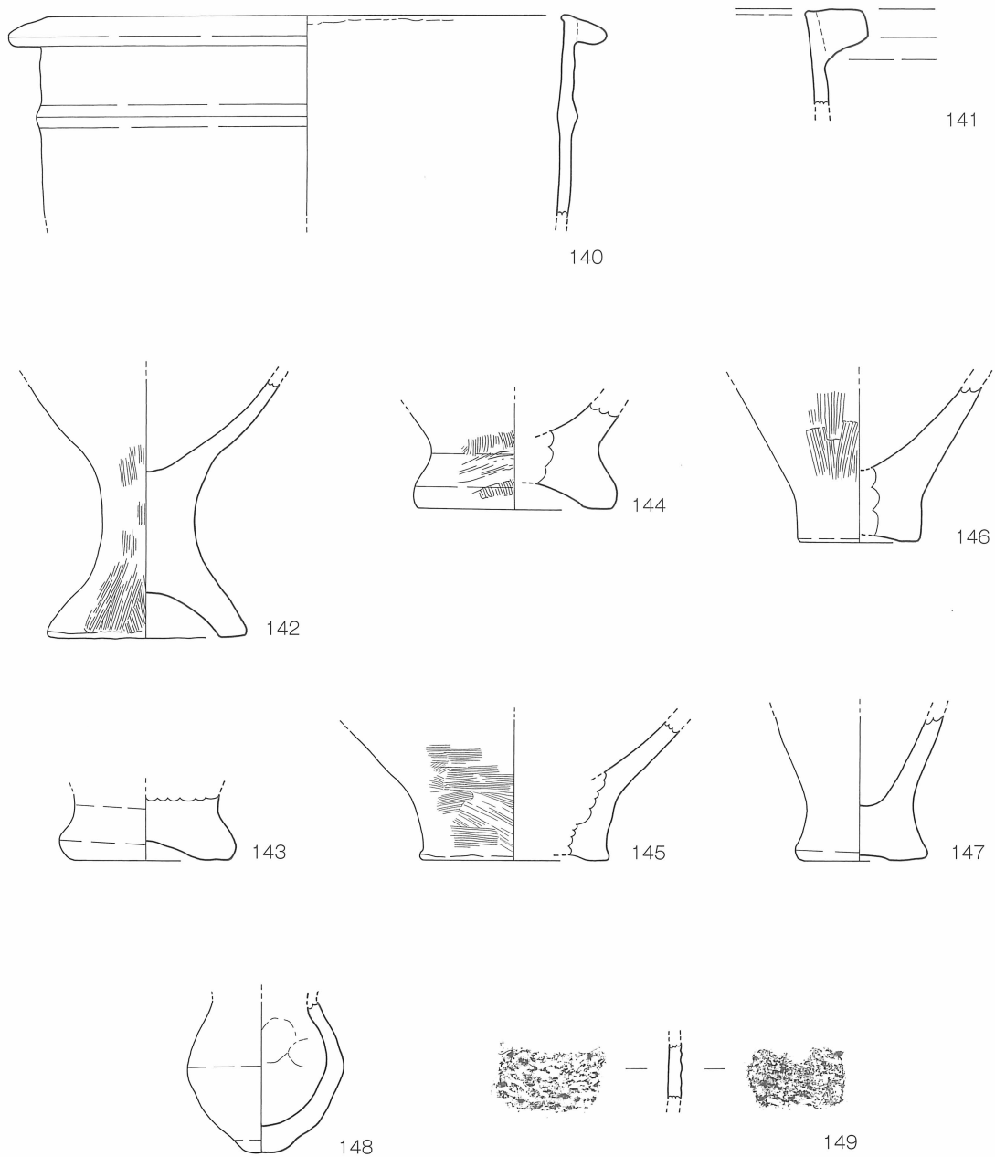
第27図 7号竪穴住居，3～5・8・11～14号不明遺構 出土遺物実測図〔1／3〕
