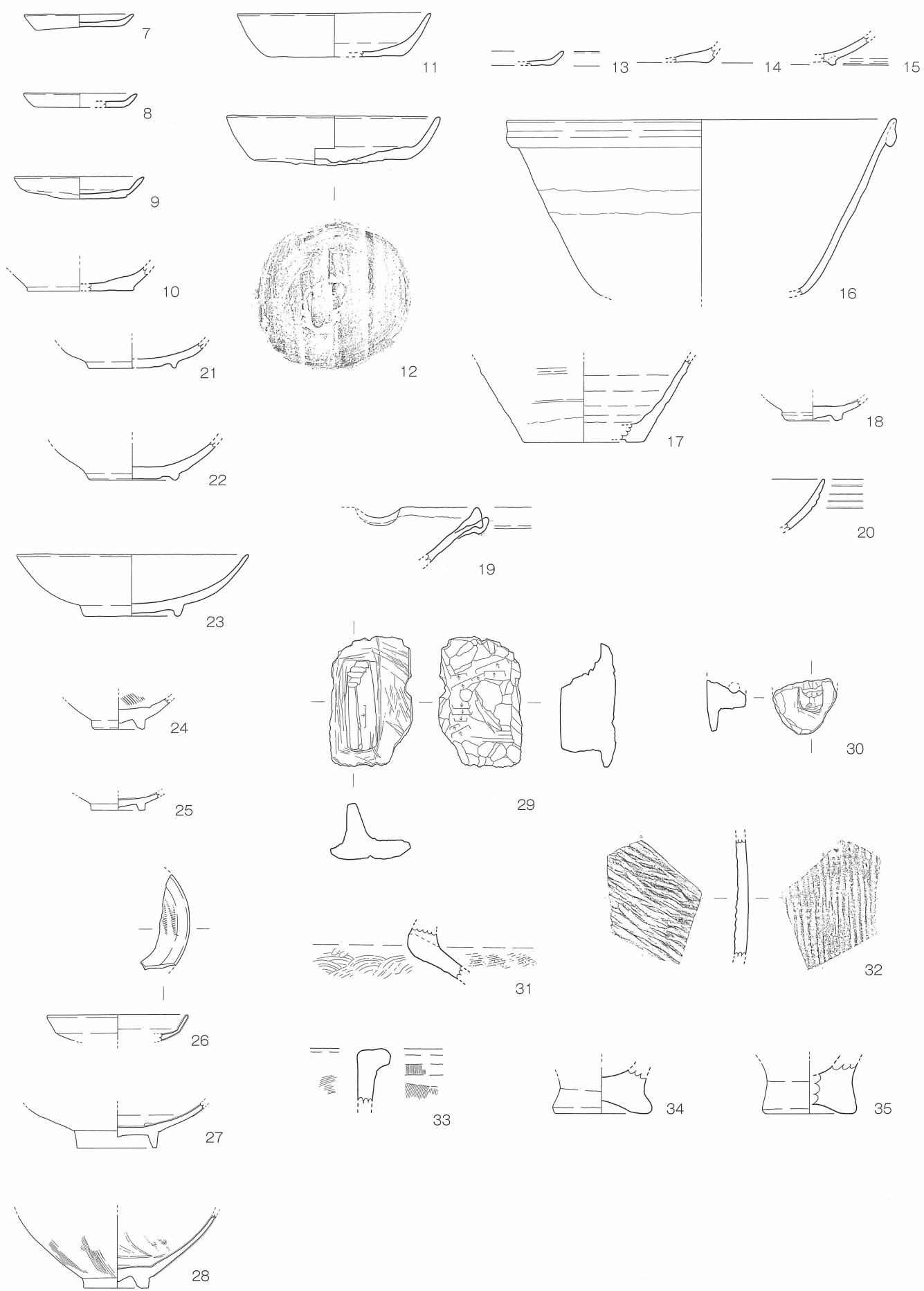
第10図 1号井戸 出土遺物実測図〔1／4〕
