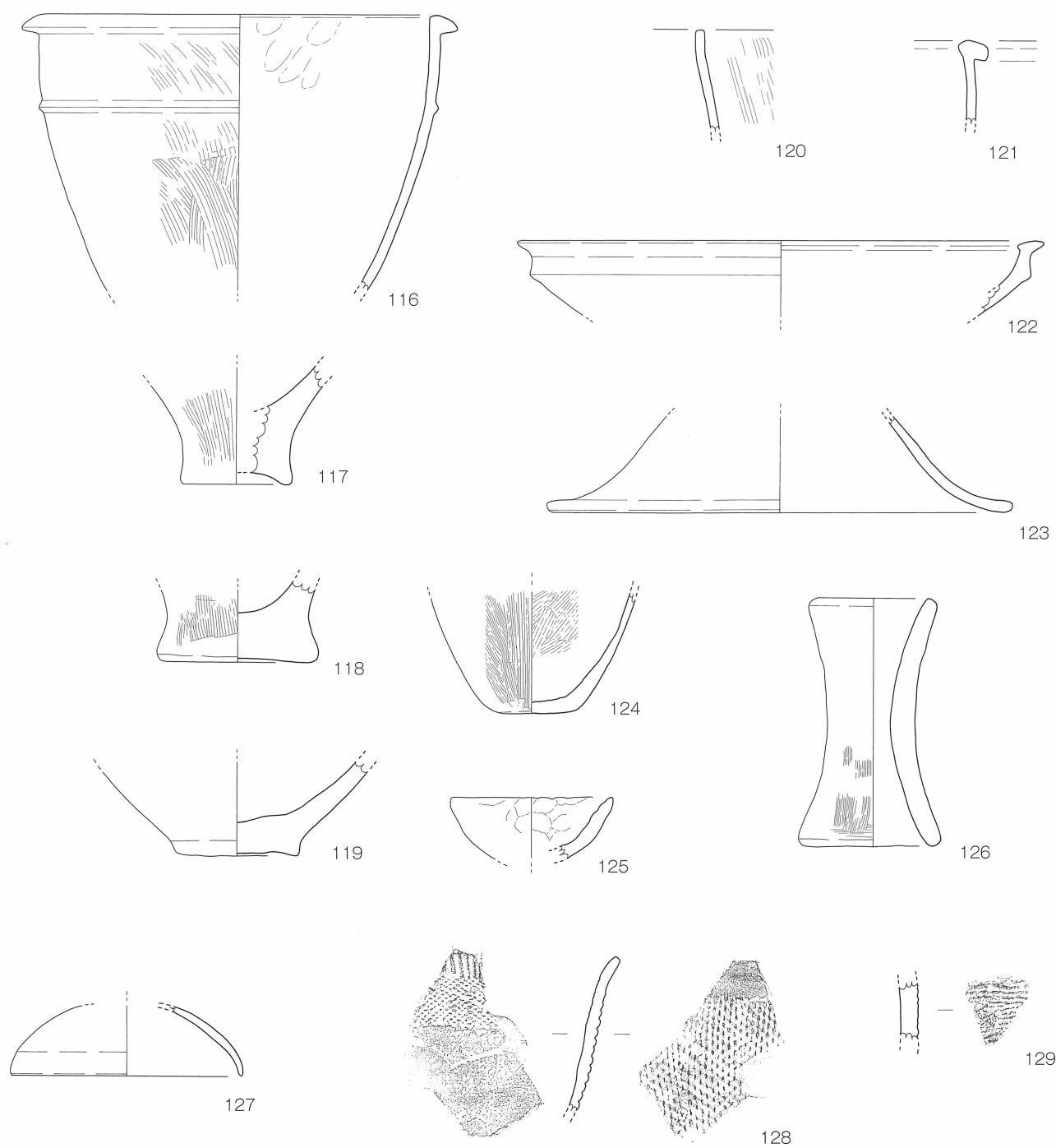
第25図 5・6号竪穴住居 出土遺物実測図〔1／4〕
