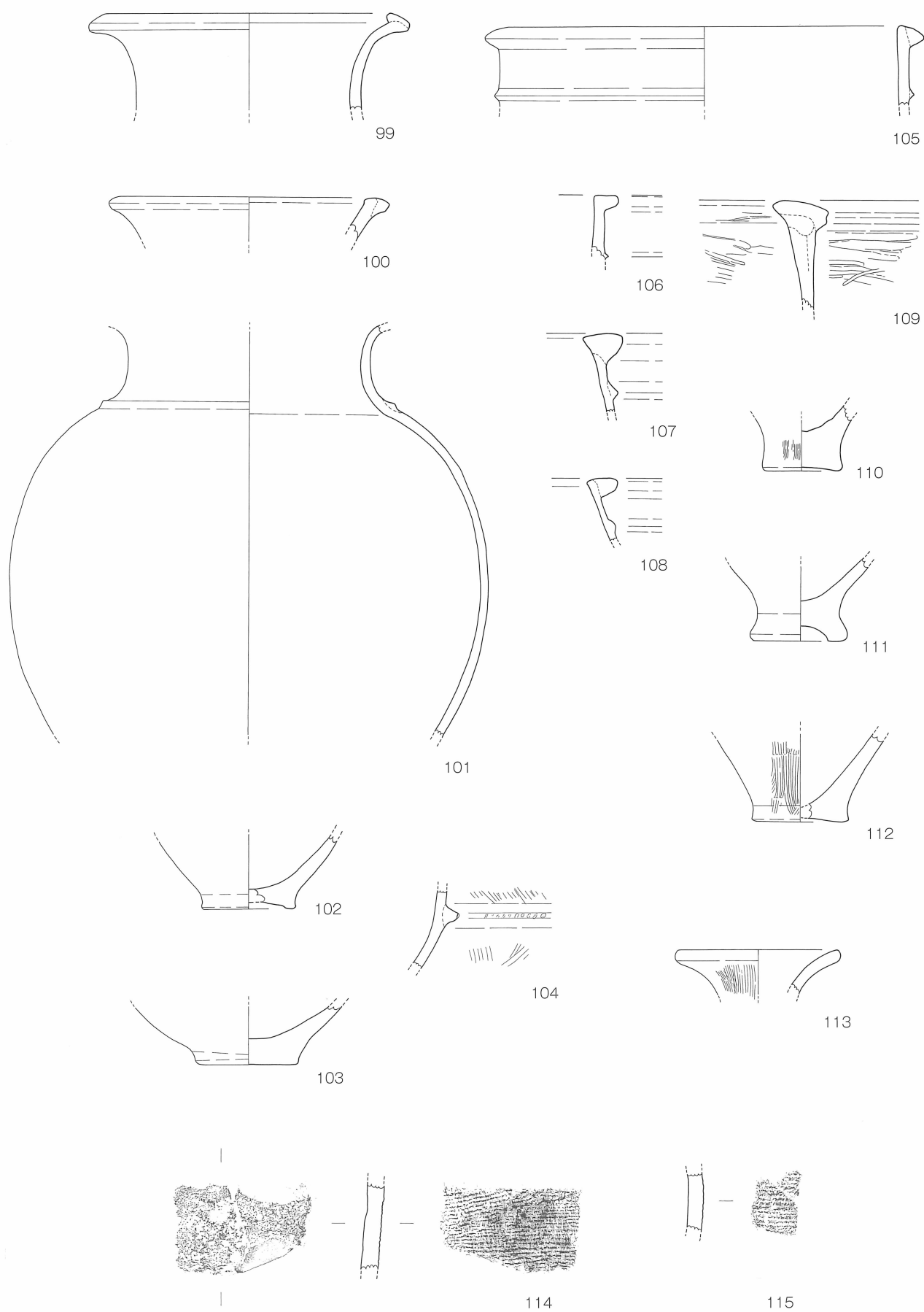
第24図 4号竪穴住居 出土遺物実測図〔1／4〕
