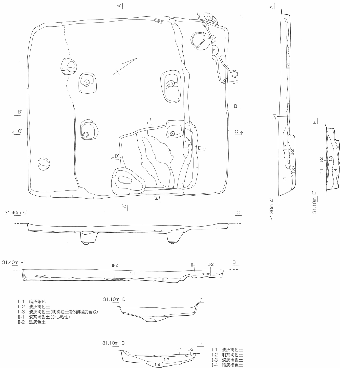
第15図 3号竪穴住居・7号土壌 実測図〔1/60〕
