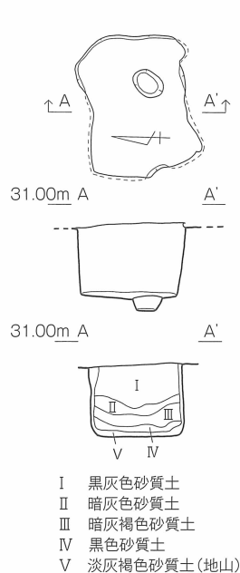
第19図 8号不明遺構 実測図 〔1/60〕
